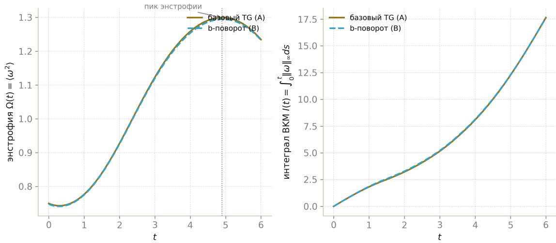
Рис. 8. P5, прогоны А и В: энтрофия \Omega(t) с пиком при t = 4.90 (слева) и огибающая Била-Като-Майды I(t) (справа). Траектории статистически неразличимы.
