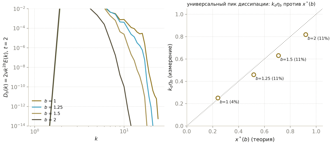
Рис. 9. P5, b -семейство: оболочечная диссипация D_b(k) = 2\nu k^{2b} E(k) при t = 2 с измеренными пиками (слева) и универсальный коллапс k_d \eta_b против x^*(b) (справа); отклонения 4-11 % ограничены разрешением и подписаны у точек.
