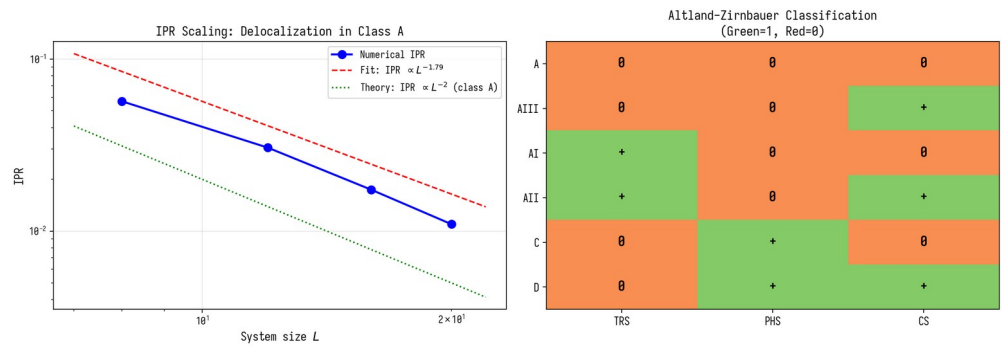
Рис. 17. 4.1.1 Топологическая классификация Альтланда-Зирнбауэра
