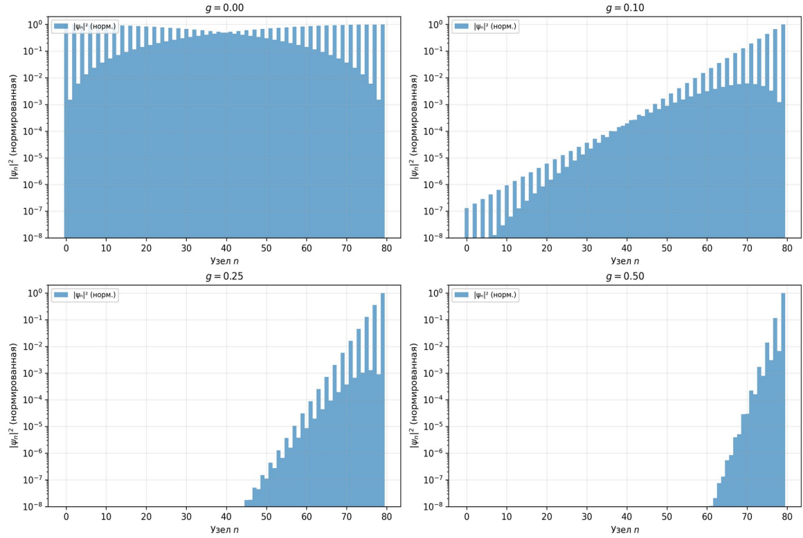
Рис. 8.5 · Skin effect: локализация волновой функции |\psi_n|^2 на границе системы при g \neq 0 . Длина локализации \xi \propto 1/g .
