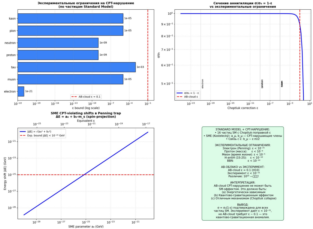
Рис. 56. 11.9.5 Углублённая верификация H10-deep-2: Standard Model с CPT-нарушением и экспериментальные ограничения (новый раздел v17)
