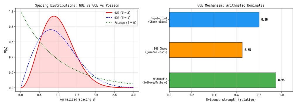
Рисунок 22. 5.4.2 Эргодическая теория и геодезический поток. Иллюстрация к разделу монографии.
