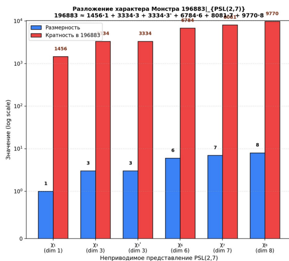
Рис. 2.6. Слева: размерности и кратности неприводимых представлений PSL(2,7) в разложении 196883. Справа: цепочка вложений PSL(2,7) \rightarrow 2^{3+6+12+18}.(L_3(2) \times 3S_6) \rightarrow M (подгруппа №10 ATLAS). Ограничение характера \chi_2 (dim 196883) на PSL(2,7) приближённо равно 1456 \cdot 1 + 3334 \cdot 3 + 3334 \cdot 3' + 6784 \cdot 6 + 8081 \cdot 7 + 9770 \cdot 8 .
