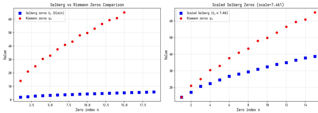
Рисунок 2.1. Сравнение нулей Селберга (кватрика Клейна) и нулей Римана.
