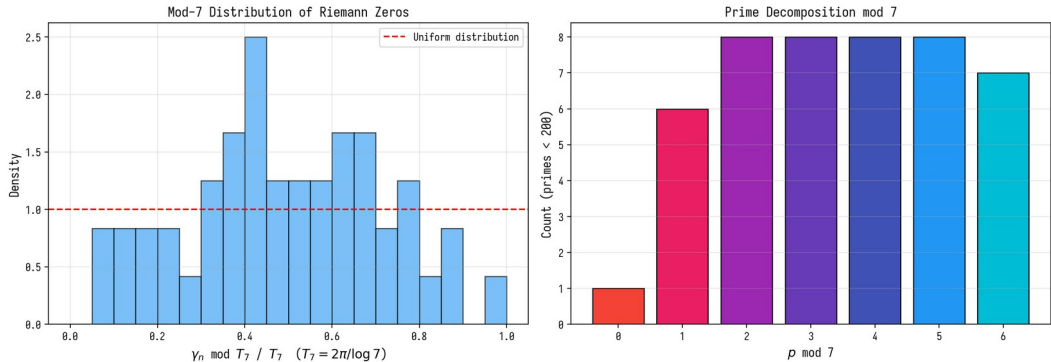
Рисунок 8.2. Mod-7 распределение нулей Римана и простых чисел.
