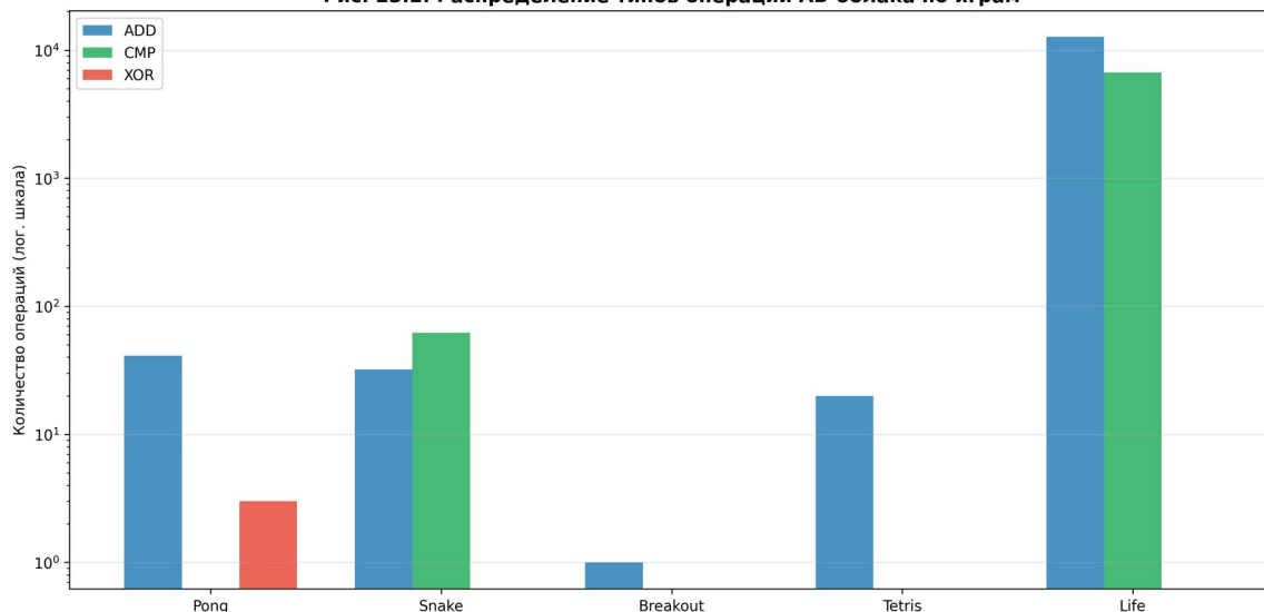
Рис. 23.2. Распределение типов операций АВ-облака по играм (логарифмическая шкала).
