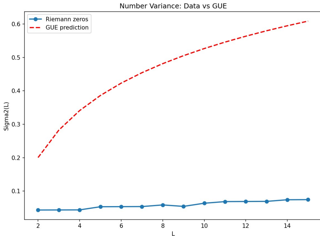
Рисунок 11.3. Числовая дисперсия \Sigma^2(L) : нули \zeta vs GUE-прогноз.
