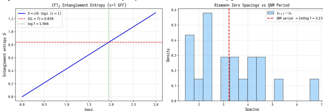
Рисунок 5.3. Энтропия запутывания и QNM-период.
