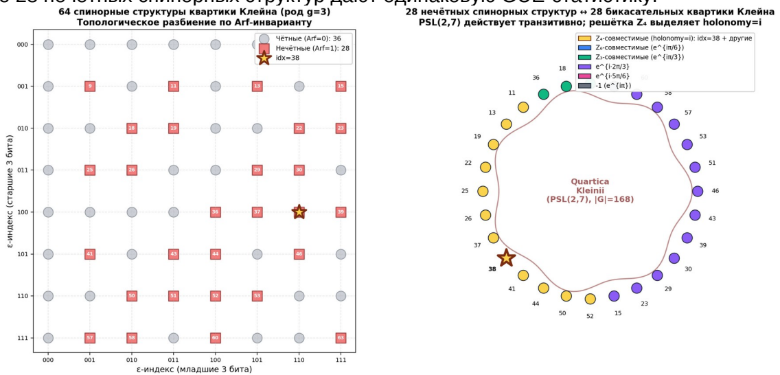
Рис. 3.3. Слева: 64 спинорные структуры квартики Клейна, окрашенные по \text{Arf} -инварианту (36 чётных + 28 нечётных); idx=38 выделен звездой. Справа: 28 нечётных структур как бикасательные на схематичной квартике Клейна; цвет кодирует Z_4 -совместимость голономии. PSL(2,7) действует транзитивно; Z_4 -подгруппа квадратной решётки выделяет структуры с голономией i .
