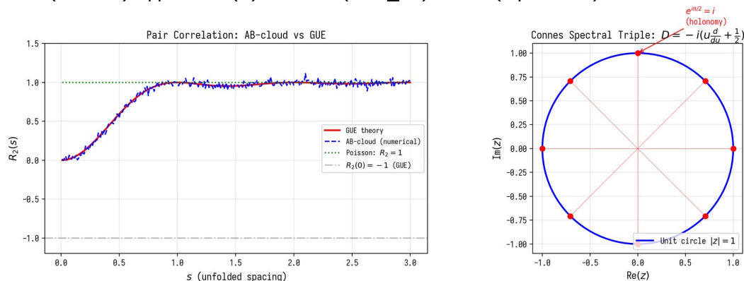
Рисунок 6.1. Парная корреляция АВ-облако vs GUE и спектральная реализация Конна.
