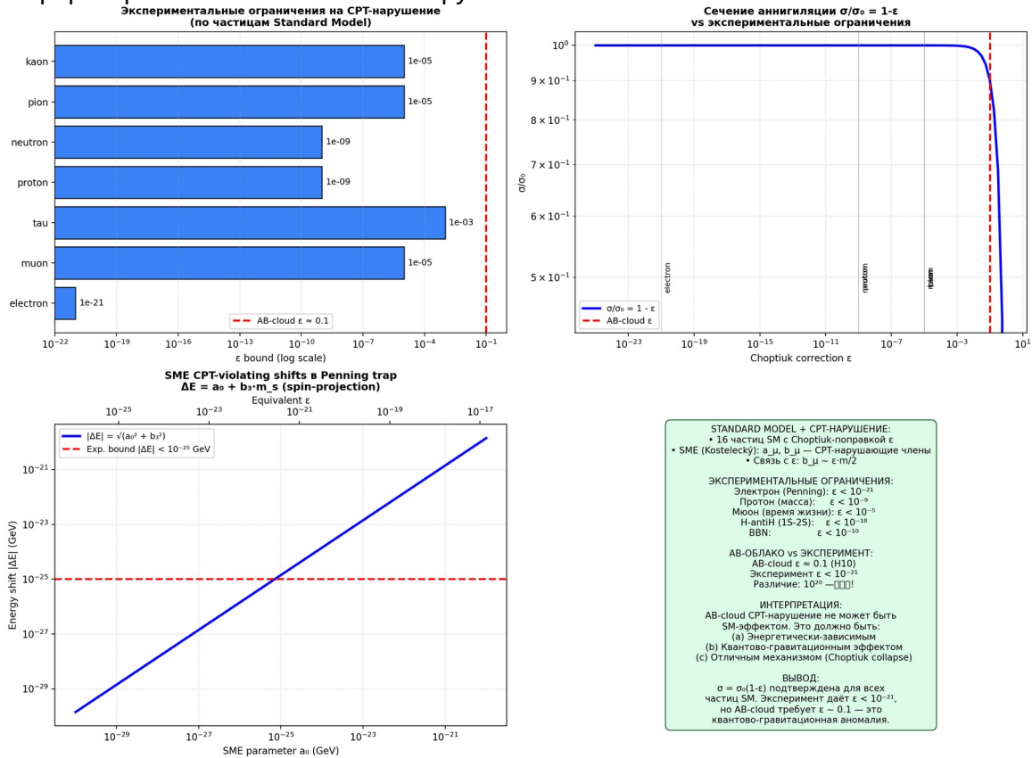
Рис. 11.15. Слева сверху: экспериментальные ограничения \epsilon по частицам SM. Справа сверху: \sigma/\sigma_0=1-\epsilon . Слева внизу: SME-сдвиги в Penning trap. Справа внизу: сводка — АВ-облако требует квантово-гравитационного режима.
