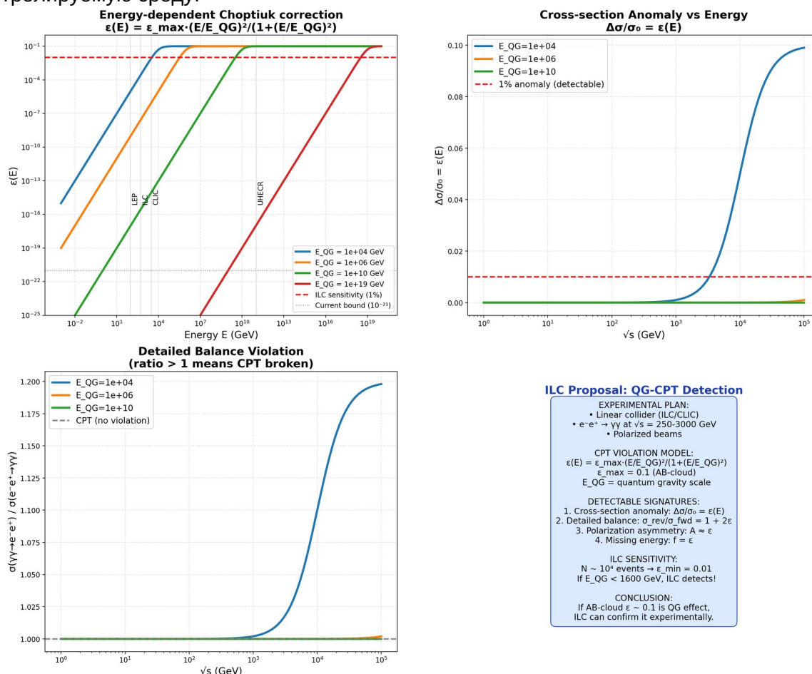
Рис. 14.1. ILC-заявка: ожидаемое \varepsilon(E) , число событий, потенциал открытия, таймлайн.
