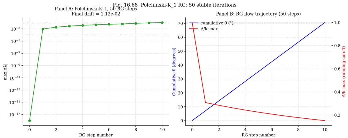
Рис. 16.68. 50 шагов Polchinski- K_1 : drift (слева) и траектория RG-потока — cumulative \theta и бегающий cutoff \Lambda(\theta)/k_{\max} (справа).
