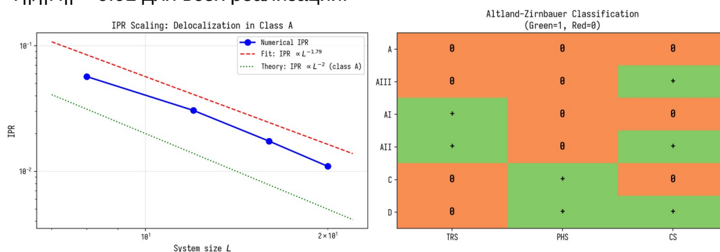
Рисунок 4.1. IPR-скейлинг и классификация Альтланда-Зирнбауэра.
