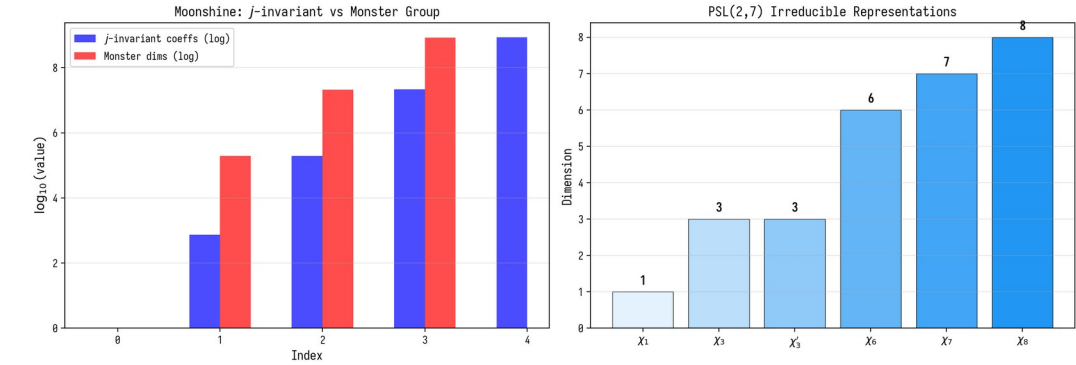
Рисунок 2.4. Moonshine-связь: j-инвариант и группа Монстр; представления PSL(2,7).
