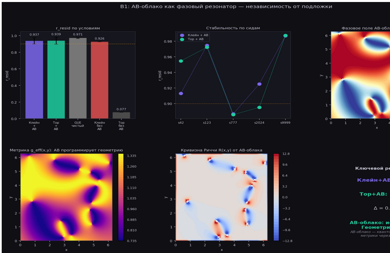
Рисунок 2. B1: r_{\text{resid}} для разных подложек. Клейн+АВ \approx Тор+АВ. Тор без АВ = 0.077.
