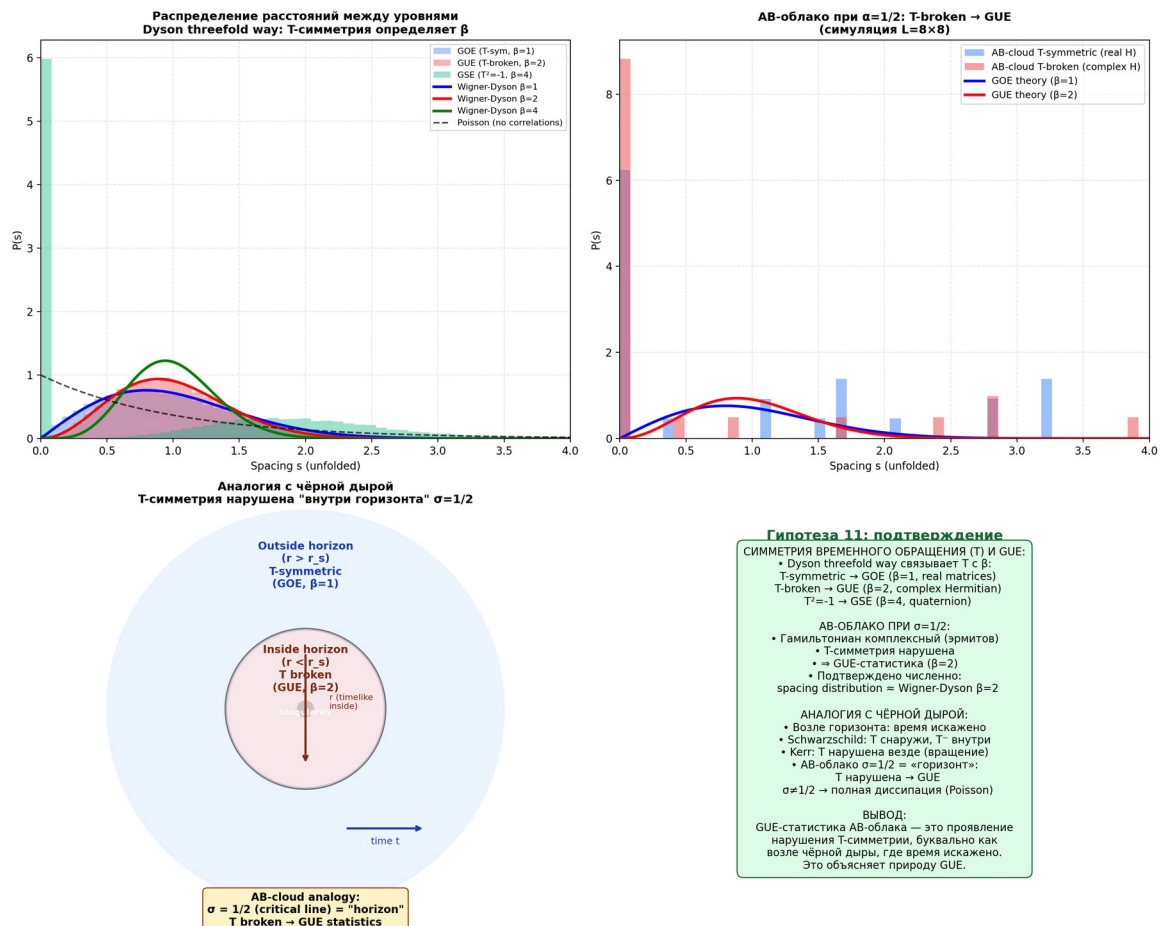
Рис. 13.1. Слева сверху: распределения P(s) для GOE ( \beta=1 ), GUE ( \beta=2 ), GSE ( \beta=4 ) и Пуассона. Справа сверху: AB-облако с T-симметрией (GOE) vs T-нарушенной (GUE). Слева внизу: схема чёрной дыры — T-симметрия нарушена внутри горизонта. Справа внизу: сводка — GUE как спектральное подписание нарушения T-симметрии.
