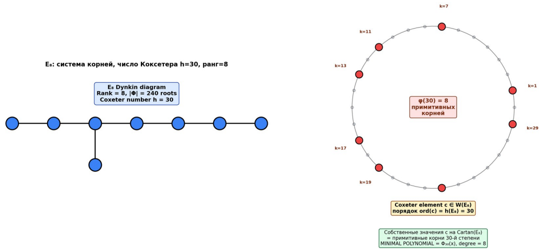
Рис. Е.4. Слева: диаграмма Дынкина E_8 (ранг 8, число Кокстера h=30 ). Справа: примитивные корни 30-й степени из единицы — собственные значения элемента Кокстера E_8 . Минимальный многочлен — \Phi_{30}(x) степени 8 = \text{rank}(E_8) = \dim(\chi_8(\text{PSL}(2,7))) .
