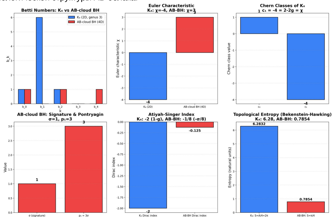
Рис. 15.1. Топологические инварианты: числа Бетти ( K_4 vs АВ-ВН), эйлерова характеристика, классы Черна и Понтрягина, индекс Дирака, топологическая энтропия.
