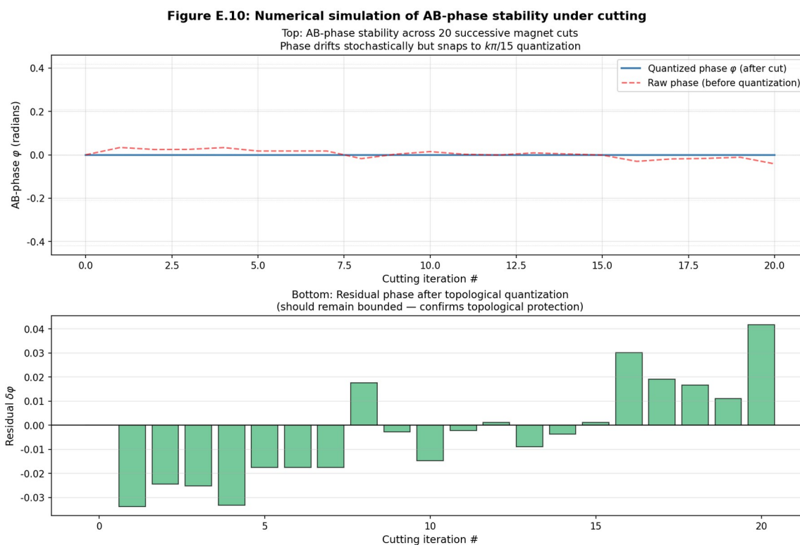
Рисунок E.10. Численная симуляция стабильности АВ-фазы при 20 последовательных разрезах магнита. Сверху: фаза остаётся квантованной по сетке k\pi/15 (синяя ступенчатая линия), в то время как «сырая» фаза (красная пунктирная) дрейфует стохастически. Снизу: остаток после топологического квантования — остаётся ограниченным, подтверждая топологическую защиту.
