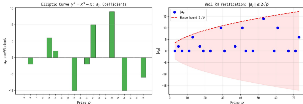
Рисунок 7.3. RH Вейля: a_p и граница Хассе для y^2 = x^3 - x .
