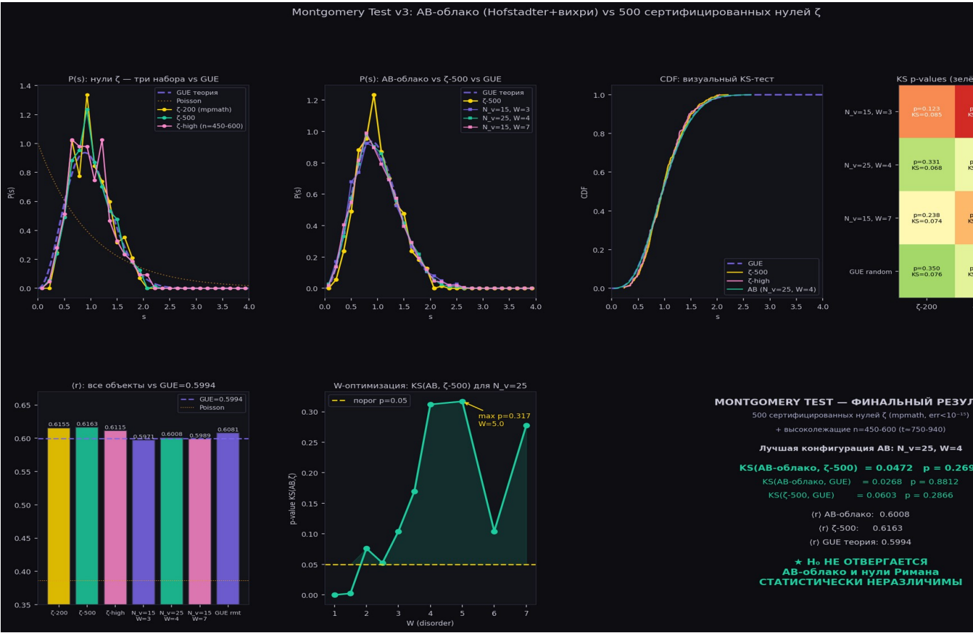
Рисунок 4. Итоговый тест Монтгомери: АВ-облако vs 500 сертифицированных нулей \zeta . H_0 не отвергается.
