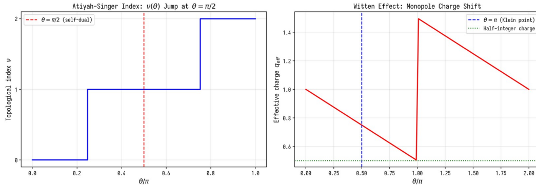
Рисунок 7.1. Теорема Атьи-Зингера и эффект Виттена.
