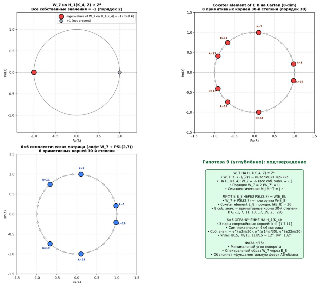
Рис. 6.5. Слева сверху: W_7 = -I_6 на H_1(K_4, Z) (все собственные значения -1 ). Справа сверху: 8 примитивных корней 30-й степени — собственные значения элемента Коксетера E_8 на Картане. Слева внизу: 6×6 ограничение с 3 парами корней (углы 12°, 84°, 132°). Справа внизу: сводка — фаза \pi/15 как минимальный угол вращения лифта W_7 к E_8 .
