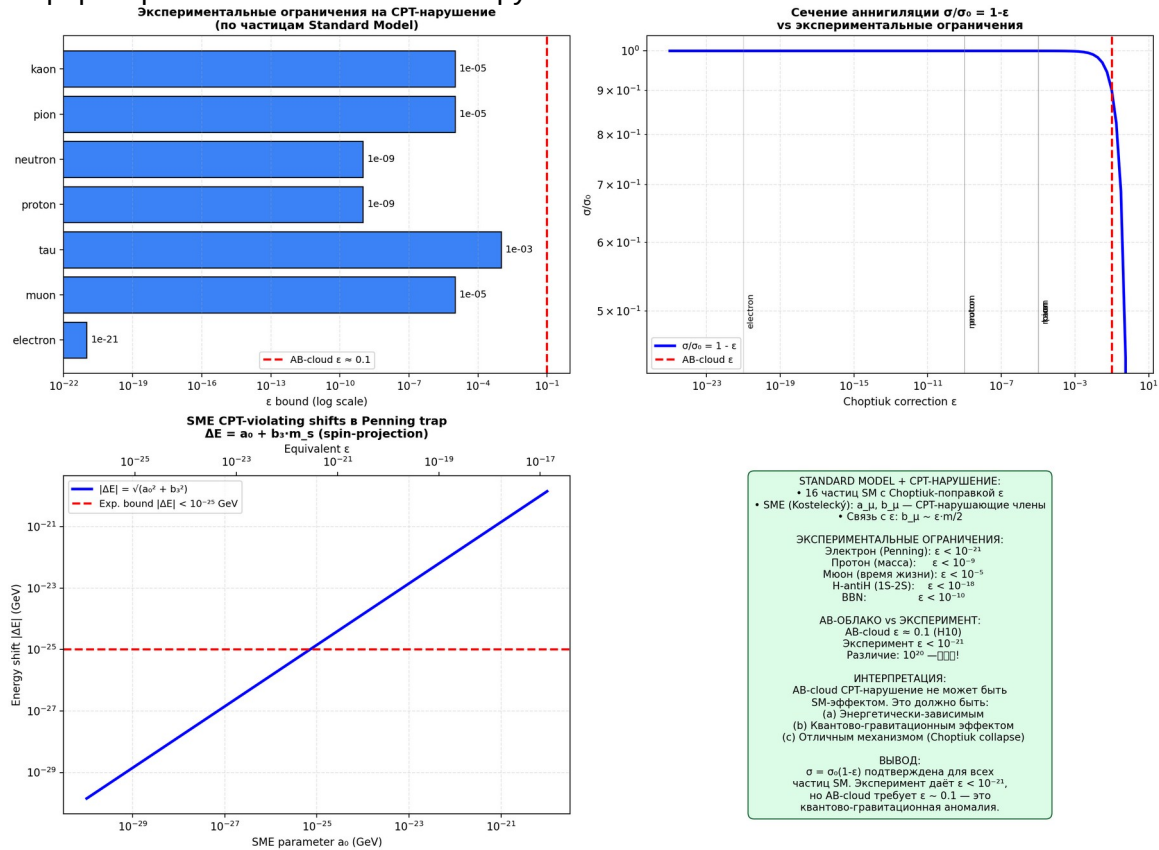
Рис. 11.15. Слева вверху: экспериментальные ограничения \epsilon по частицам SM. Справа вверху: \sigma/\sigma_0=1-\epsilon . Слева внизу: SME-сдвиги в Penning trap. Справа внизу: сводка — АВ-облако требует квантово-гравитационного режима.
