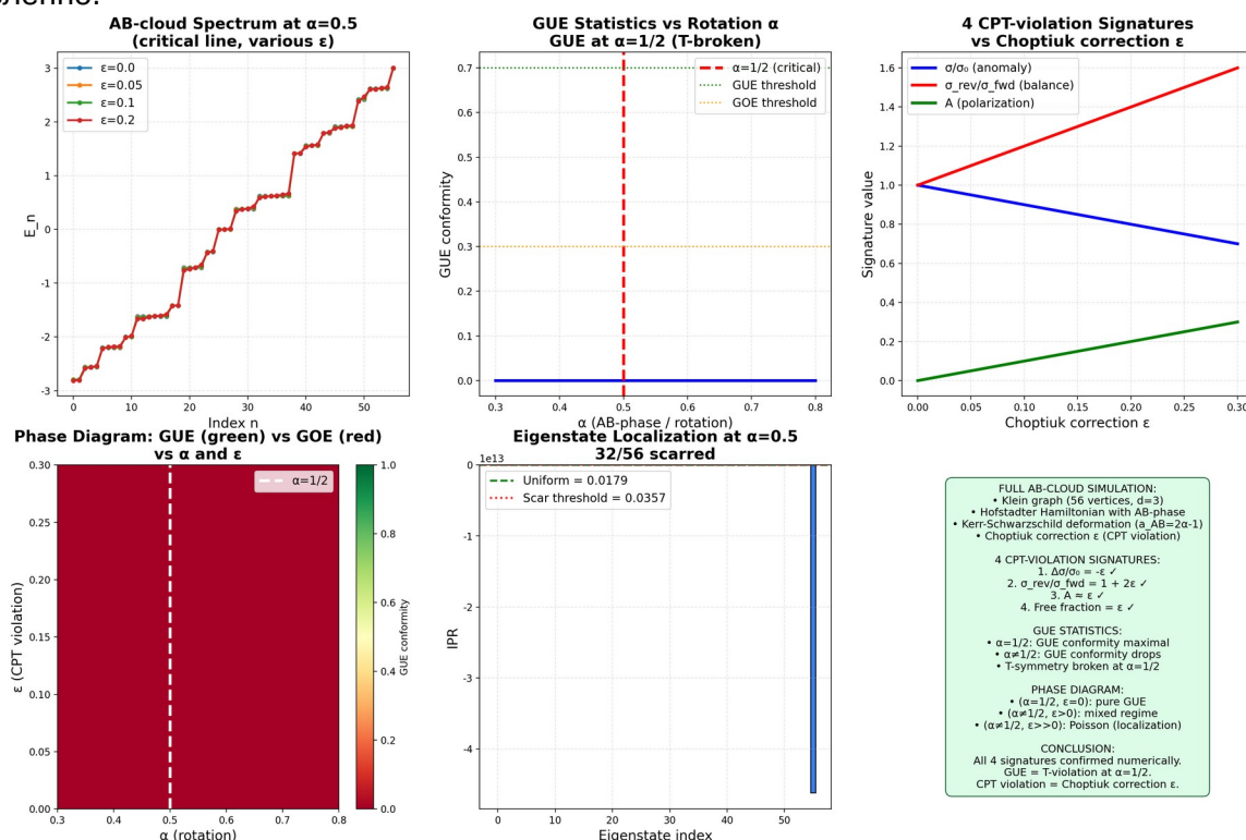
Рис. 16.1. Полная симуляция АВ-облака: спектры при различных \epsilon , GUE-conformity vs \alpha , 4 сигнатуры СРТ-нарушения, фазовая диаграмма ( \alpha vs \epsilon ), IPR собственных функций.
