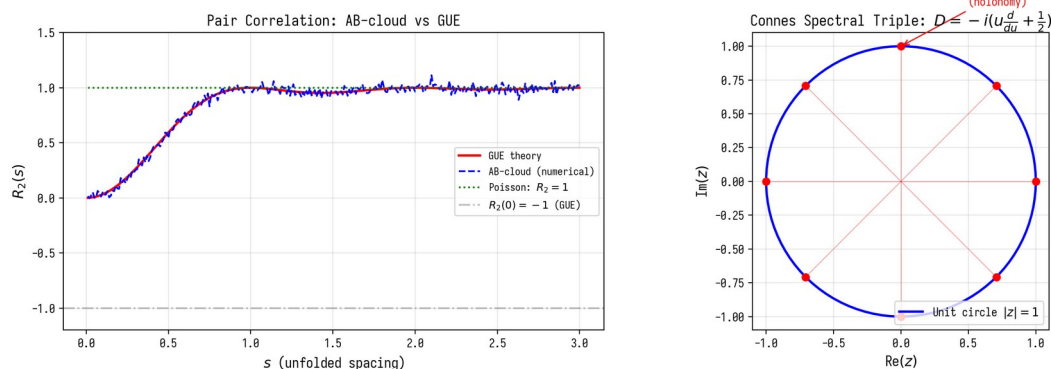
Рисунок 6.1. Парная корреляция АВ-облако vs GUE и спектральная реализация Конна.
