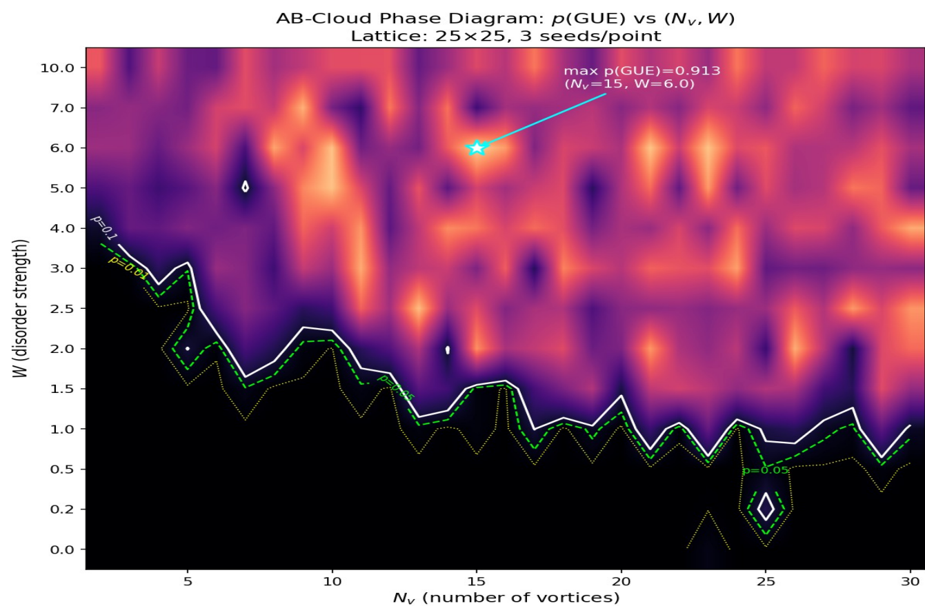
Рисунок 3. Фазовая диаграмма p(\text{GUE})(N_v, W) . GUE — широкое плато при W \geq 2 , N_v \geq 5 .
