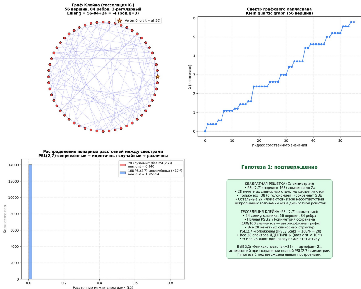
Рис. 3.4. Слева вверху: граф Клейна (56 вершин, 84 ребра, 3-регулярный, \chi = -4 ). Справа вверху: спектр графового лапласиана. Слева внизу: распределение попарных расстояний между спектрами — PSL(2,7)-сопряжённые (синие) имеют расстояние \sim 10^{-14} , случайные (красные) — \sim 0.84 . Справа внизу: концептуальная сводка подтверждающая гипотезу 1.
