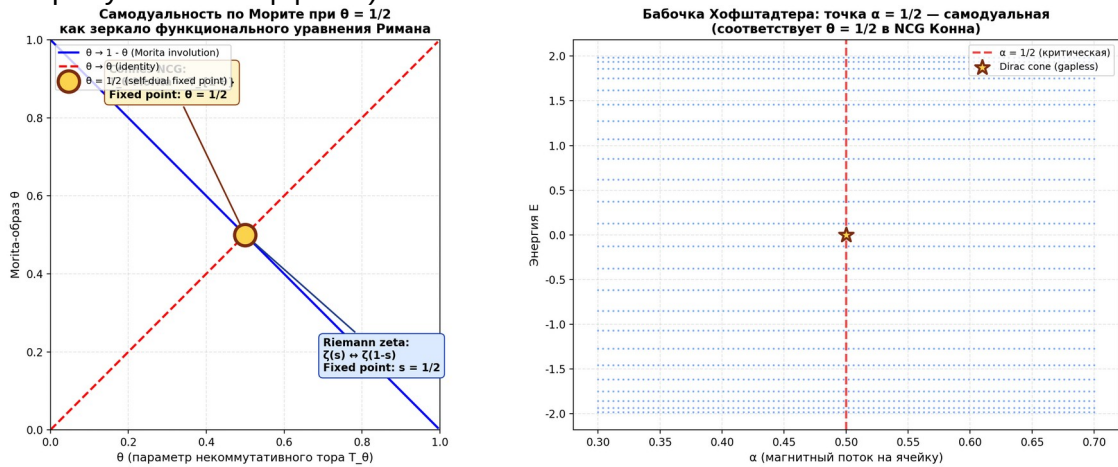
Рис. 6.3. Слева: инволюция Мориты \theta \rightarrow 1-\theta с неподвижной точкой \theta = 1/2 (самодуальность T_{1/2} ), параллельная инволюции s \rightarrow 1-s с неподвижной точкой s = 1/2 (функциональное уравнение Римана). Справа: бабочка Хофштадтера; точка \alpha = 1/2 — самодуальная (дираковский конус без щели).
