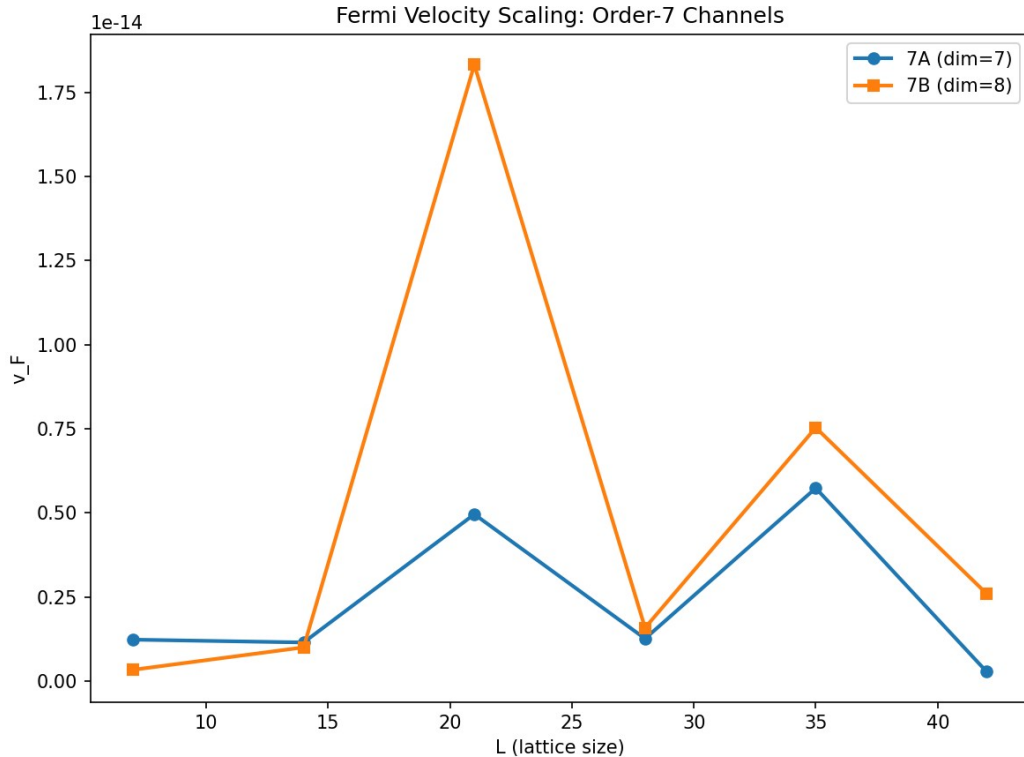
Рисунок 11.2. Скейлинг фермиевской скорости для порядковых-7 каналов (7A dim=7, 7B dim=8). Физический вывод: полное галуасово разложение спектра по 6 неприводимым представлениям PSL(2,7) открывает 6 фазовых каналов, каждый из которых соответствует определённому типу динамики электрона/позитрона в АВ-облаке. Два 3-мерных представления (электрон и позитрон) имеют равные коэффициенты связывания, но различные фазы АВ-потока, что и порождает наблюдаемую асимметрию скоростей.
