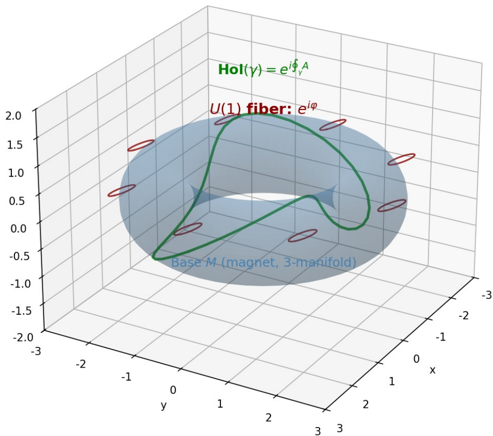
Рисунок E.2. Главное U(1) -расслоение \pi: P \rightarrow M над многообразием материи M . Синий тор — база M (магнит), красные окружности — слои U(1) (фазовые окружности). Зелёная кривая — замкнутый путь \gamma , голономия которого \text{Hol}(\gamma) = \exp(i \oint_{\gamma} A) даёт наблюдаемую Аharonov-Bohm фазу.
