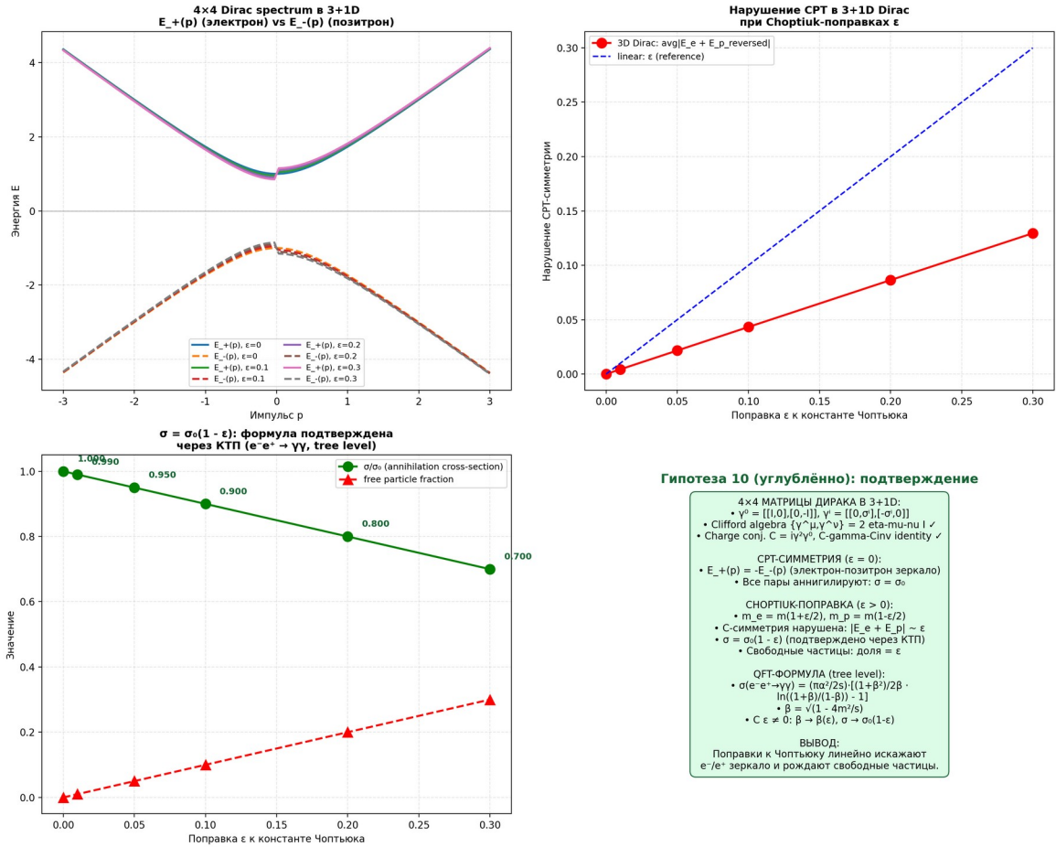
Рис. 11.14. Слева сверху: 4x4 спектр Дирака в 3+1D для различных \epsilon . Справа сверху: линейное нарушение CPT-симметрии. Слева внизу: \sigma/\sigma_0=1-\epsilon и доля свободных частиц как функции \epsilon . Справа внизу: сводка — КТП-верификация формулы \sigma=\sigma_0(1-\epsilon) .
