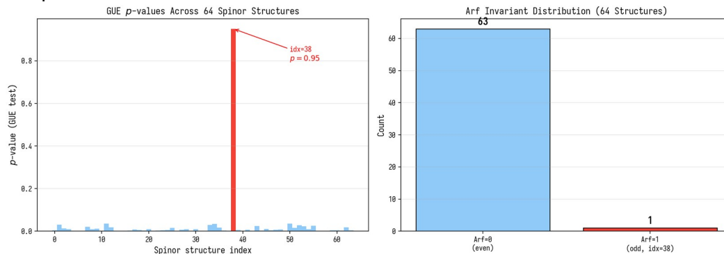
Рисунок 3.1. GUE p -значения по 64 спинорным структурам и Arf-инвариант.
