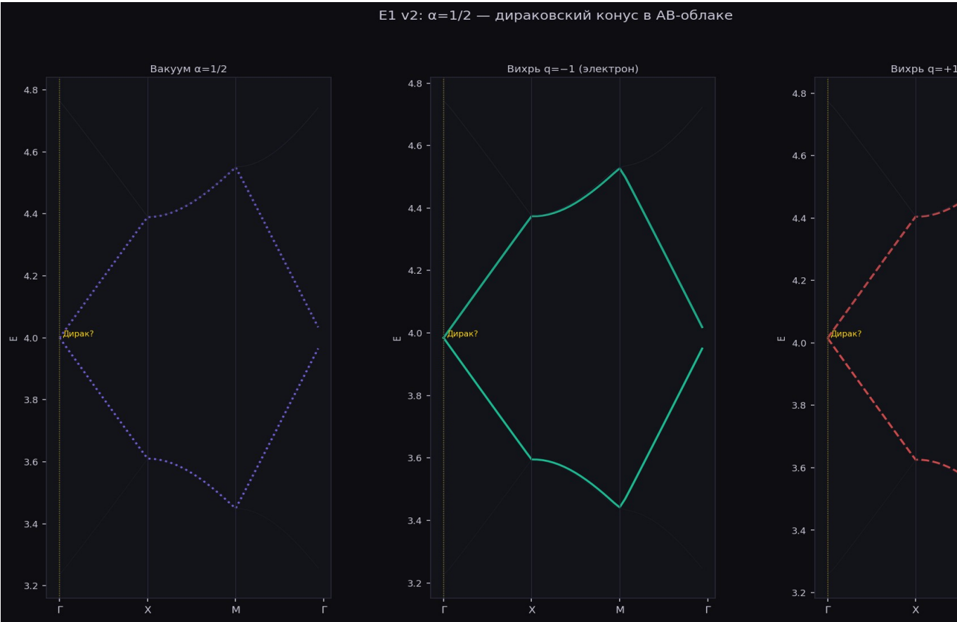
Рисунок 6. E1 v2: дисперсионный закон вихря при \alpha=1/2 . Линейный конус Дирака.
