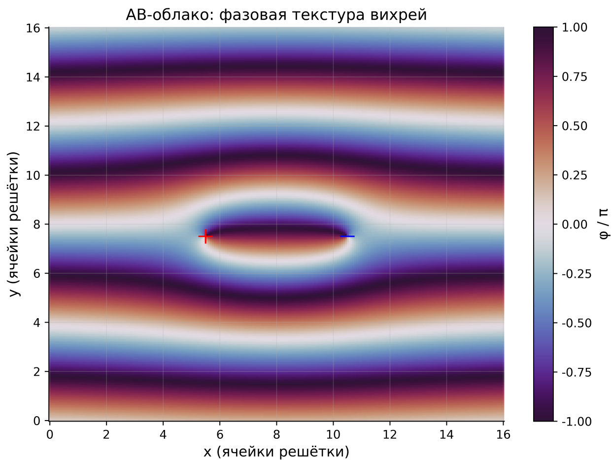
Рис. 18: Рис. 18. Фазовая текстура вихревой пары q = \pm 1 на фоне калибровки Ландау: «облако» фаз, порождающее наблюдаемую статистику.
