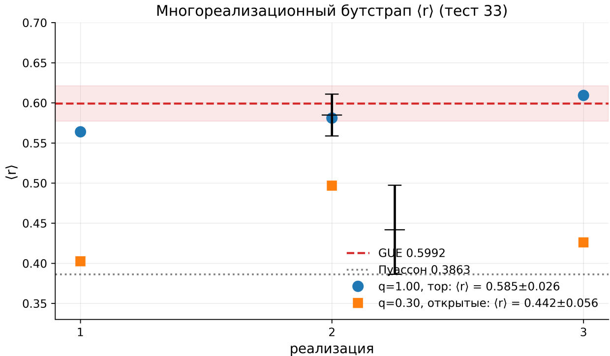
Рис. 9: Рис. 9. Тест 33: три реализации \langle r \rangle для q = 1 (тор) и q = 0,3 (открытые границы) на фоне GUE- и пуассоновской линий.
