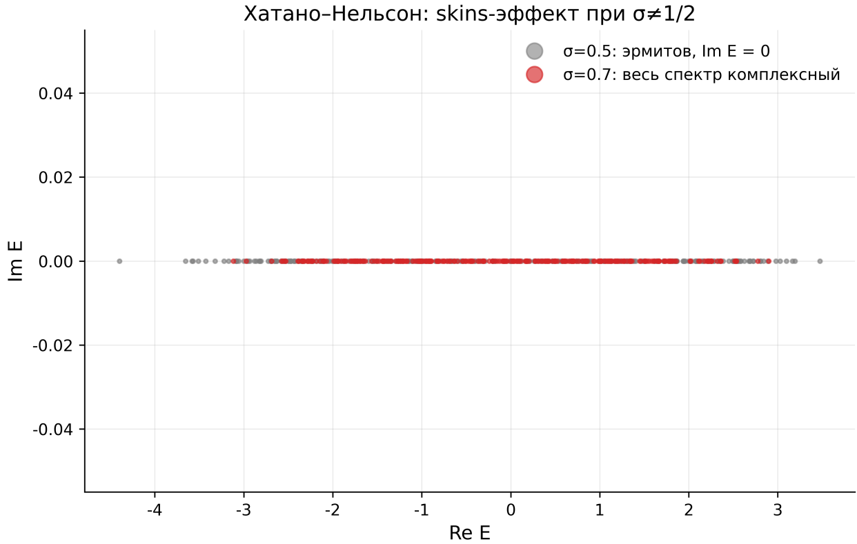
Рис. 16: Рис. 16. Хатано-Нельсон: \sigma = 0,5 — вещественный спектр; \sigma = 0,7 — весь спектр в комплексной плоскости (скин-эффект).
