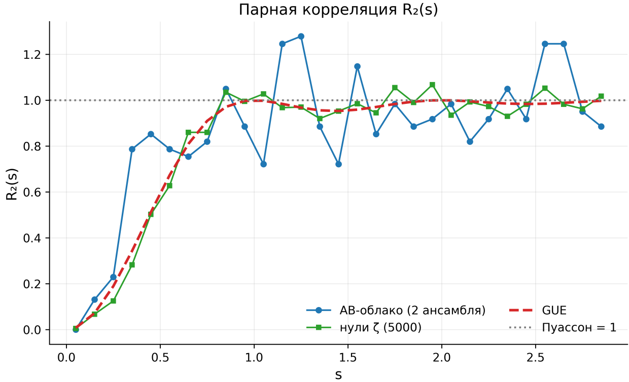
Рис. 12: Рис. 12. Парная корреляция R_2(s) : АВ-облако против нулей \zeta , GUE и Пуассона — корреляционная дыра воспроизводится обеими ветвями.
