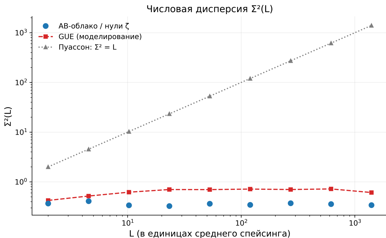
Рис. 6: Рис. 6. Числовая дисперсия \Sigma^2(L) : данные (константа) против логарифмического GUE и линейного Пуассона — 9/9 точек ближе к GUE.
