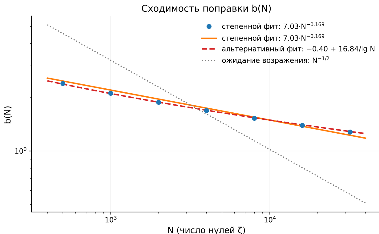
Рис. 1: Рис. 1. Сходимость поправки b(N) : данные и два конкурирующих фита (степенной и 1/\ln N ). Ожидание N^{-1/2} , на котором настаивали критики, данными исключается.
