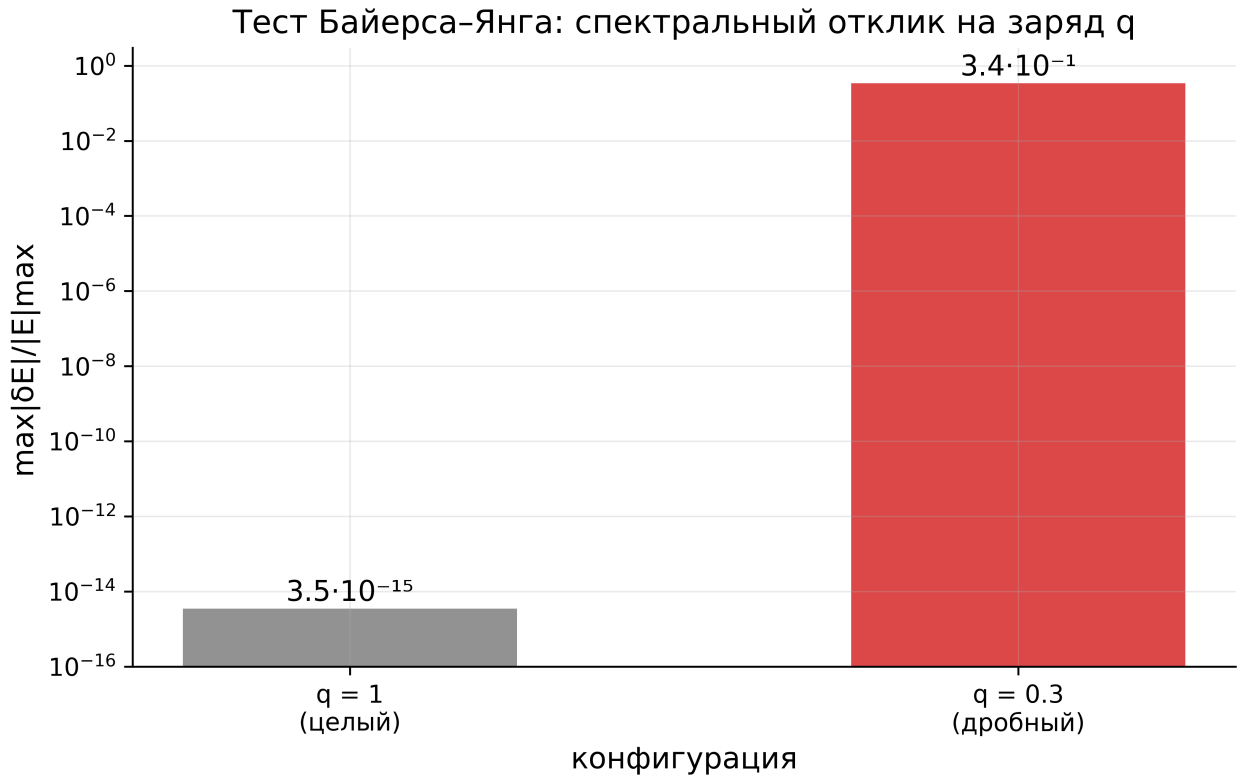
Рис. 8: Рис. 8. Тест Байерса-Янга: целый заряд спектрально невидим ( 3,5 \cdot 10^{-15} ), дробный — физичен (0,34); логарифмическая шкала.
