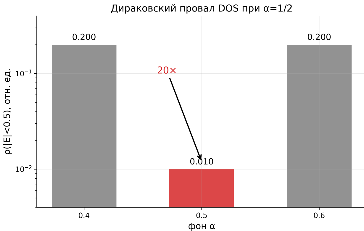
Рис. 15: Рис. 15. Дираковский провал DOS при \alpha = 1/2 : контраст 20\times в обе стороны (логарифмическая шкала).
