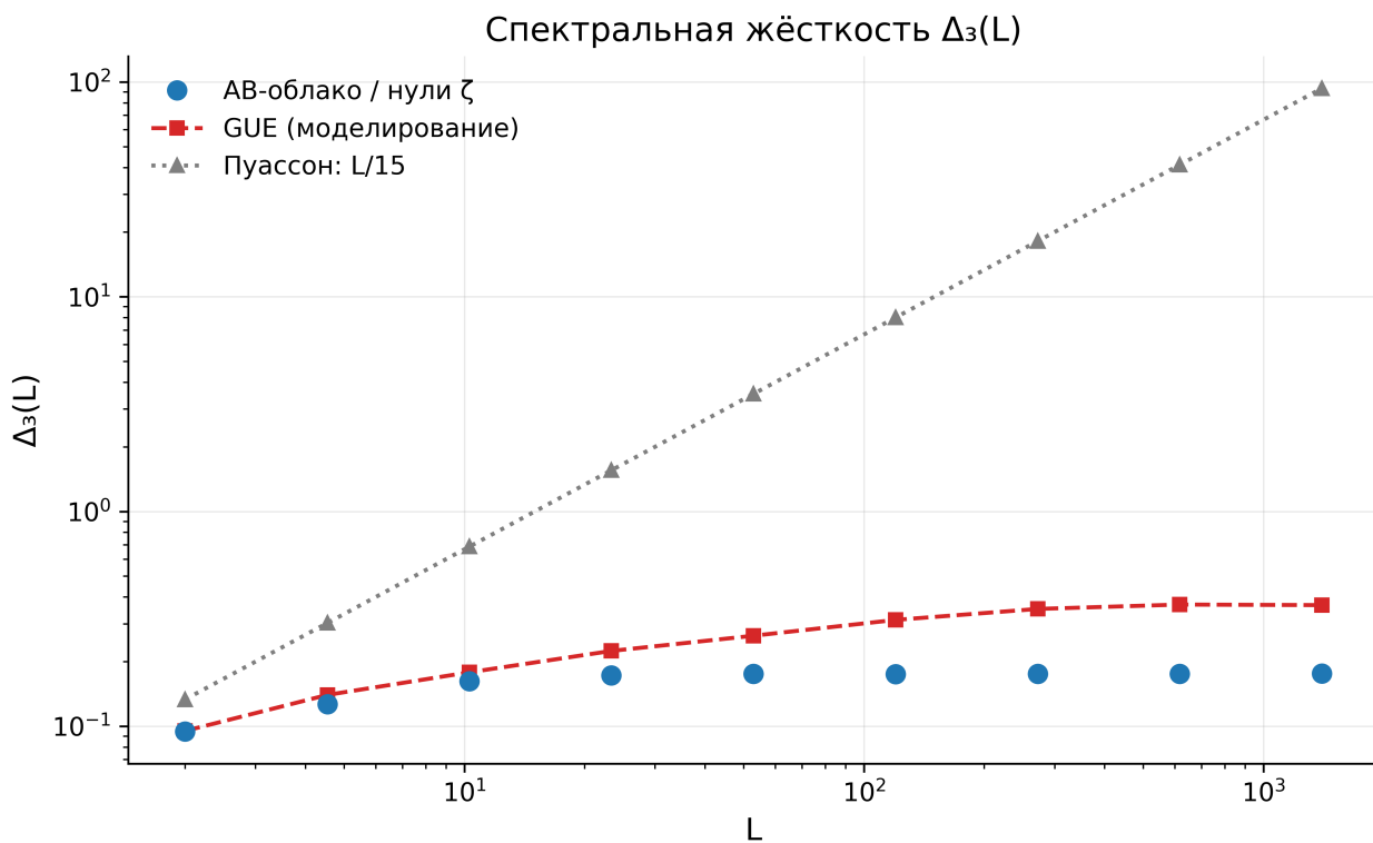
Рис. 7: Рис. 7. Спектральная жёсткость \Delta_3(L) : сверхжёсткость данных относительно даже смоделированного GUE на больших L .
