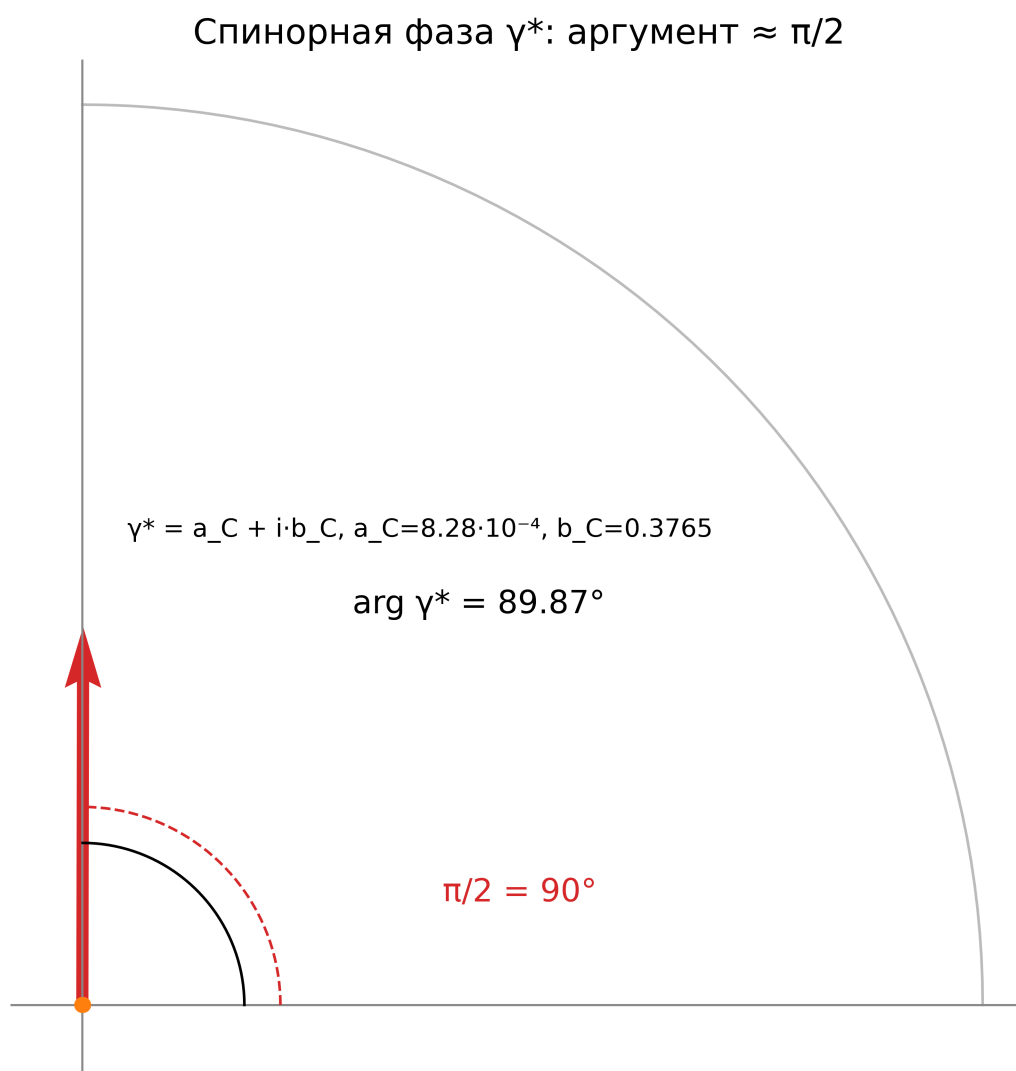
Рис. 17: Рис. 17. Спинорная фаза \gamma^* = a_C + ib_C : аргумент 89,87^\circ против эталонных 90^\circ ; доминирование b_C прижимает фазу к \pi/2 .
