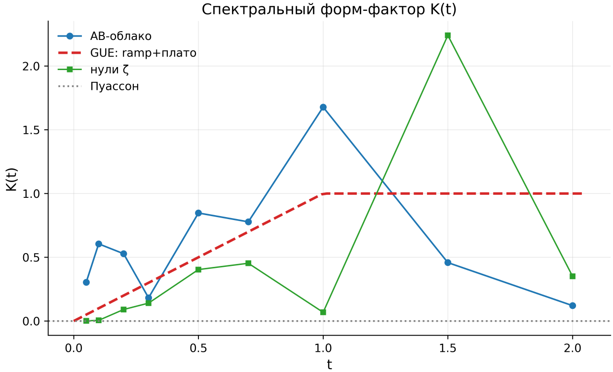
Рис. 13: Рис. 13. Спектральный формфактор K(t) : рампа+плато GUE, данные АВ-облака и нулей \zeta ; малые ансамбли дают правильную тенденцию с выбросами.
