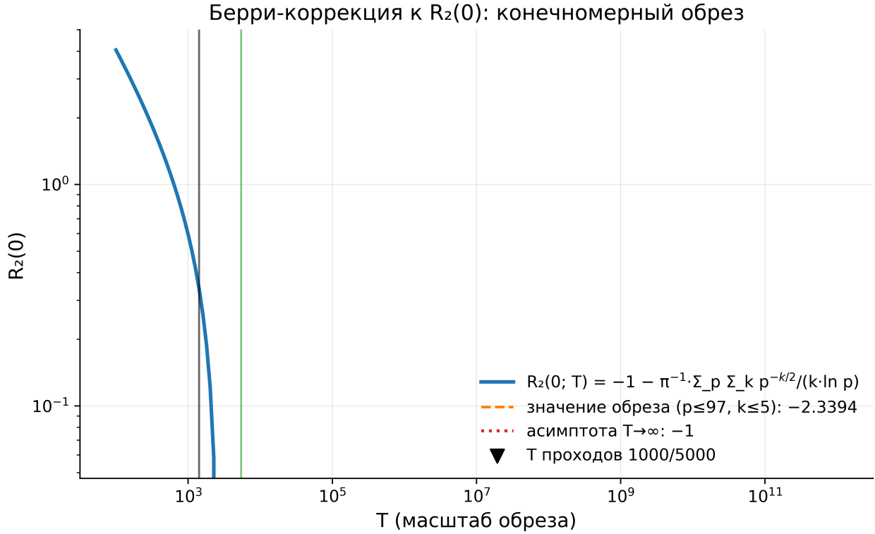
Рис. 11: Рис. 11. Берри-коррекция R_2(0; T) : конечновыборочный обрез и медленное приближение к асимптоте -1 ; вертикали — высоты двух проходов (1000/5000 нулей).
