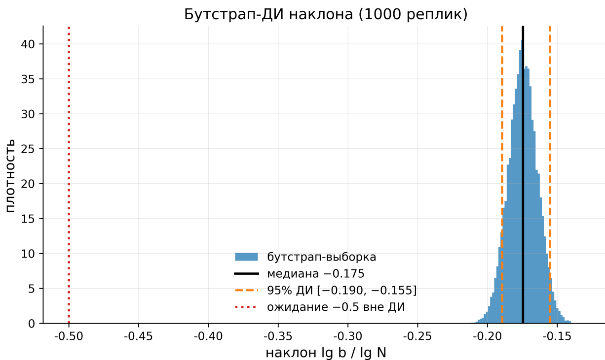
Рис. 5: Рис. 5. Бутстрап-распределение наклона (1000 реплик): 95% ДИ [-0.190; -0.155] ; значение -0.5 лежит далеко вне интервала.
