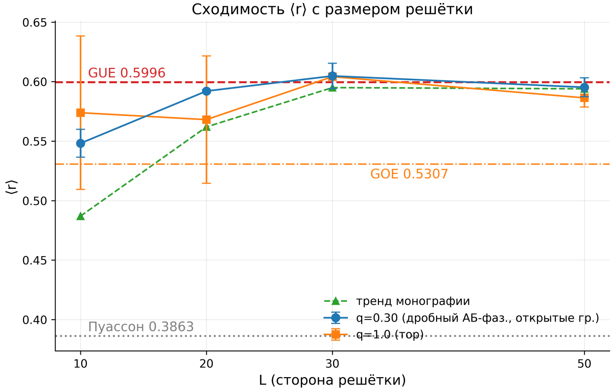
Рис. 10: Рис. 10. Тест 34: сходимость \langle r \rangle с размером решётки; обе ветки выходят на GUE-плато \approx 0,60 .
