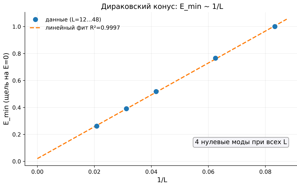
Рис. 14: Рис. 14. Дираковский конус: E_{\min} = 0,02 + 11,83/L , R^2 = 0,9997 — линейность по 1/L при четырёх нулевых модах во всех точках.
