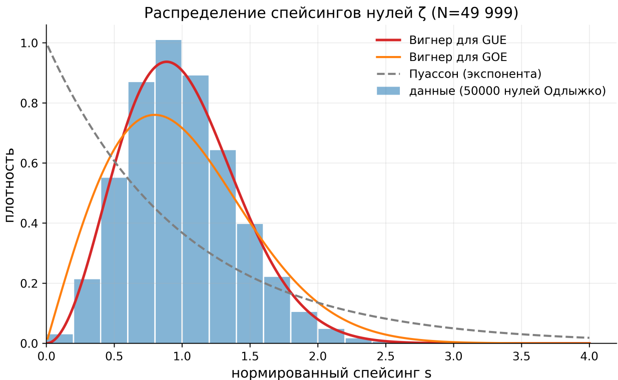
Рис. 2: Рис. 2. Гистограмма 49 999 спейсингов нулей \zeta против сюрмизов Вигнера (GUE, GOE) и пуассоновской экспоненты: форма типично «матричная», с отталкиванием уровней.
