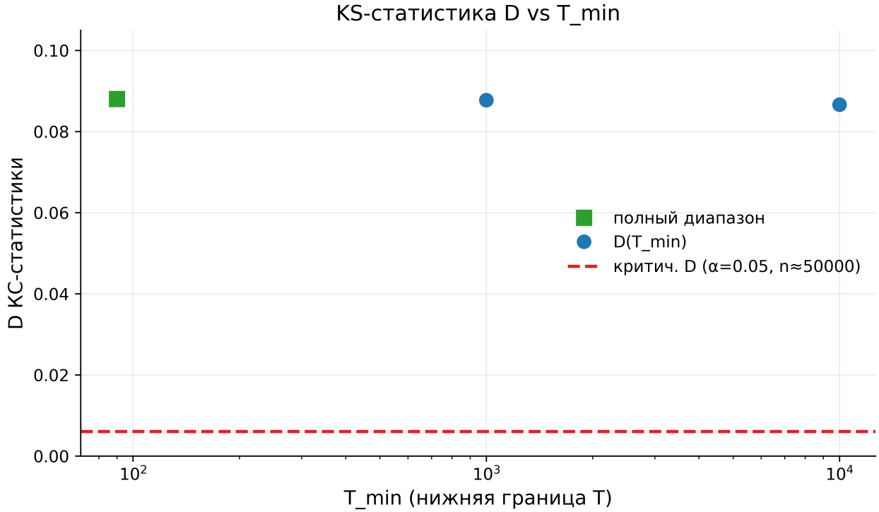
Рис. 3: Рис. 3. KS-статистика D против нижней границы T_{\min} : медленное убывание к критической линии — численное выражение асимптотичности GUE.
