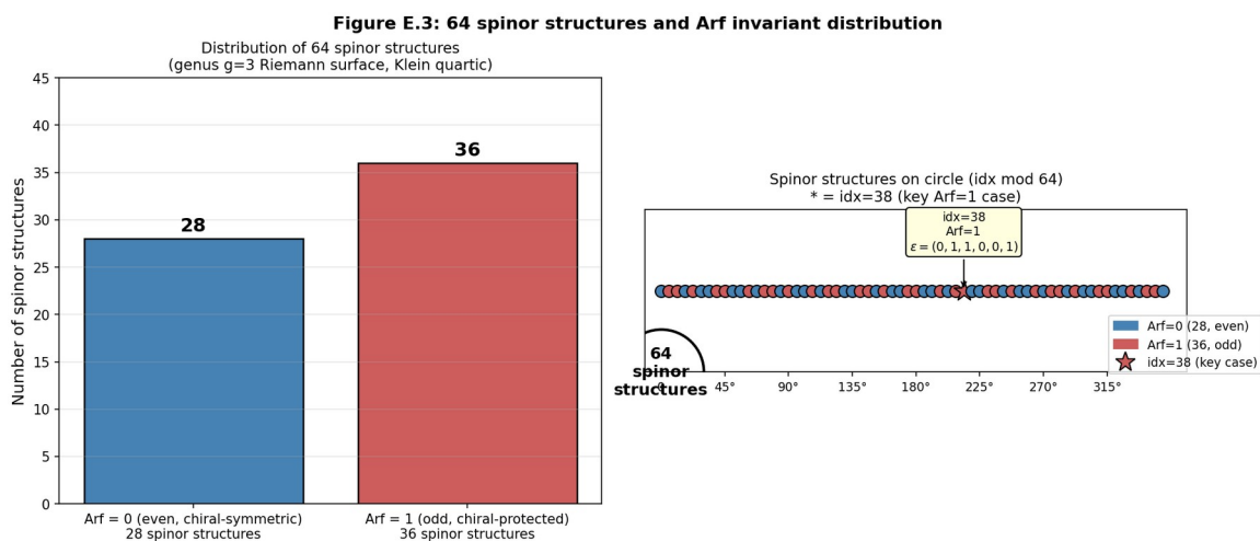
Рисунок E.3. Распределение 64 спинорных структур на кватрике Клейна по Arf-инварианту. Слева: 28 чётных ( Arf=0 , синий) и 36 нечётных ( Arf=1 , красный). Справа: расположение на окружности idx \bmod 64 ; звёздочка отмечает ключевую структуру idx=38 с \varepsilon=(0,1,1,0,0,1) и Arf=1 .
