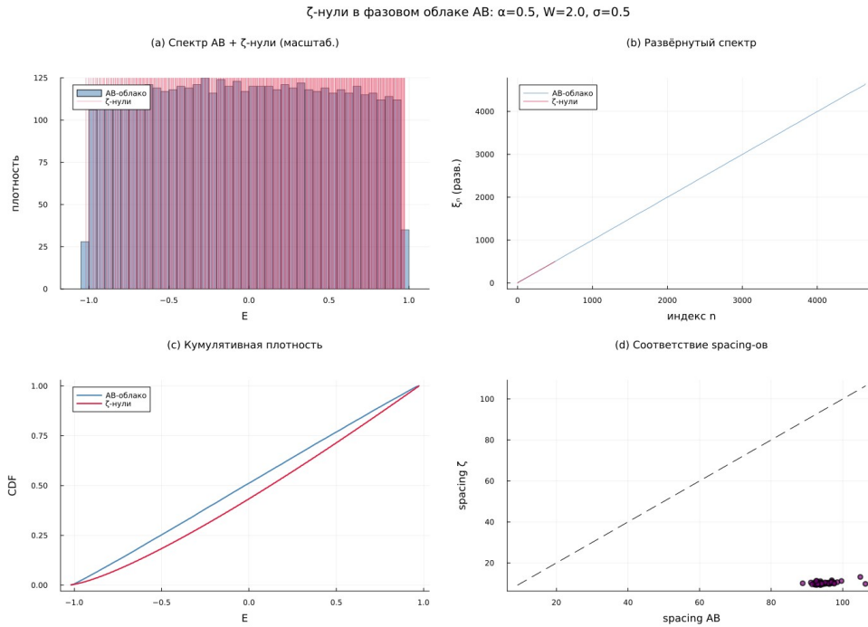
Рис. 22.2. Концептуальная визуализация: \zeta -нули внутри АВ-облака. Каждое собственное значение \lambda_n гамильтониана H_{AB} ассоциировано с нетривиальным нулём \zeta(1/2 + i\gamma_n) = 0 через гипотезу Гильберта–Поли ( \lambda_n = 1/2 + i\gamma_n ).
