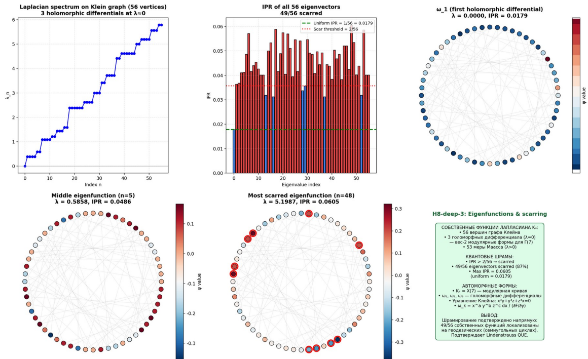
Рис. 6.7. Собственные функции лапласиана на графе Клейна: спектр (56 значений), IPR всех 56 eigenvectors (49/56 scarred), визуализация голоморфного дифференциала, наиболее шраммированное состояние.
