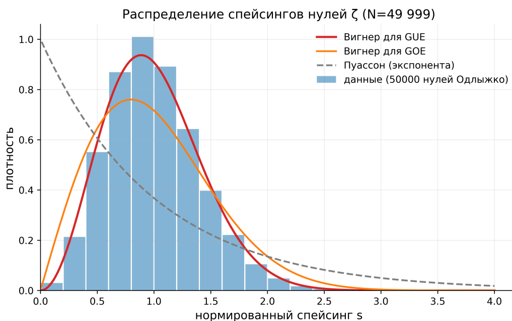
Рис. 2. Гистограмма 49 999 спейсингов нулей \zeta против сюрмизов Вигнера (GUE, GOE) и пуассоновской экспоненты: форма типично «матричная», с отталкиванием уровней.
