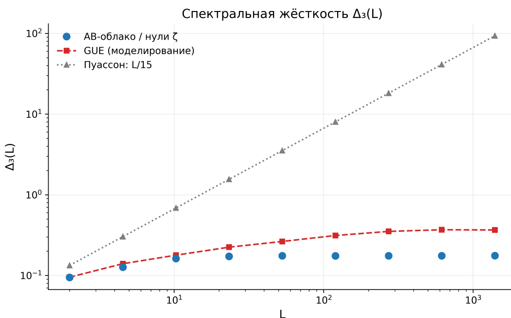
Рис. 7. Спектральная жёсткость \Delta_3(L) : сверхжёсткость данных относительно даже смоделированного GUE на больших L .
