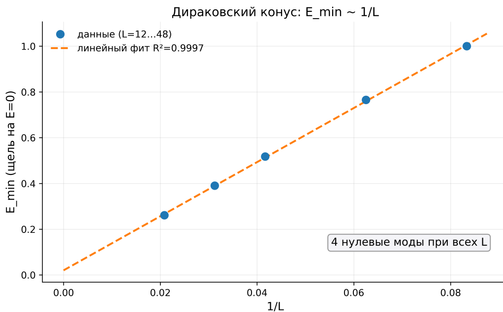
Рис. 14. Дираковский конус: E_{\min} = 0,02 + 11,83/L , R^2 = 0,9997 — линейность по 1/L при четырёх нулевых модах во всех точках.
