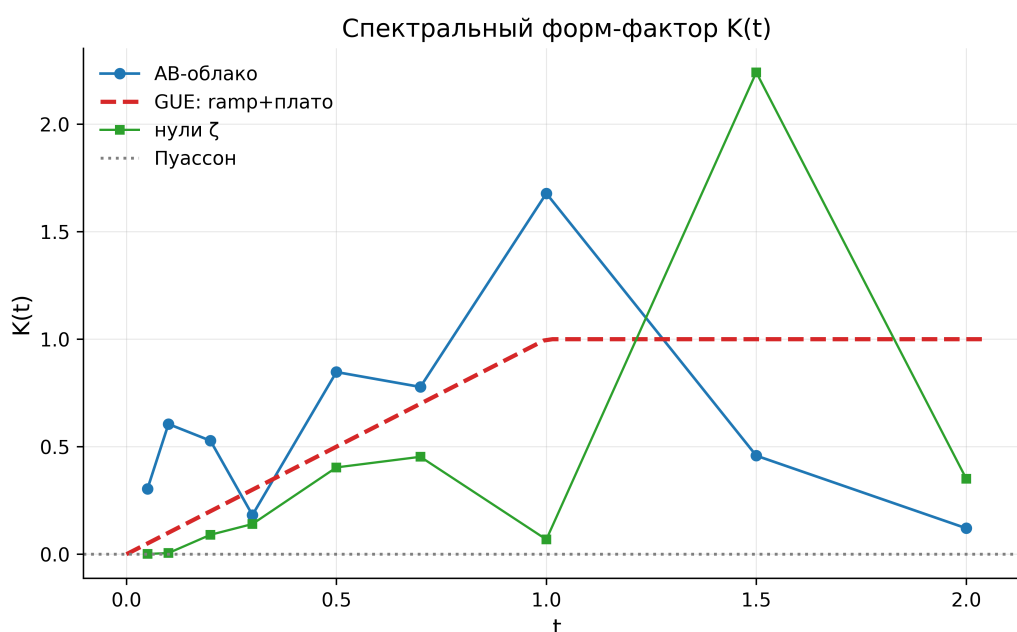
Рис. 13. Спектральный формфактор K(t) : рампа+плато GUE, данные AB-облака и нулей \zeta ; малые ансамбли дают правильную тенденцию с выбросами.
