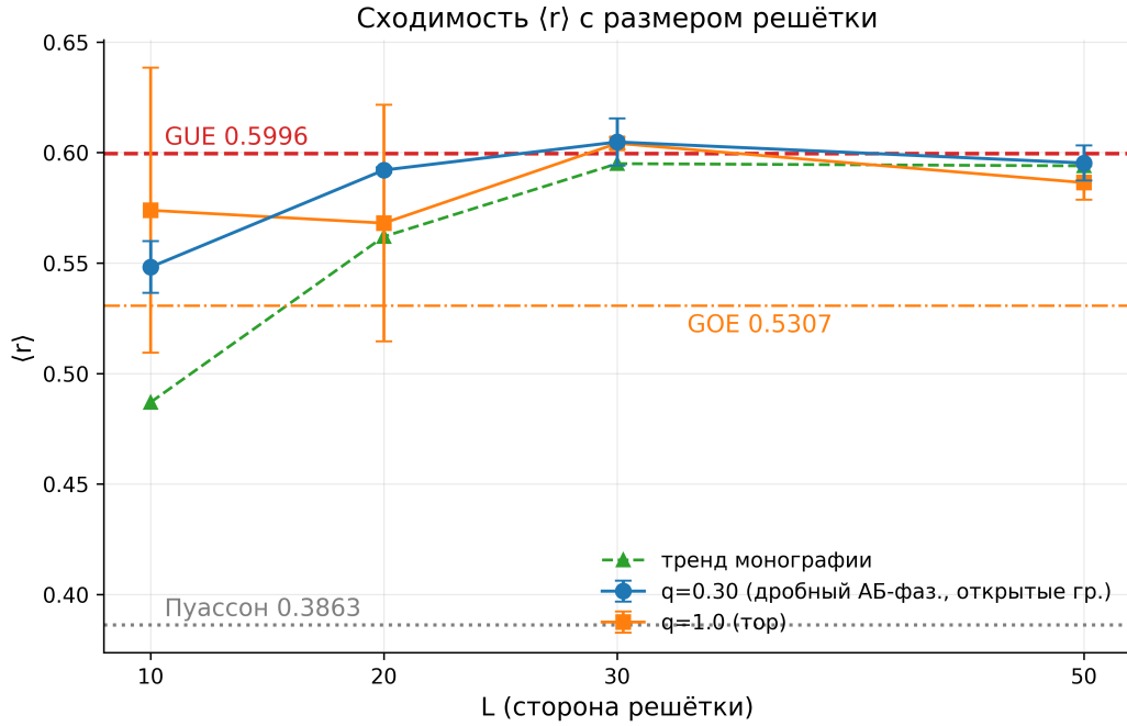
Рис. 10. Тест 34: сходимость \langle r \rangle с размером решётки; обе ветки выходят на GUE-плато \approx 0,60 .
