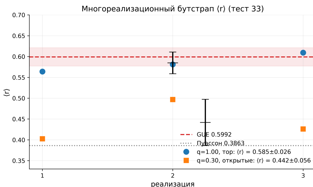
Рис. 9. Тест 33: три реализации \langle r \rangle для q = 1 (тор) и q = 0, 3 (открытые границы) на фоне GUE- и пуассоновской линий.
