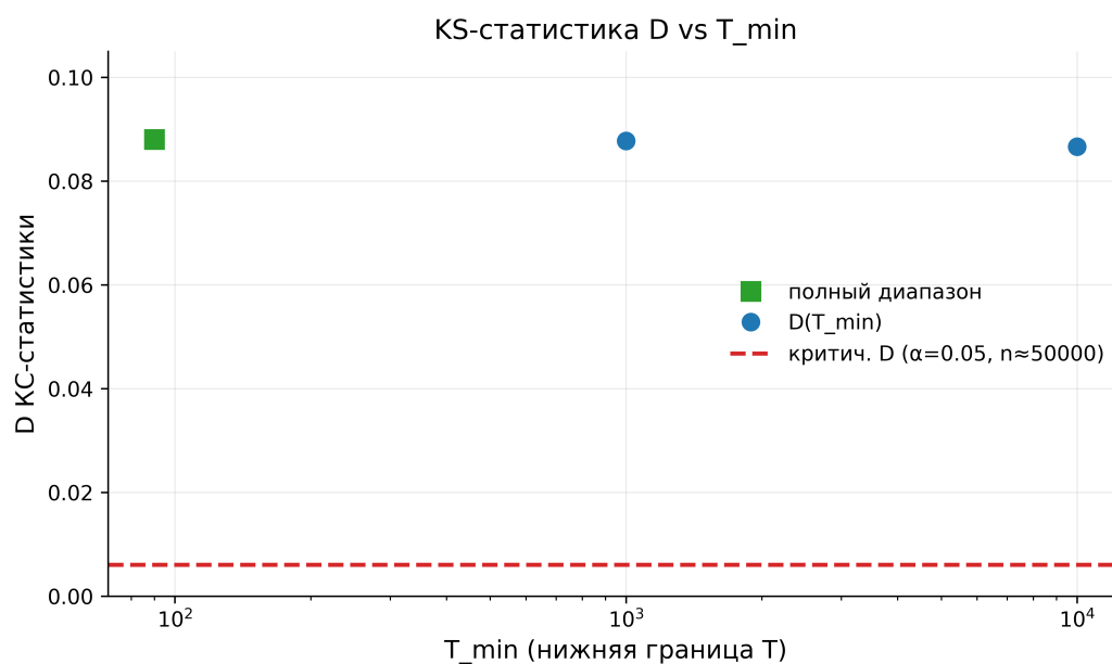
Рис. 3. KS-статистика D против нижней границы T_{\min} : медленное убывание к критической линии — численное выражение асимптотичности GUE.
