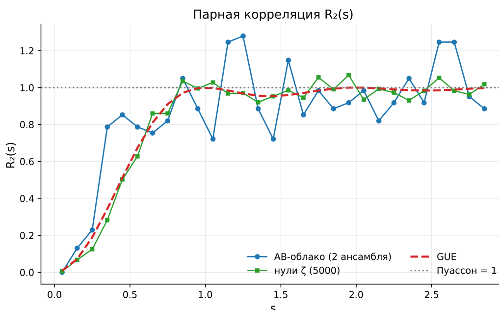
Рис. 12. Парная корреляция R_2(s) : АВ-облако против нулей \zeta , GUE и Пуассона — корреляционная дыра воспроизводится обеими ветвями.
