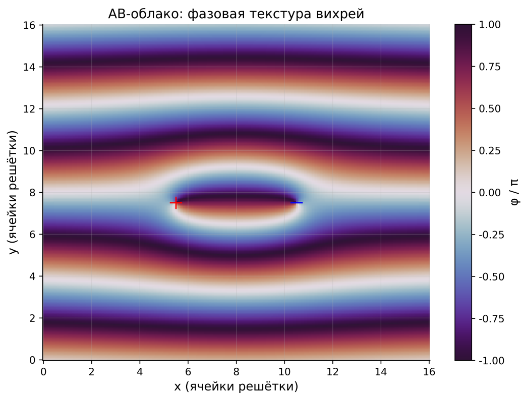
Рис. 18. Фазовая текстура вихревой пары q = \pm 1 на фоне калибровки Ландау: «облако» фаз, порождающее наблюдаемую статистику.
