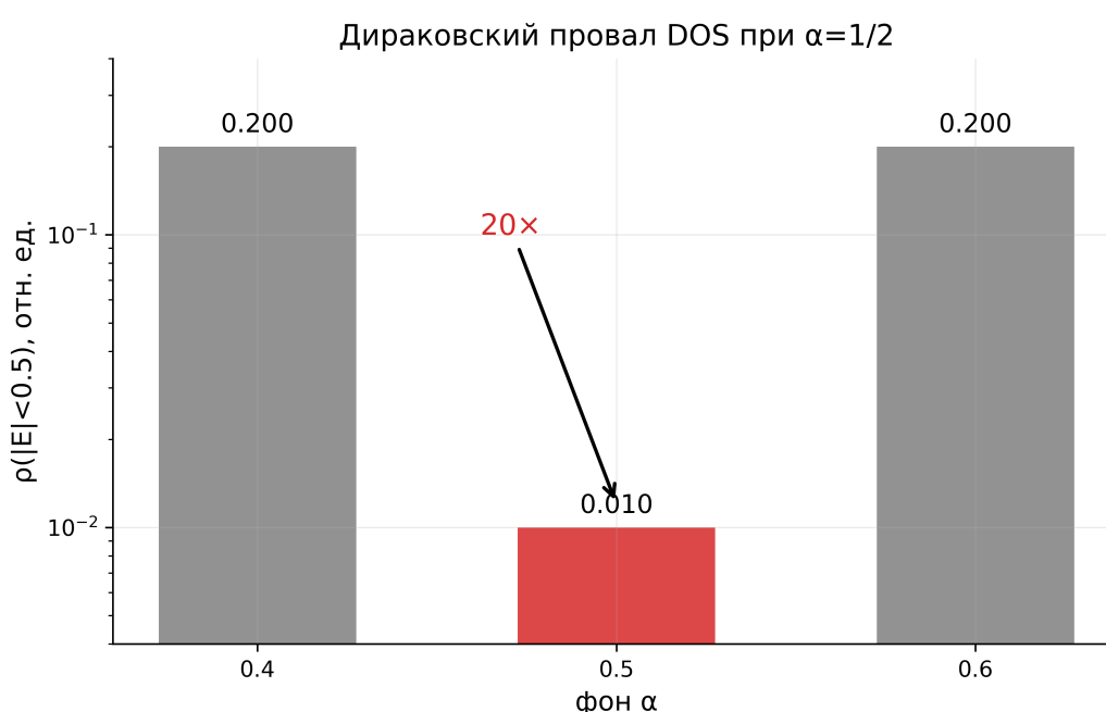
Рис. 15. Дираковский провал DOS при \alpha = 1/2 : контраст 20\times в обе стороны (логарифмическая шкала).
