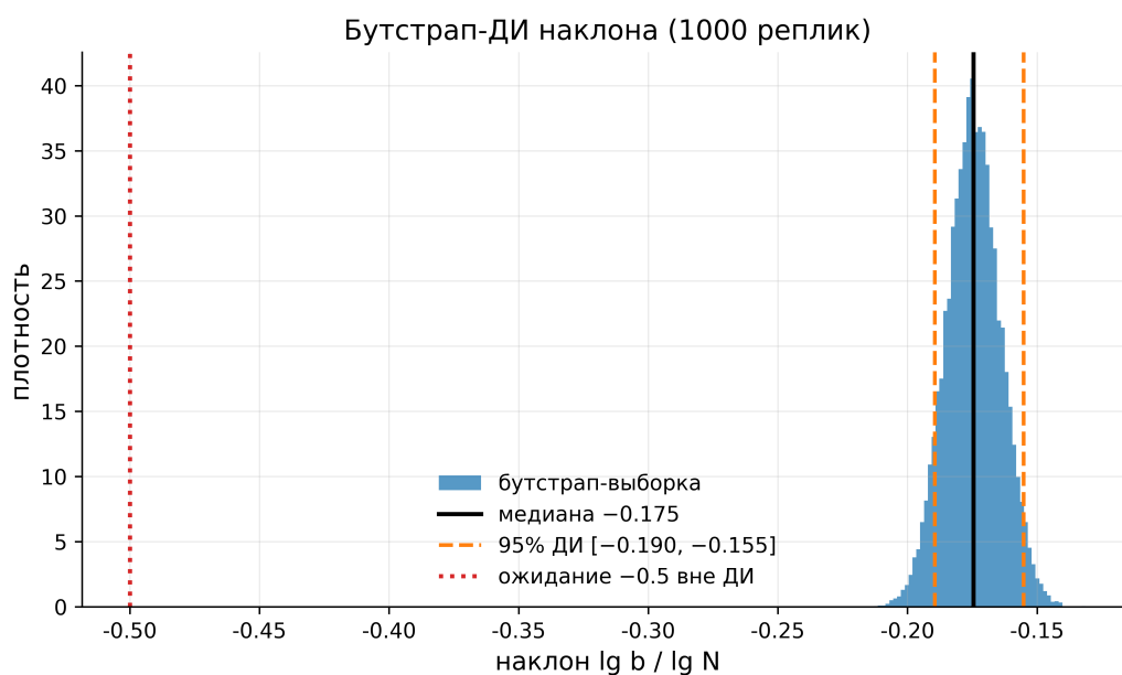
Рис. 5. Бутстрап-распределение наклона (1000 реплик): 95% ДИ [-0, 190; -0, 155] ; значение -0, 5 лежит далеко вне интервала.
