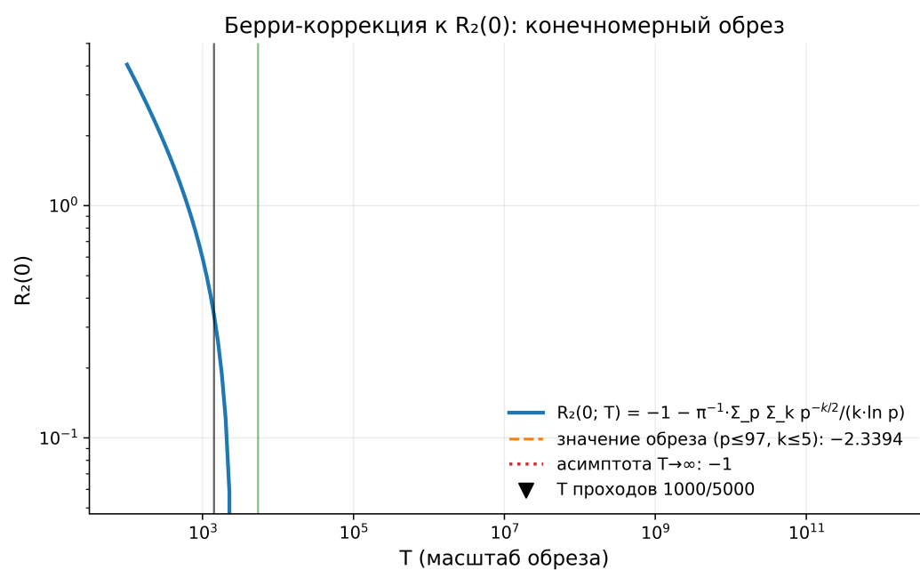
Рис. 11. Берри-коррекция R_2(0; T) : конечновыборочный обрез и медленное приближение к асимптоте -1 ; вертикали — высоты двух проходов (1000/5000 нулей).
