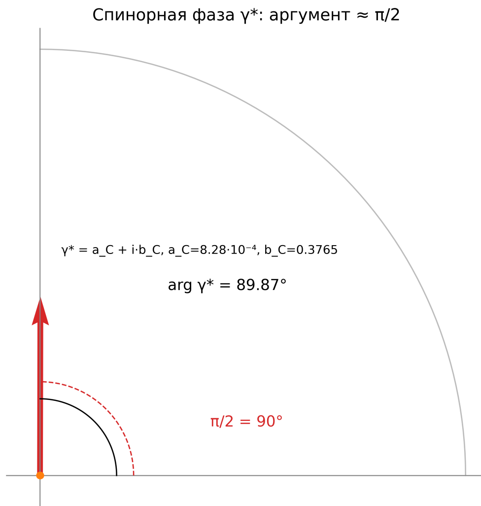
Рис. 17. Спинорная фаза \gamma^* = a_C + ib_C : аргумент 89,87^\circ против эталонных 90^\circ ; доминирование b_C прижимает фазу к \pi/2 .
