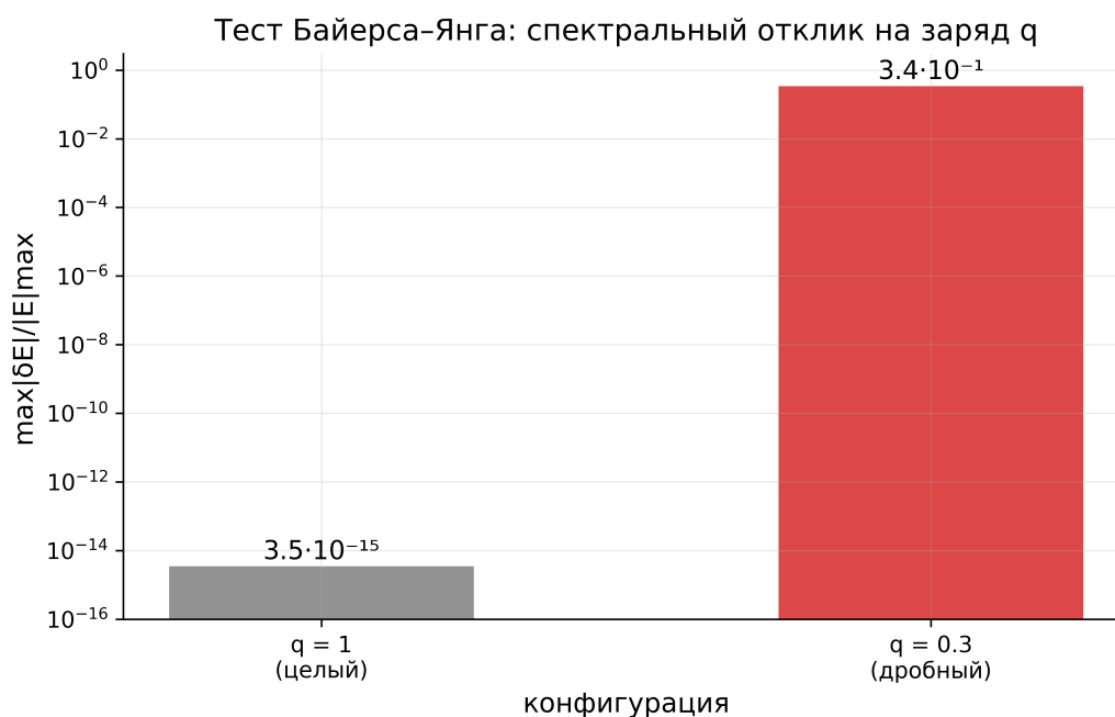
Рис. 8. Тест Байерса–Янга: целый заряд спектрально невидим ( 3,5 \cdot 10^{-15} ), дробный — физичен ( 0,34 ); логарифмическая шкала.
