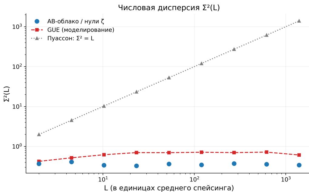
Рис. 6. Числовая дисперсия \Sigma^2(L) : данные (константа) против логарифмического GUE и линейного Пуассона — 9/9 точек ближе к GUE.
