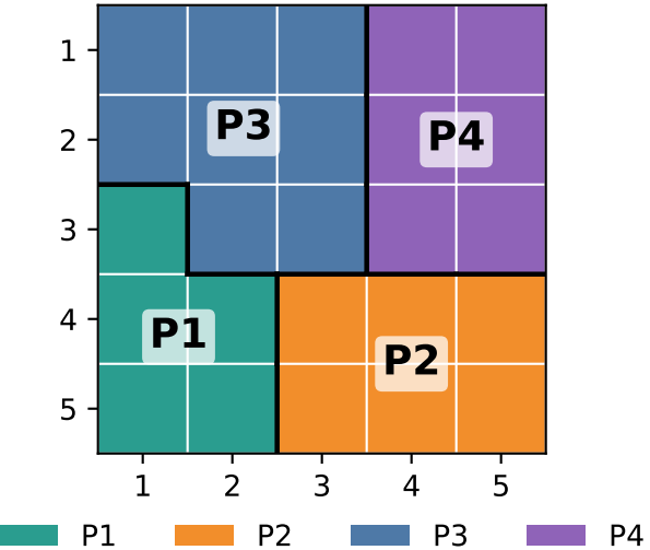
C Four macroprofiles on the actual SOM lattice
