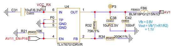
LDO AV11 1.1V
