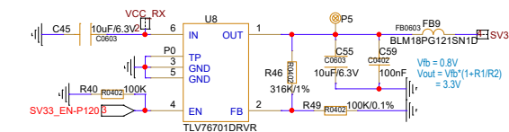
LDO SV33 3.3V
