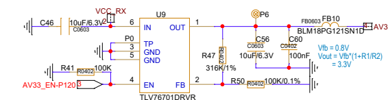
LDO AV33 3.3V
