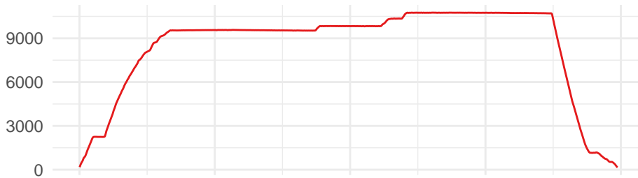
CO 2 / ppmv
