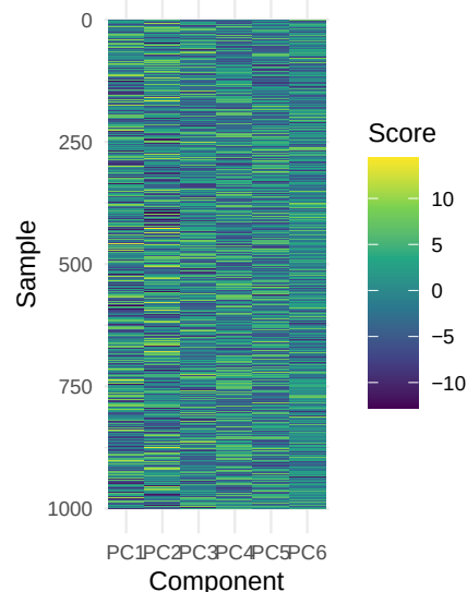
Simulation 5: oracle PCA
