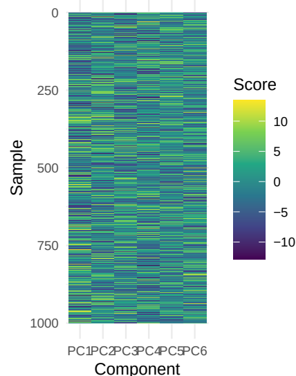
Simulation 3: oracle PCA
