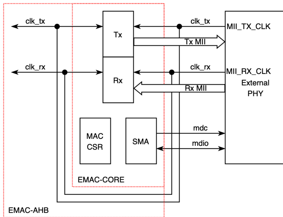
图 50.4-4. MII 时钟
