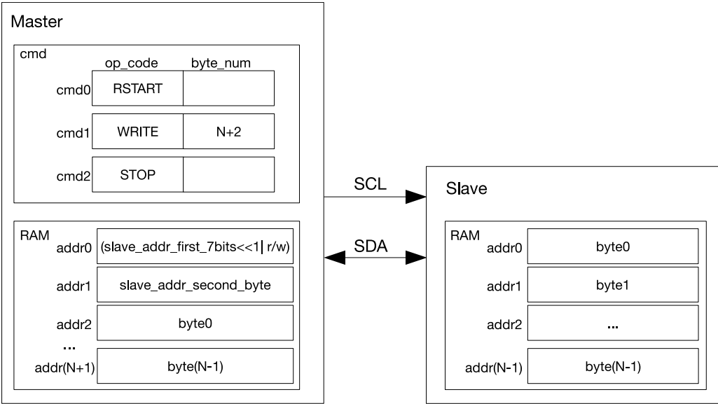
图 42.6-2. I2C 主机写 10 位寻址的从机
