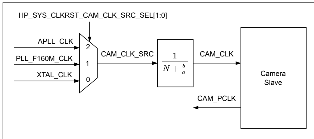
图 36.3-3. Camera 时钟
