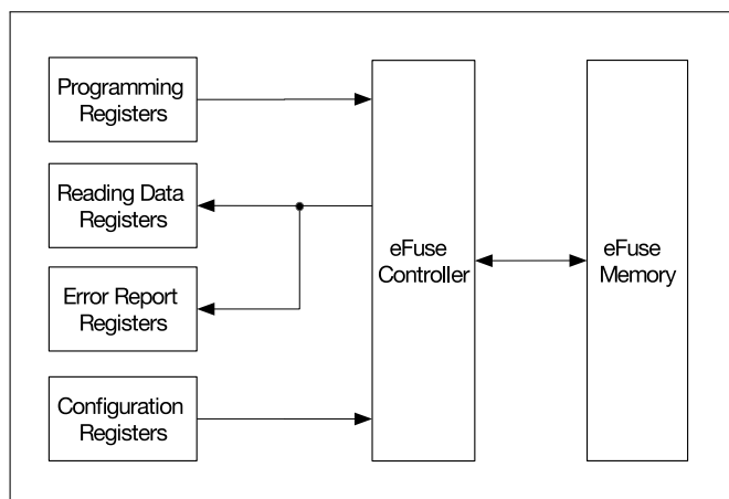
图 8.3-1. eFuse 系统数据通路
