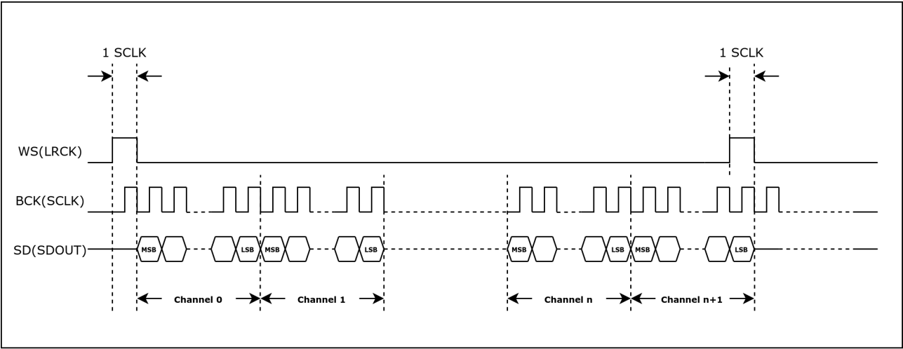
图 44.5-3. 时序图 – TDM PCM 标准
