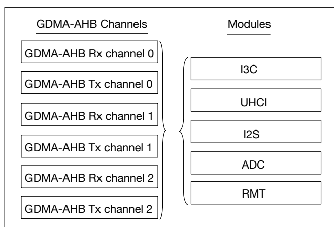
图 4.1-1. 共用 GDMA-AHB 通道的模块
