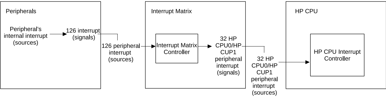
图 12.2-1. ESP32-P4 的中断流
