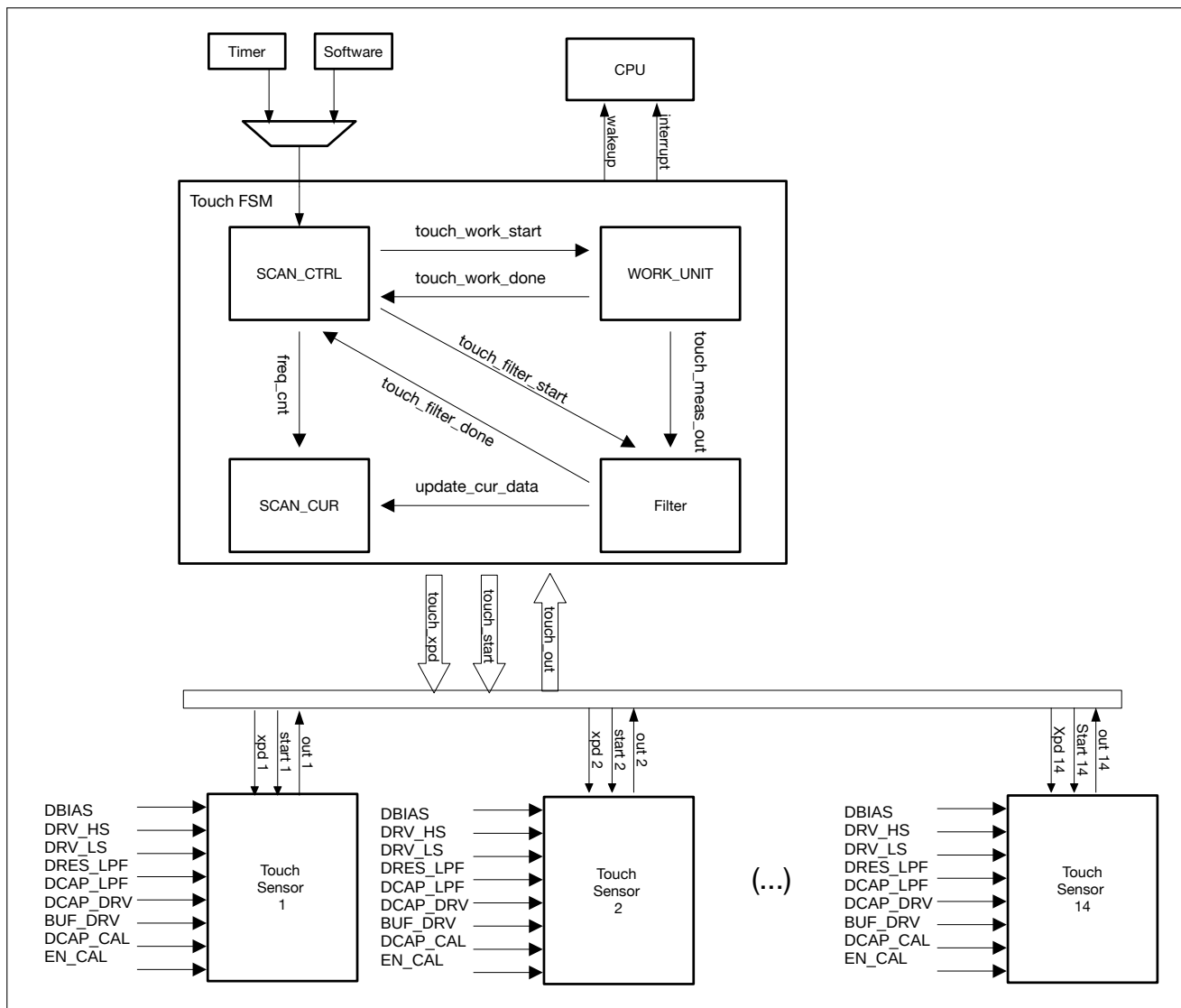
图 58.4-1. Touch FSM 内部结构和工作原理
