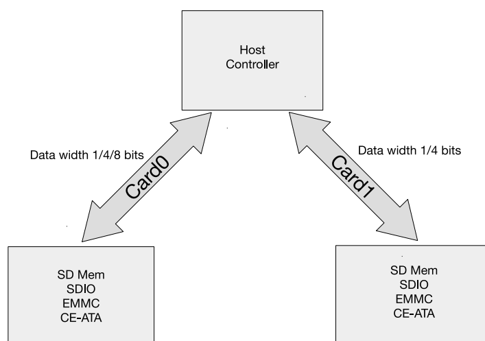
图 52.2-1. SD/MMC 控制器连接的拓扑结构
