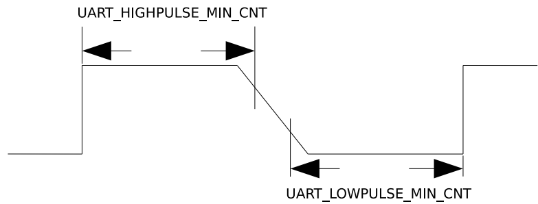
图 40.4-2. UART 信号下降沿较差时序图
