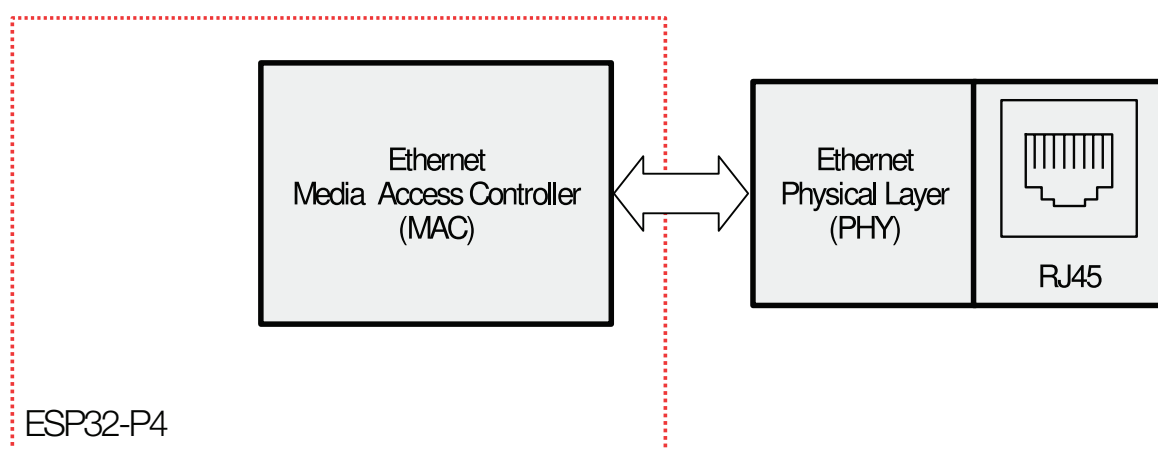
图 50.1-1. Ethernet MAC 功能概述
