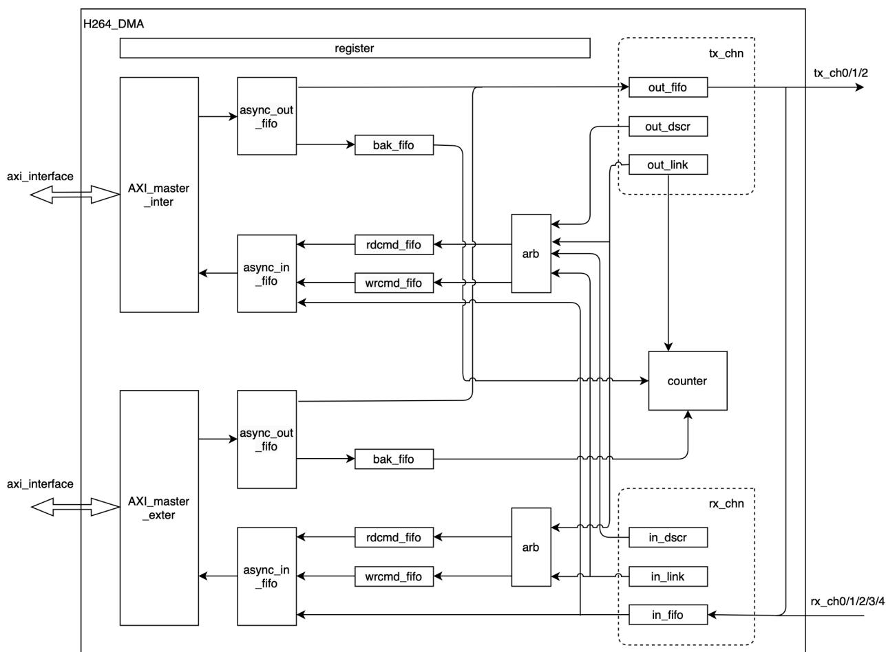
图 37.5-2. H264_DMA 架构
