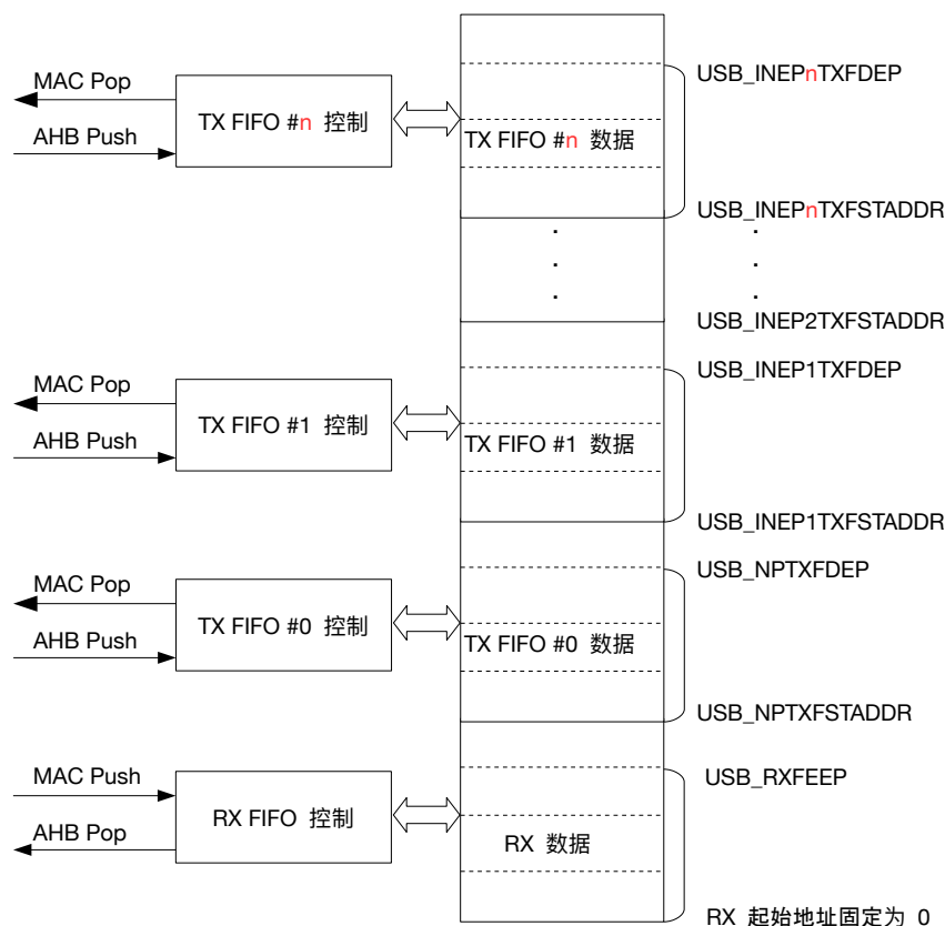
图 48.4-4. 设备模式 FIFO
