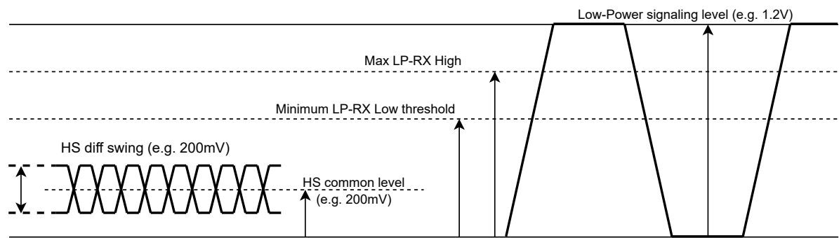
图 38.5-1. MIPI 通道线路电平
