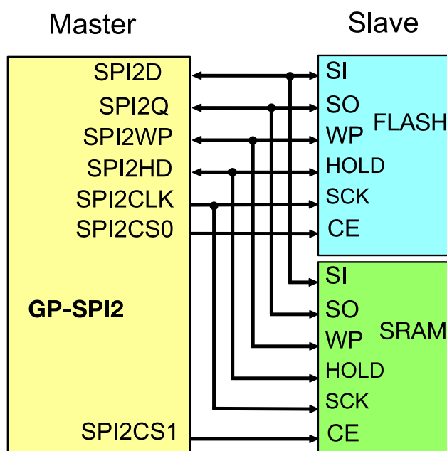
图 41.5-7. 4-bit 模式下 GP-SPI2 与 Flash 以及外部 RAM 的连接方式
