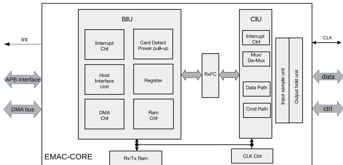
图 52.4-1. SDIO 主机结构框图
