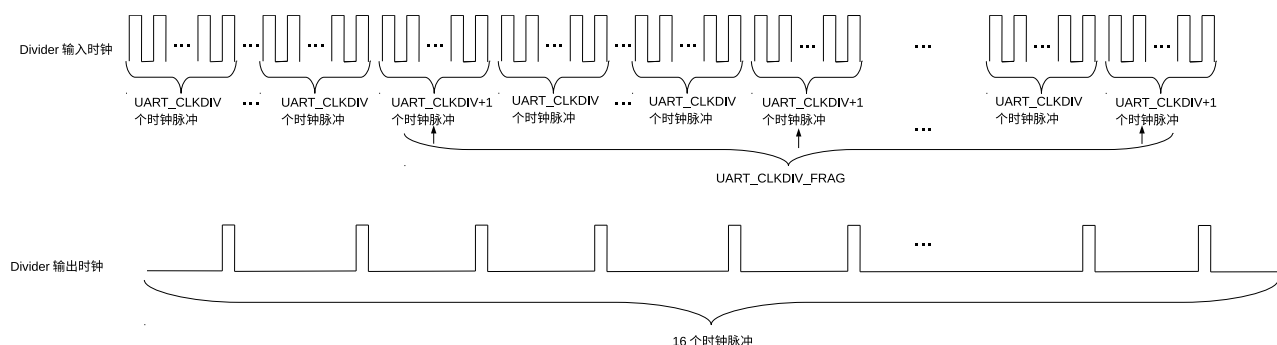
图 40.4-1. UART 控制器分频
