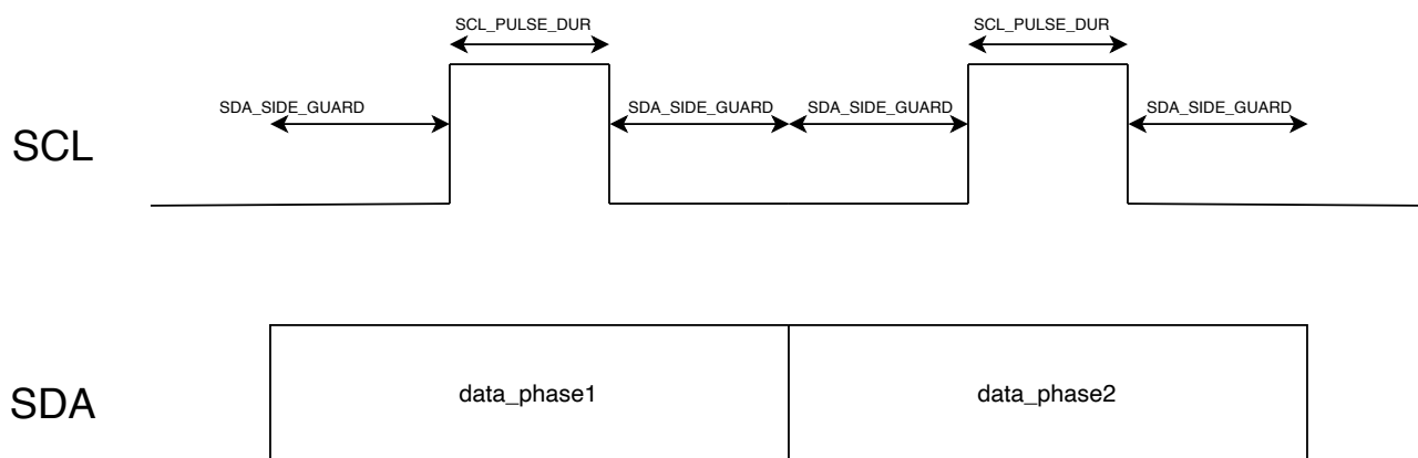
图 43.4-1. 信号相位图
