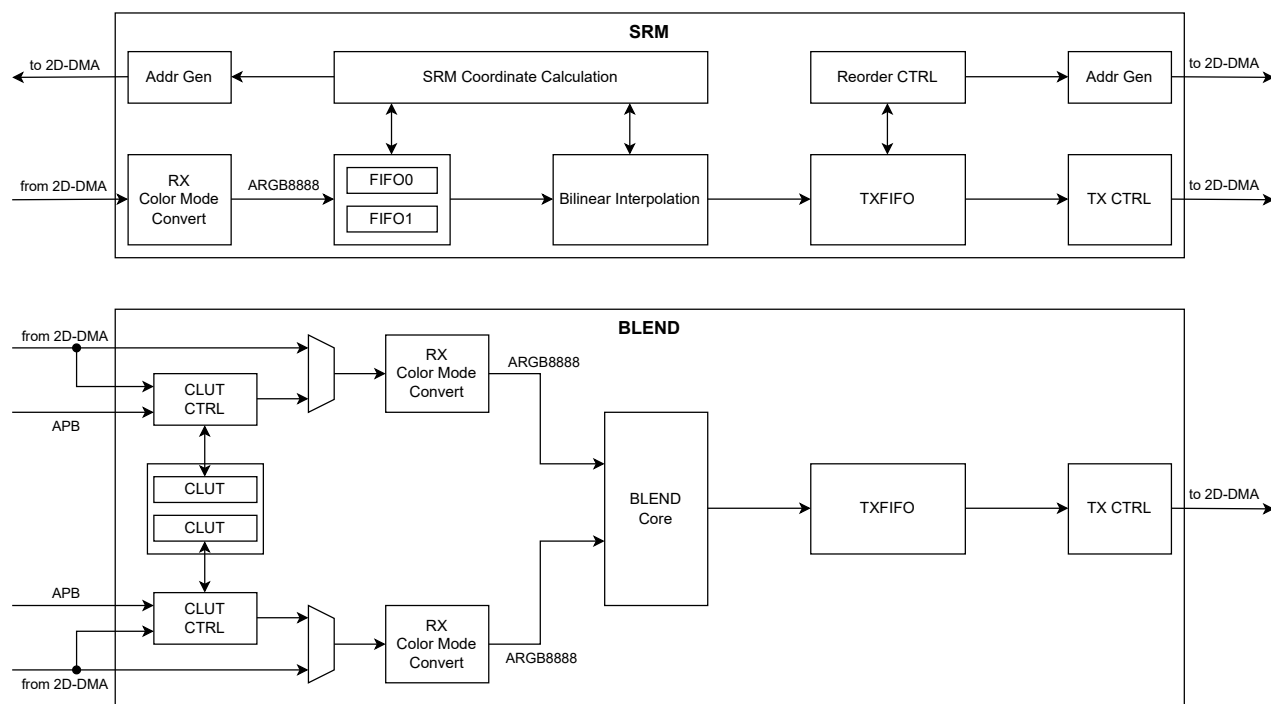
图 35.4-1. PPA 系统架构
