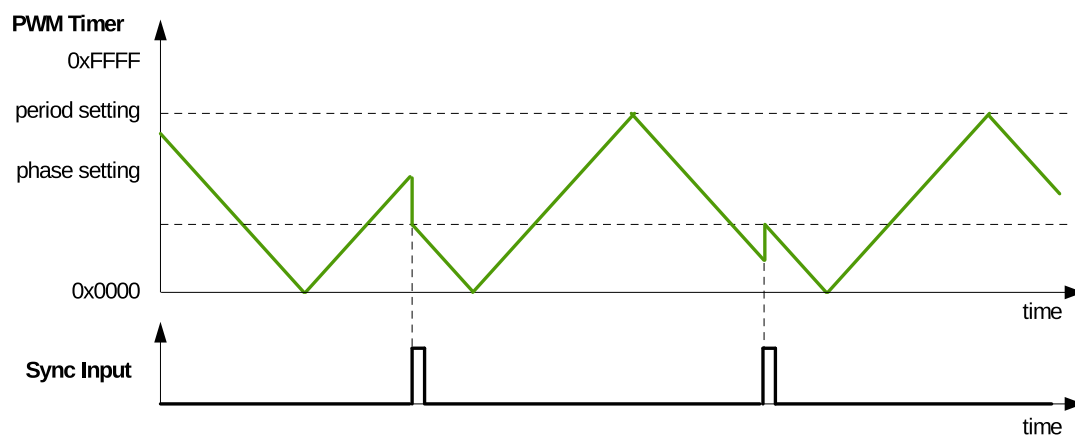
图 54.3-7. 递增递减循环模式波形，同步事件后递减
