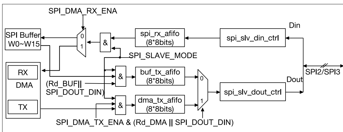
图 41.5-4. GP-SPI 用作从机时的数据流控制
