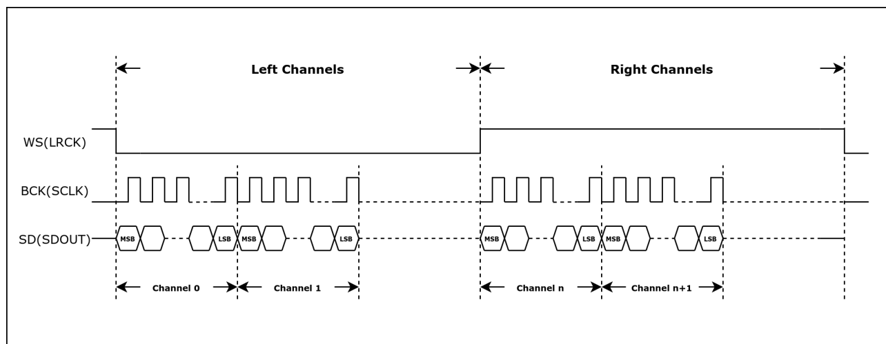
图 45.4-2. 时序图 – TDM MSB 对齐标准
