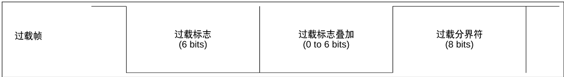
图 51.2-3. 过载帧中的位域
