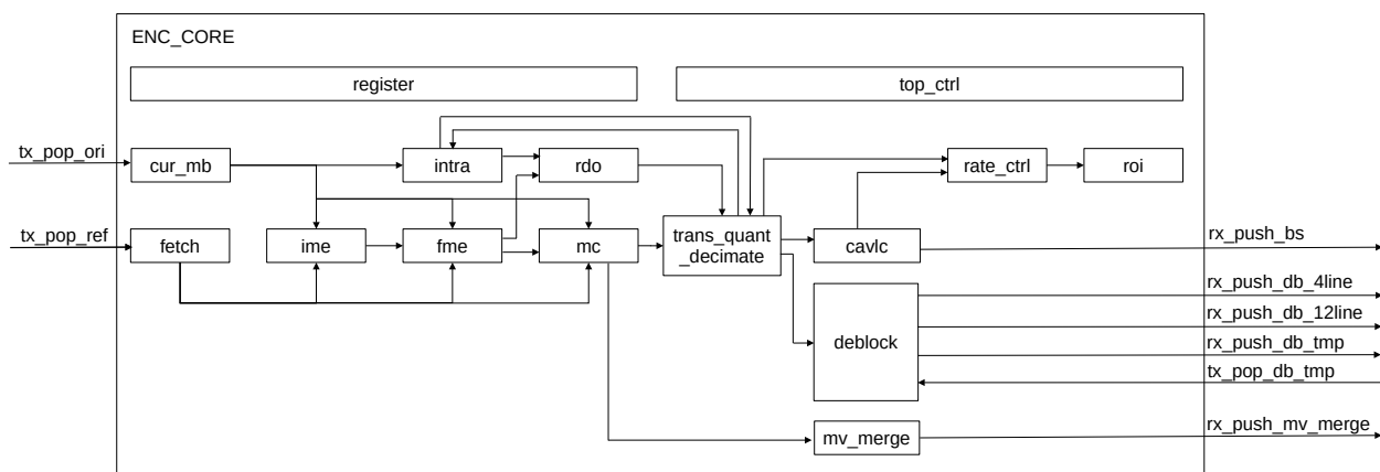
图 37.5-1. ENC_CORE 架构
