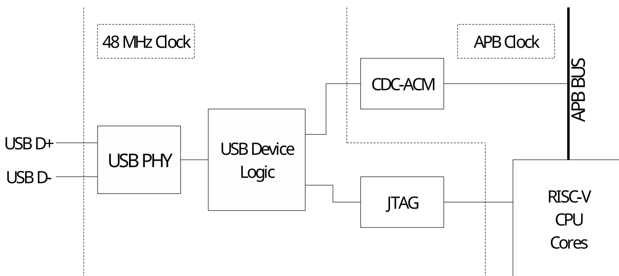
图 49.2-1. USB 串口/JTAG 控制器高层框图
