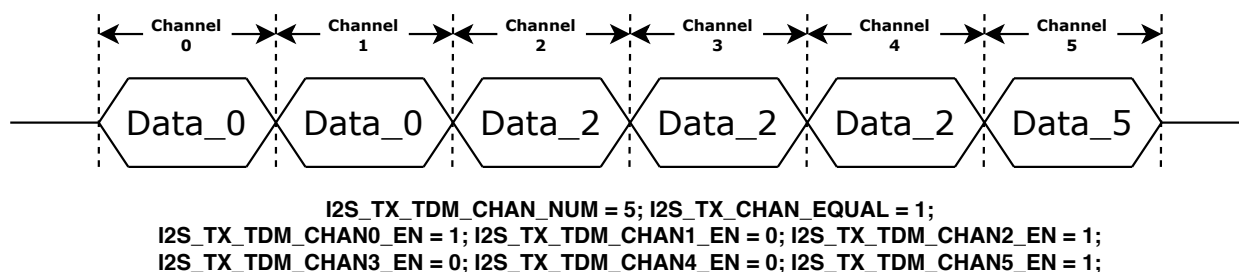
图 44.9-2. TDM 通道控制
