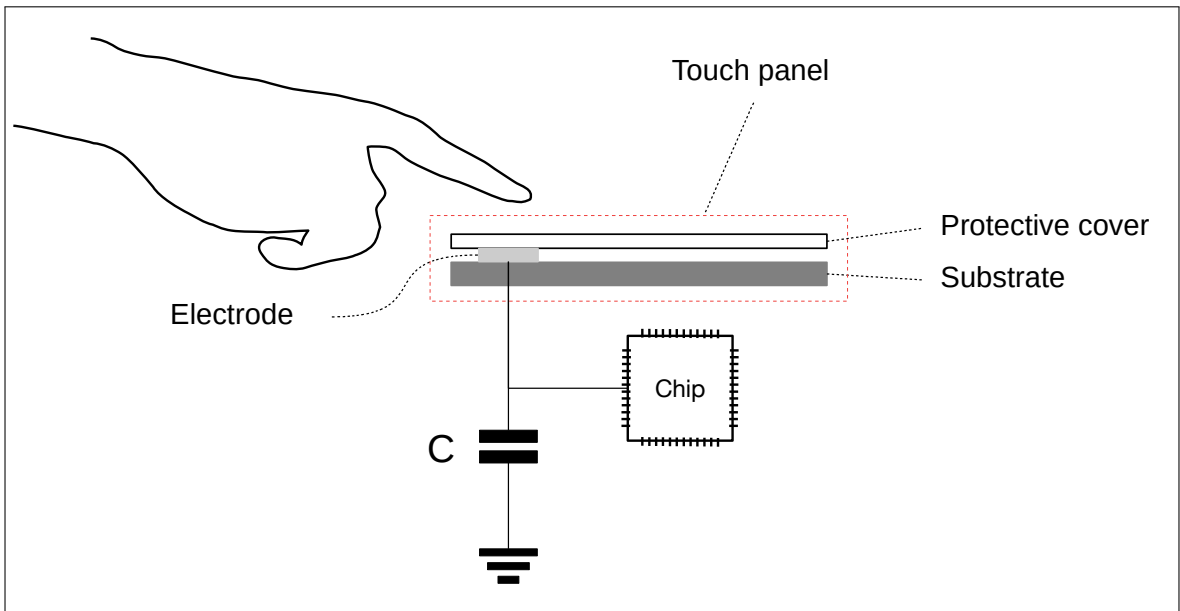
图 58.3-1. 触摸传感器系统
