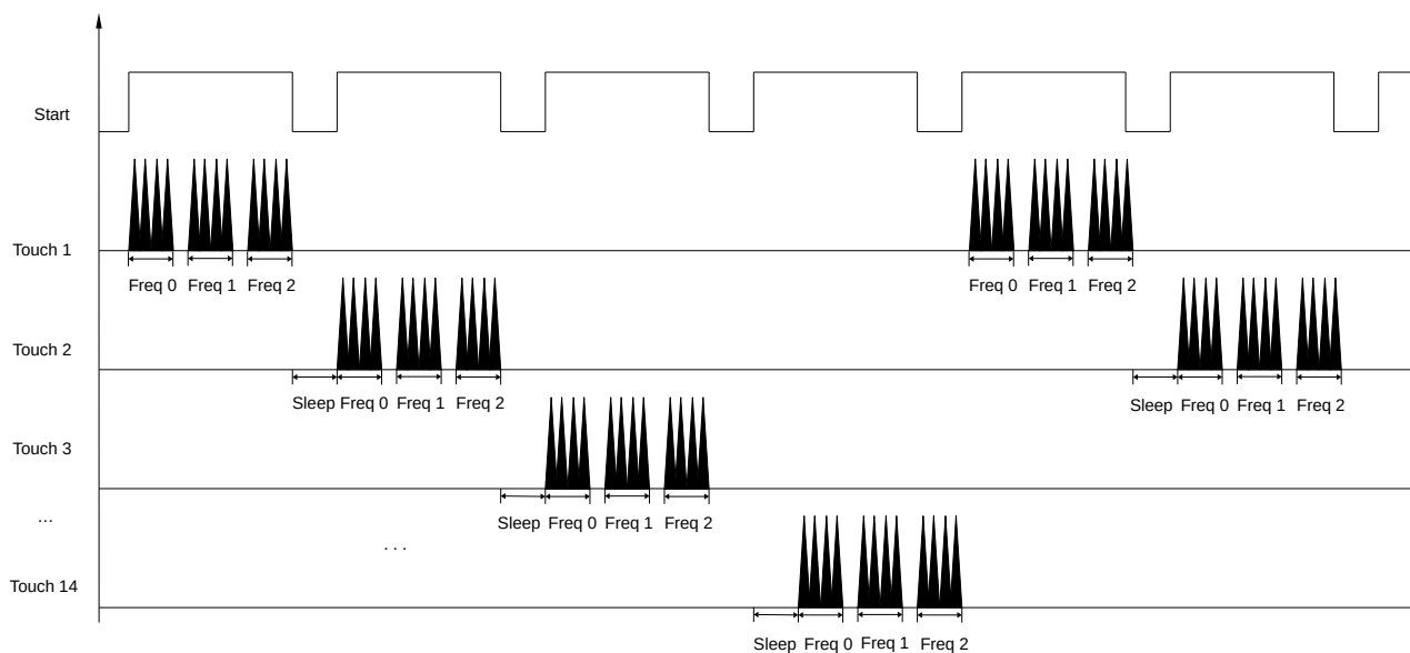
图 58.4-4. 触摸传感器跳频时序图
