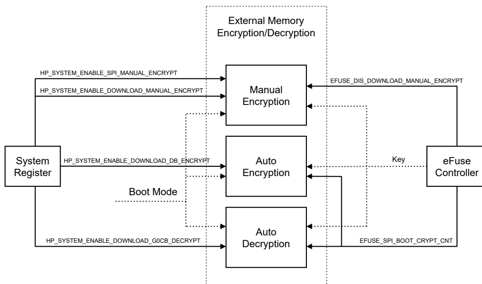
图 31.3-1. 片外存储器加解密结构
