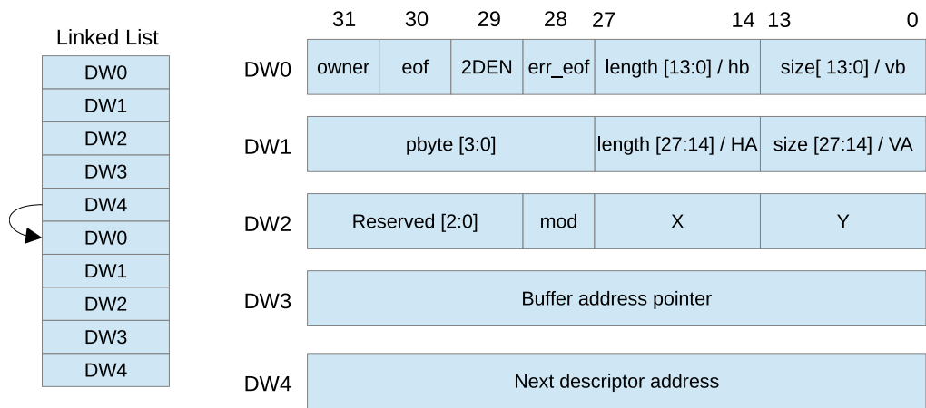
图 6.4-1. 链表结构图
