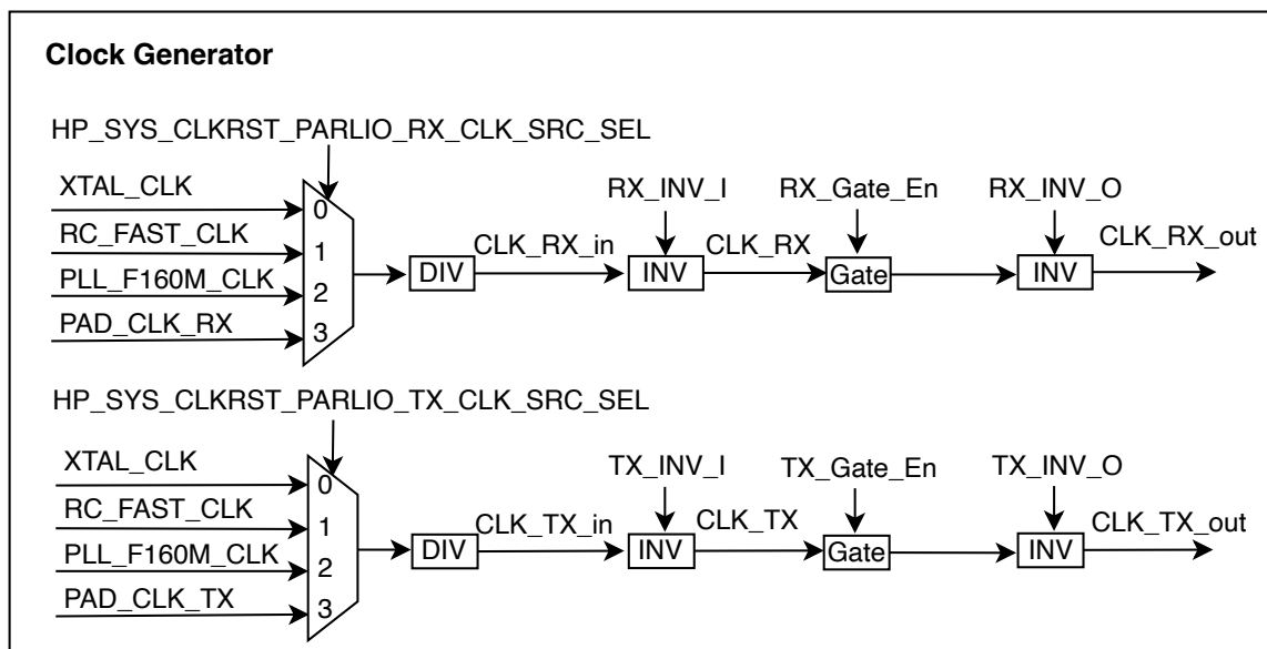
图 56.5-1. PARLIO 时钟生成
