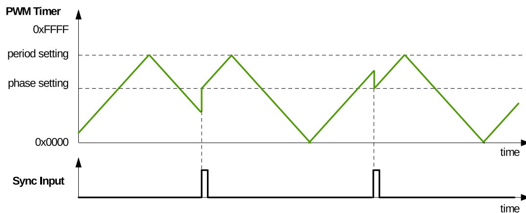
图 54.3-8. 递增递减循环模式波形，同步事件后递增
