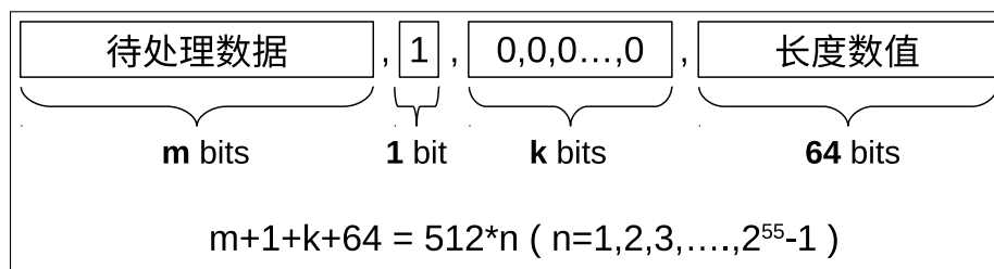
图 26.3-1. HMAC 附加填充位示意图
