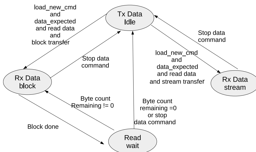
图 52.4-4. 数据接收状态机
