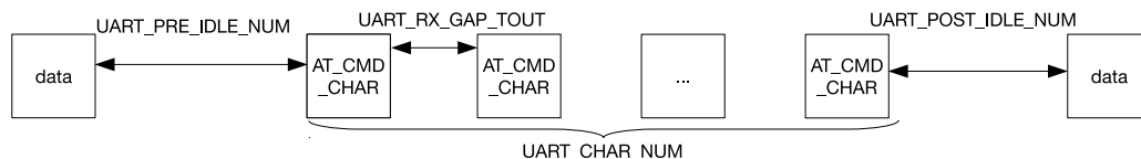
图 40.4-4. AT_CMD 字符格式
