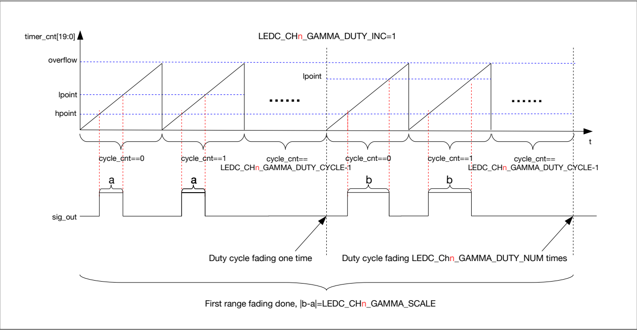
图 53.4-4. 输出信号占空比线性渐变图
