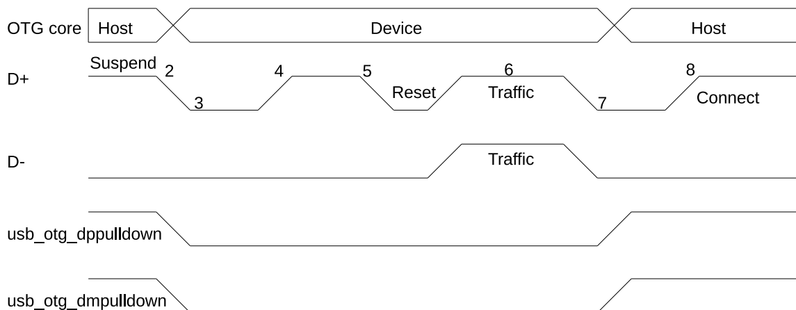
图 48.5-3. A 设备 HNP
