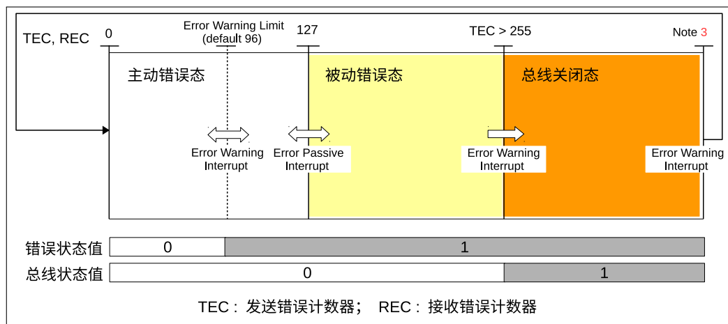
图 51.4-4. 错误状态变化
