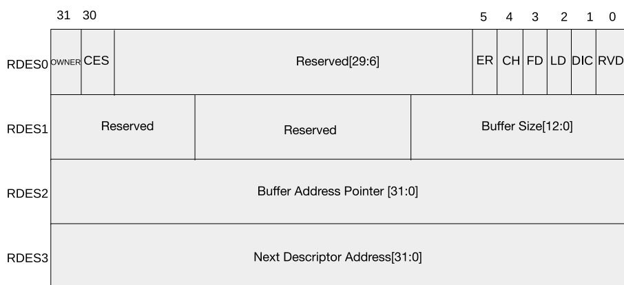
图 52.8-1. 描述符结构
