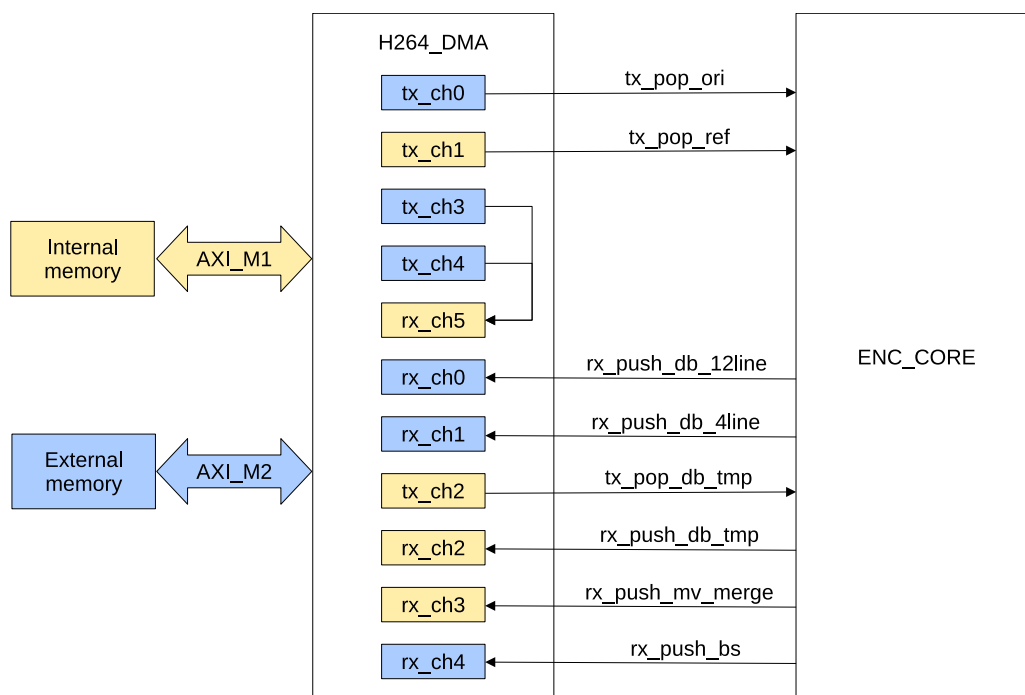
图 37.4-1. H264 编码器架构
