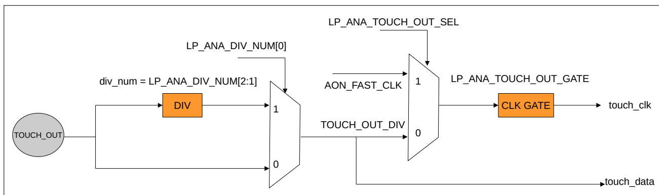
图 58.4-2. TOUCH_OUT 信号预处理
