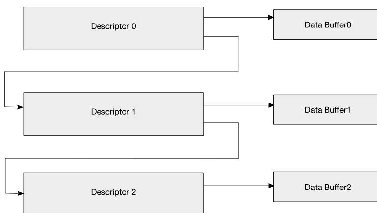
图 52.7-1. 链表结构
