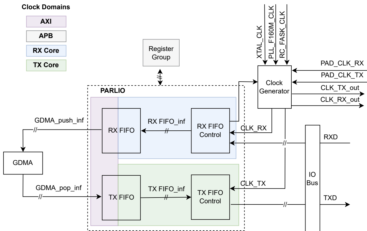
图 56.4-1. PARLIO 系统框图
