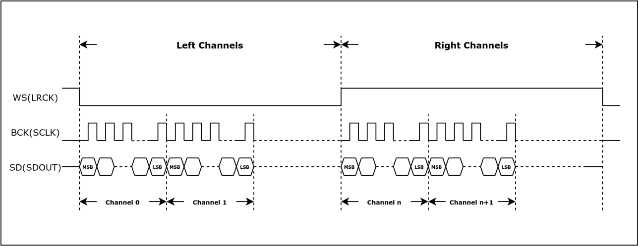
图 44.5-2. 时序图 – TDM MSB 对齐标准
