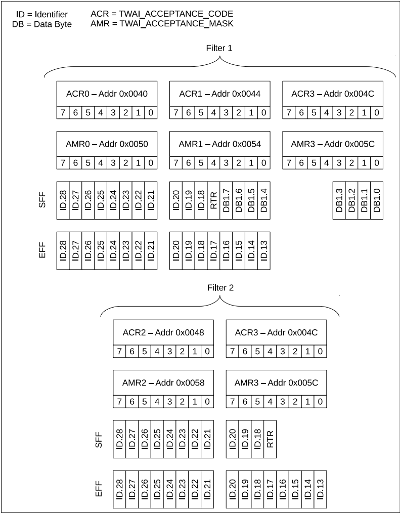
图 51.4-3. 双过滤模式
