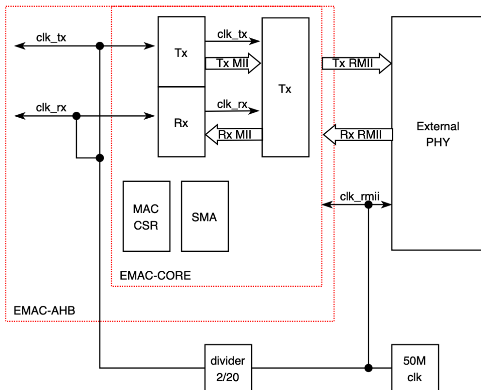
图 50.4-6. RMII 时钟
