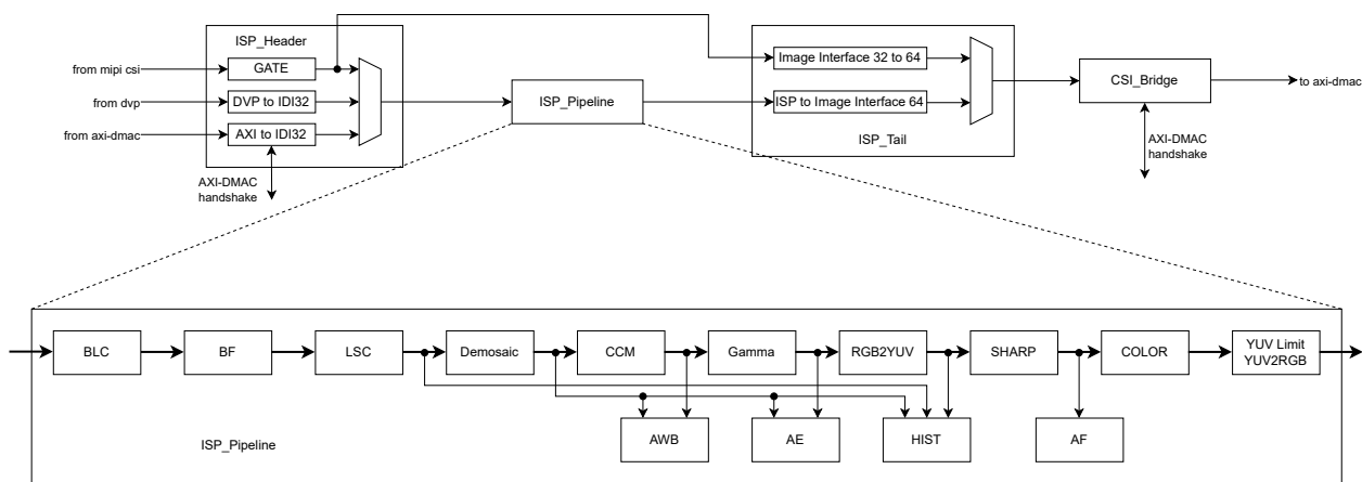
图 34.4-1. ISP 架构
