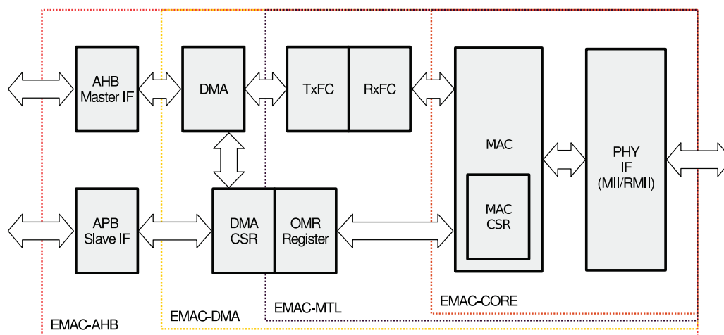
图 50.3-1. EMAC 功能框图
