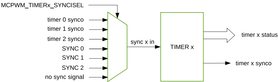
图 54.3-1. 定时器模块
