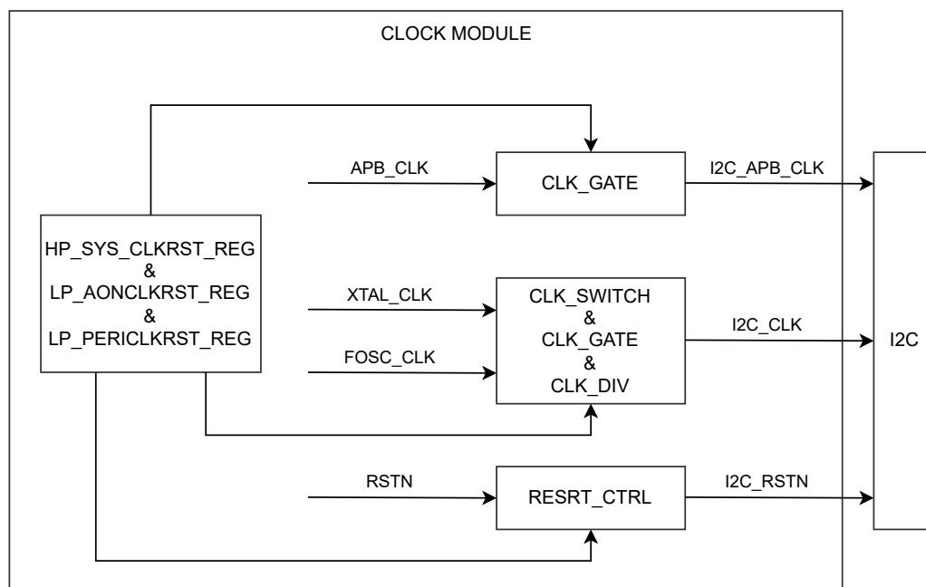
图 10.3-1. 时钟配置示例
