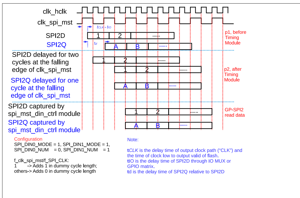
图 41.8-2. GP-SPI2 主机模式下时序补偿
