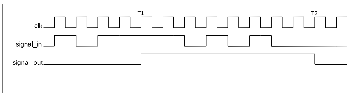
图 9.4-3. 毛刺滤波器时序示例
