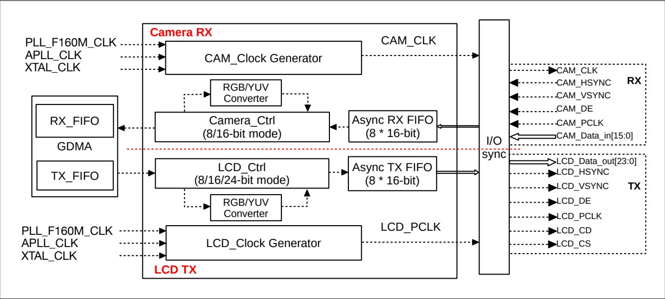
图 36.3-1. LCD_CAM 功能框图
