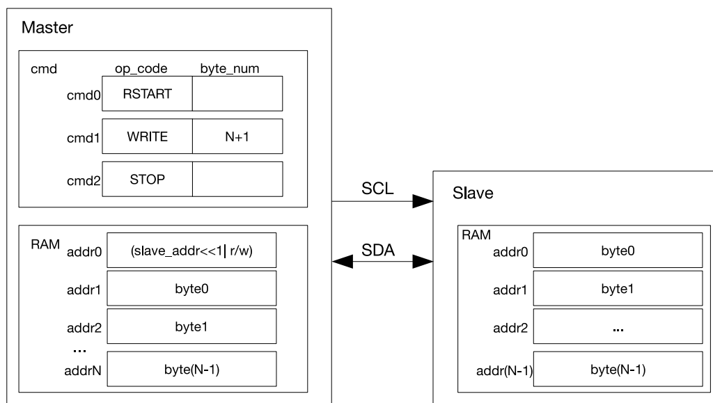
图 42.6-1. I2C 主机写 7 位寻址的从机
