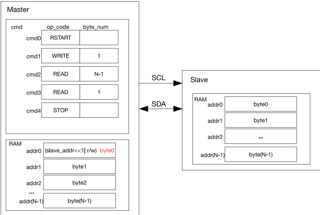
图 42.6-5. I2C 主机读 7 位寻址的从机
