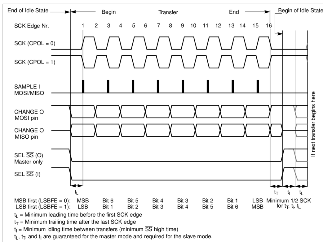
图 41.7-1. SPI 时钟模式 0 和时钟模式 2
