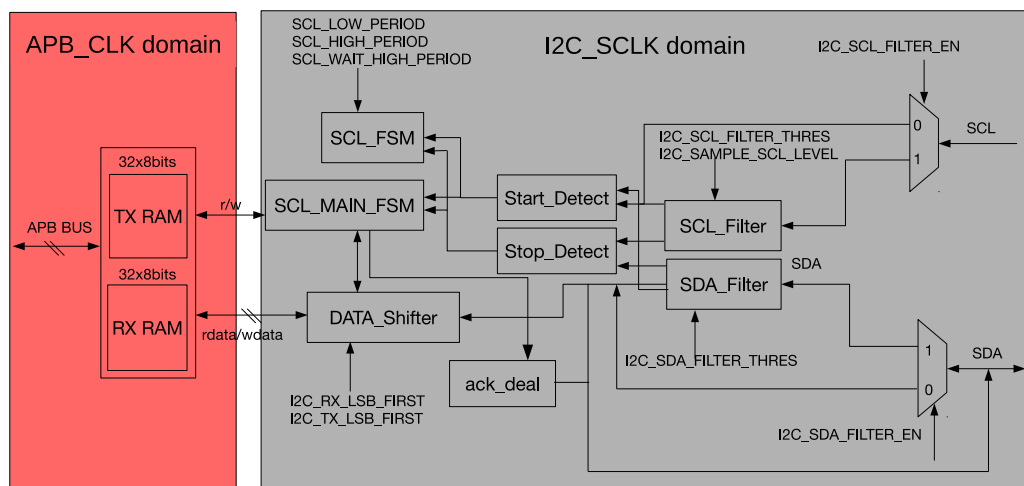
图 42.3-2. I2C 从机基本架构
