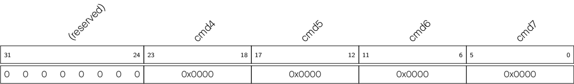
图 60.5-3. ADC_SAR x _PATT_TAB2_REG 包含样式 4 - 7
