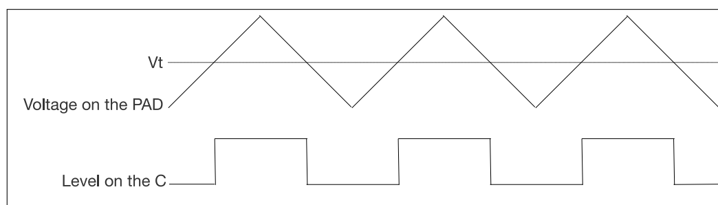
图 9.10-1. 未使能迟滞功能时 PAD 上的电平翻转示例
