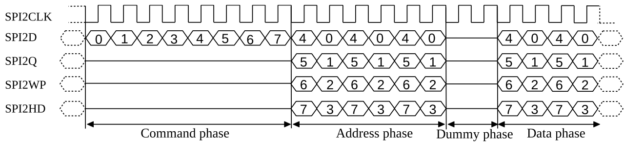
图 41.5-8. GP-SPI2 发送到 Flash 的 SPI Quad I/O Read 命令序列
