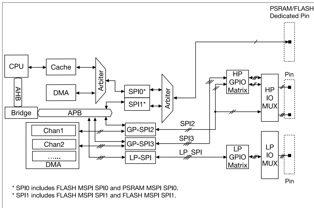
图 41.4-1. SPI 模块概览
