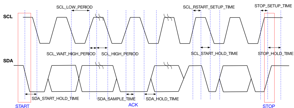
图 42.4-1. I2C 时序图
