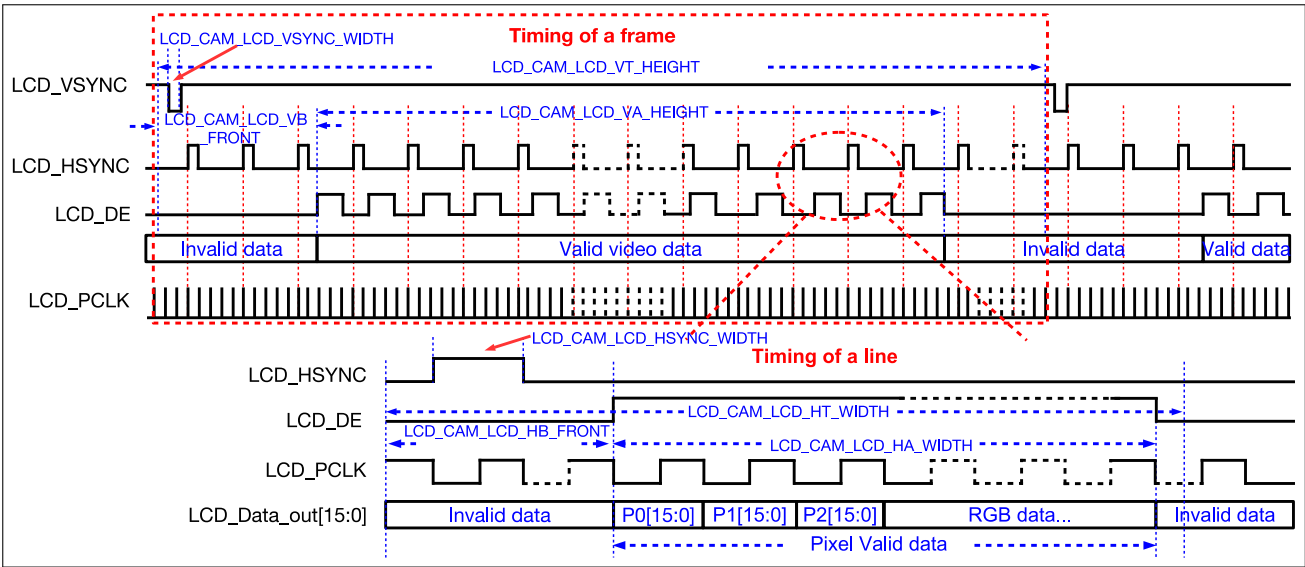
图 36.3-5. LCD 时序 (RGB 格式)
