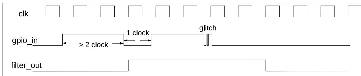
图 9.4-2. GPIO 输入信号滤波时序图
