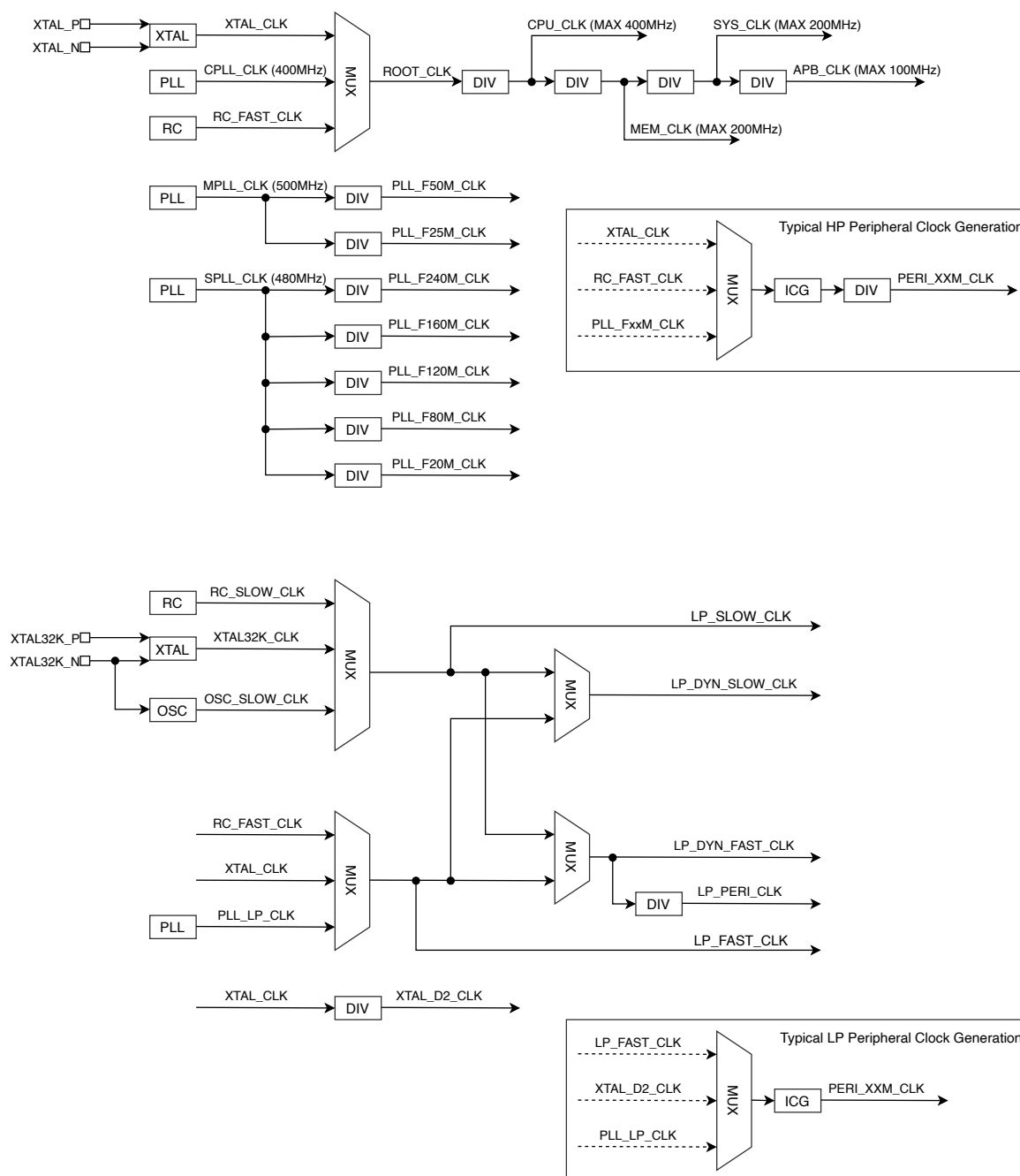
图 10.2-1. HP/LP 系统时钟
