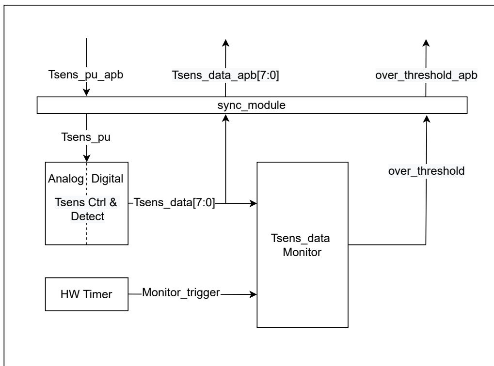
图 59.3-1. 温度传感器结构框图
