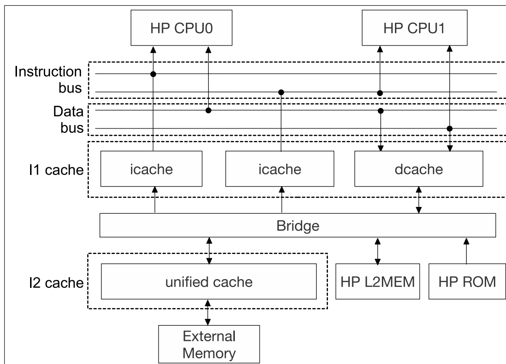
图 7.3-2. cache 结构
