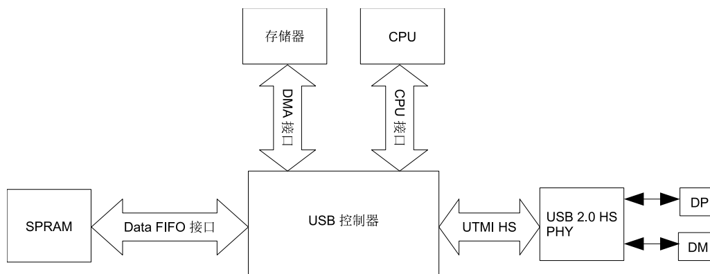
图 47.4-1. OTG_HS 系统架构
