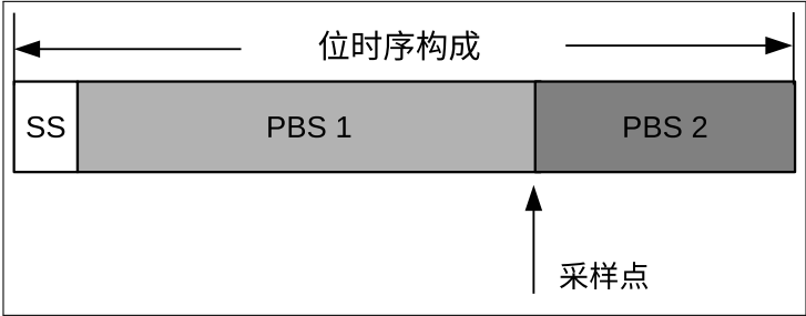
图 51.2-5. 标称位构成
