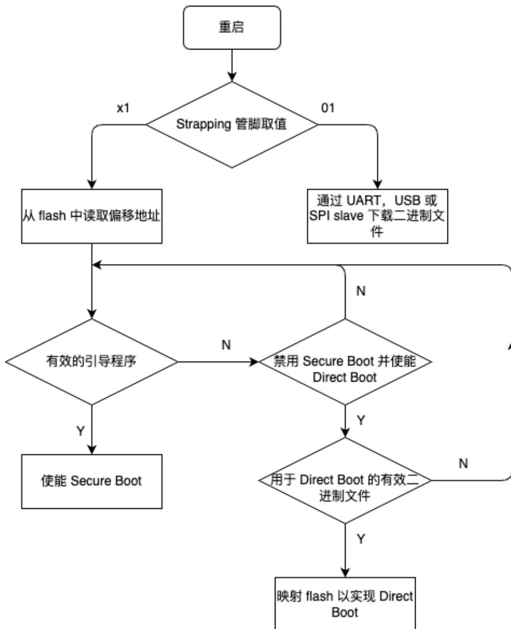
图 11.2-1. 芯片 Boot 流程
