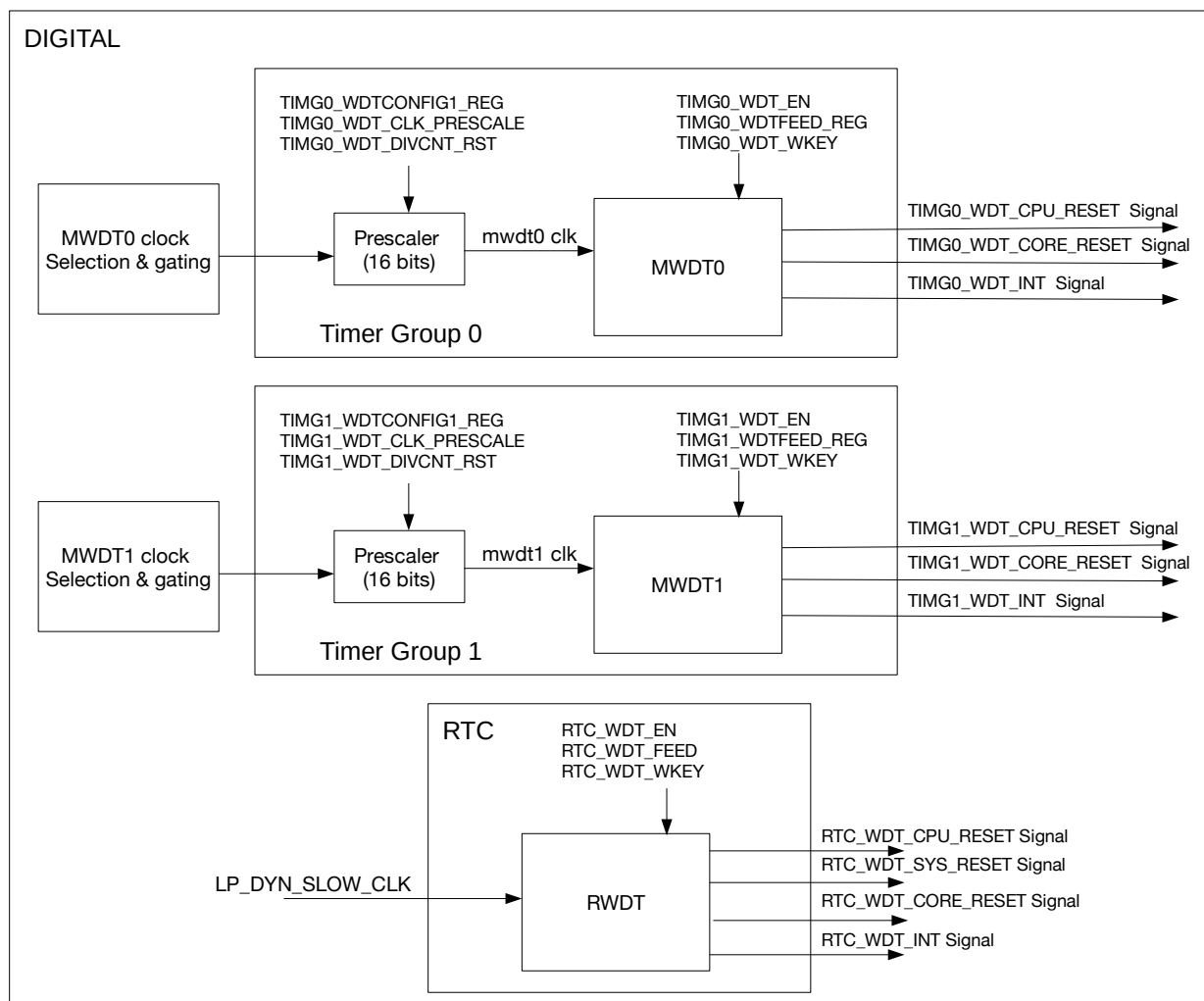
图 17.2-1. ESP32-P4 的数字看门狗定时器
