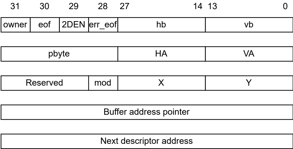
图 35.5-3. 2D-DMA 链表
