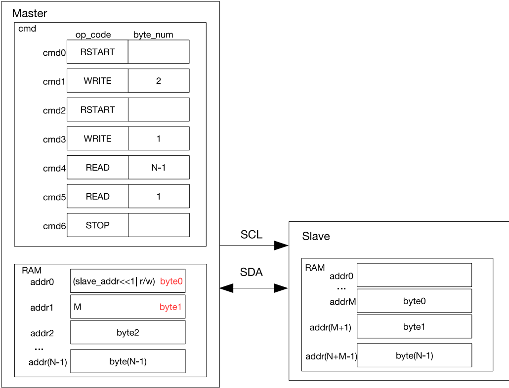
图 42.6-7. I2C 主机从 7 位双寻址从机的 M 地址读取 N 个数据
