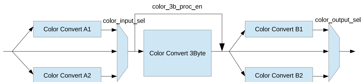
图 6.4-5. 颜色空间转换示意图
