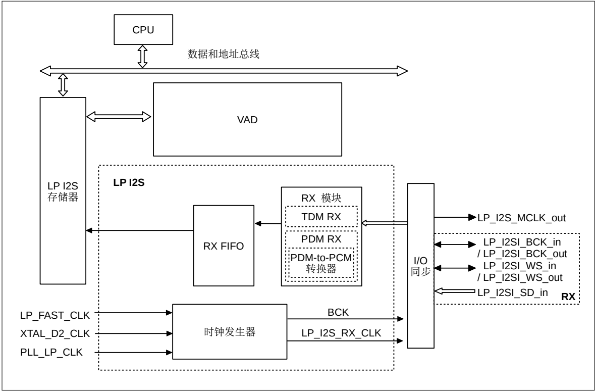
图 45.3-1. ESP32-P4 LP I2S 系统架构
