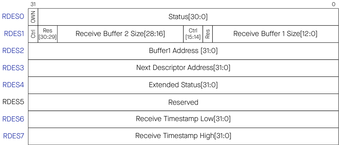
图 50.4-2. 接收链表结构
