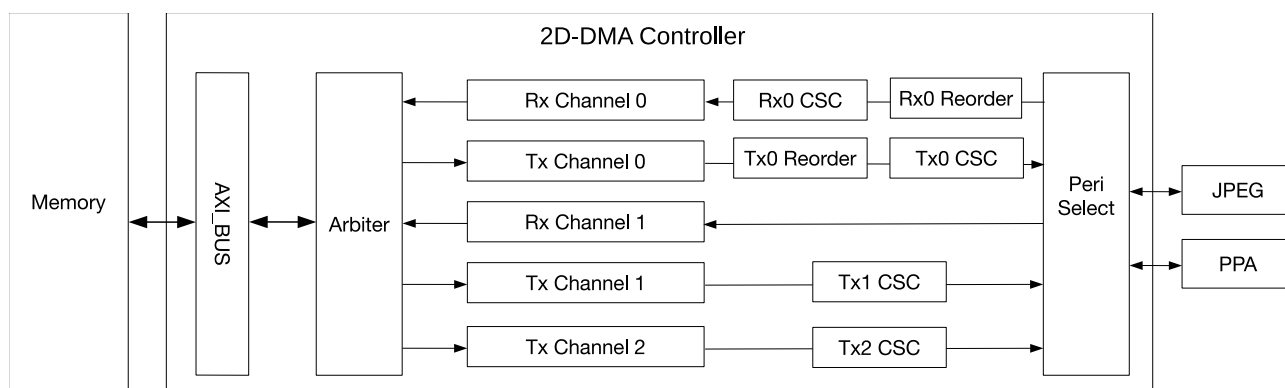
图 6.3-1. 2D-DMA 基本架构图
