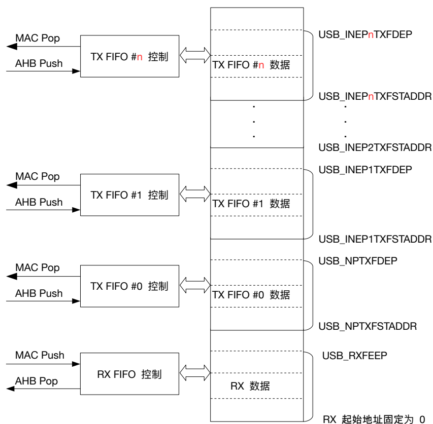
图 47.4-4. 设备模式 FIFO
