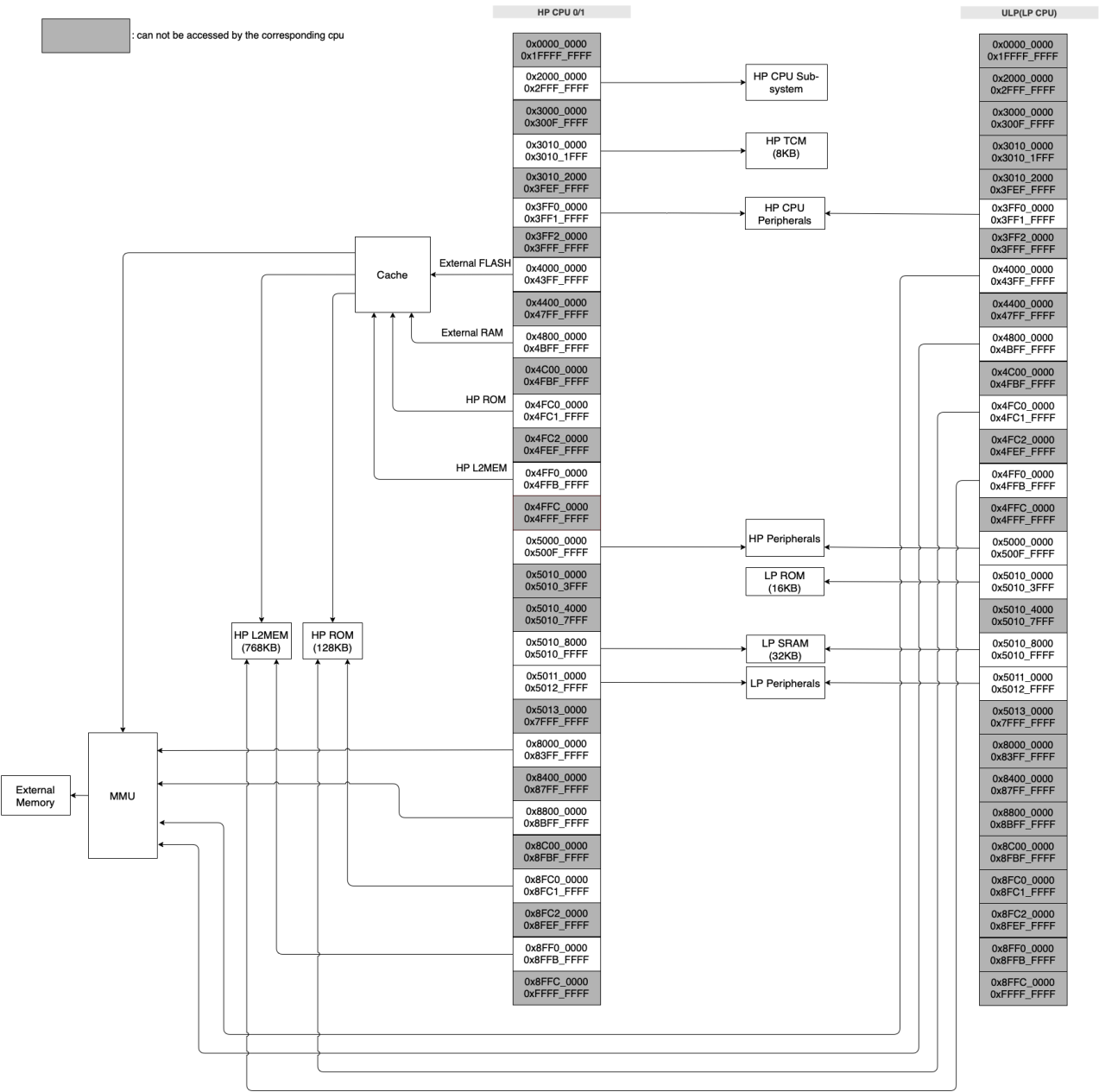
图 7.3-1. 系统结构和地址映射
