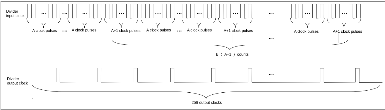
图 53.4-1. LEDC_CLK_DIV 为非整数时的分频
