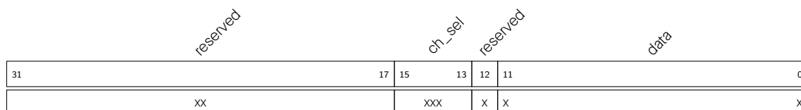
图 60.5-9. GDMA 数据格式
