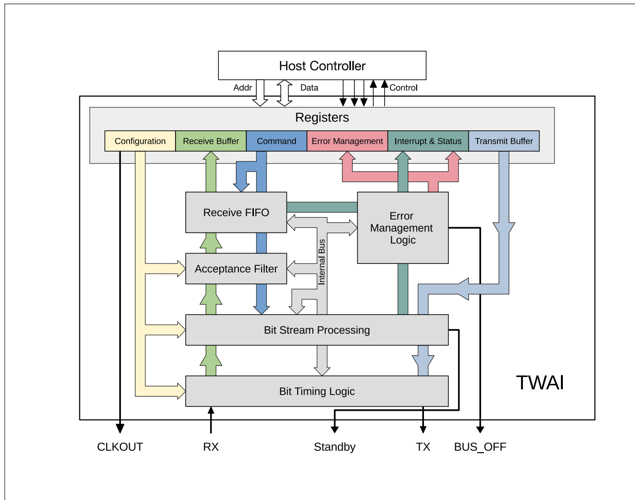
图 51.3-1. TWAI 概略图
