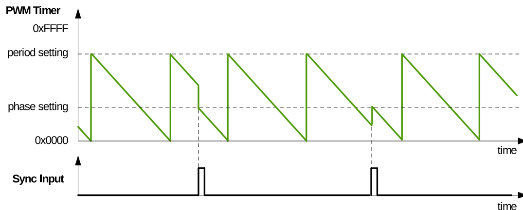
图 54.3-6. 递减计数模式波形
