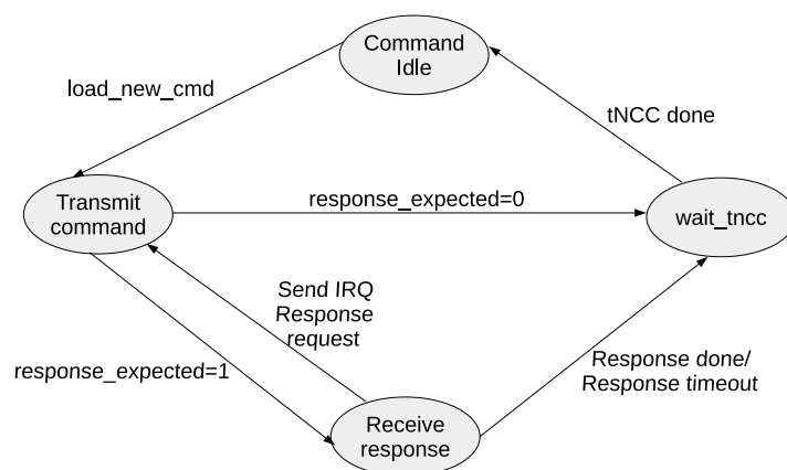
图 52.4-2. 命令通路状态机
