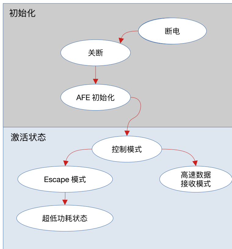
图 38.5-2. MIPI RX D-PHY 操作状态和模式
