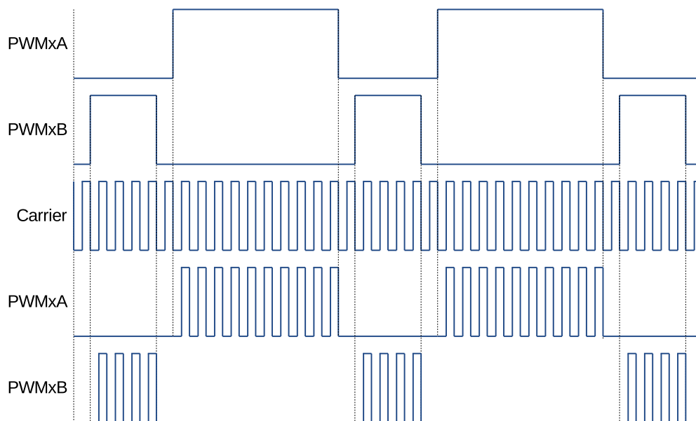
图 54.3-26. PWM 载波操作的波形示例
