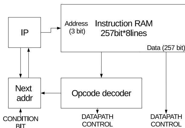
图 57.3-2. 比特调节器控制路径图
