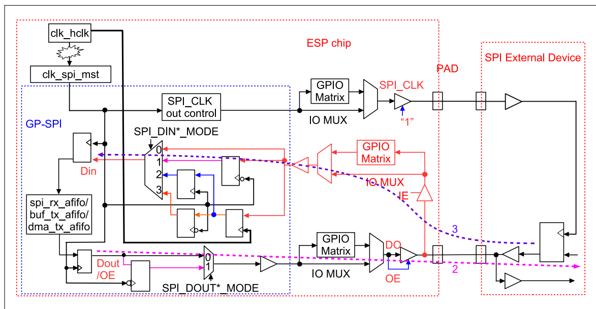
图 41.8-1. GP-SPI 主机时序补偿控制图
