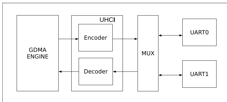
图 40.4-10. GDMA 模式数据传输
