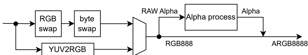
图 35.5-1. PPA SRM 输入像素处理
