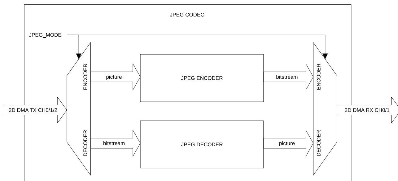
图 33.2-1. JPEG 图像编解码器的系统连接框图
