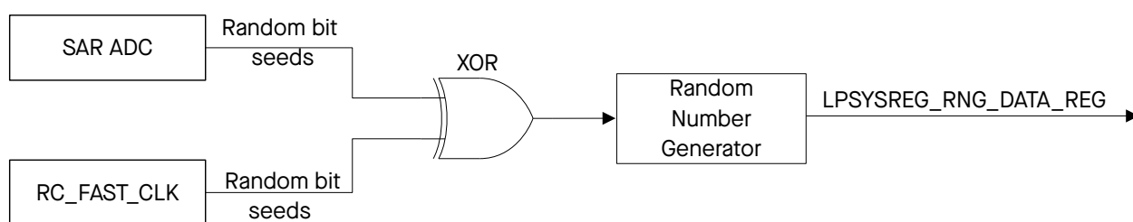
图 32.3-1. 噪声源
