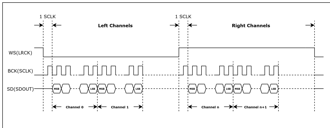
图 45.4-1. 时序图 – TDM Philips 标准
