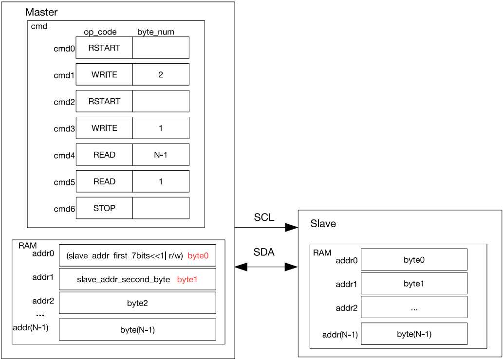
图 42.6-6. I2C 主机读 10 位寻址的从机
