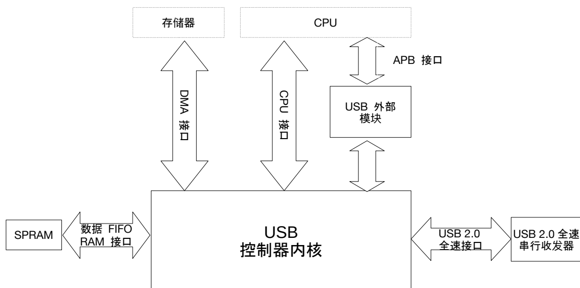
图 48.4-1. OTG_FS 系统架构
