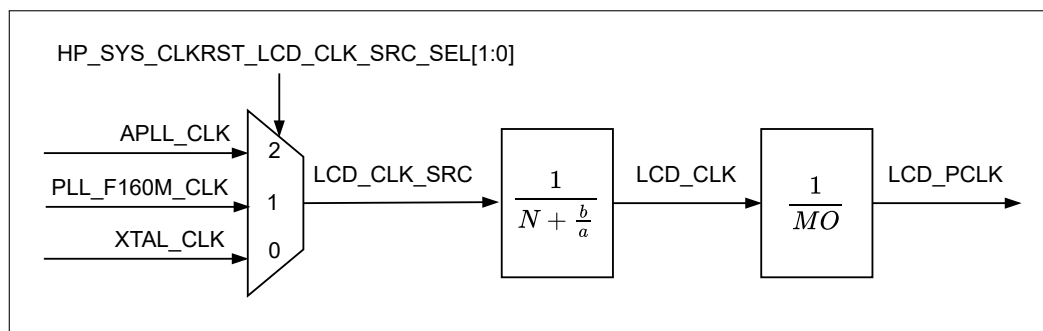
图 36.3-2. LCD 时钟
