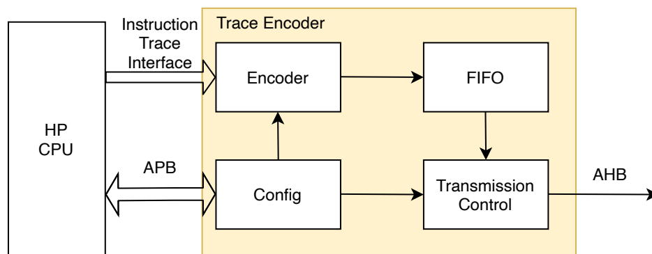
图 2.0-1. 追踪编码器概述图
