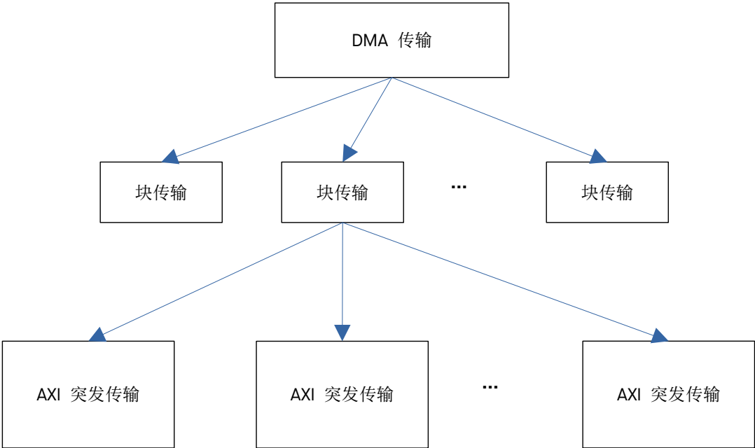
图 5.5-2. 存储器的传输层次结构
