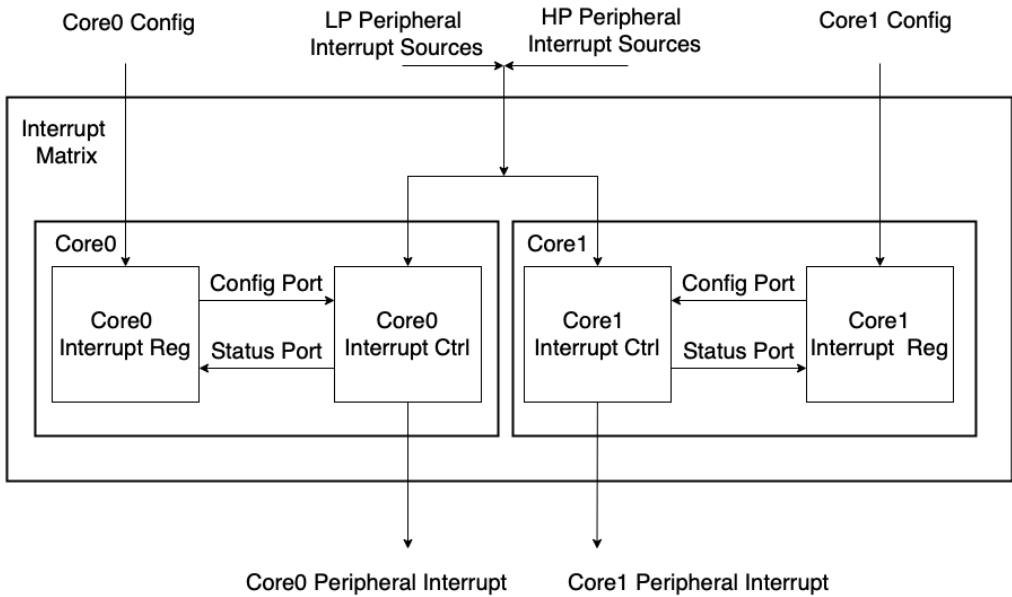
图 12.3-1. 中断矩阵结构图
