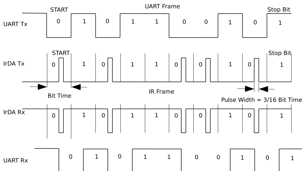
图 40.4-6. SIR 模式编解码时序图
