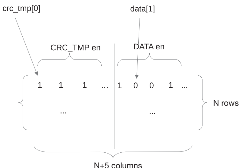
图 4.4-3. CRC 计算矩阵示意图
