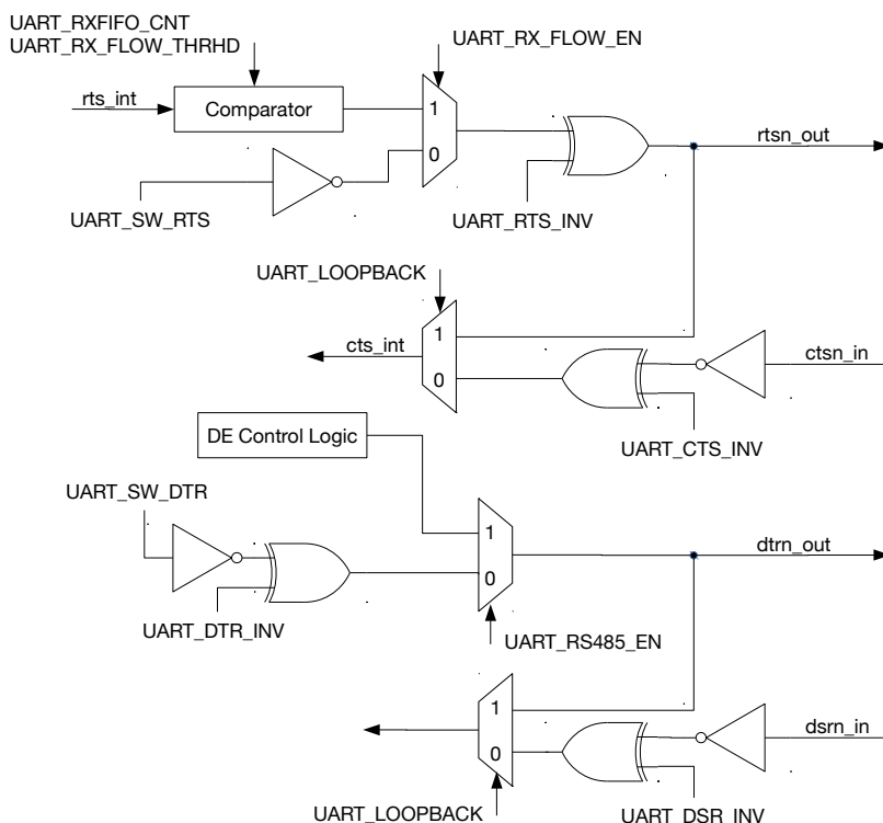
图 40.4-8. 硬件流控图
