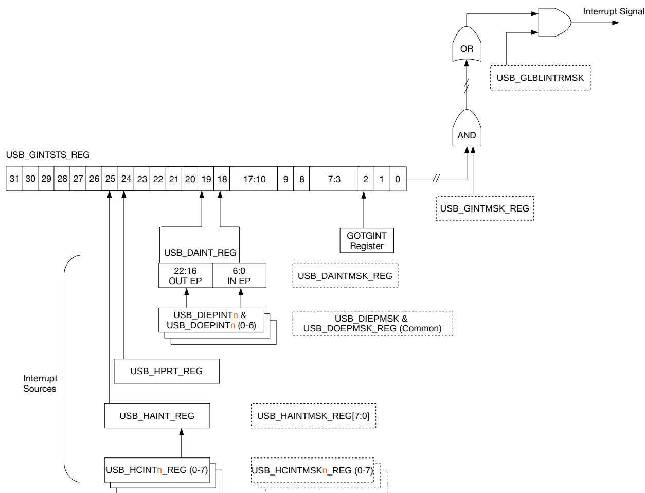
图 48.4-5. OTG_FS 中断层次结构图
