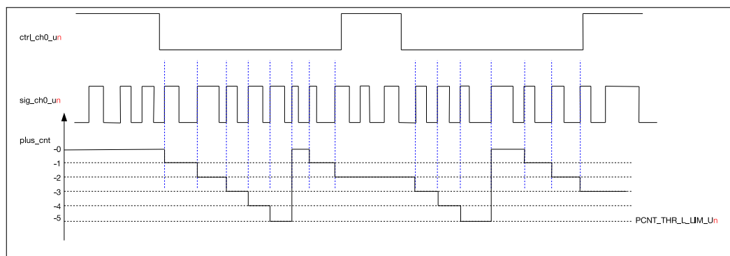
图 46.6-2. 通道 0 递减计数图
