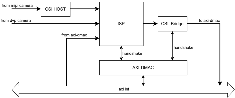
图 34.1-1. ESP32-P4 ISP 系统架构
