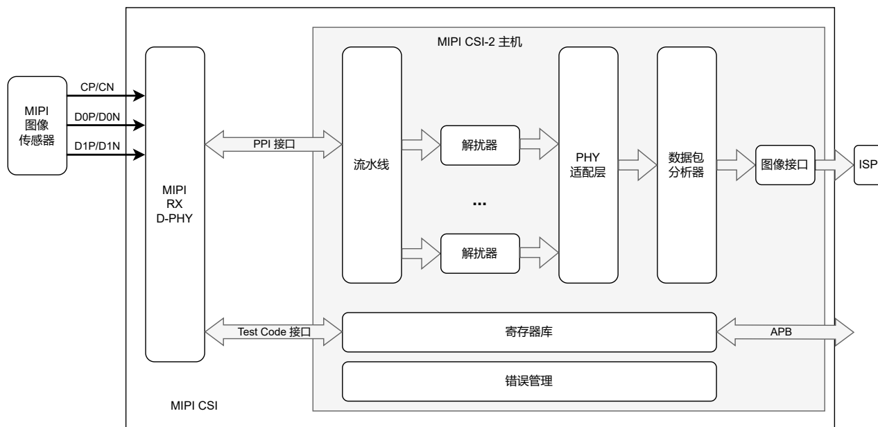
图 38.4-1. MIPI CSI 架构
