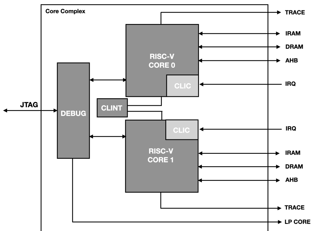
图 1.1-1. CPU 核心系统框图
