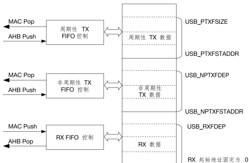
图 48.4-3. 主机模式 FIFO
