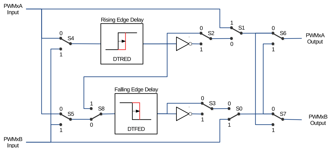
图 54.3-21. 死区模块的开关拓扑
