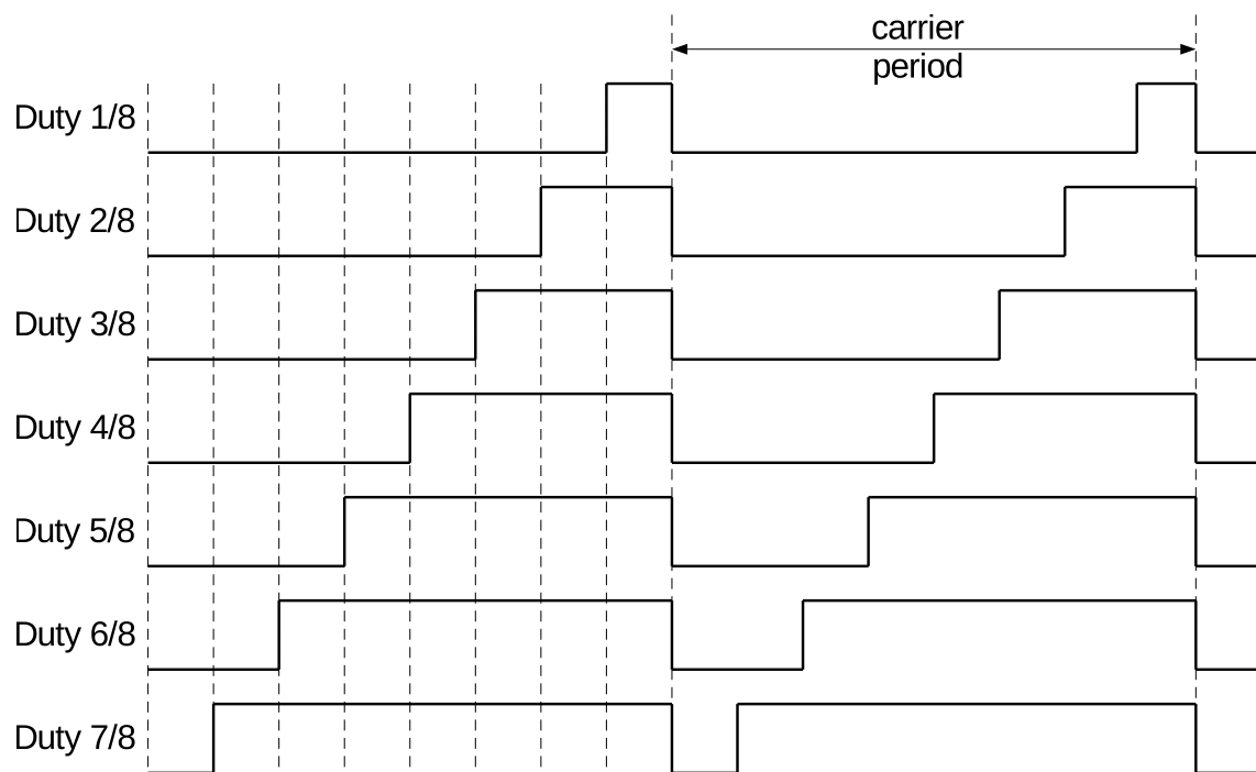
图 54.3-28. PWM 载波模块中持续脉冲的 7 种占空比设置
