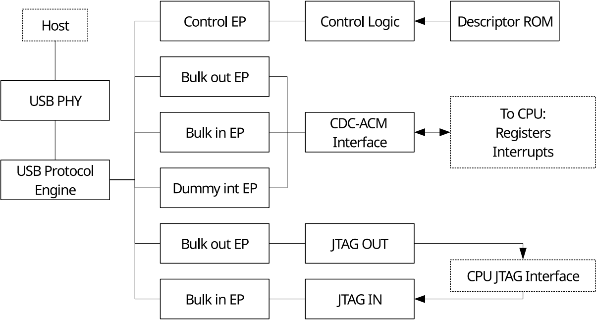
图 49.2-2. USB 串口/JTAG 控制器框图
