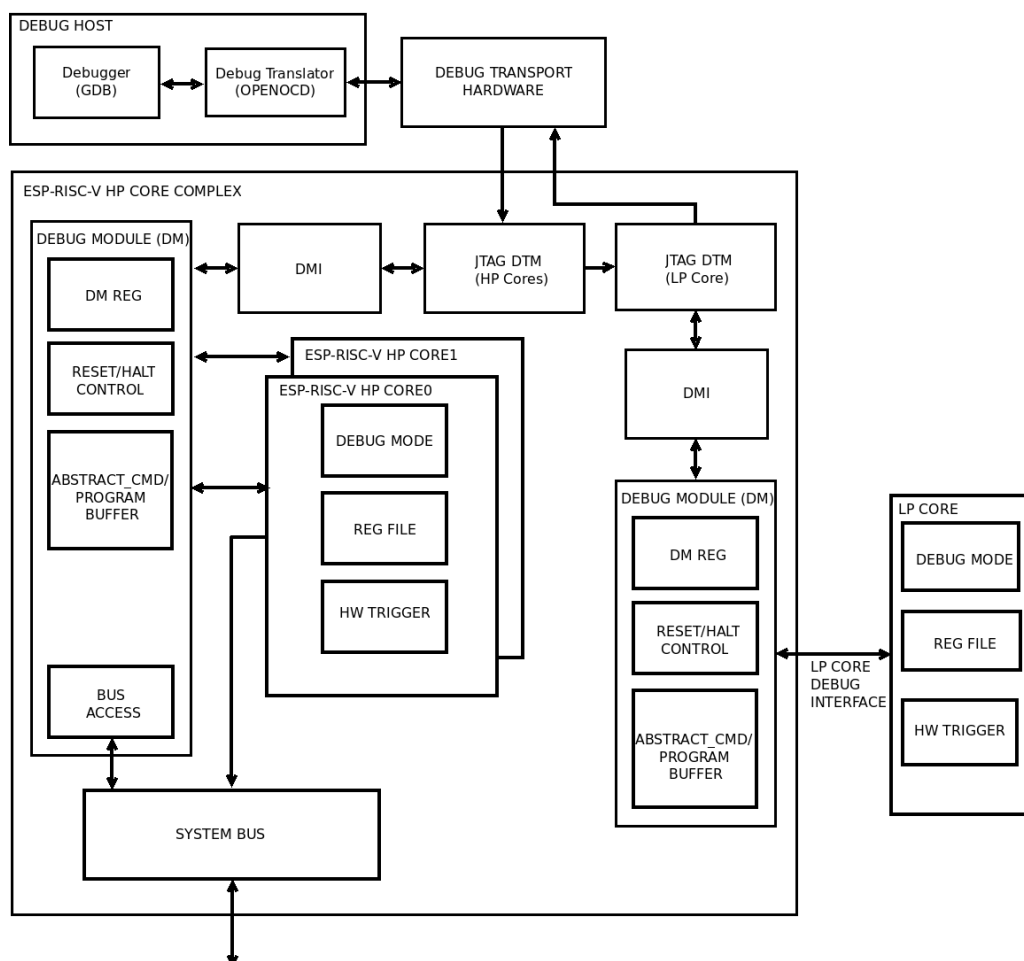
图 1.11-1. 调试系统概述
