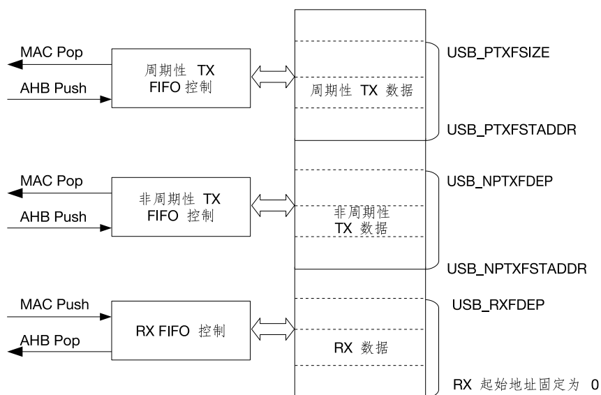
图 47.4-3. 主机模式 FIFO
