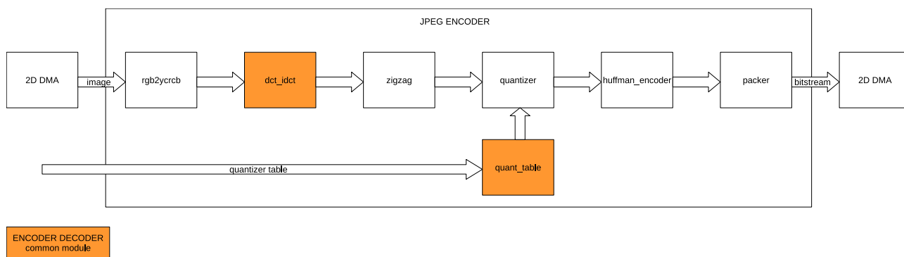
图 33.4-1. JPEG 编码器架构
