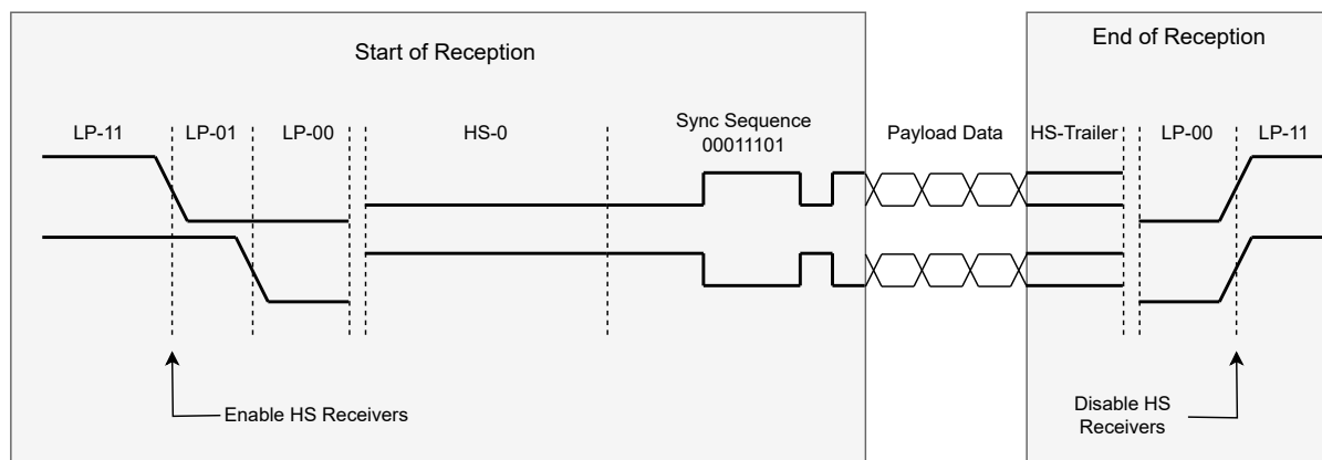
图 38.5-3. MIPI CSI HS 数据接收序列
