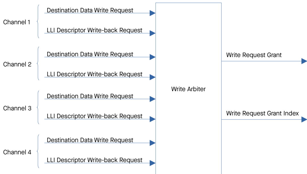
图 5.5-4. VDMA 写仲裁器
