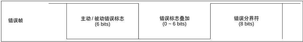
图 51.2-2. 错误帧中的位域
