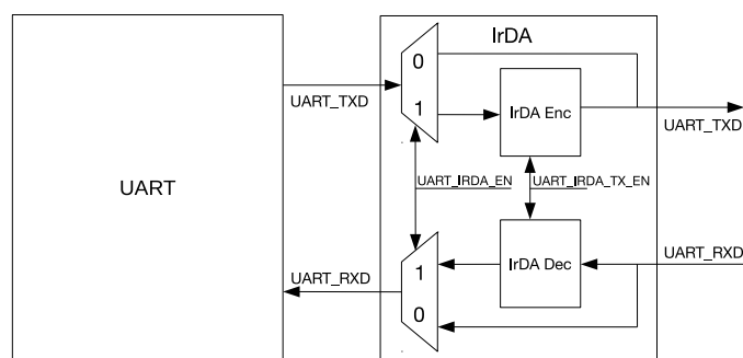
图 40.4-7. IrDA 编解码结构图
