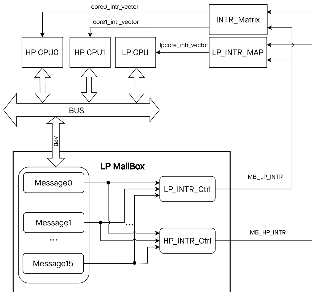
图 22.3-1. LP 信箱控制器系统框图
