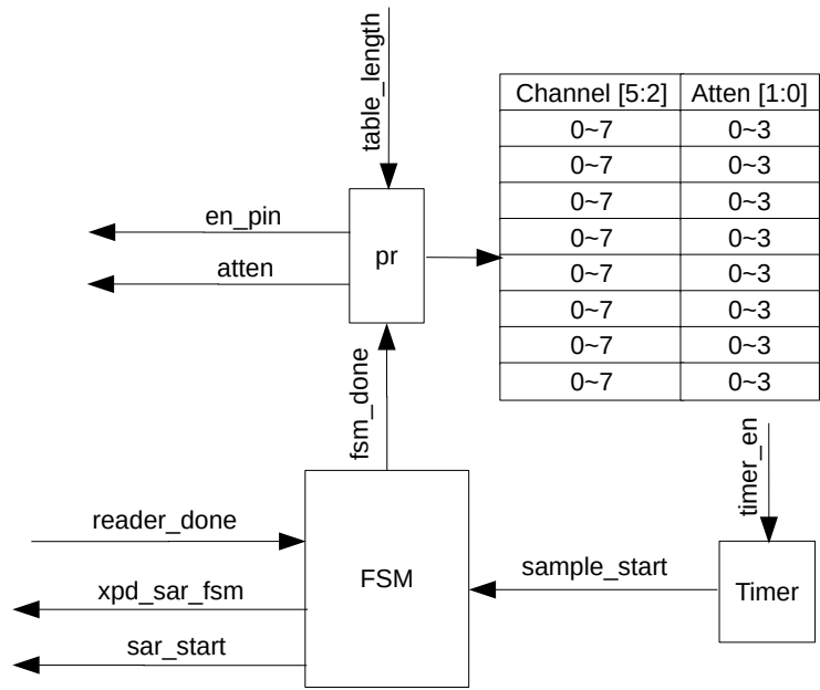
图 60.5-1. HP ADC FSM 概况
