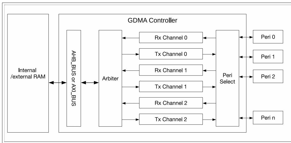
图 4.3-1. GDMA 控制器的架构
