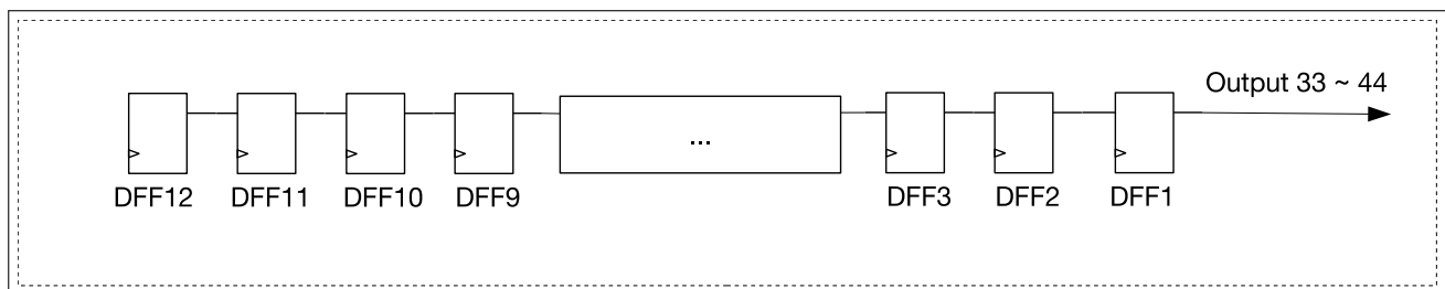
图 8.3-3. 移位寄存器电路图 (后 12 字节)
