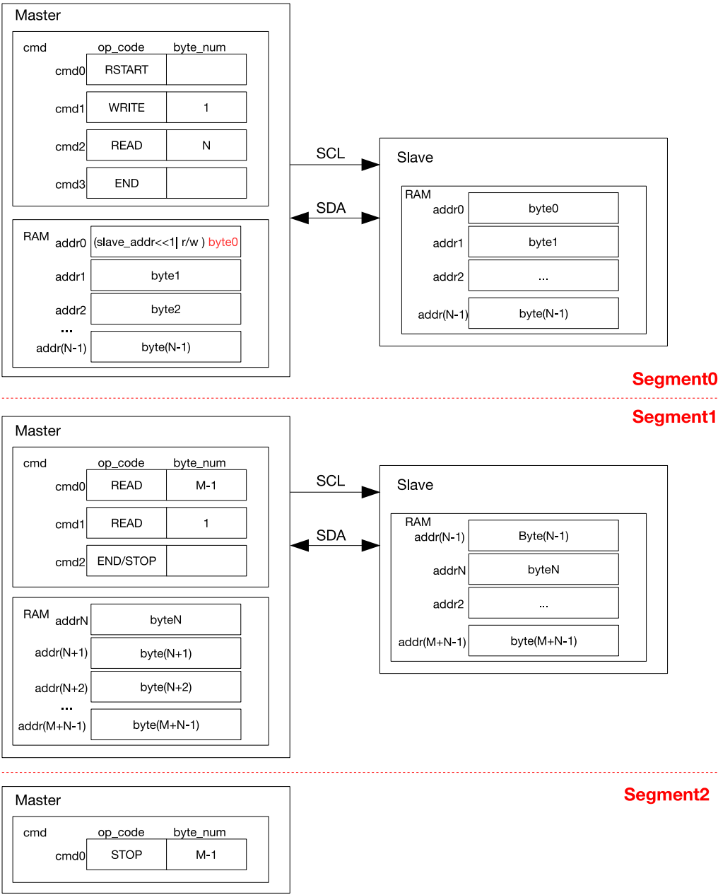
图 42.6-8. I2C 主机分段读 7 位寻址的从机
