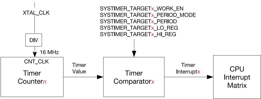
图 15.5-1. 系统定时器生成报警
