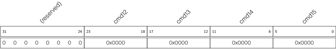
图 60.5-5. ADC_SAR x _PATT_TAB4_REG 包含样式 12 - 15
