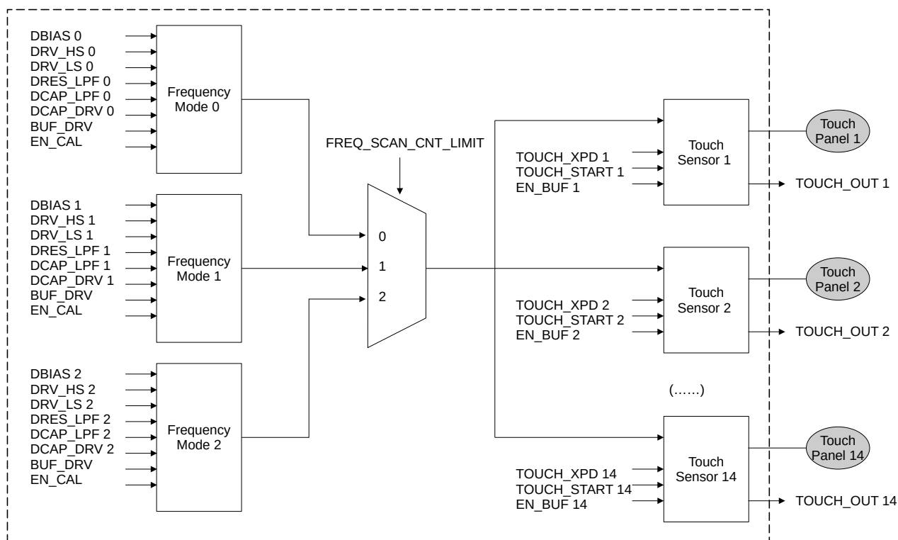
图 58.3-2. 触摸传感器内部结构
