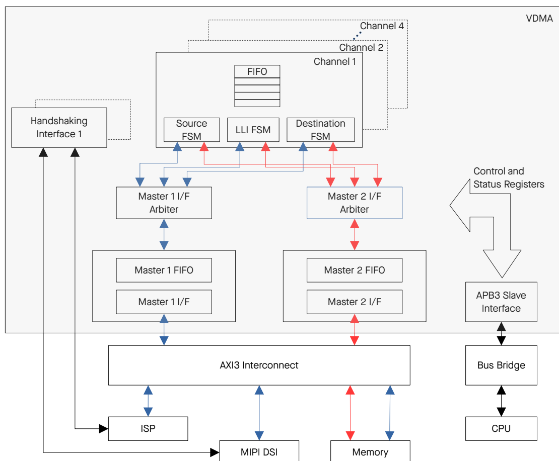
图 5.4-1. VDMA 架构
