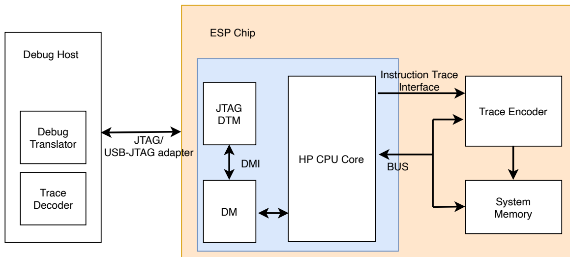
图 2.2-1. 指令追踪流程概览
