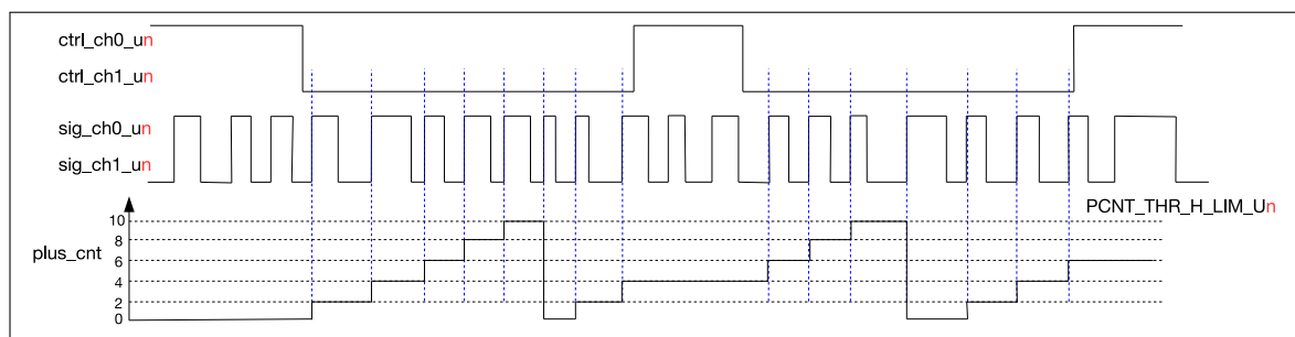
图 46.6-3. 双通道递增计数图
