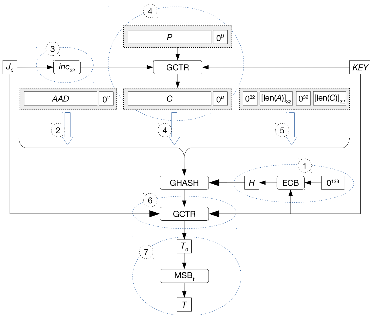
图 24.7-1. GCM 加密过程
