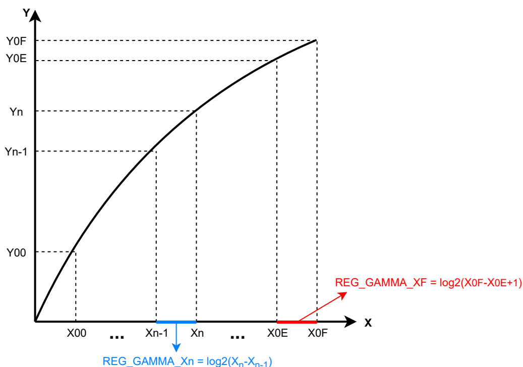
图 34.5-1. gamma 曲线示意
