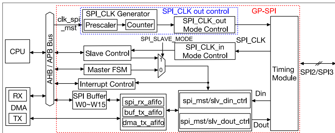
图 41.5-2. GP-SPI 功能块图
