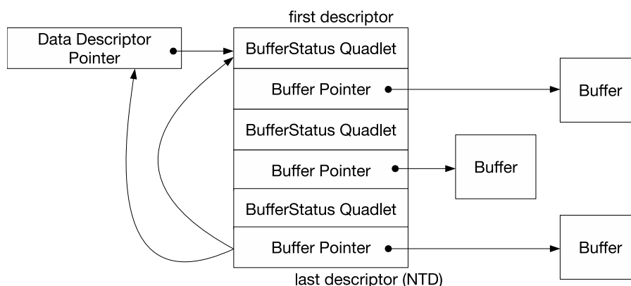
图 47.4-6. Scatter/Gather DMA 链表结构
