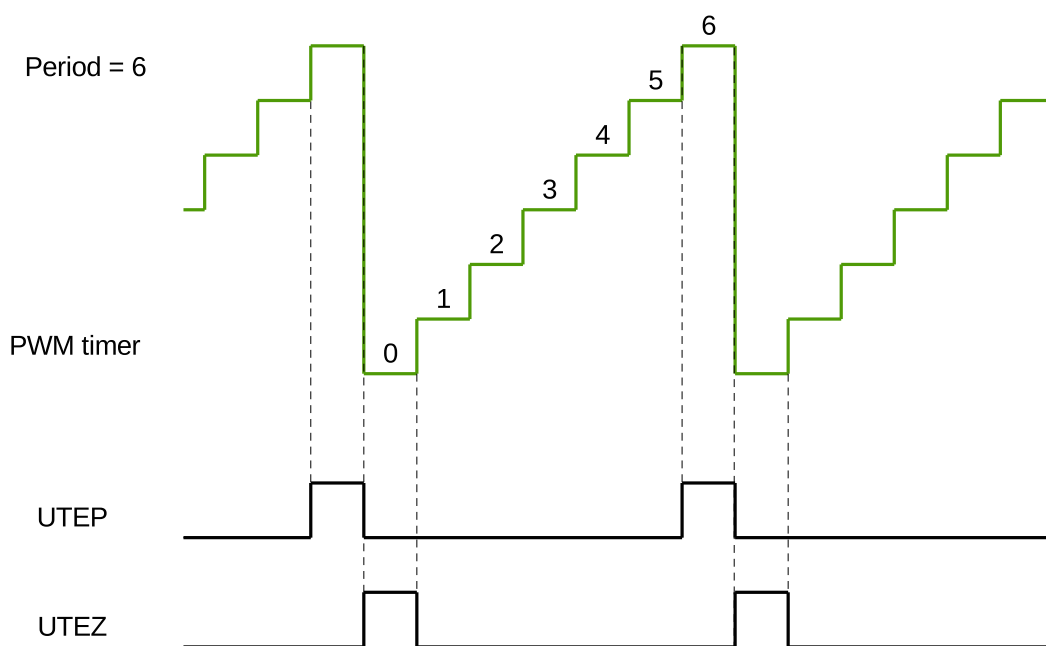
图 54.3-9. 递增模式中生成的 UTEP 和 UTEZ
