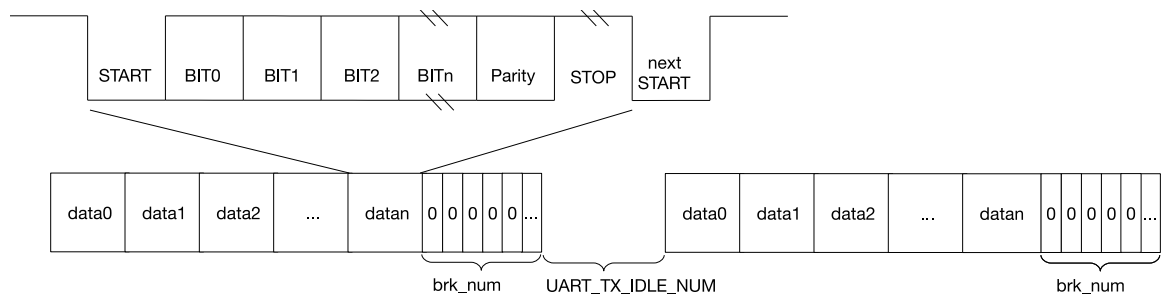
图 40.4-3. UART 数据帧结构
