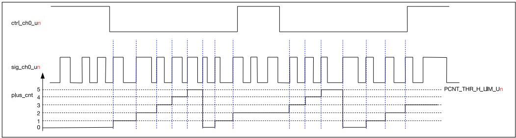
图 46.6-1. 通道 0 递增计数图
