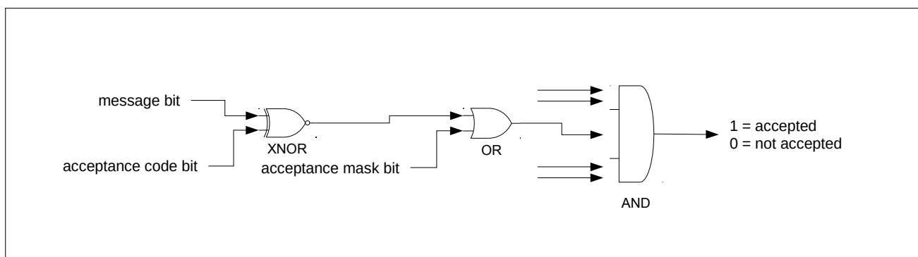
图 51.4-1. 接收过滤器
