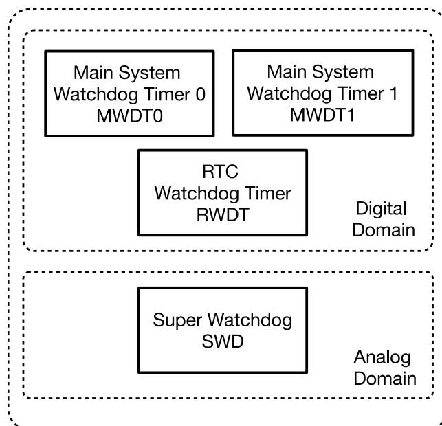
图 17.1-1. 看门狗定时器概览
