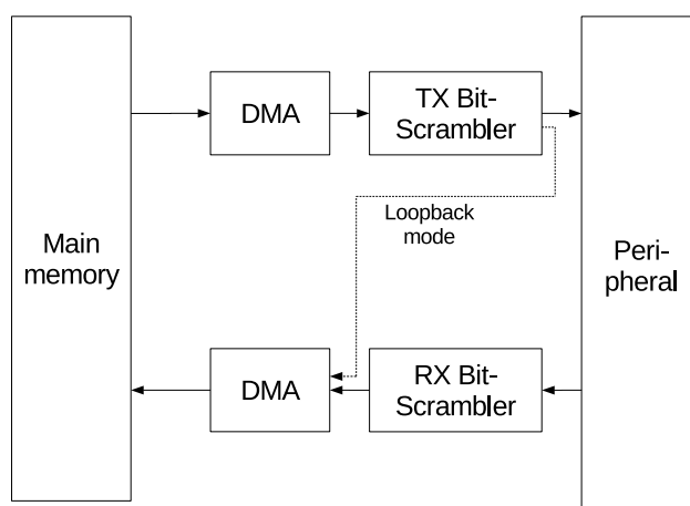
图 571-1. 比特调节器系统架构图
