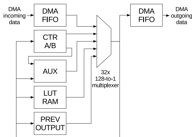
图 57.3-1. 比特调节器数据路径图
