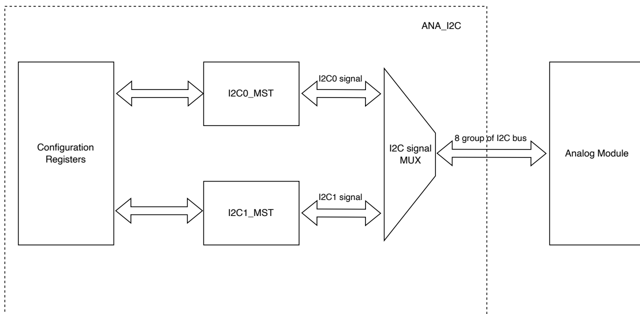
图 43.3-1. 模拟 I2C 主机模块结构图
