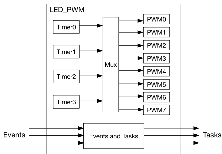
图 53.3-1. LED PWM 控制器架构
