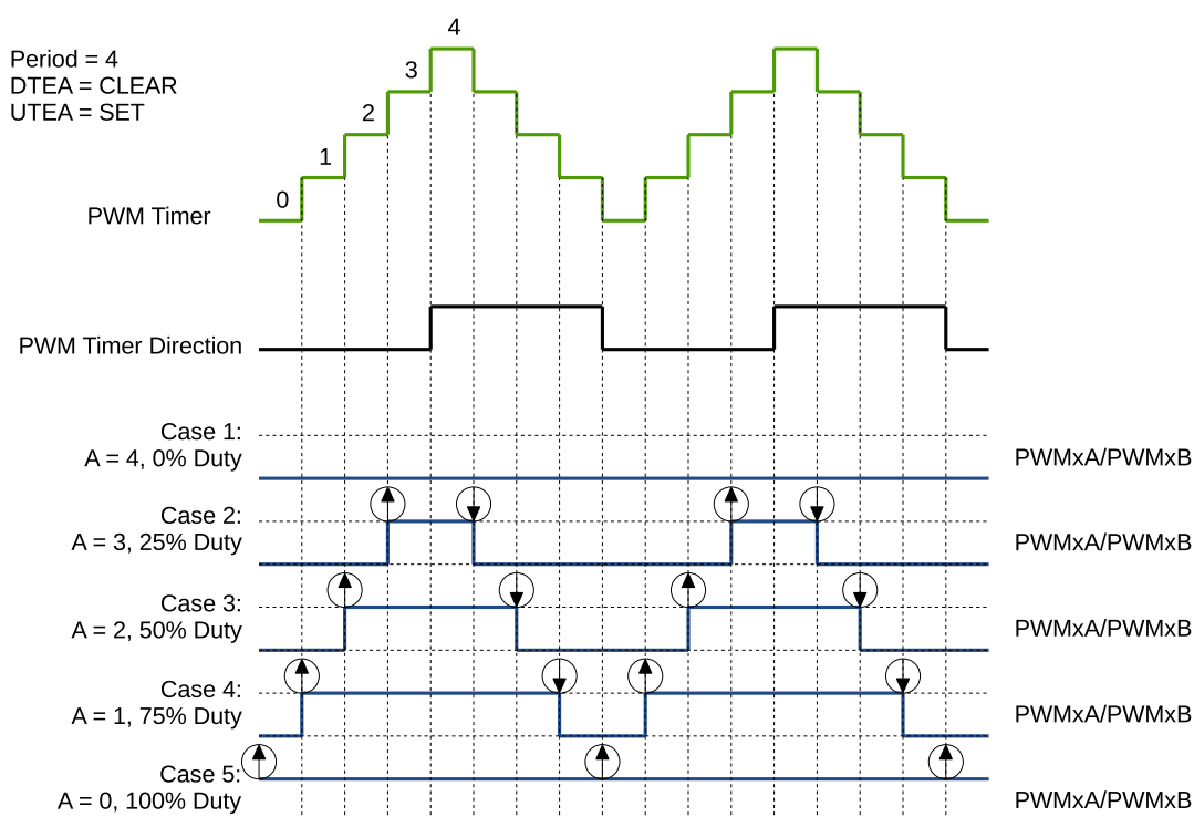
图 54.3-13. 递增递减模式下的对称波形
