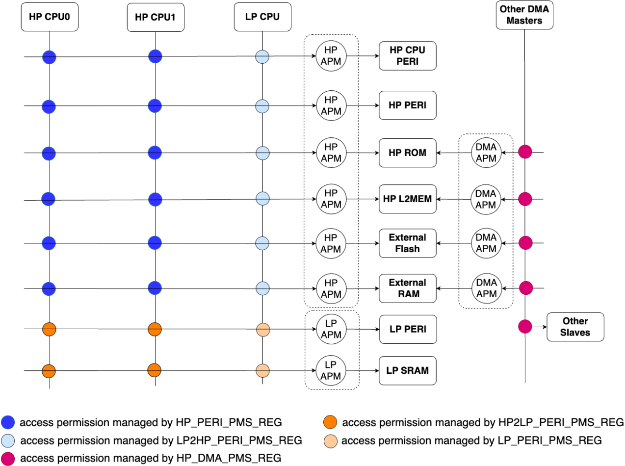
图 19.3-1. APM 控制器结构图
