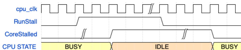
图 1.13-1. 使用 RunStall 时 CPU 核心状态的切换
