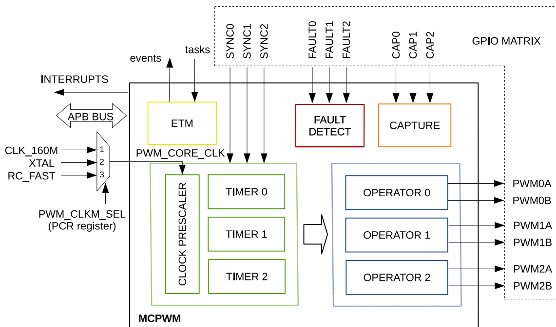
图 54.2-1. MCPWM 外设概览
