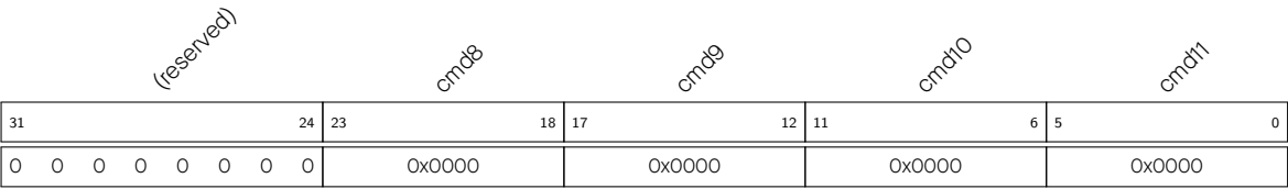
图 60.5-4. ADC_SAR x _PATT_TAB3_REG 包含样式 8 - 11
