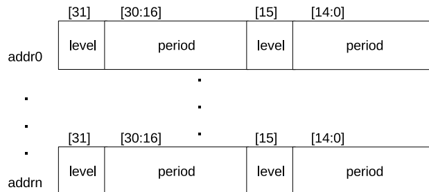
图 55.3-2. RAM 中脉冲编码结构
