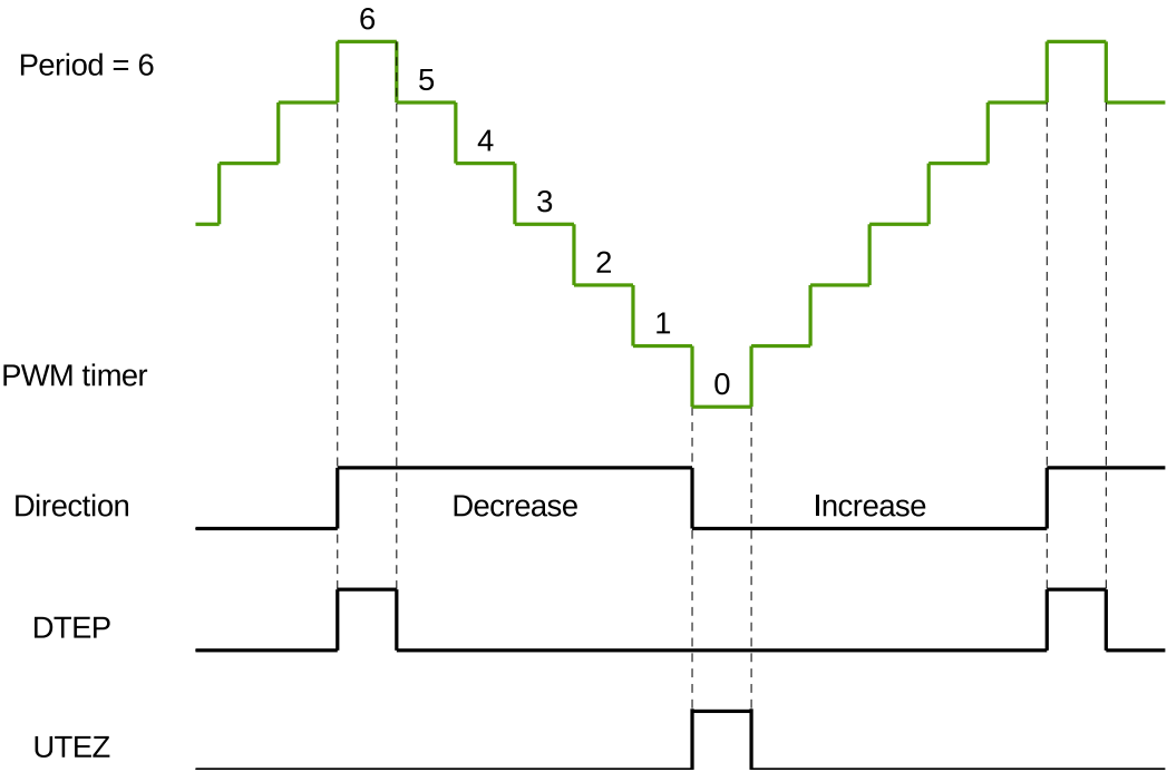
图 54.3-11. 递增递减模式中生成的 DTEP 和 UTEZ
