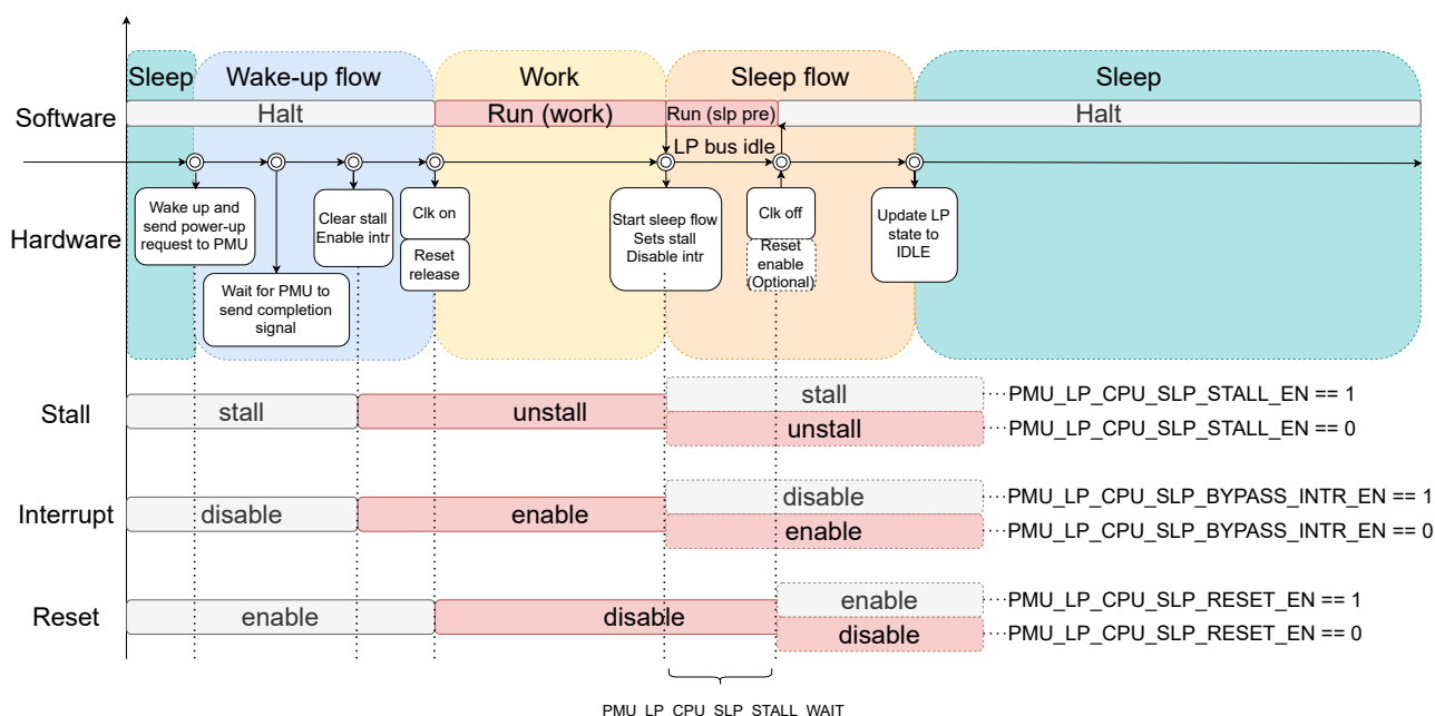
图 3.10-1. LP CPU 唤醒和睡眠流程
