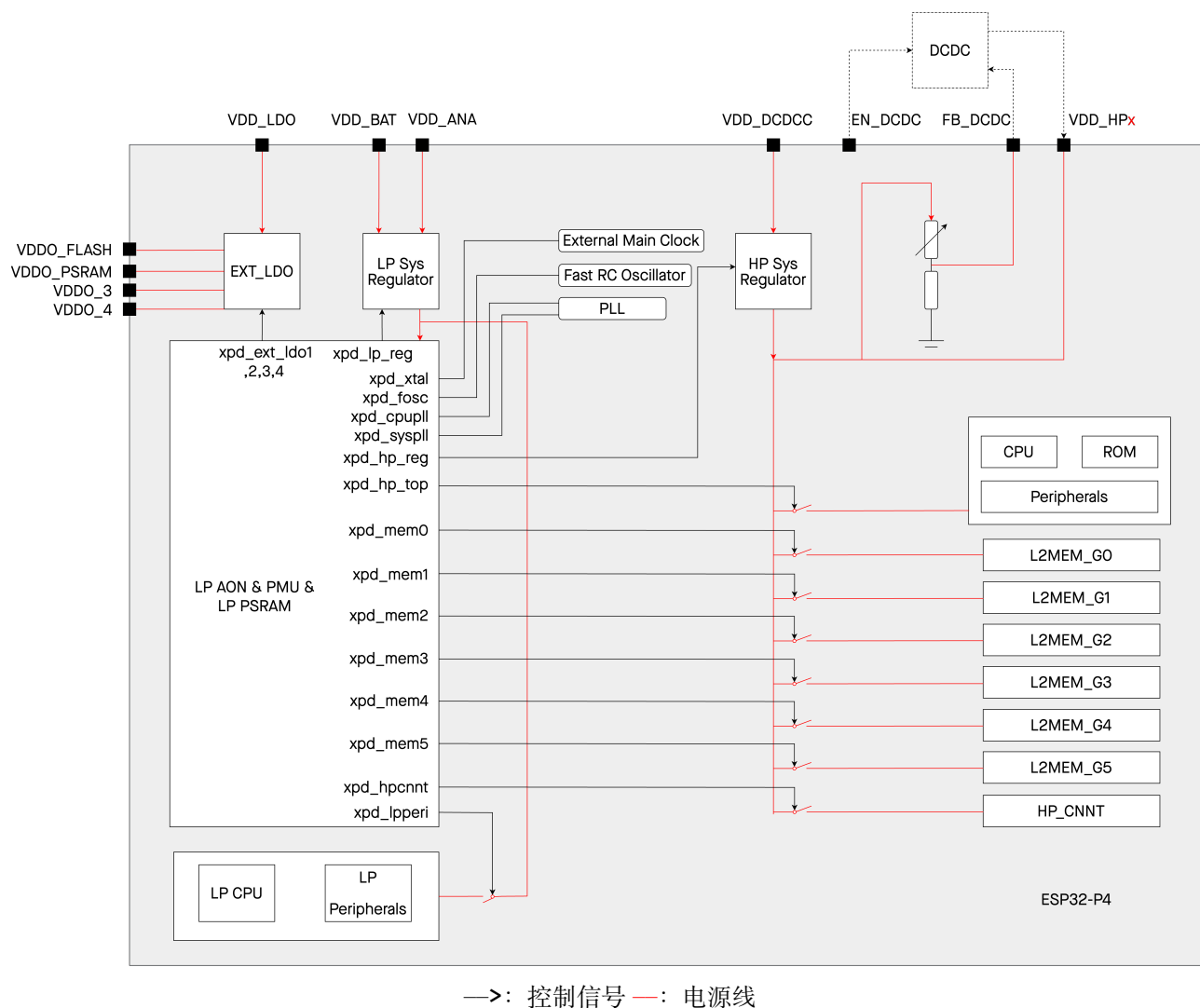
图 14.4-1. ESP32-P4 电源结构
