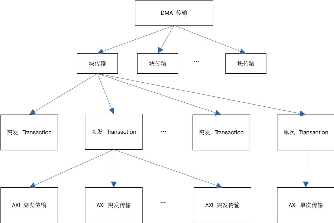
图 5.5-1. 外设的传输层次结构
