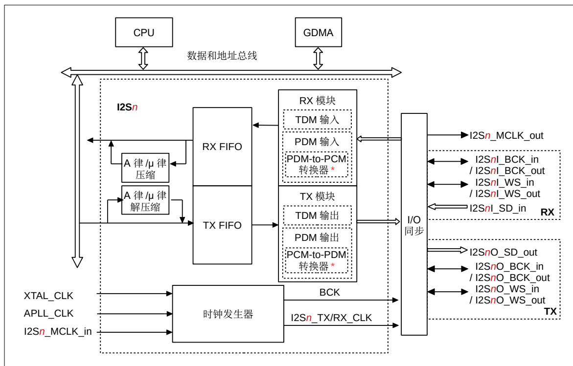
图 44.4-1. ESP32-P4 I2S 系统框图
