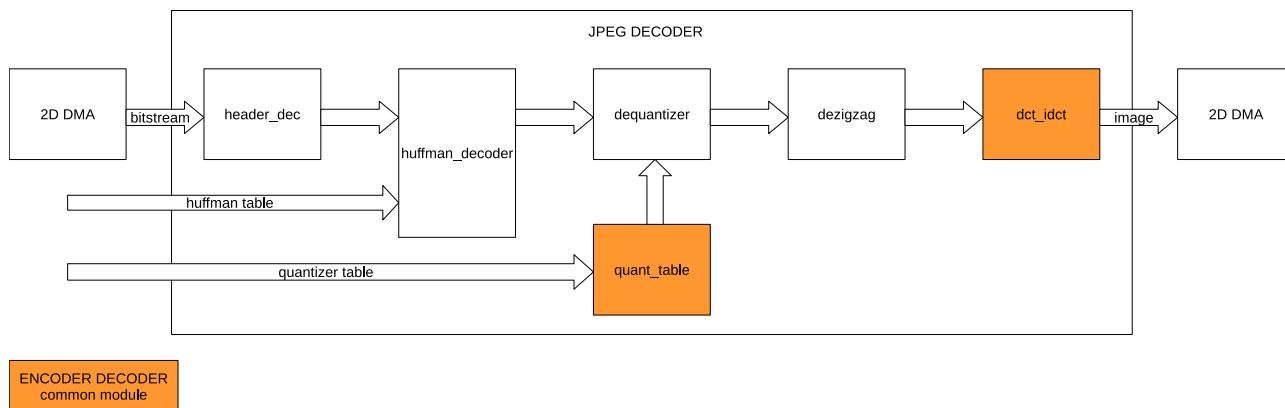
图 33.4-2. JPEG 解码器架构
