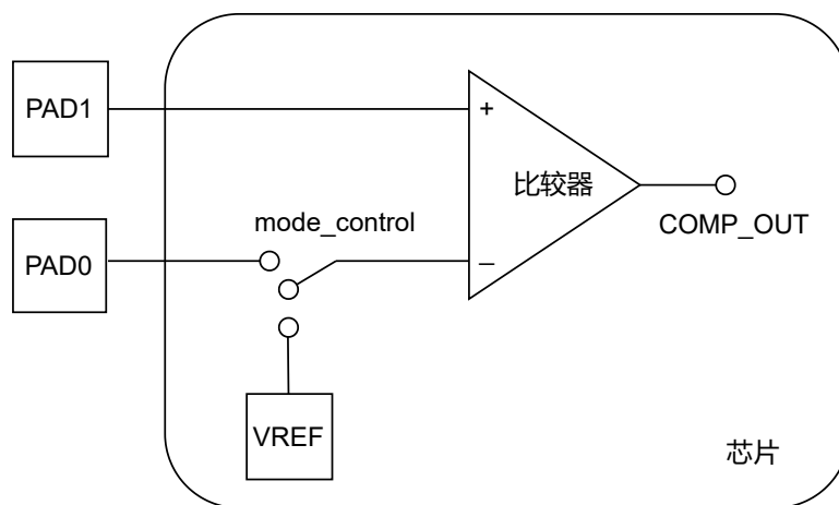
图 61.3-1. 模拟电压比较器系统框图
