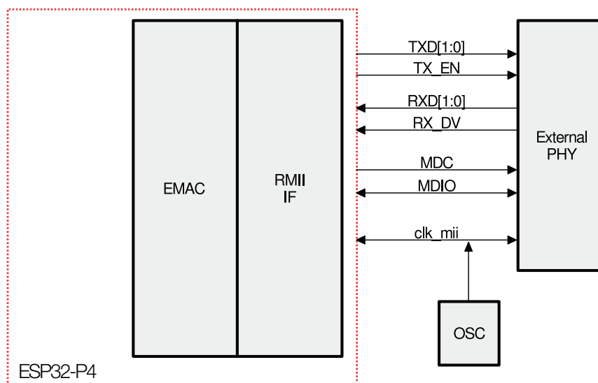
图 50.4-5. RMII 接口
