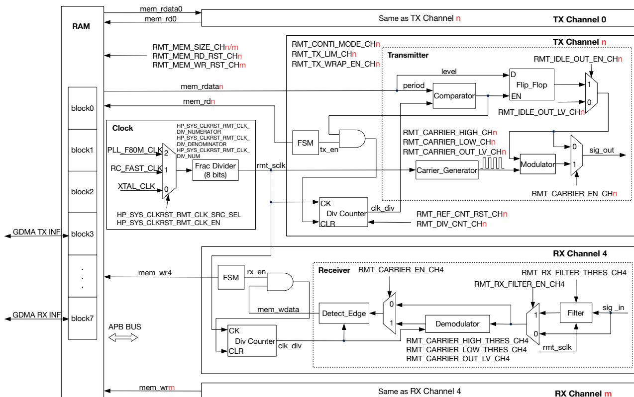
图 55.3-1. RMT 结构框图
