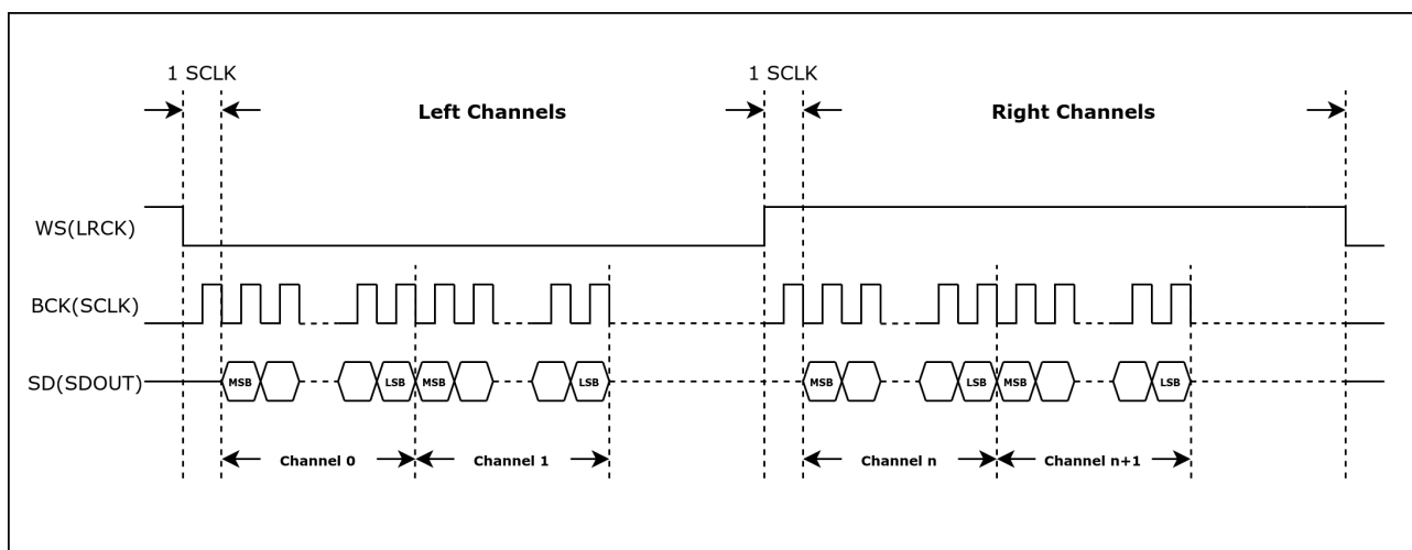
图 44.5-1. 时序图 – TDM Philips 标准
