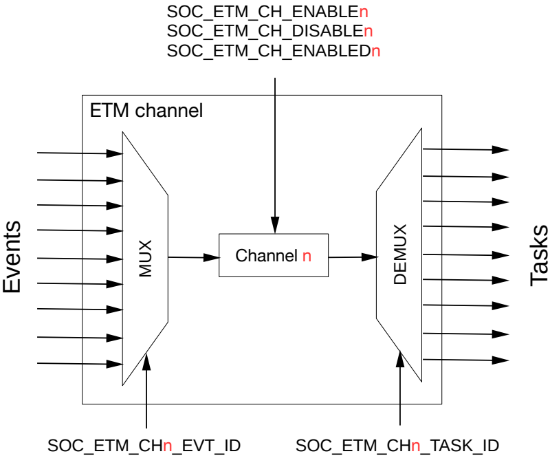
图 13.3-1. 事件任务矩阵通道n 架构
