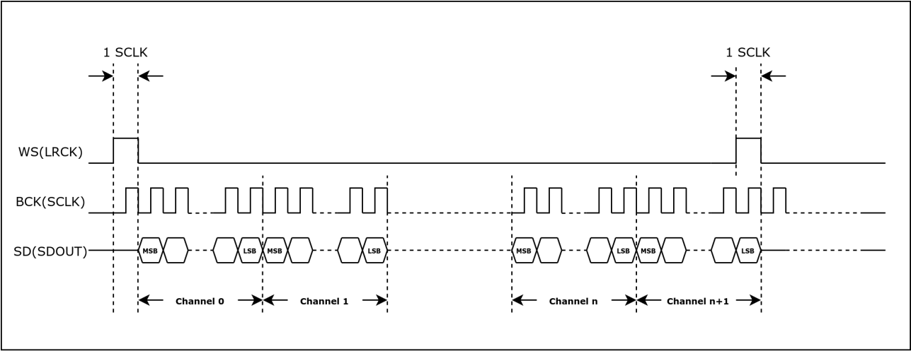
图 45.4-3. 时序图 – TDM PCM 标准
