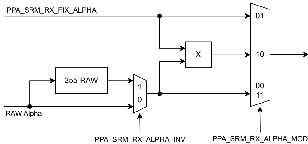
图 35.5-2. PPA SRM Alpha 配置逻辑
