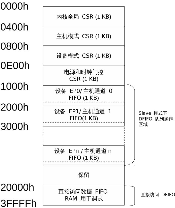
图 48.4-2. 内核地址映射
