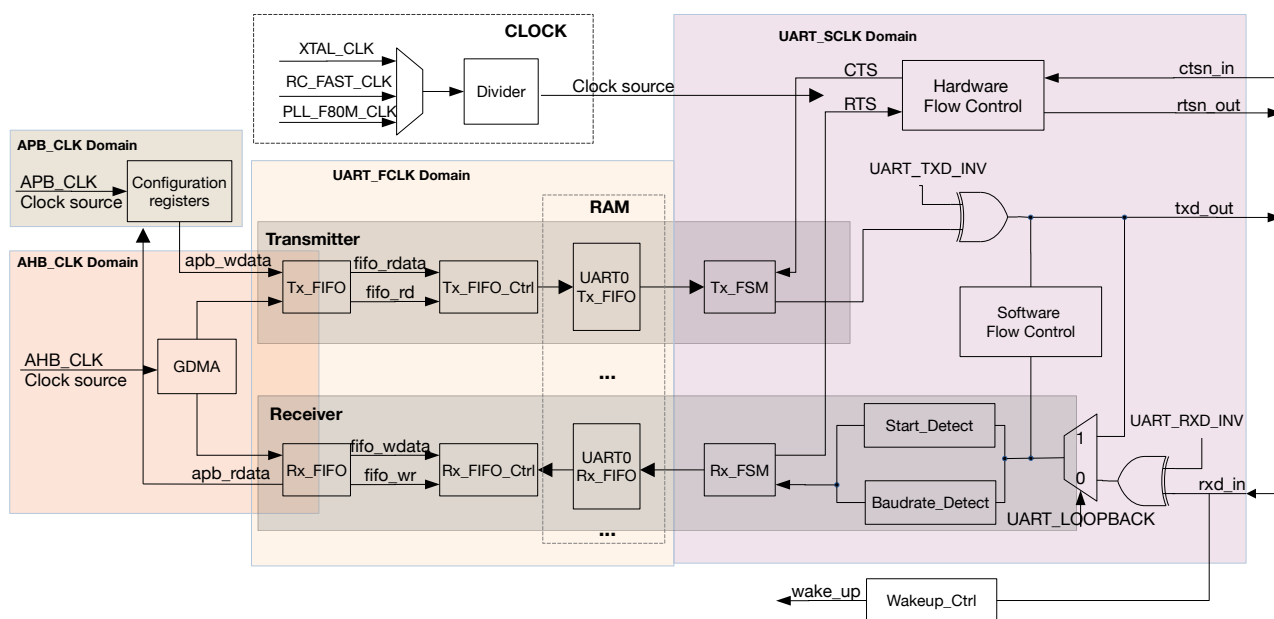
图 40.3-1. UART 基本架构图
