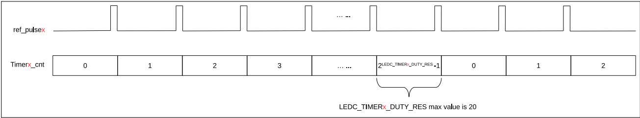
图 53.4-2. 计数器和 PWM 信号精度关系
