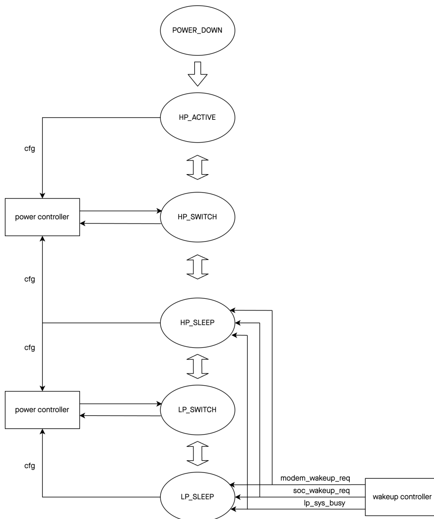
图 14.4-2. PMU 的主要工作流程
