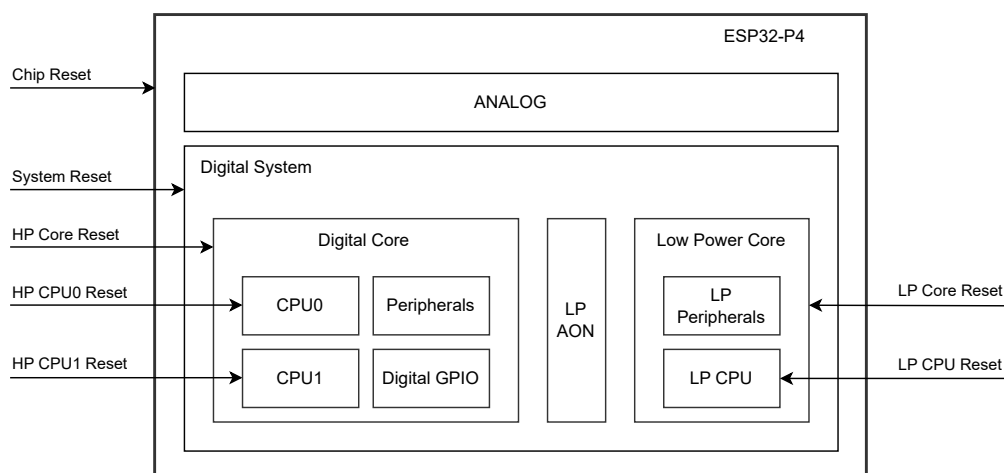
图 10.1-1. 四种复位等级
