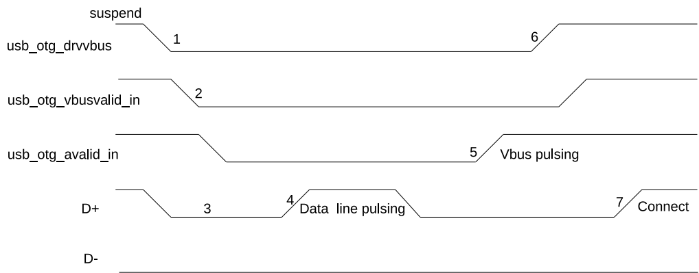
图 48.5-1. A 设备 SRP
