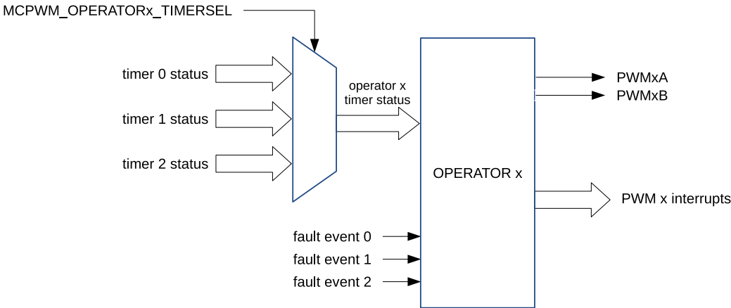
图 54.3-2. 操作器模块
