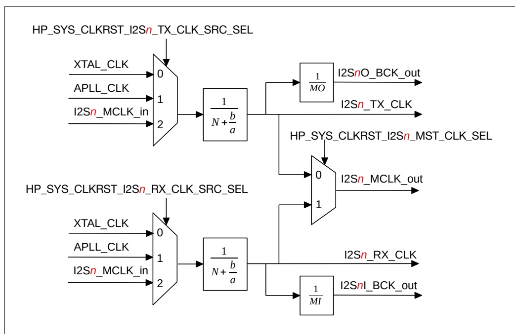
图 44.6-1. I2S n 时钟分频器
