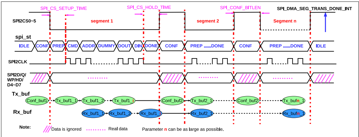
图 41.5-9. DAM 控制的分段配置传输
