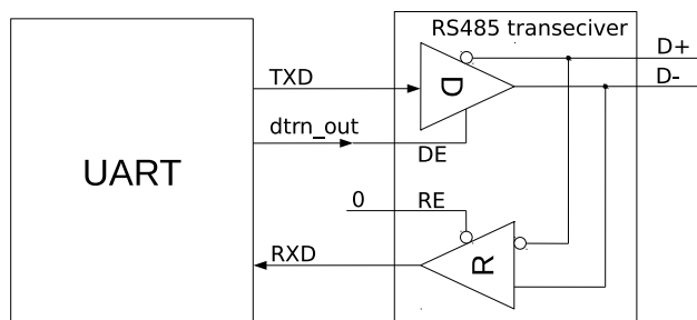
图 40.4-5. RS485 模式驱动控制结构图
