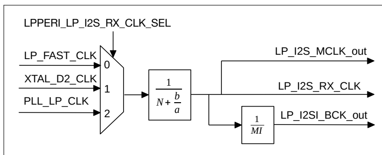
图 45.5-1. LP I2S 时钟分频器
