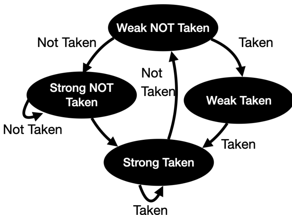
图 1.12-1. 2 位饱和计数器
