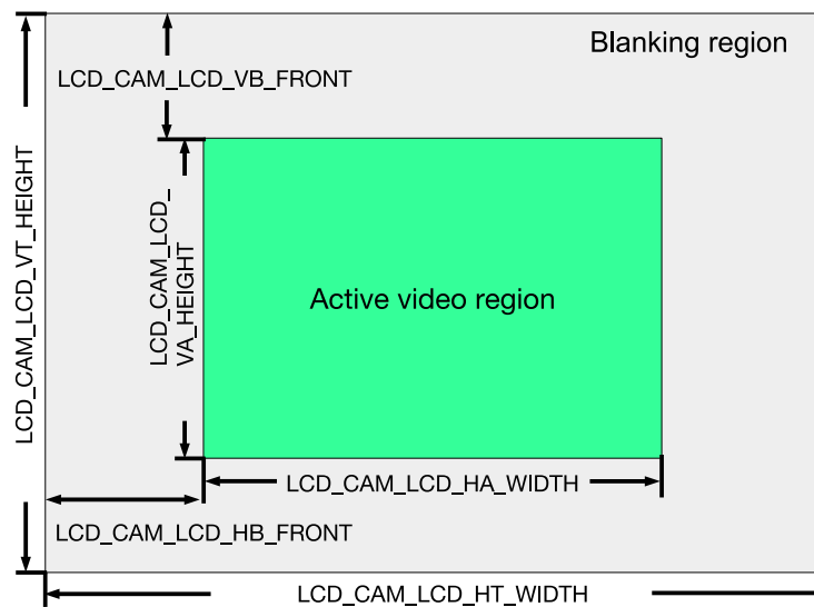
图 36.3-4. LCD 视频帧结构
