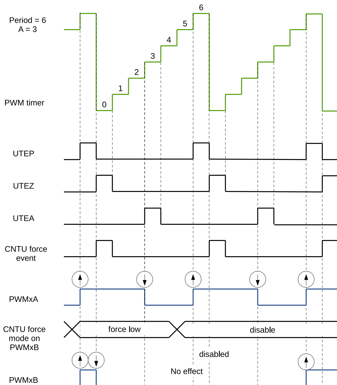
图 54.3-20. CNTU 在 PWMxB 输出上软件强制事件示例
