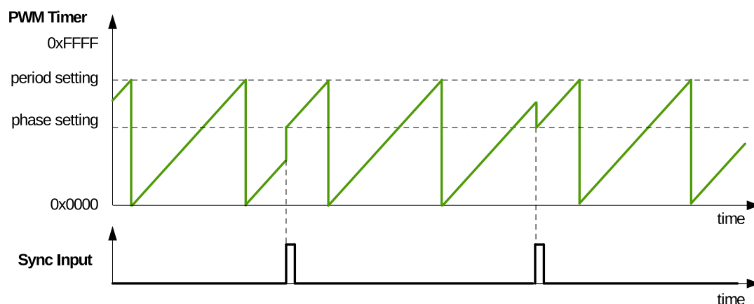
图 54.3-5. 递增计数模式波形
