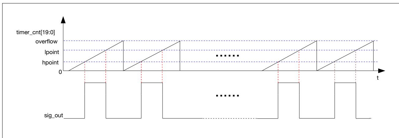
图 53.4-3. LED PWM 输出信号图
