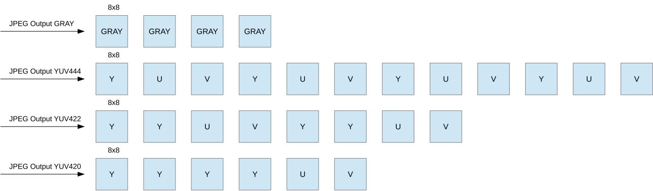
图 6.4-4. JPEG 解码输出数据宏块排布
