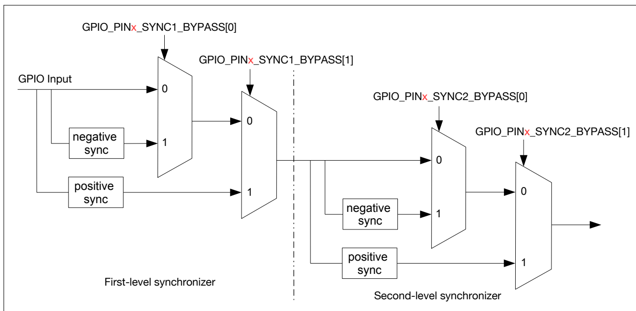
图 9.4-1. GPIO 输入经 HP IO MUX 运行时钟上升沿或下降沿同步
