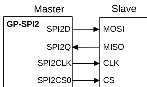
图 41.5-6. GP-SPI2 主机使用全双工与 SPI 从机通信
