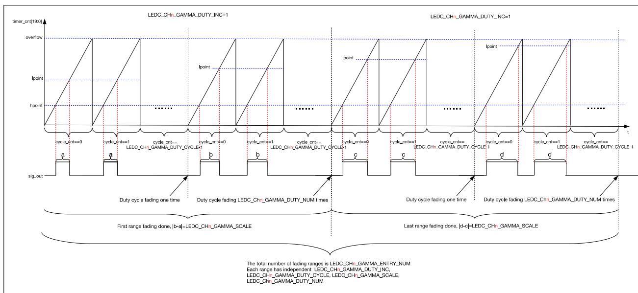
图 53.4-5. 输出信号占空比伽马曲线渐变图
