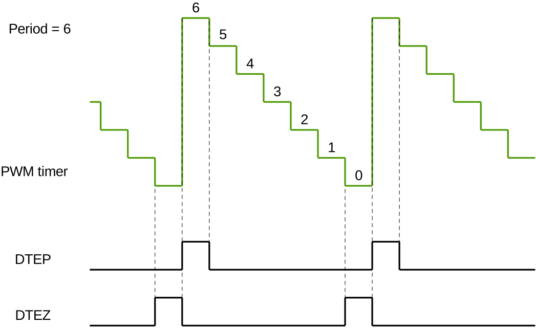
图 54.3-10. 递减模式中生成的 DTEP 和 DTEZ
