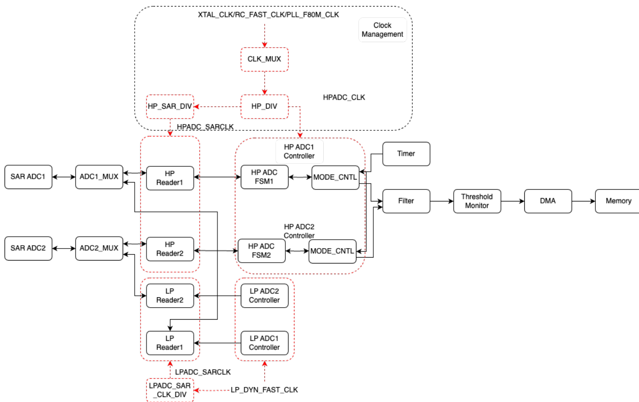
图 60.4-1. SAR ADC 结构图
