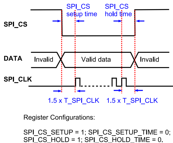
图 41.6-2. GP-SPI 访问 Flash 时推荐的 CS 时序配置
