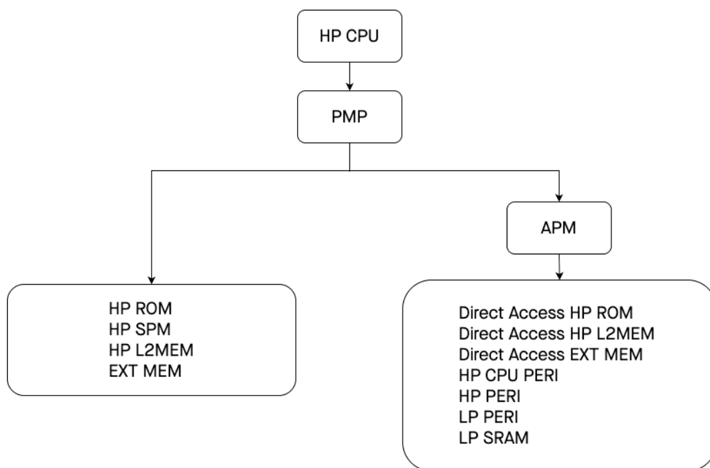
图 19.1-1. PMP 和 APM 的管控关系
