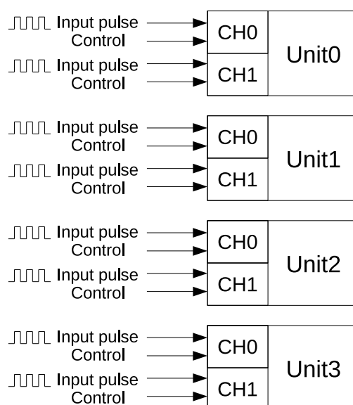
图 46.1-1. PCNT 框图
