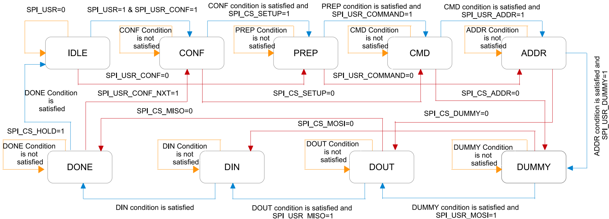
图 41.5-5. GP-SPI 主机状态机
