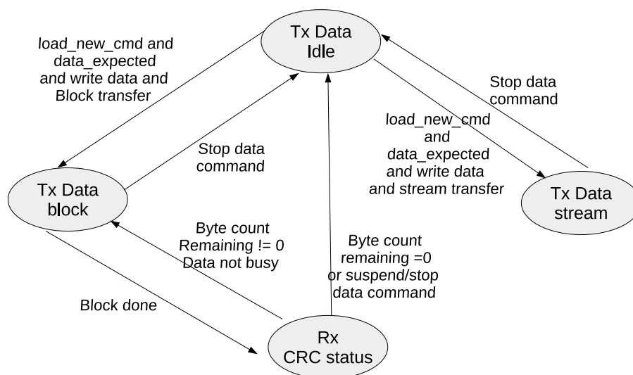
图 52.4-3. 数据发送状态机
