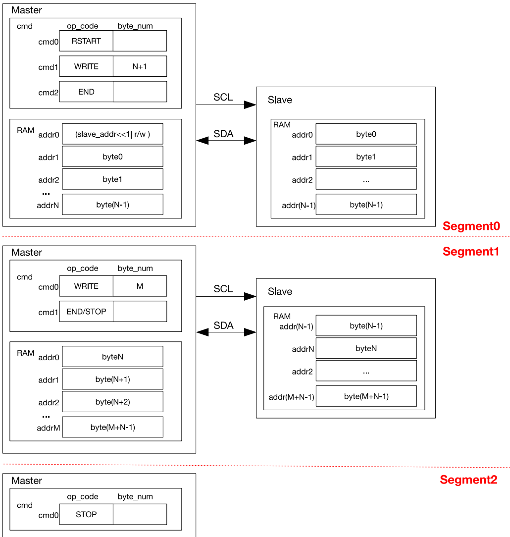
图 42.6-4. I2C 主机分段写 7 位寻址的从机
