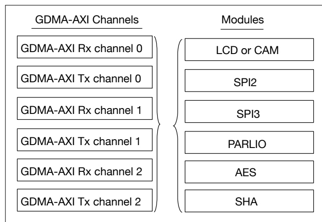
图 4.1-2. 共用 GDMA-AXI 通道的模块
