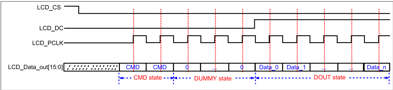
图 36.3-6. LCD 时序 (I8080/MOTO6800 格式)
