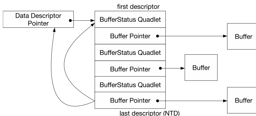
图 48.4-6. Scatter/Gather DMA 链表结构
