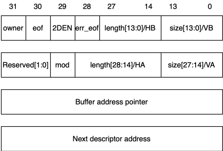
图 37.5-3. H264_DMA 链表描述符
