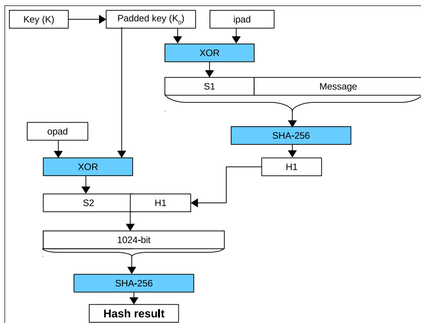
图 26.3-2. HMAC 结构示意图
