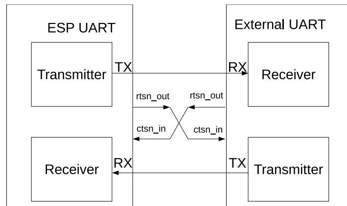
图 40.4-9. 硬件流控信号连接图
