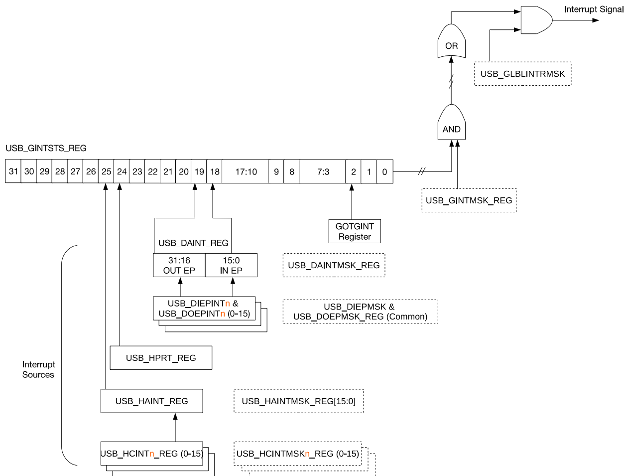
图 47.4-5. OTG_HS 中断层次结构图
