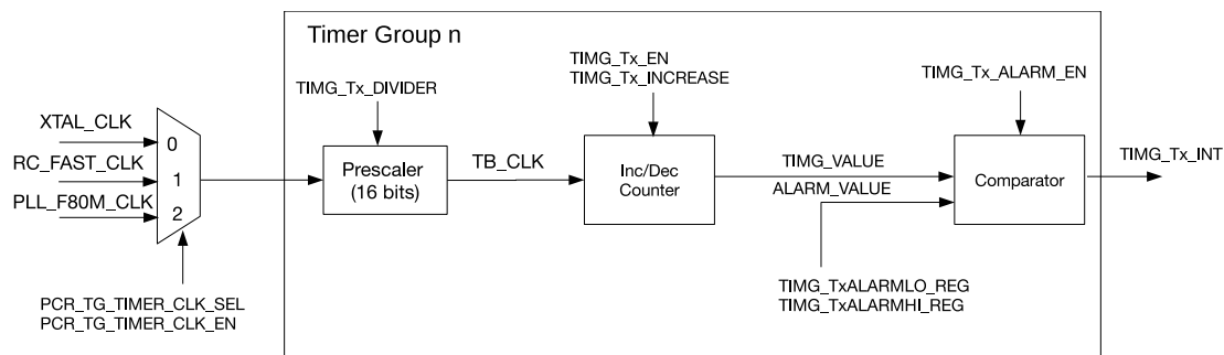
图 16.3-1. 定时器组架构
