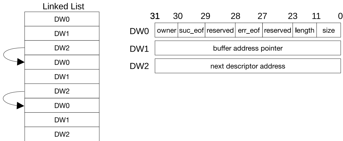
图 4.4-1. 链表结构图
