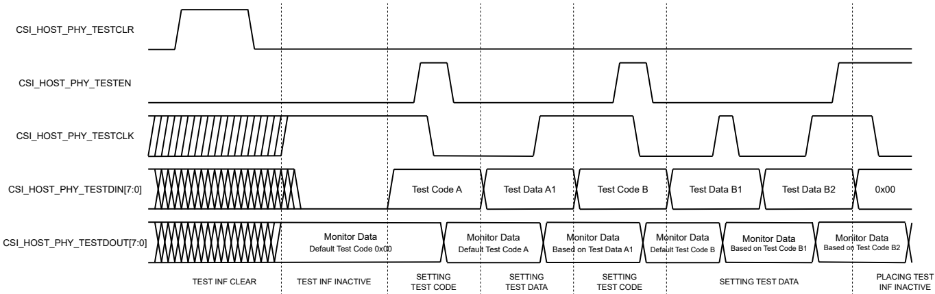
图 38.5-5. 控制接口时序图
