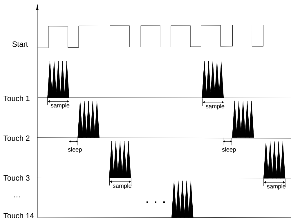
图 58.4-3. 扫描模式时序图
