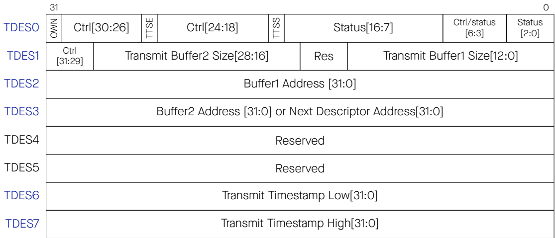
图 50.4-1. 发送描述符
