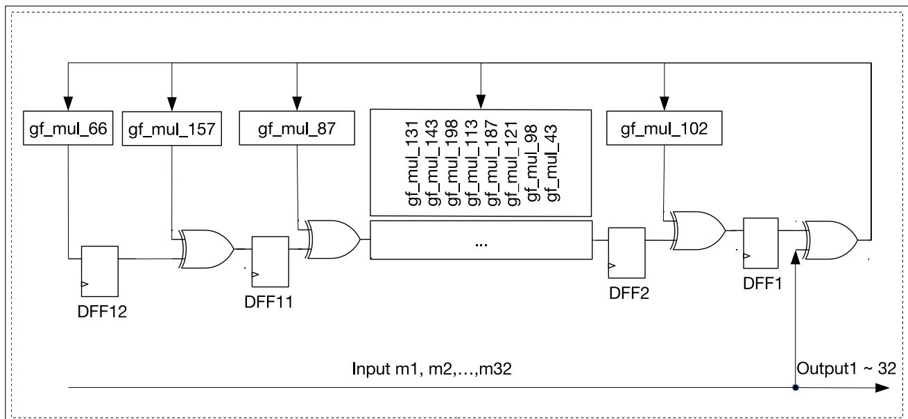
图 8.3-2. 移位寄存器电路图 (前 32 字节)
