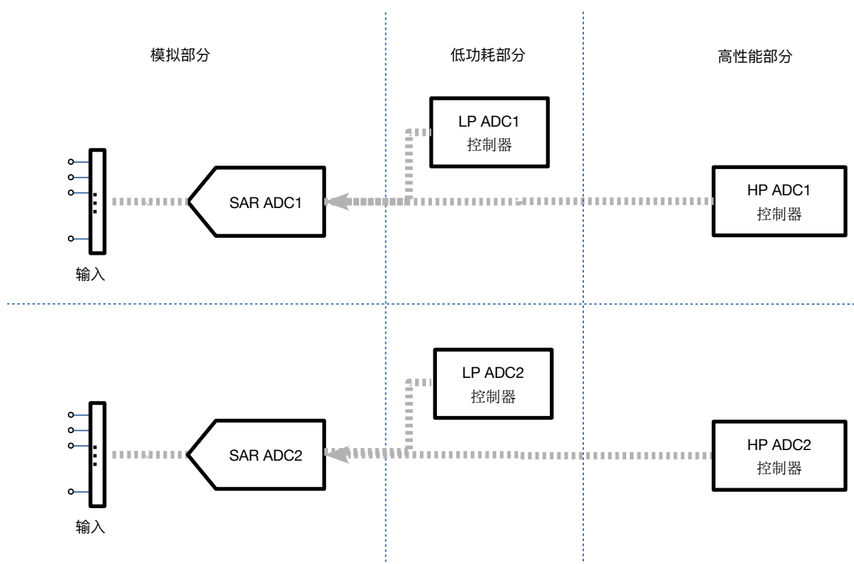
图 60.1-1. SAR ADC 结构概图
