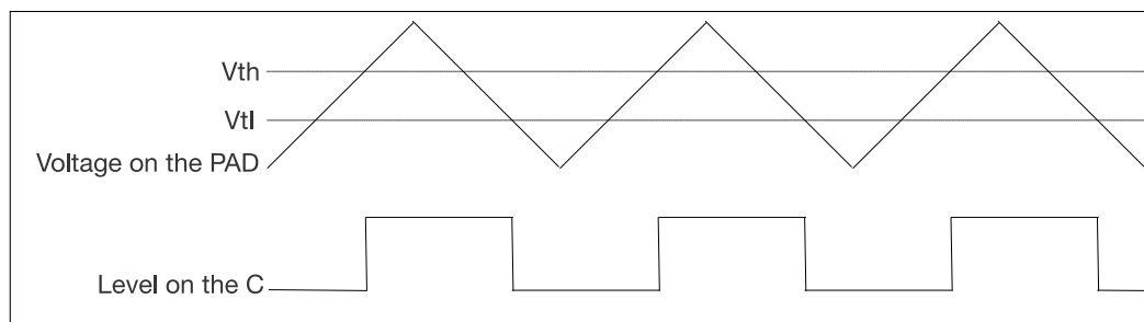
图 9.10-2. 使能迟滞功能时 PAD 上的电平翻转示例
