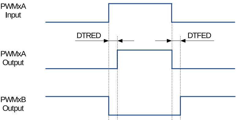
图 54.3-22. 高电平有效互补 (AHC) 死区波形
