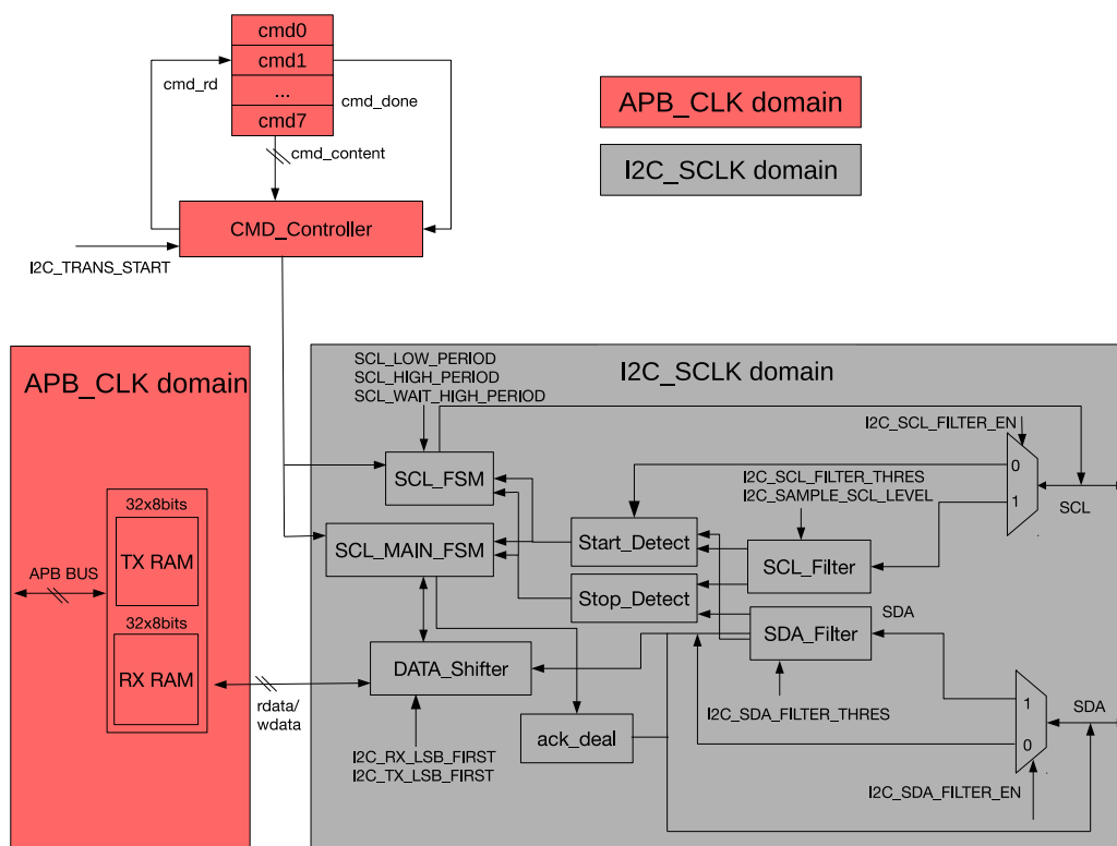
图 42.3-1. I2C 主机基本架构
