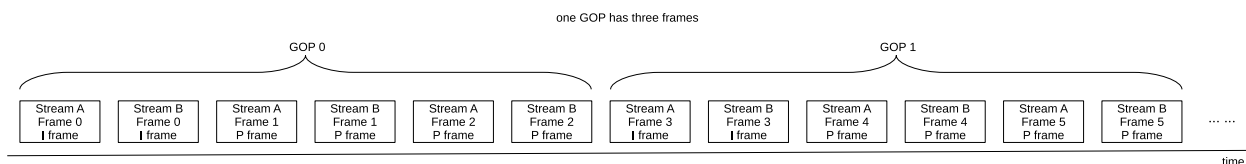
图 377-2. 双流模式下图像编码的顺序
