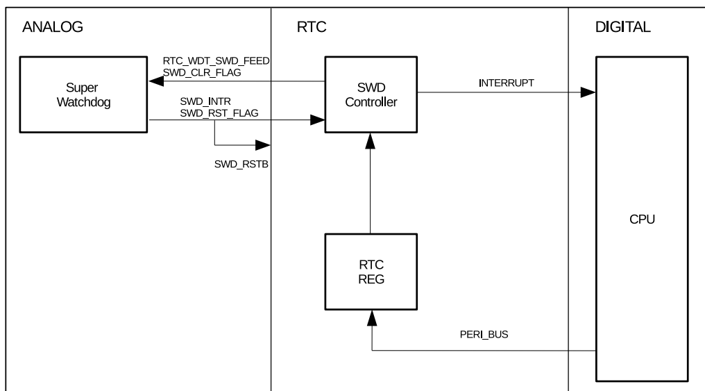
图 17.3-1. SWD 控制器结构
