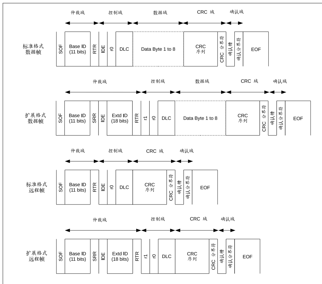
图 51.2-1. 数据帧和远程帧中的位域
