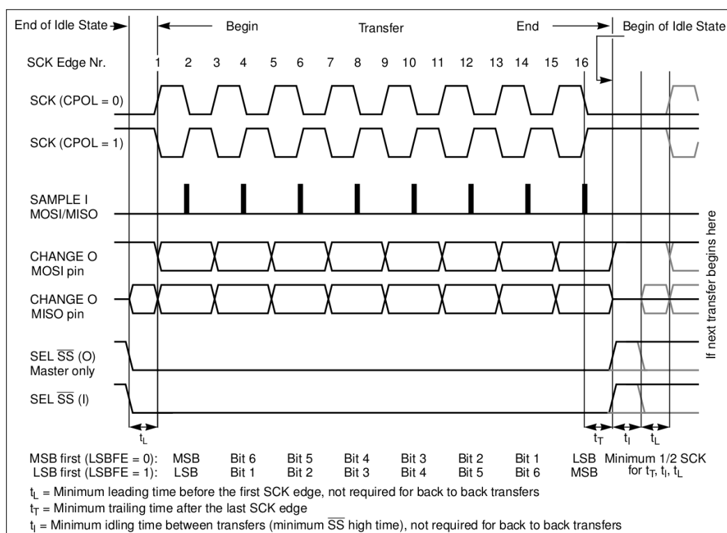
图 41.7-2. SPI 时钟模式 1 和时钟模式 3
