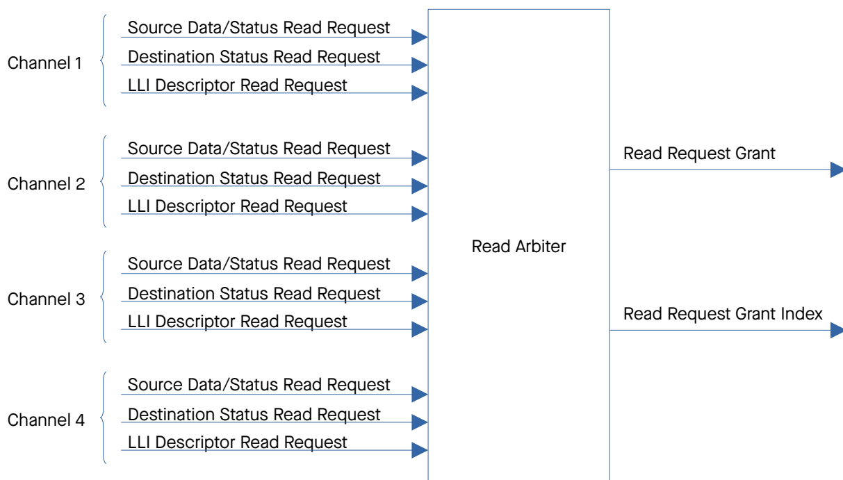
图 5.5-3. VDMA 读仲裁器
