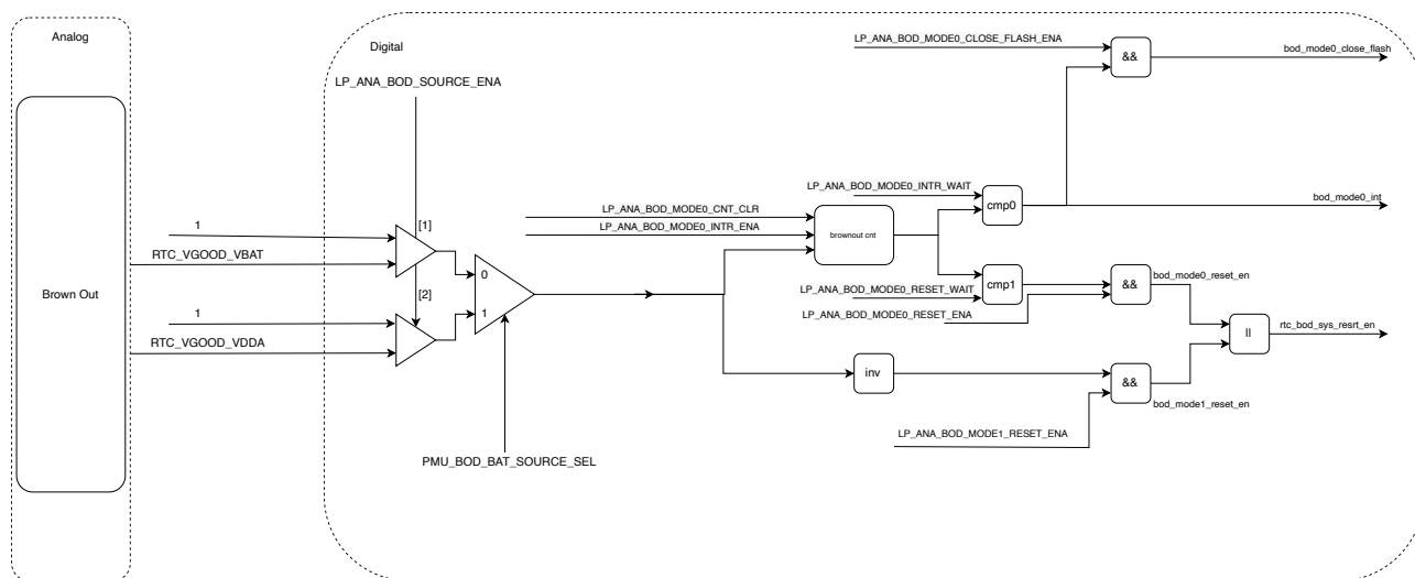
图 23.3-1. 欠压检测模块结构图
