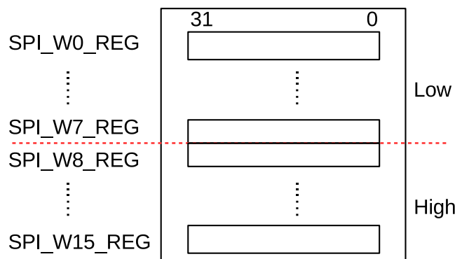
图 41.5-1. CPU 控制的传输中使用的数据 Buffer
