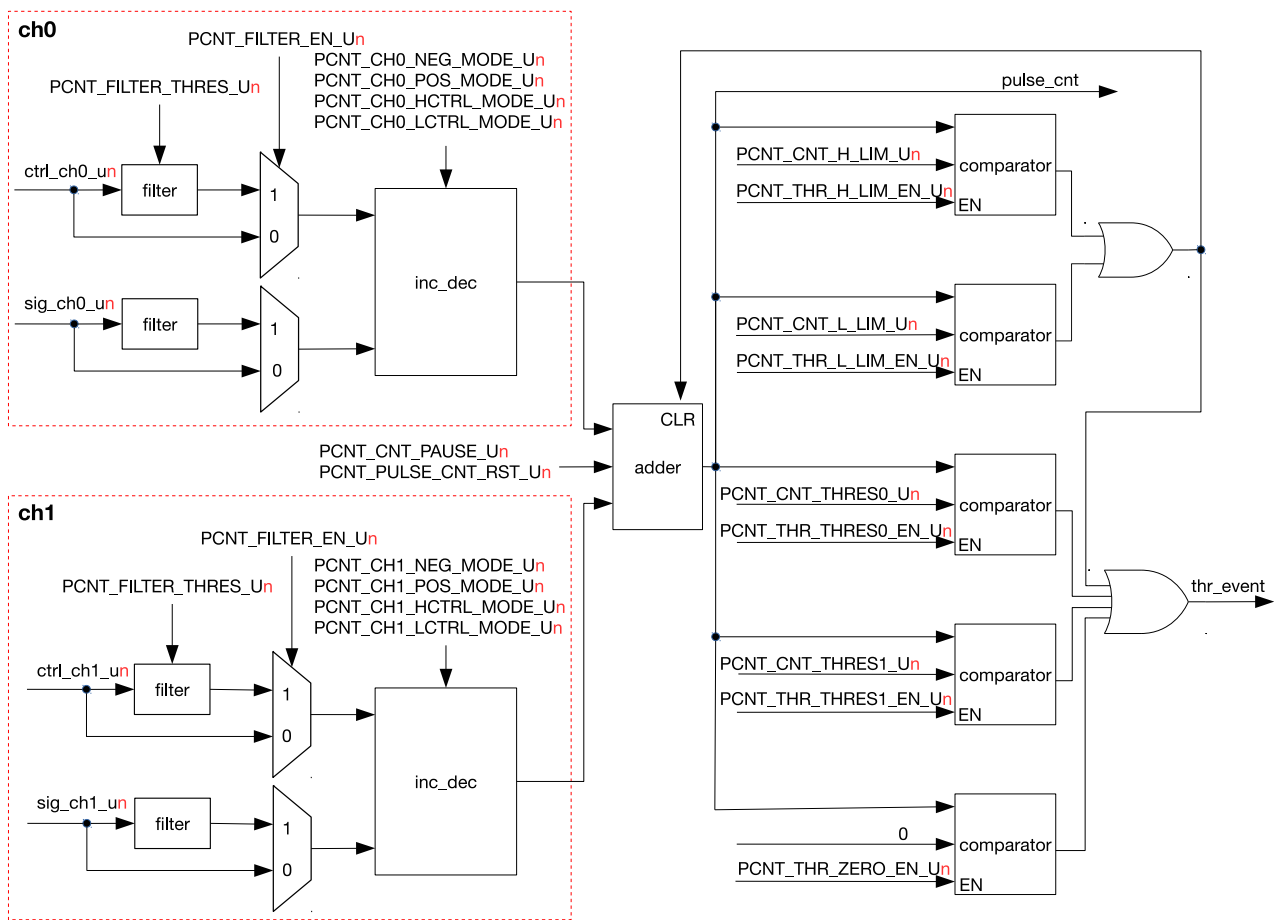
图 46.3-1. PCNT 单元基本架构图
