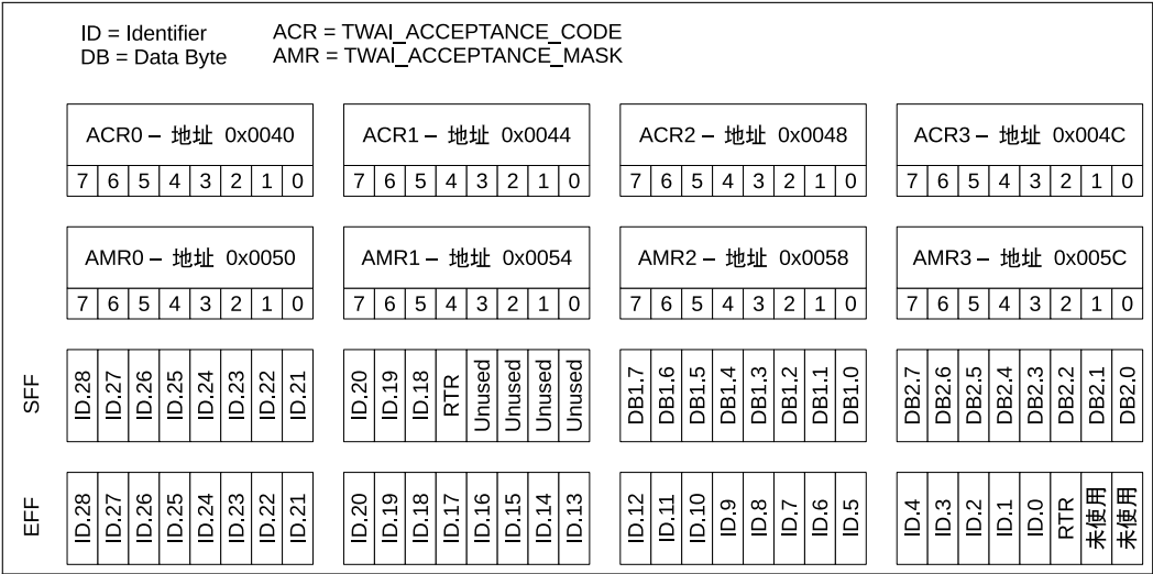
图 51.4-2. 单过滤模式
