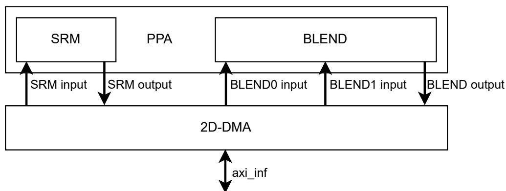
图 35.1-1. PPA 2D-DMA 连接关系
