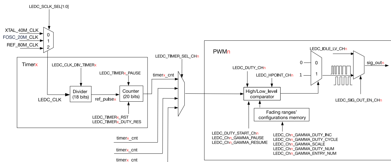
图 53.3-2. 定时器和 PWM 生成器功能框图
