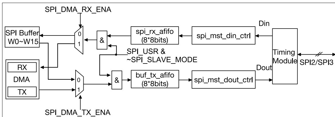
图 41.5-3. GP-SPI 用作主机时的数据流控制
