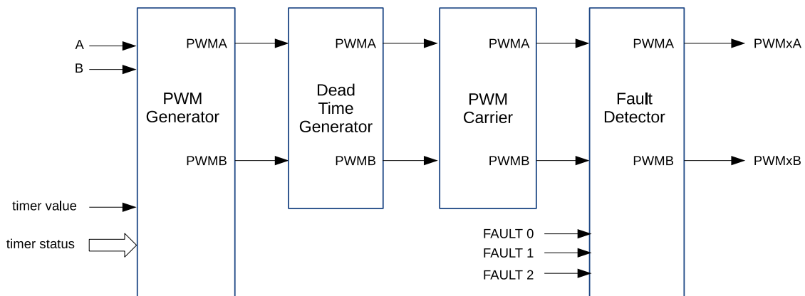
图 54.3-12. PWM 操作器的子模块
