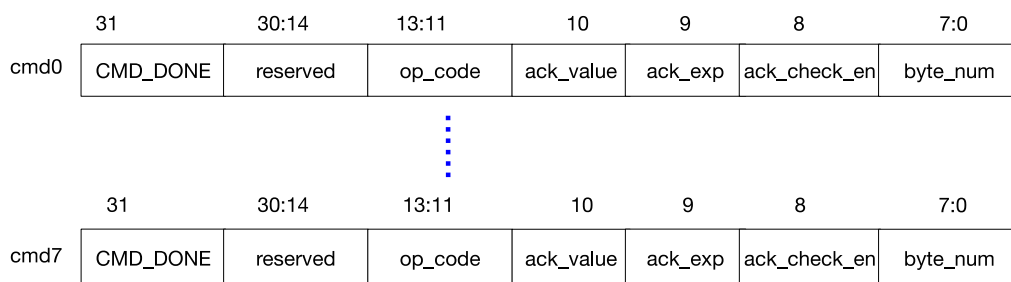
图 42.4-2. I2C 命令寄存器结构
