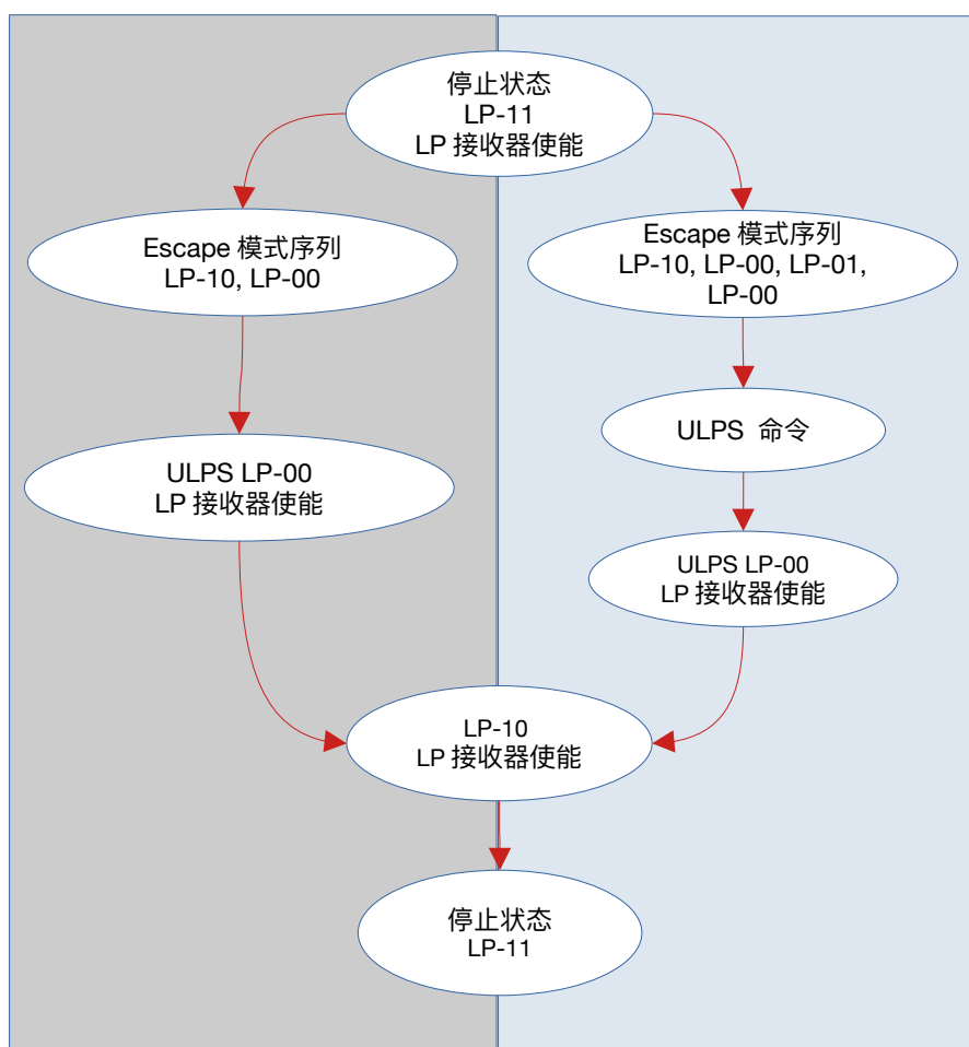
图 38.5-4. 时钟和数据通道 ULPS 序列
