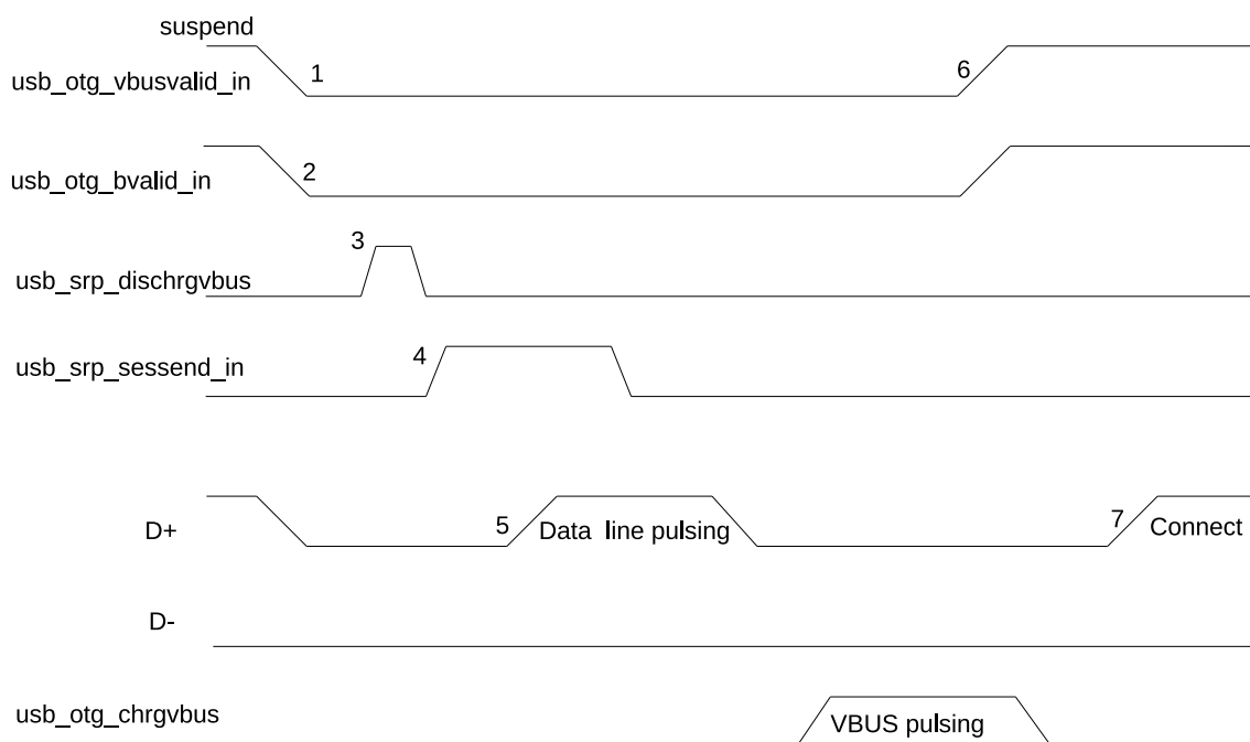
图 48.5-2. B 设备 SRP
