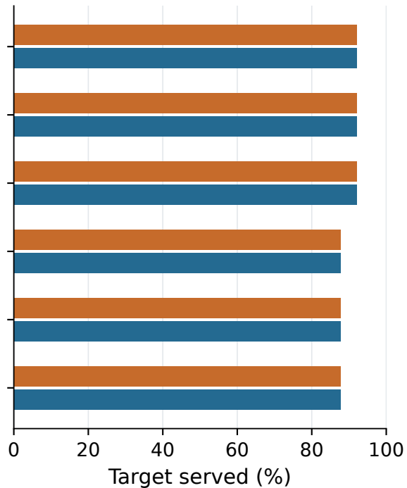
(b) 2040
