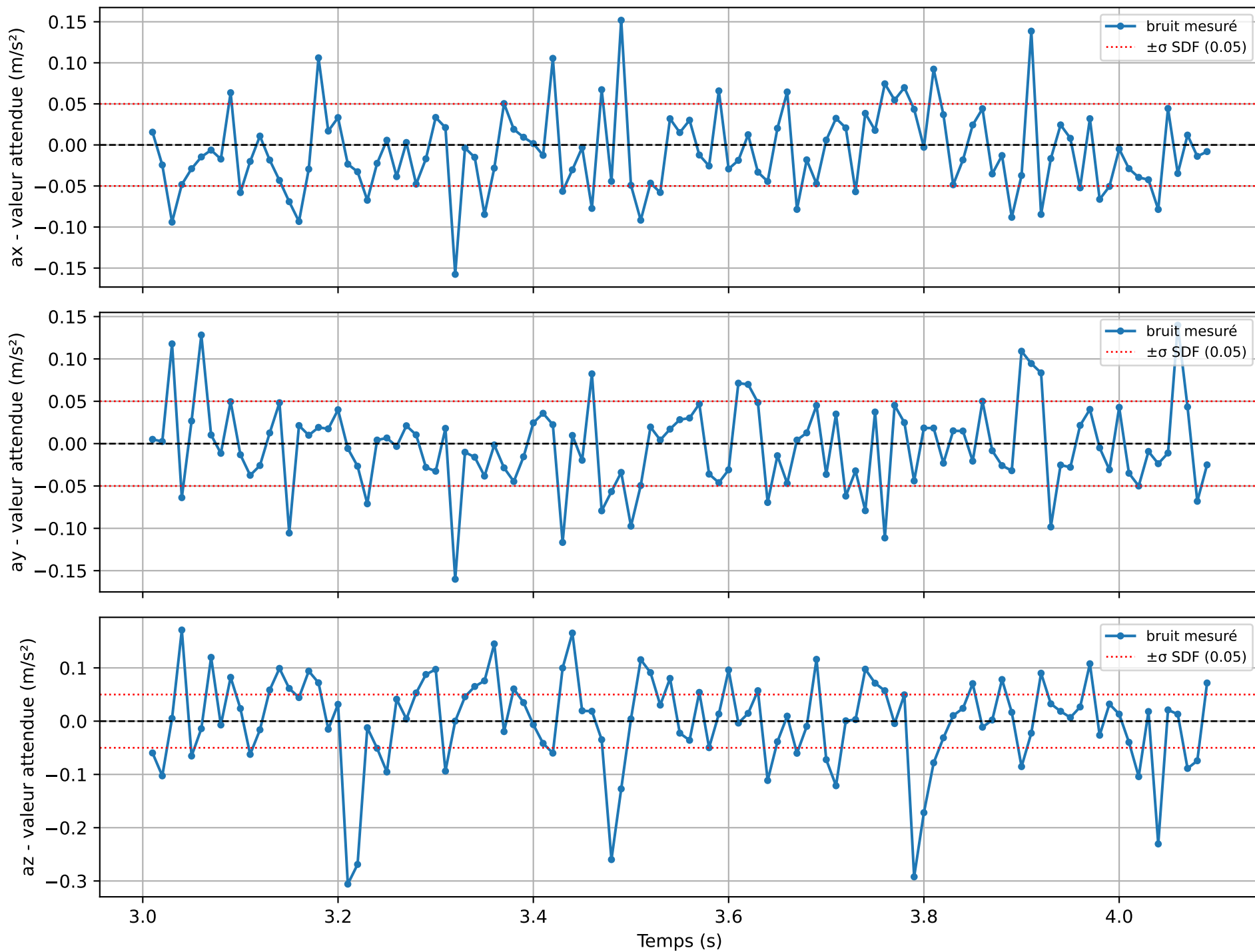
Bruit IMU isolé (mesure - valeur physique attendue) — fenêtre 3-4.1s
