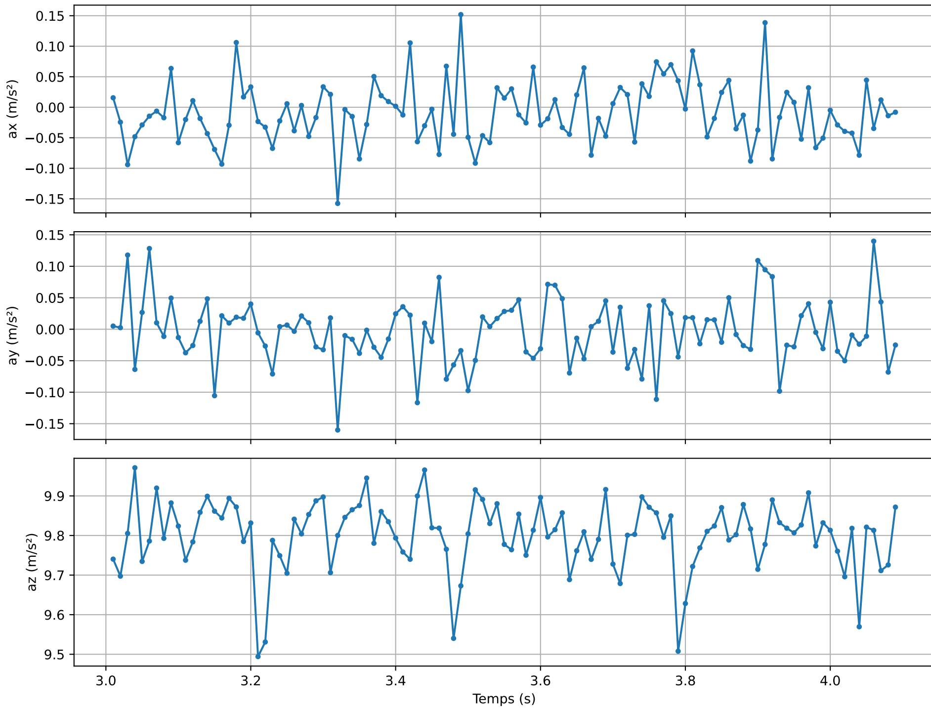
IMU brut (non integre) - fenetre 3-4.1s
