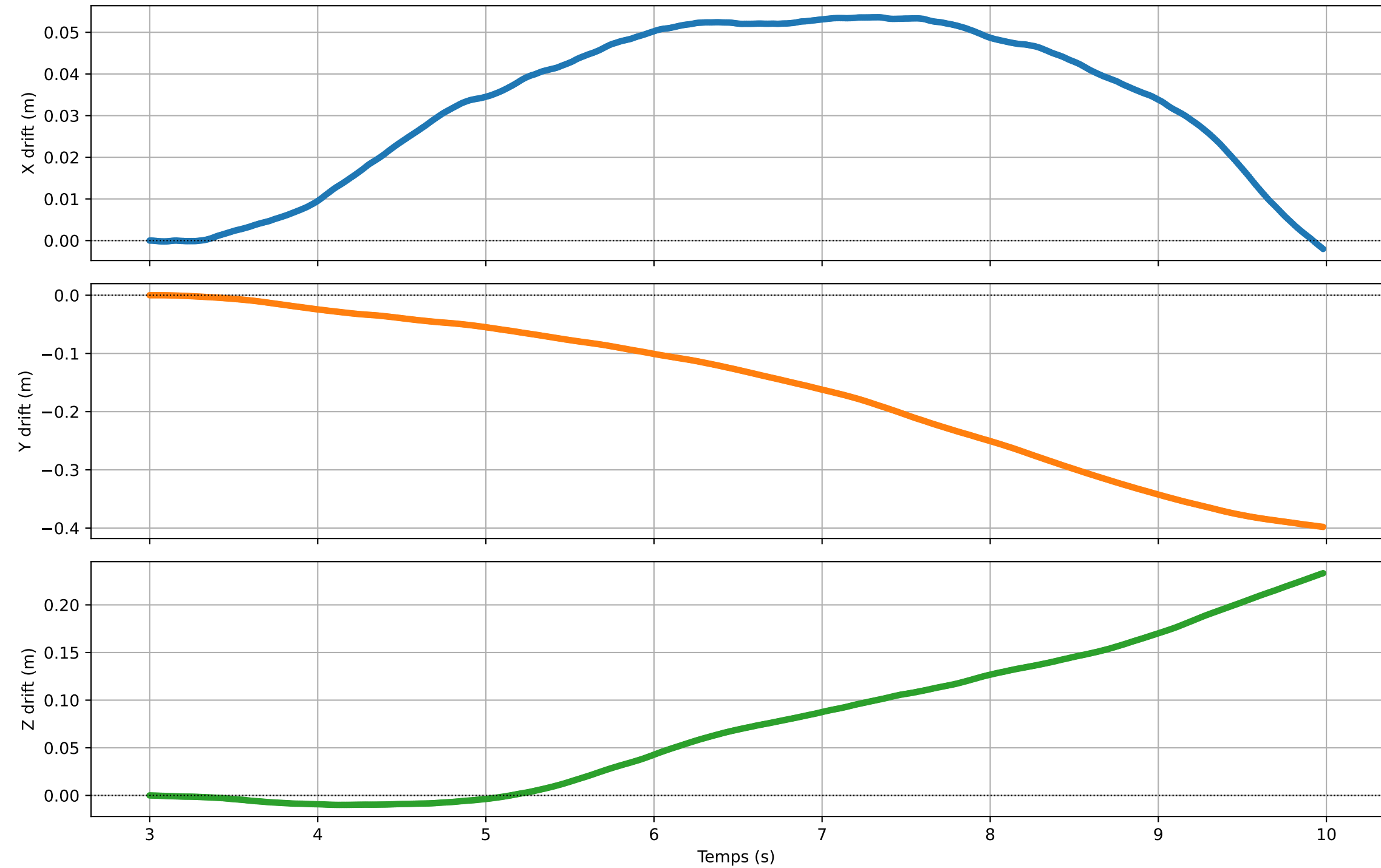
Dérive IMU pure (offset retiré) — rotation
