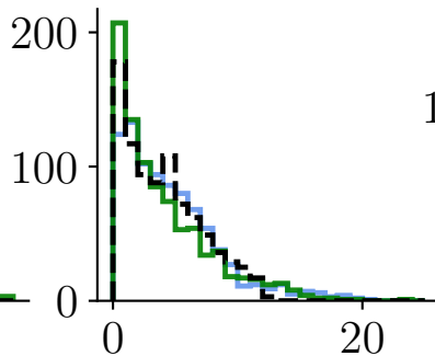
UGT2B11
