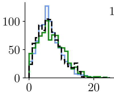
CPB1
