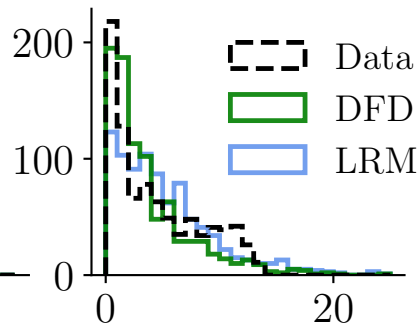
CLEC3A
