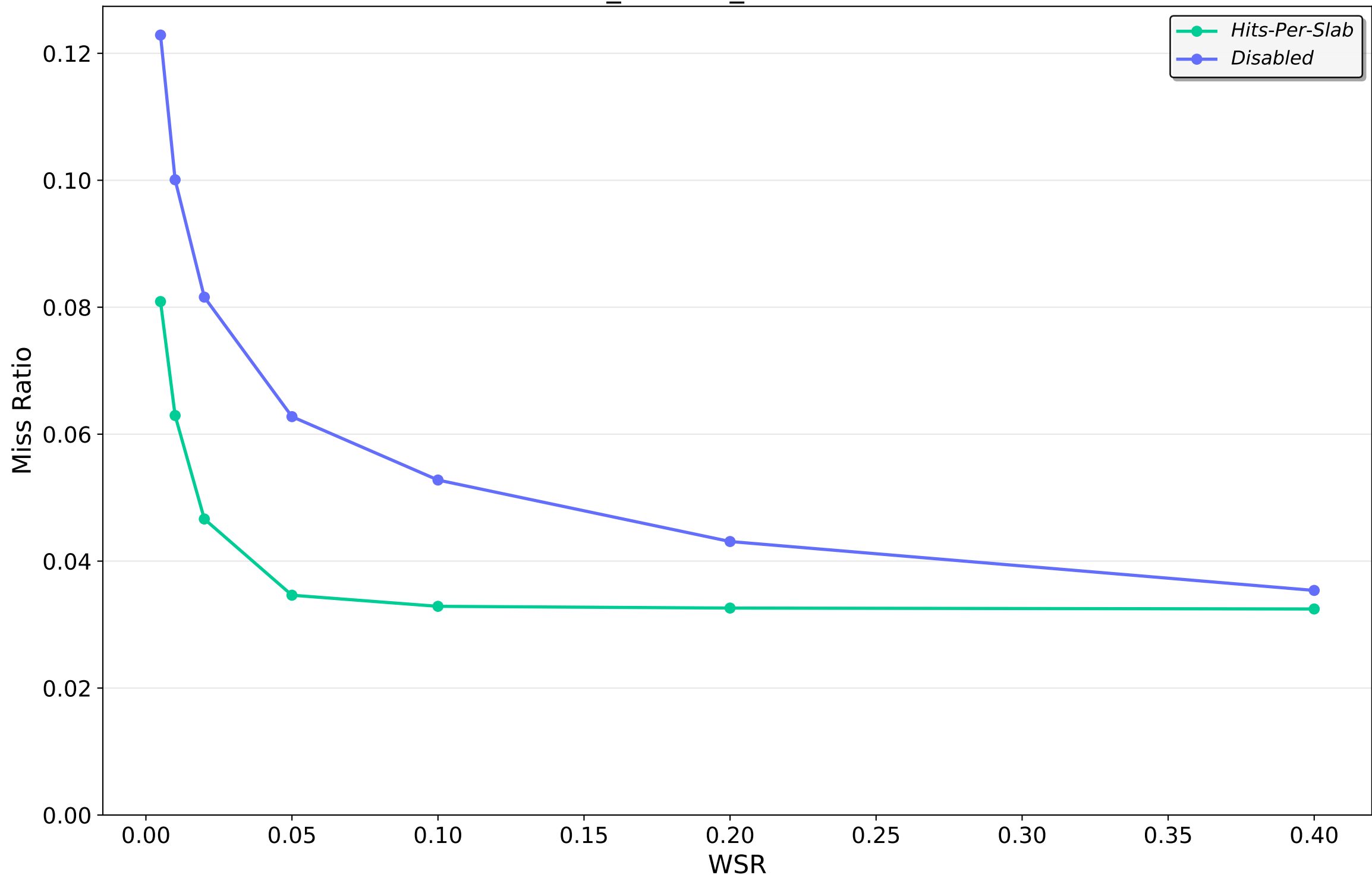
meta_202210_kv — TINYLFU
