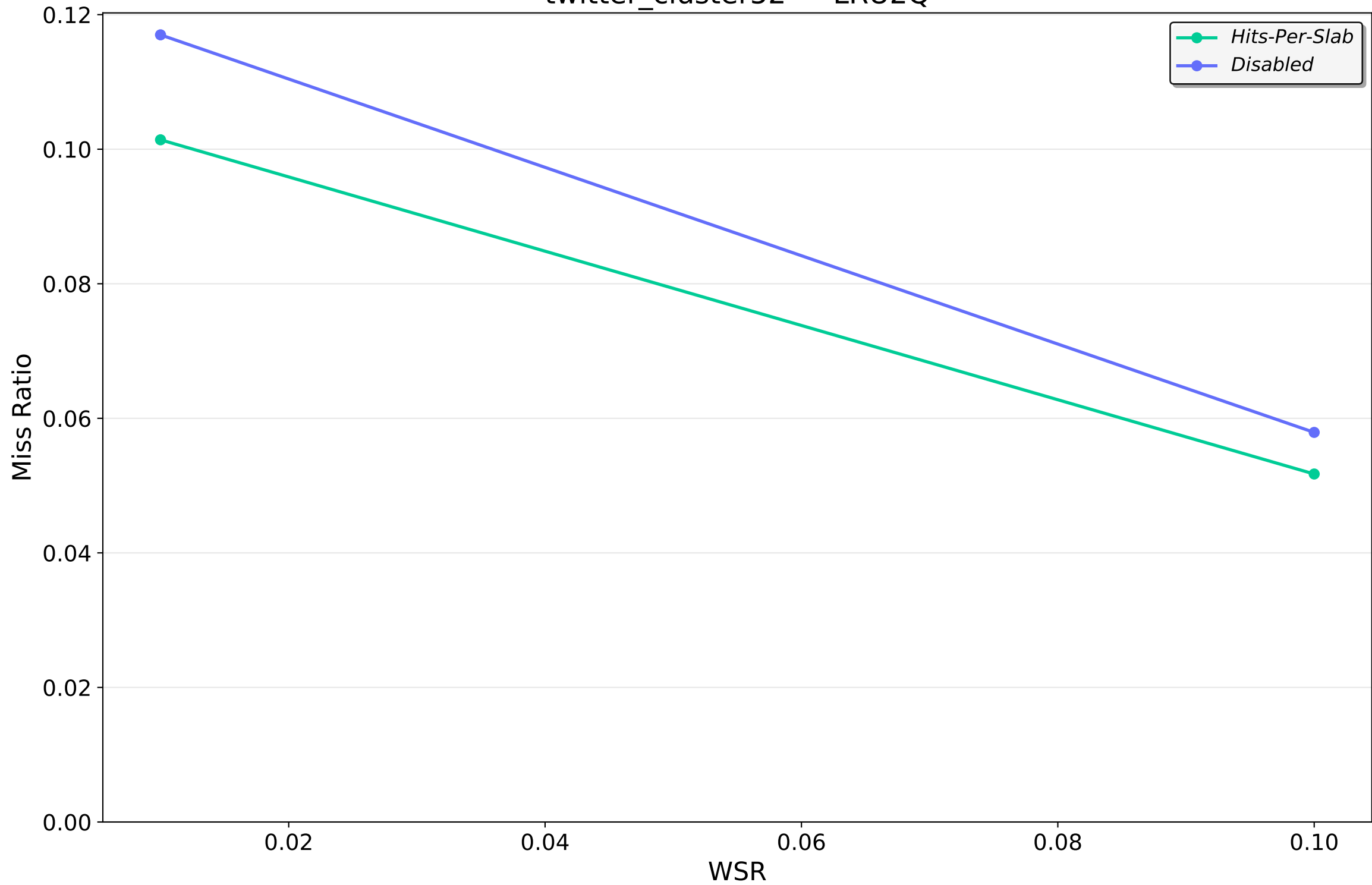
twitter_cluster52 — LRU2Q
