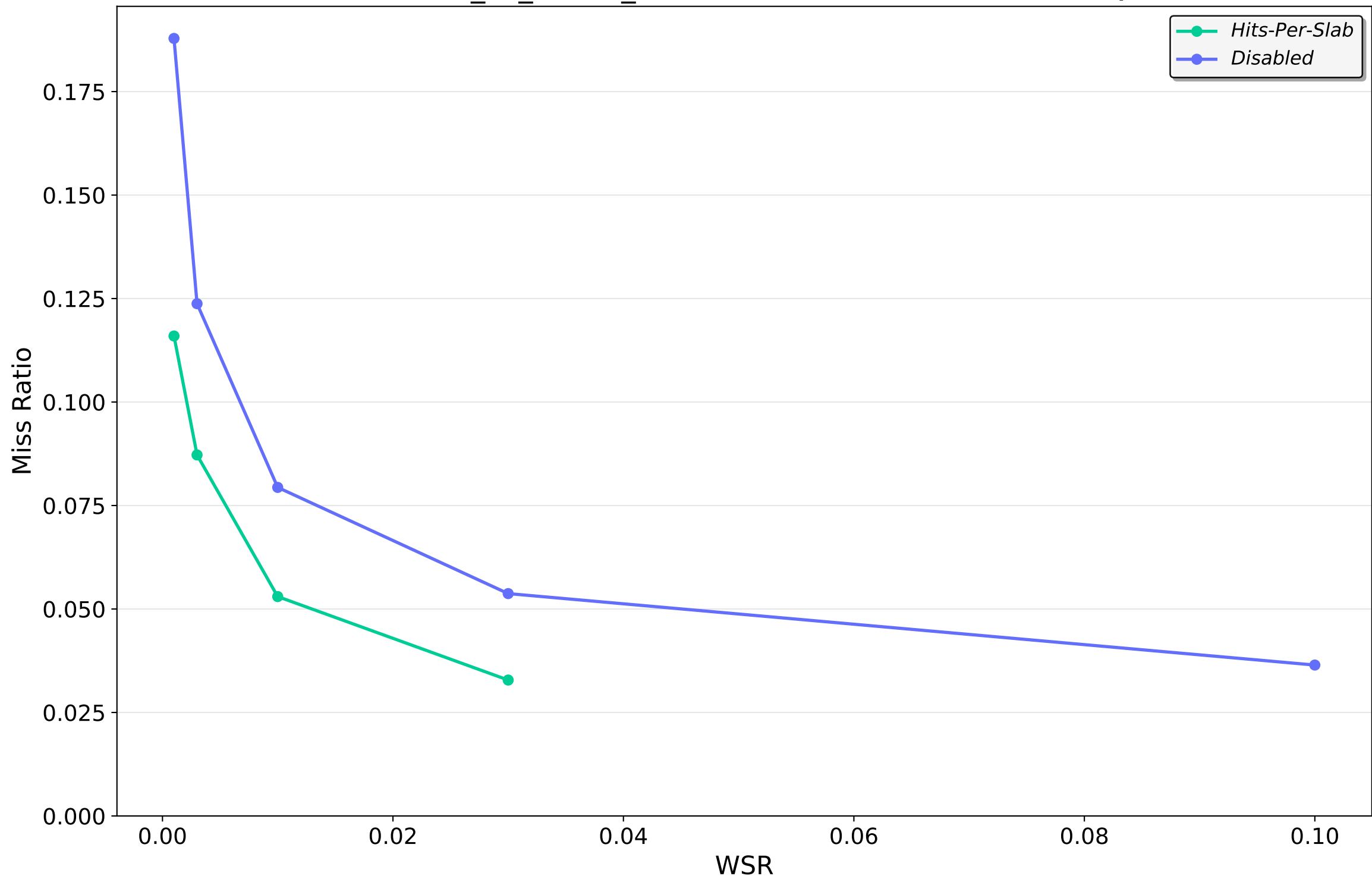
202312_kv_traces_all.csv.oracleGeneral.zst — LRU2Q
