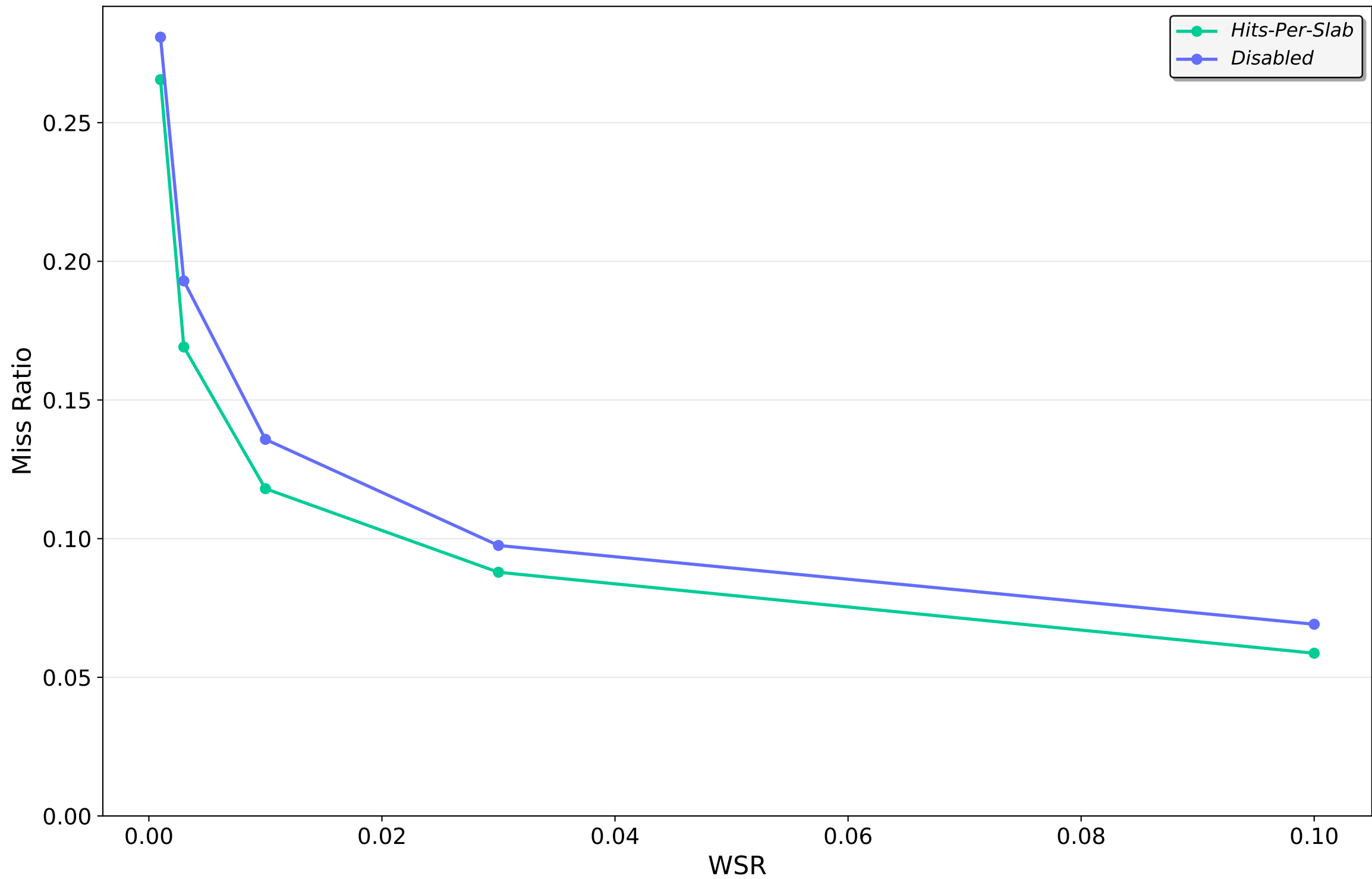
cluster52.oracleGeneral.zst — S3FIFO
