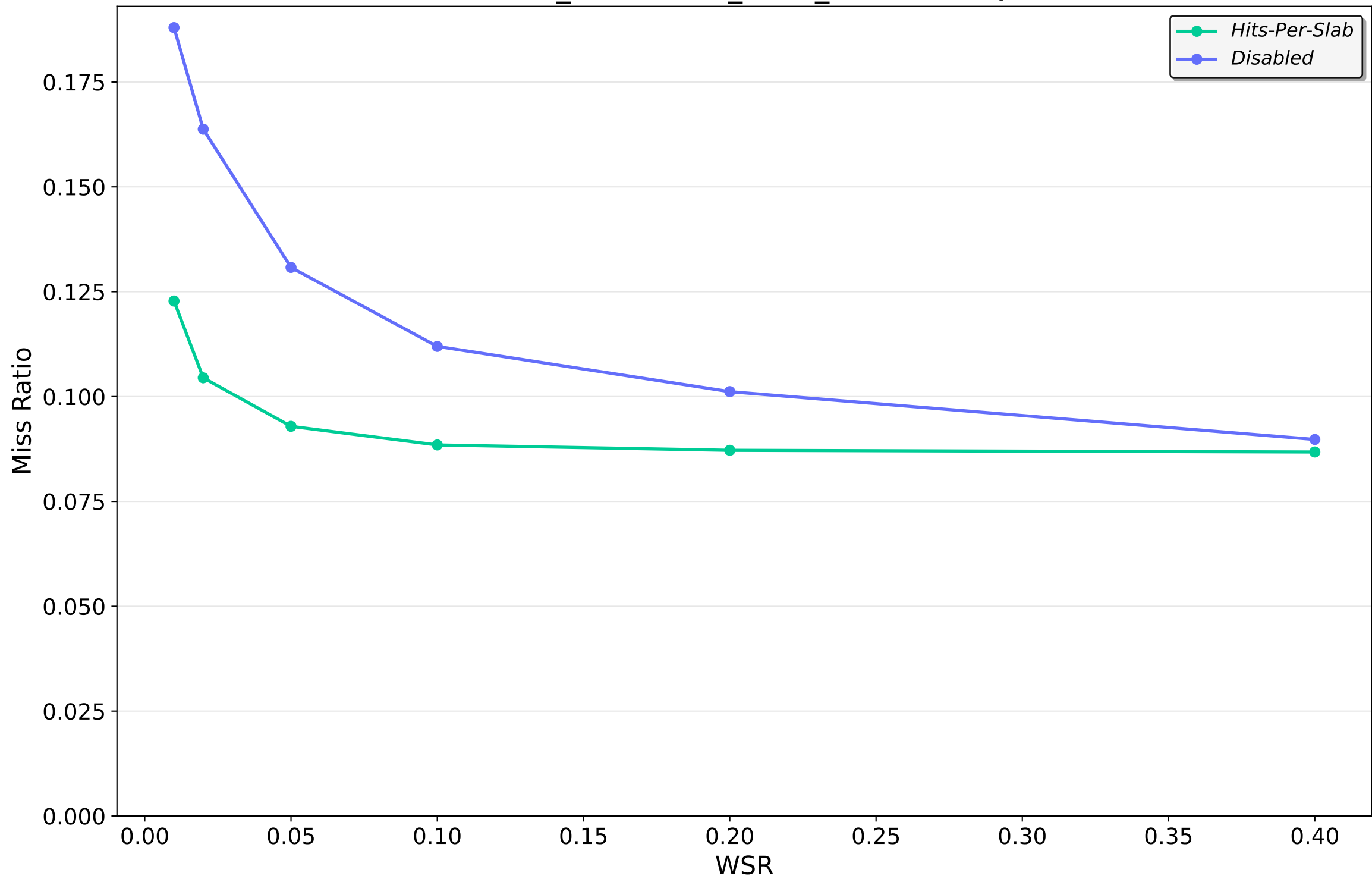
meta_memcache_2024_kv — LRU2Q
