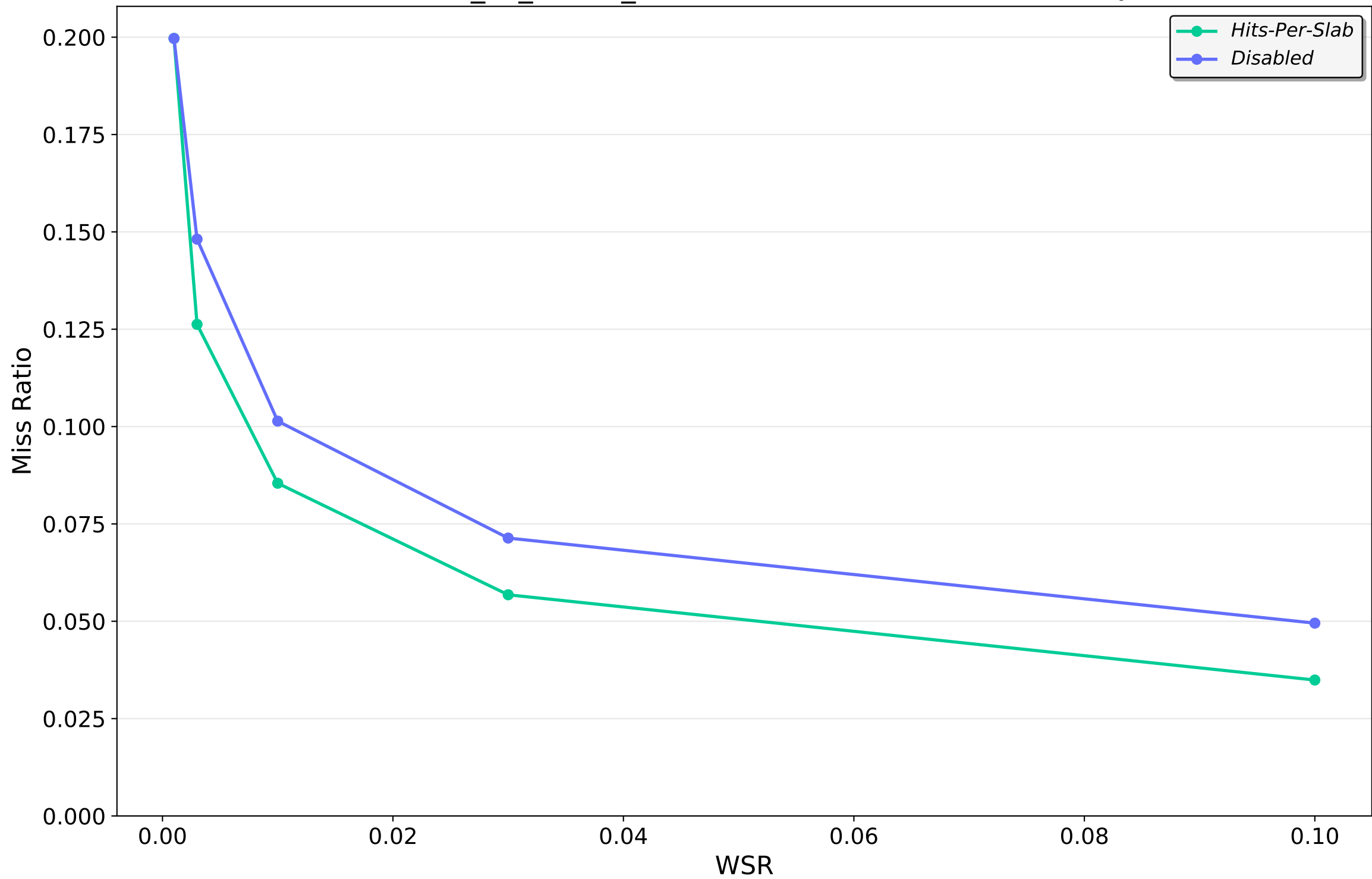
202206_kv_traces_all.csv.oracleGeneral.zst — LRU2Q
