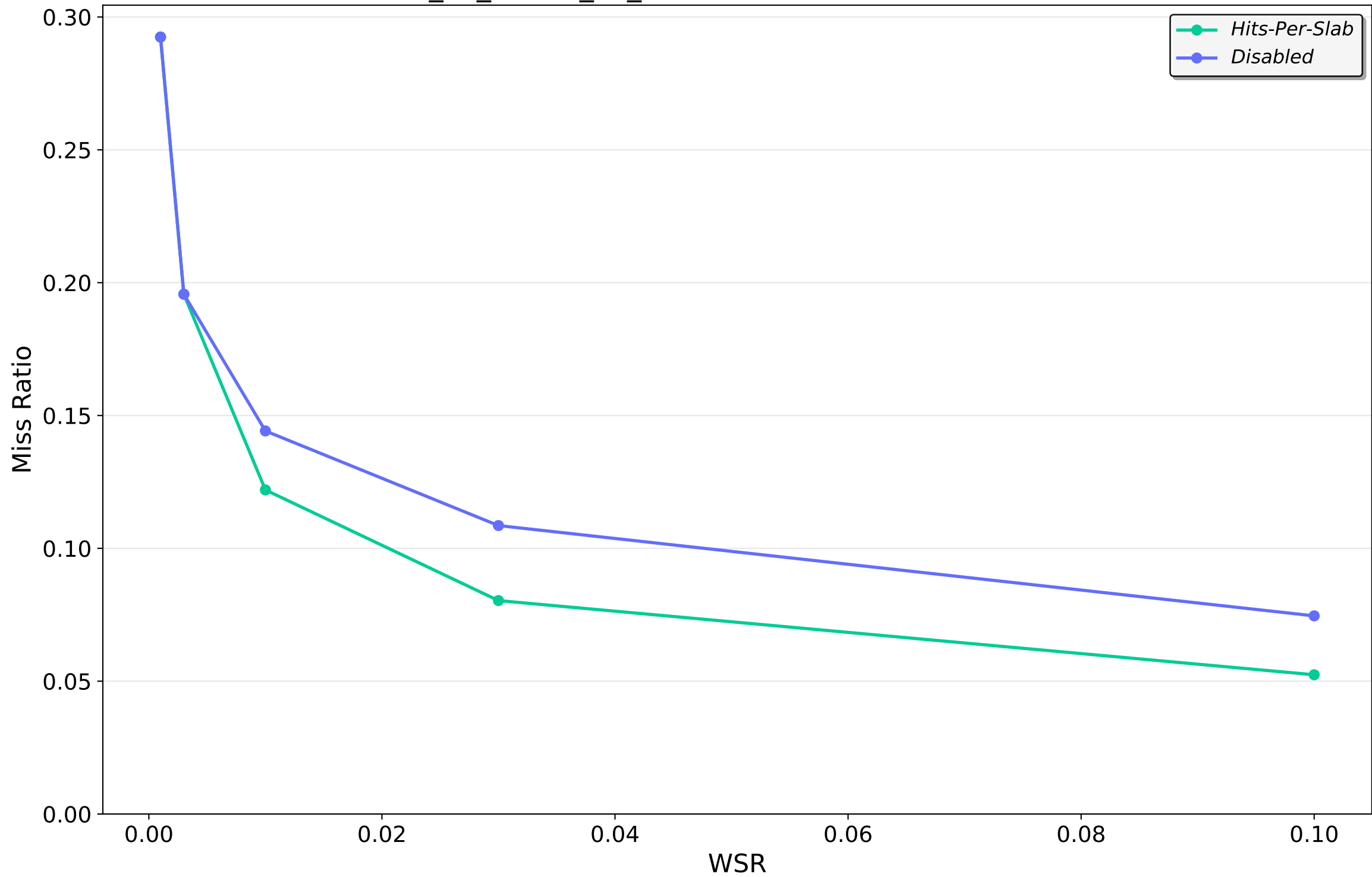
202401_kv_traces_all_sort.csv.oracleGeneral.zst — LRU2Q
