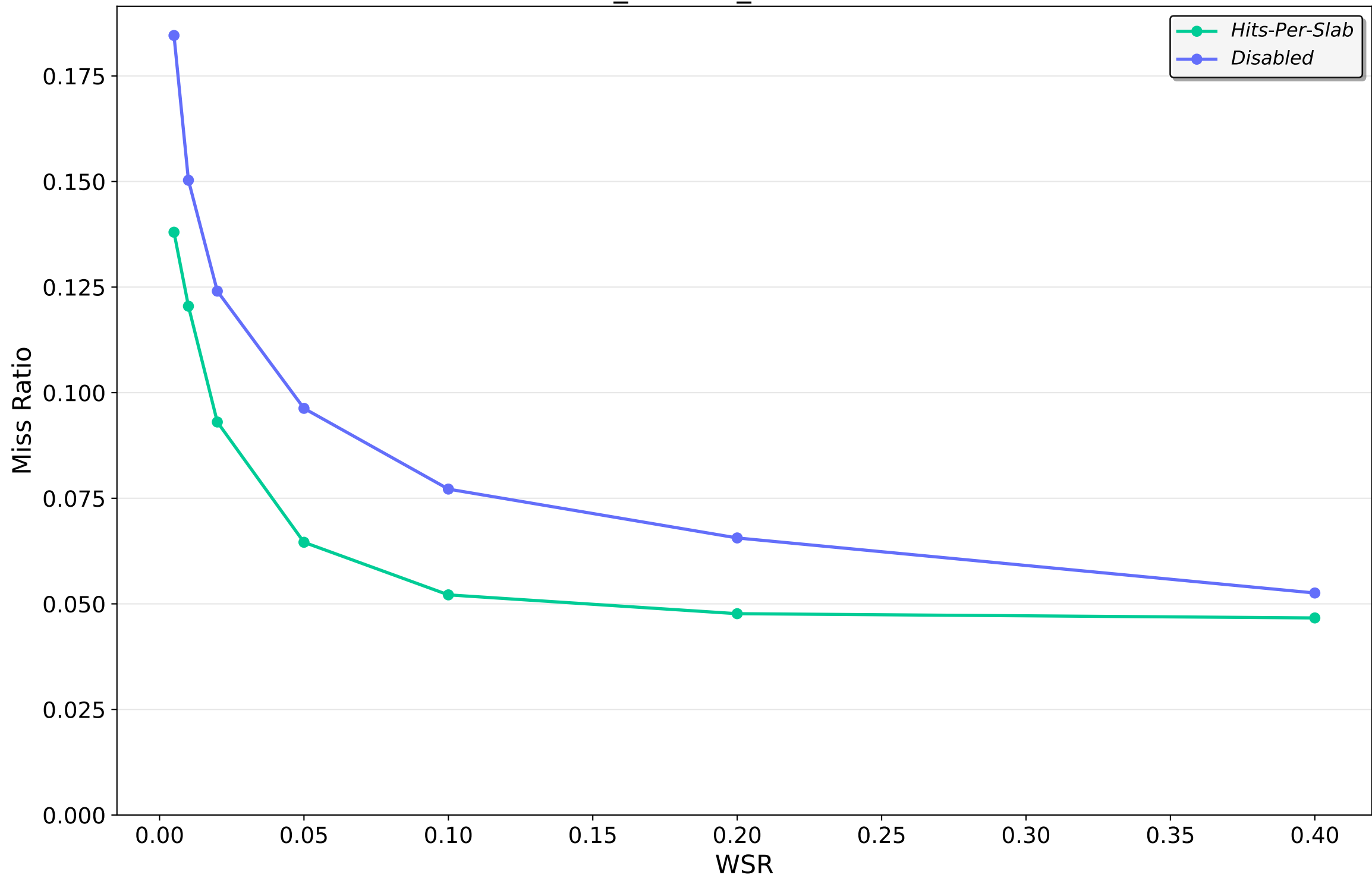
meta_202401_kv — TINYLFU
