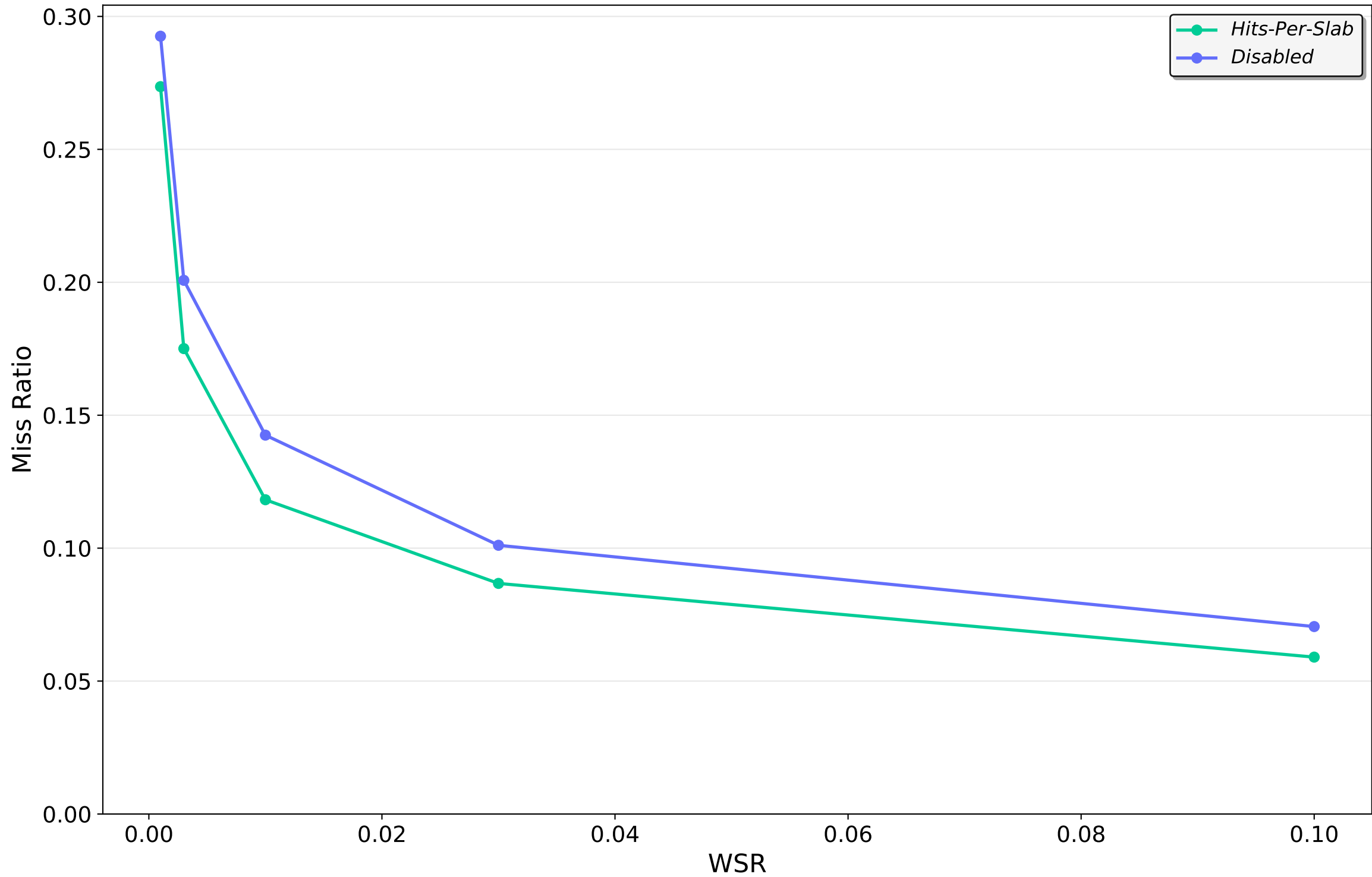
cluster52.oracleGeneral.zst — TINYLFU
