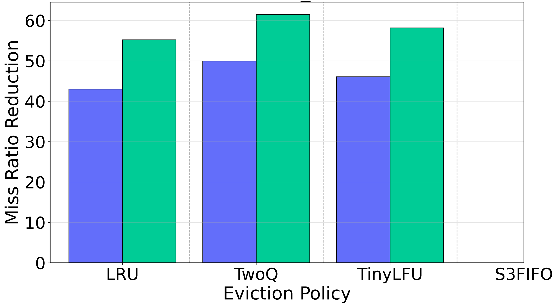
Trace: twitter_cluster14
