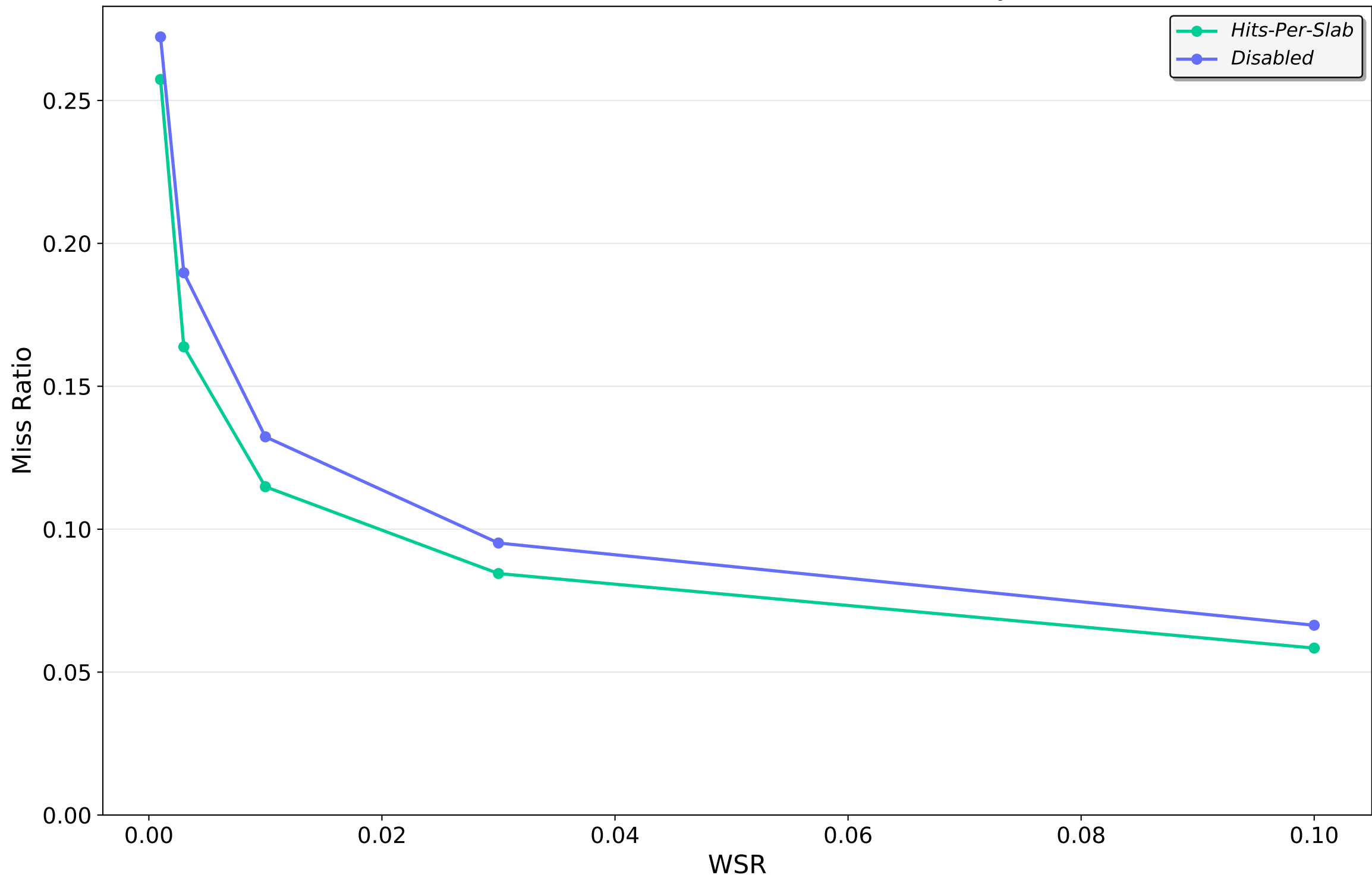
cluster52.oracleGeneral.zst — LRU2Q
