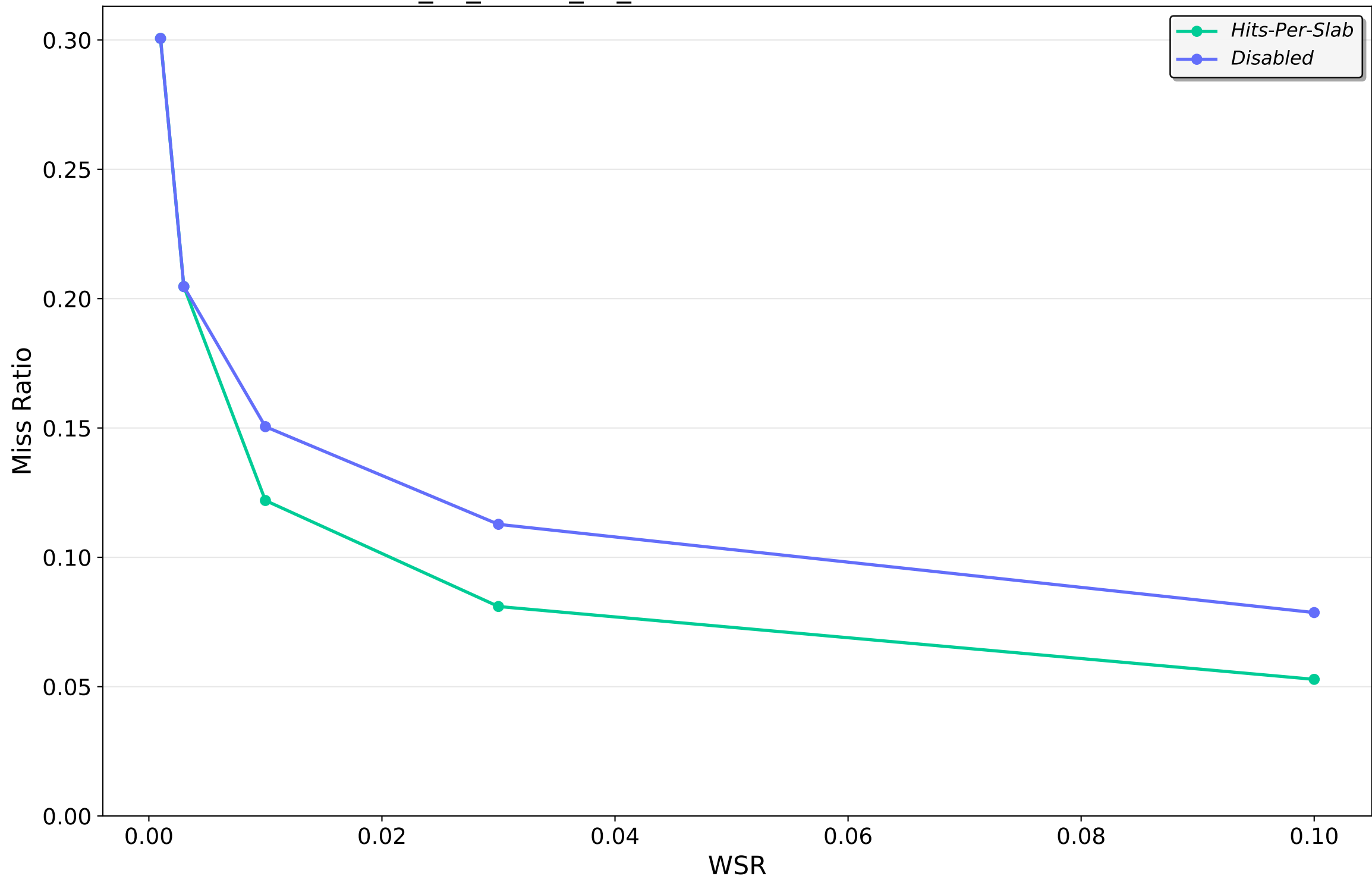
202401_kv_traces_all_sort.csv.oracleGeneral.zst — TINYLFU
