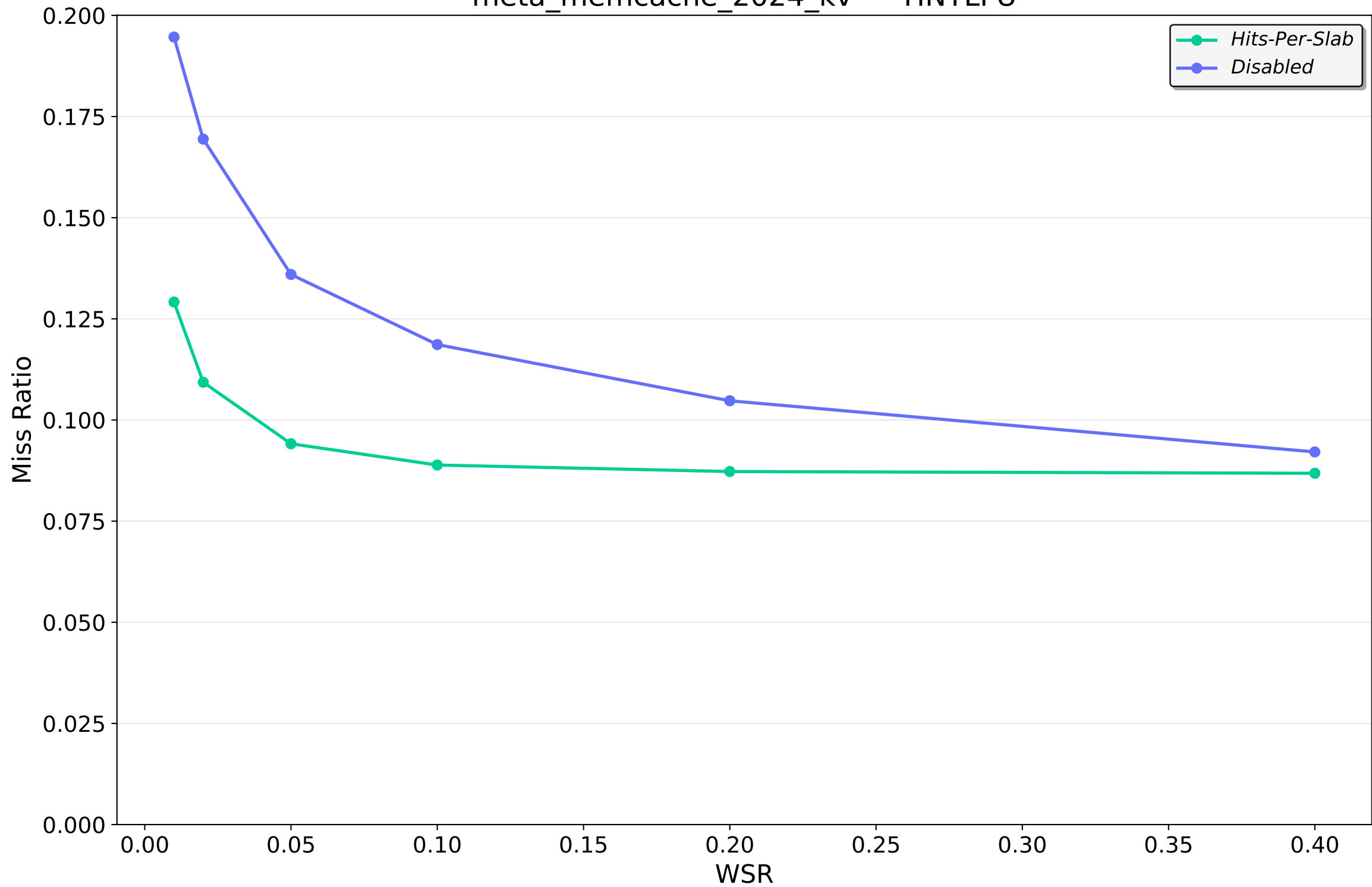
meta_memcache_2024_kv — TINYLFU
