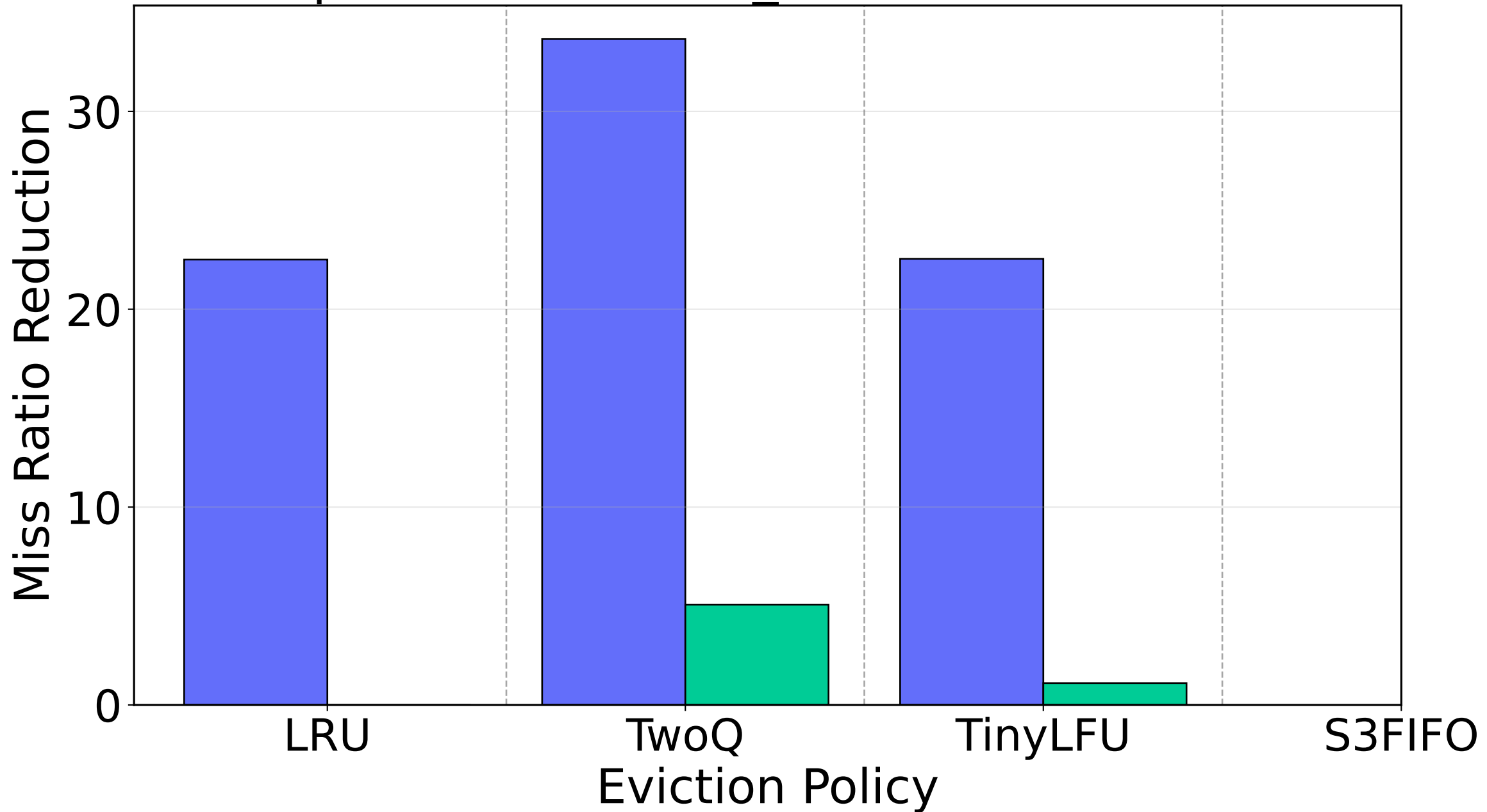
Paper Trace: twitter_cluster25, WSR: 0.1
