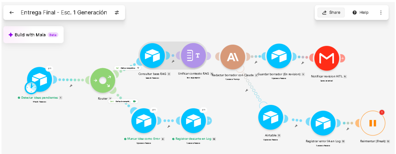
Figura 6. Escenario 1 completo: trigger, router con dos rutas filtradas, pipeline RAG → Claude → Airtable → Gmail y error handler con directiva Retry (Break). Nodos nombrados por función.
