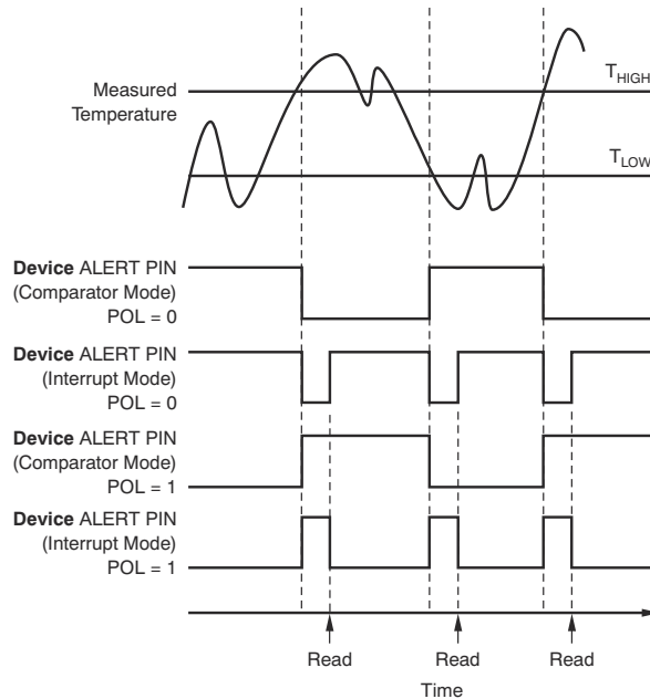
图 6-7. Output Transfer Function Diagrams
