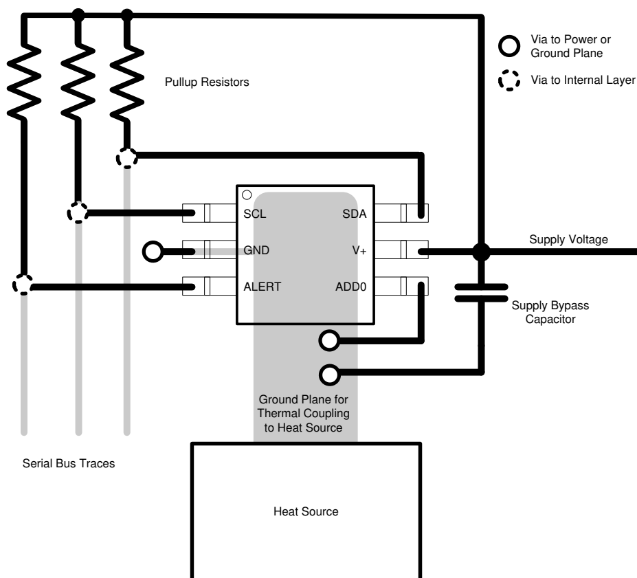
图 7-4. TMP102 Layout Example
