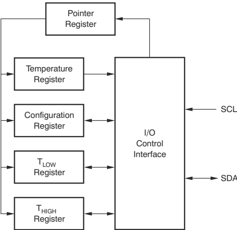
图 6-6. Internal Register Structure
