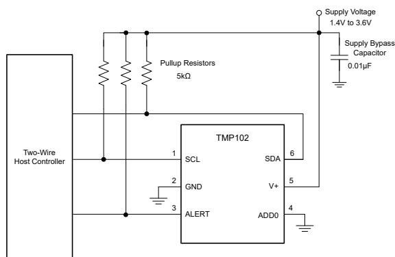
简化原理图
