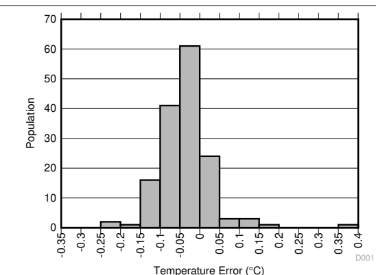
图 5-6. Temperature Error at 25°C
