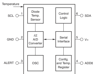
方框图
