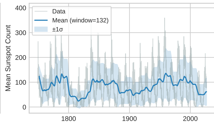
(d) SILSO Sunspots
