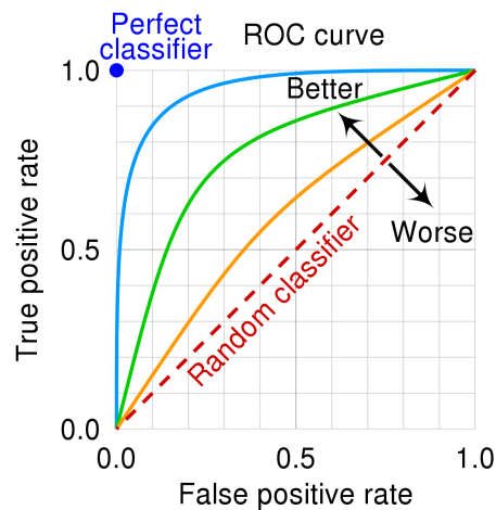
Figure 2.10: Une courbe ROC. La performance d'un modèle naïf (aléatoire) est indiquée en pointillés. Plus la courbe tend à épouser les axes supérieurs gauches, plus le modèle est performant
