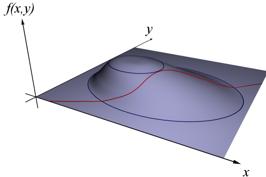
Figure 3.16: Illustration 3D de la méthode des multiplicateurs de Lagrange. Sur cette figure, il s'agit de trouver le point le plus élevé possible, tout en satisfaisant la contrainte d'être sur la ligne rouge.
