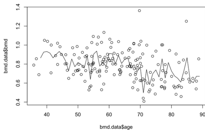
Figure 3.6: Utilisation de KNN en régression. Source bookdown.org
