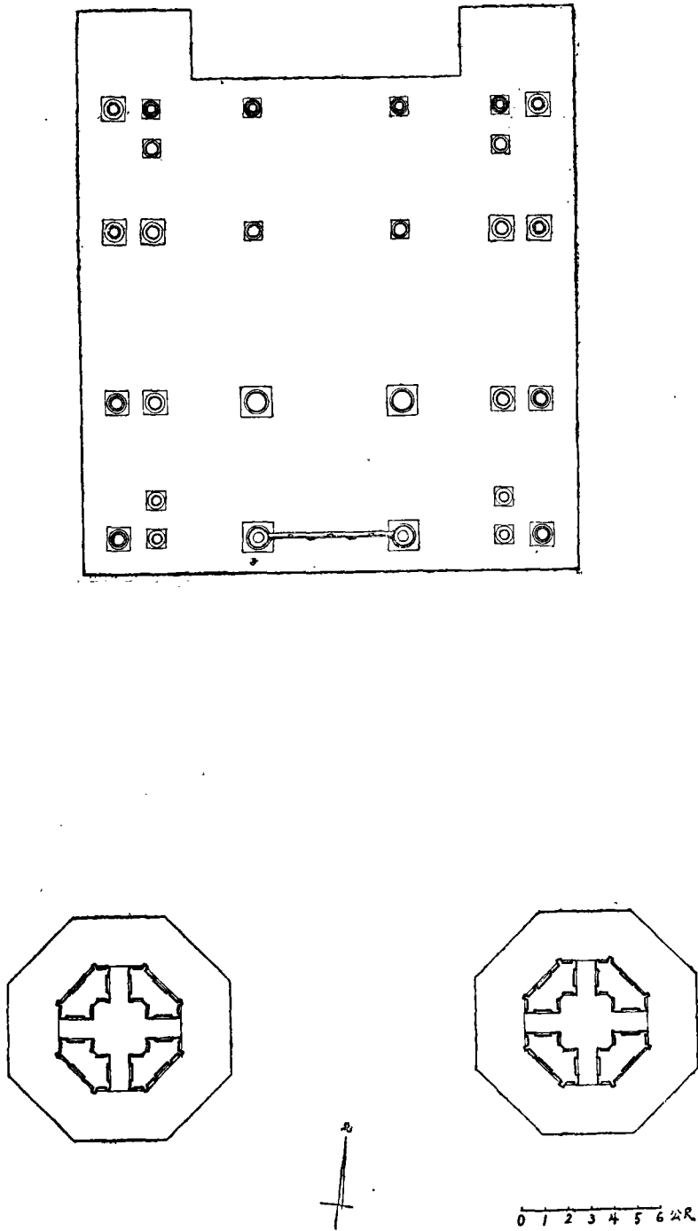
蘇州羅漢院双塔暨正殿遺址平面图
