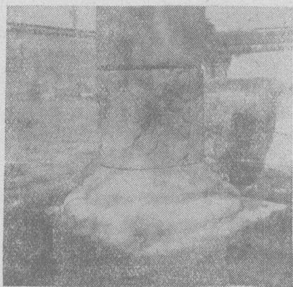
圖十 罗汉院正殿石柱及柱础
