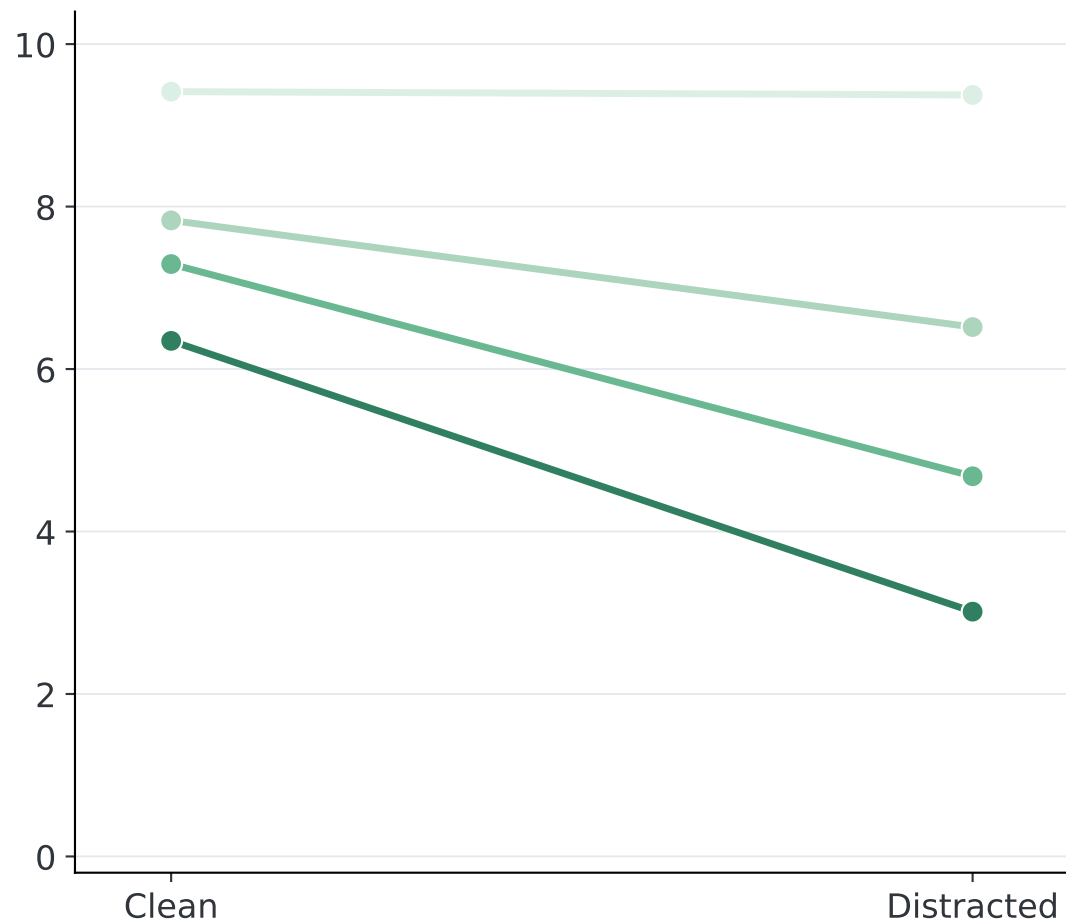
(b) CPB
