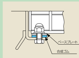
■ ボルト固定式
