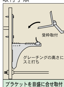
受枠ブラケット 型式UWH
