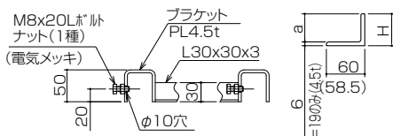
スペーサー詳細
