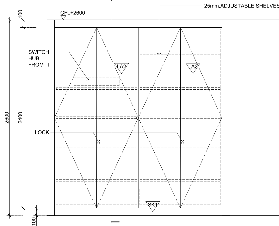
ELEVATION 1 Scale: 1:25
