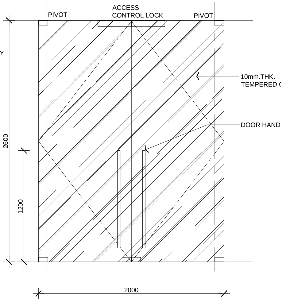
D1 ELEVATION Scale: 1:25
