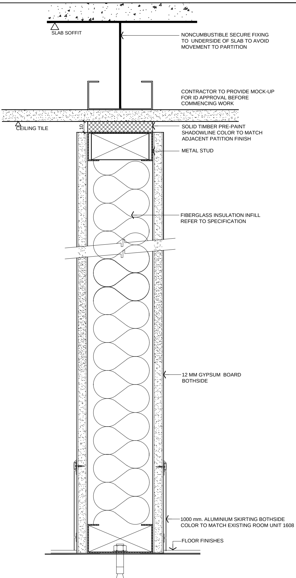
P2 DETAIL - DRYWALL PARTITION-SINGLE LAYER Scale: N.T.S.
