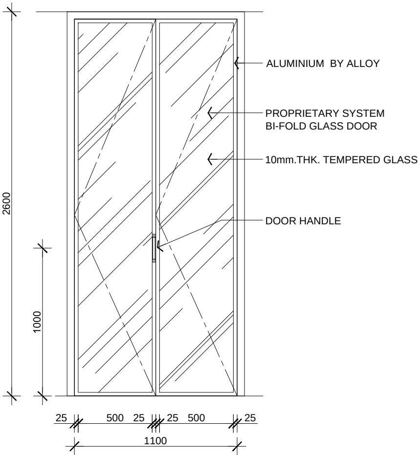
D6 ELEVATION Scale: 1:25
