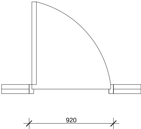
D7 PLAN Scale: 1:25
