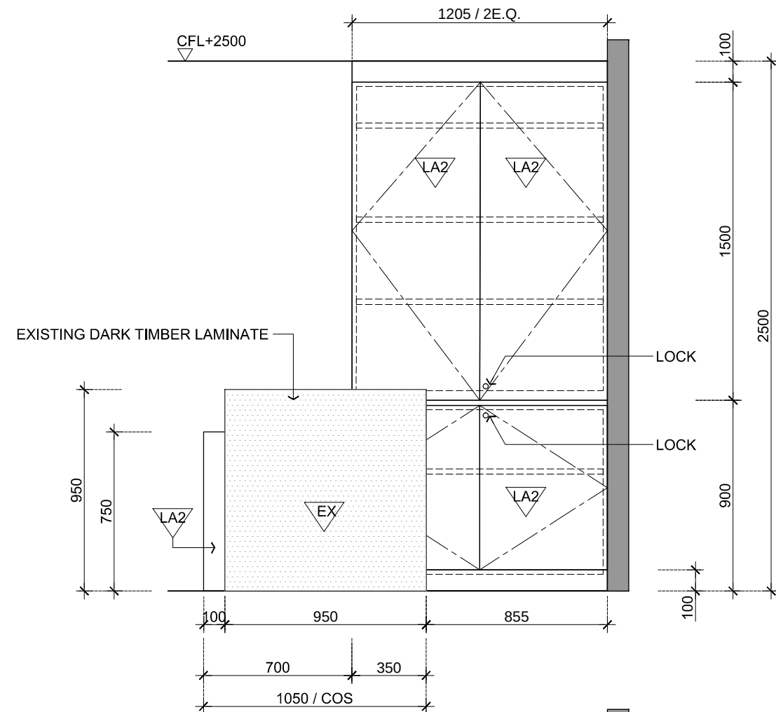
ELEVATION 3 Scale: 1:25
