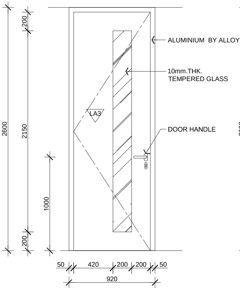
D7 ELEVATION Scale: 1:25
