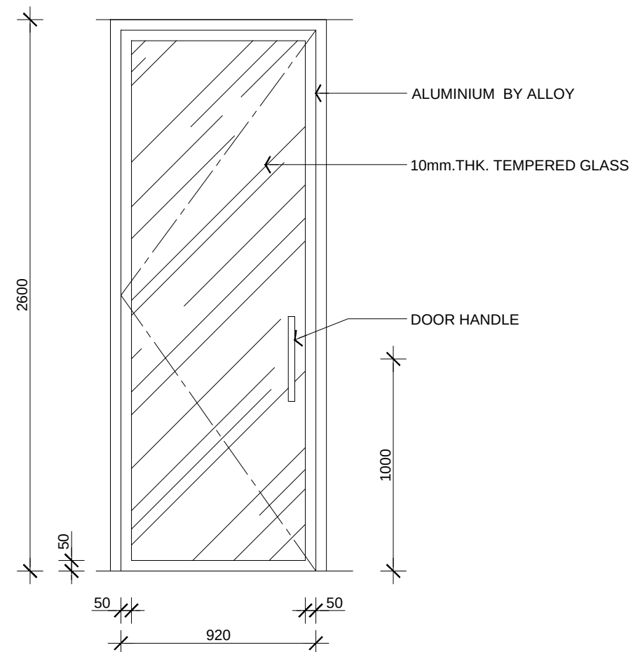
D2 ELEVATION Scale: 1:25
