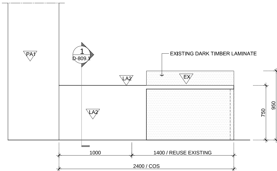
ELEVATION 1 Scale: 1:25
