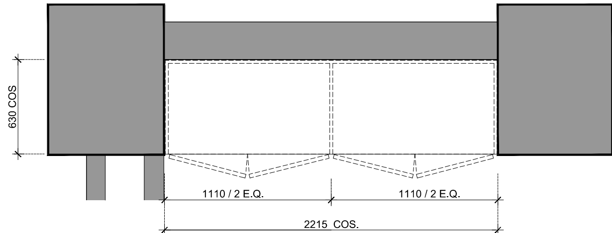
PLAN JU-14 Scale: 1:25
