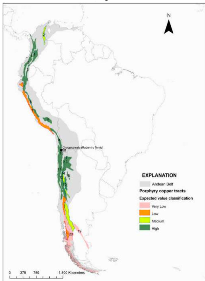
Figura 1. Mapa de distribución de tramos de interés para depósitos de cobre tipo pórfido a lo largo de la cordillera de los Andes en Suramérica, según clasificaciones de valor 3 .
