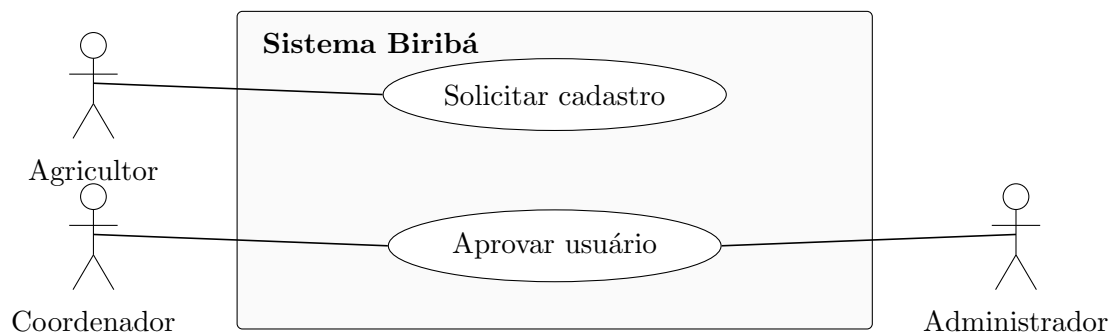
Figura A.1: Diagrama UML dos casos de uso de acesso ao sistema
