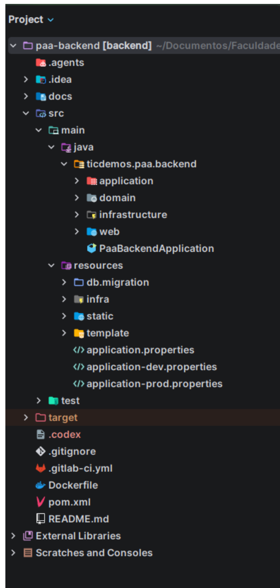
Figura 4.3: Estrutura de diretórios do backend
