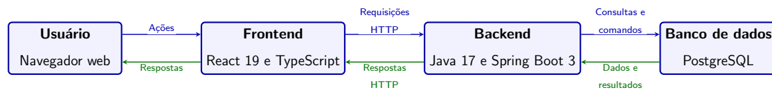
Figura 4.2: Comunicação entre os módulos da arquitetura do sistema Biribá
