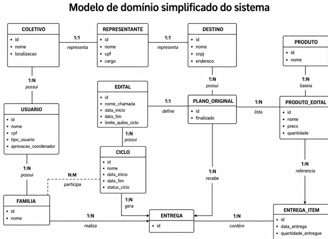
Figura 4.1: Modelo de domínio simplificado do sistema
