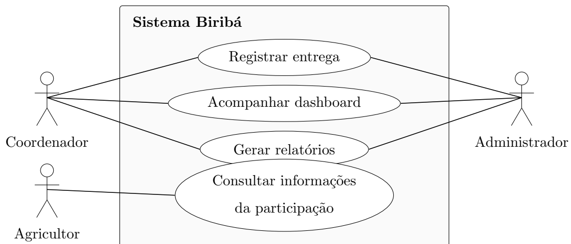
Figura A.3: Diagrama UML dos casos de uso de execução e acompanhamento
