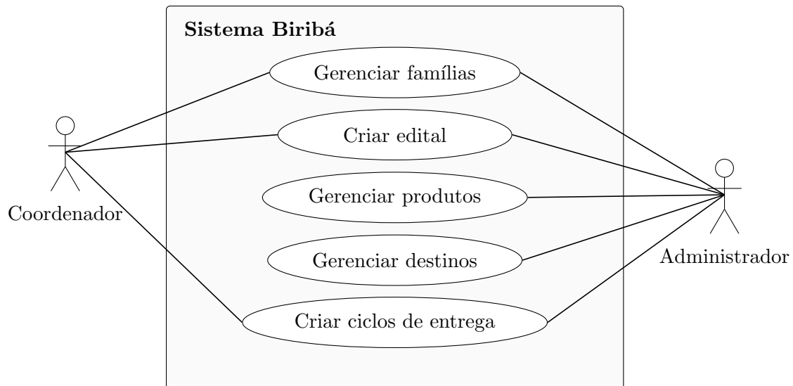
Figura A.2: Diagrama UML dos casos de uso de configuração do edital
