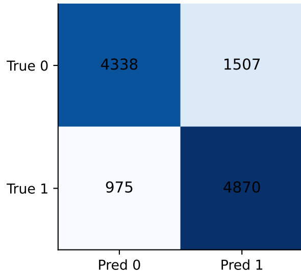
k-mer LR
