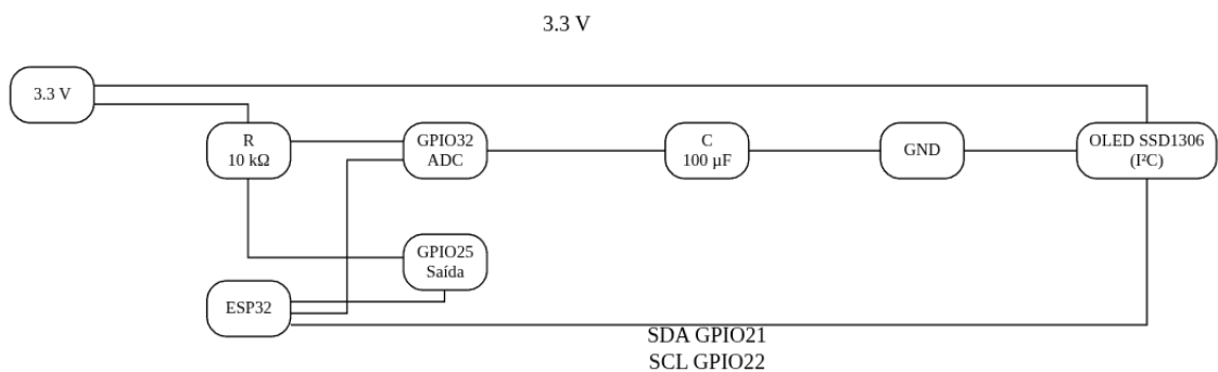
Figura 3 – Diagrama de montagem elétrica
