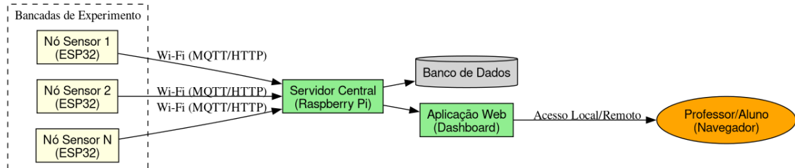
Figura 2 – Arquitetura Proposta
