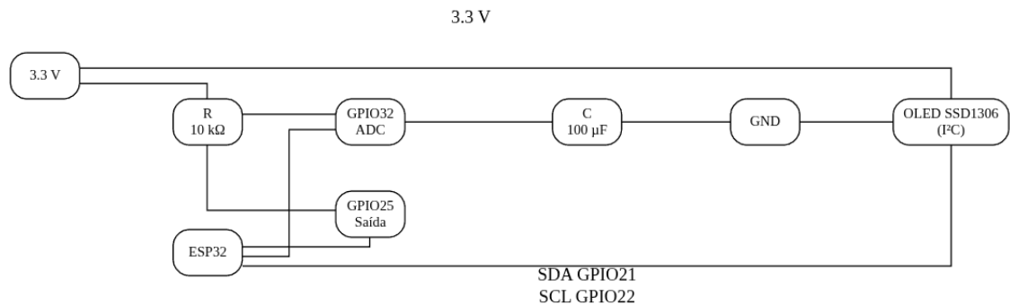
Figura 2 – Diagrama de montagem elétrica
