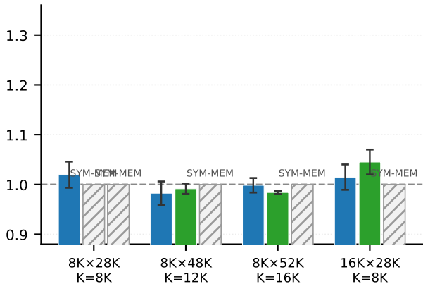
GEMM-AR
