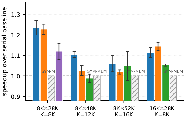
GEMM-RS
