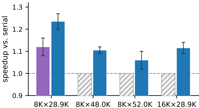
GEMM-RS
