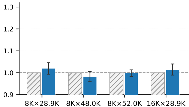
GEMM-AR
