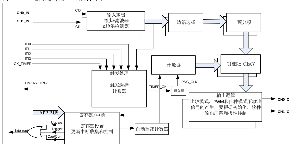
图 16-44. 通用定时器 L1 结构框图
