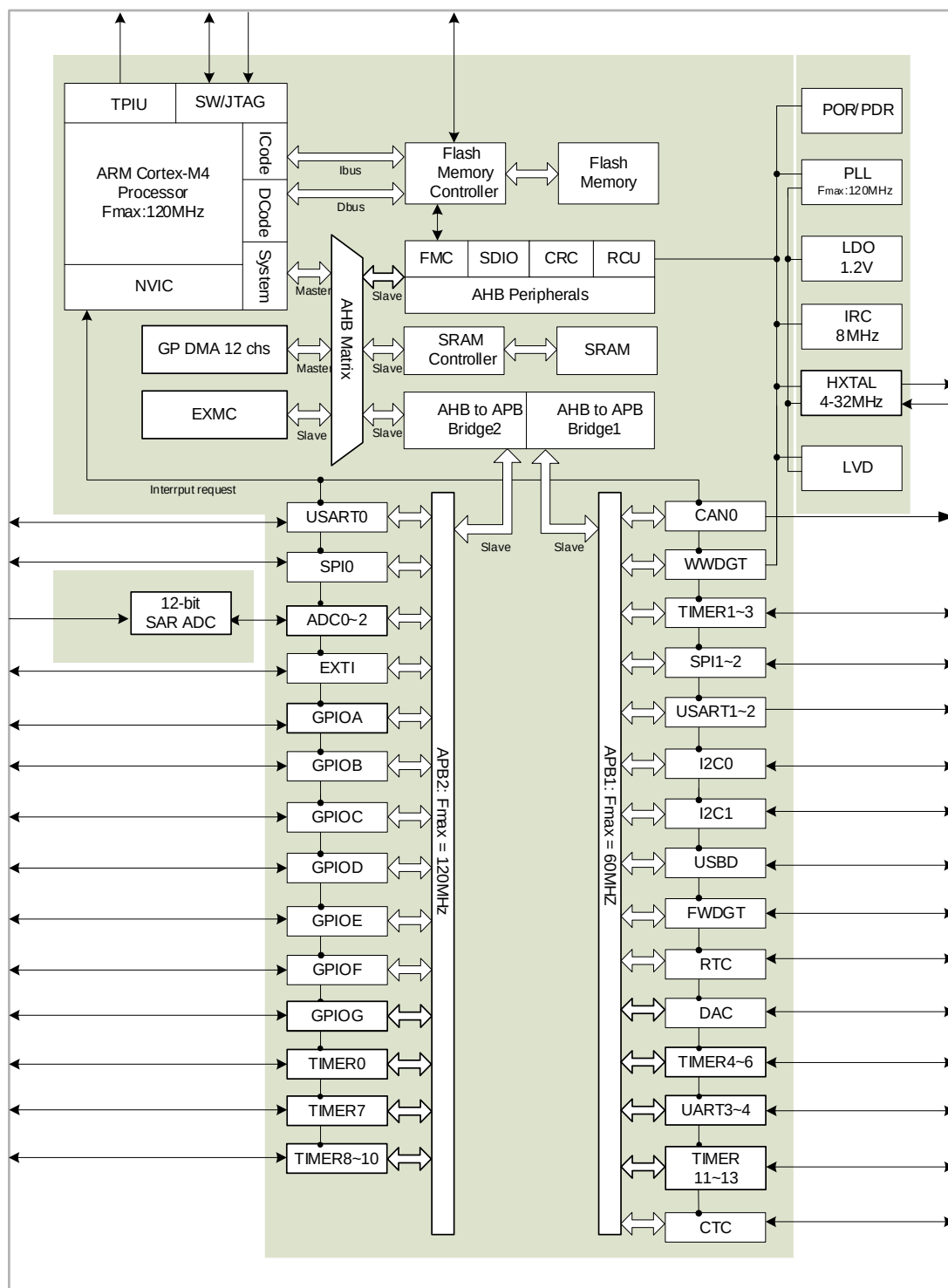
图 1-2. GD32F303 系列的系统架构
