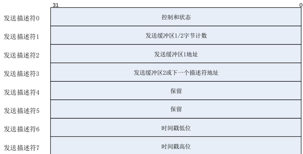
图 23-8. 增强发送描述符
