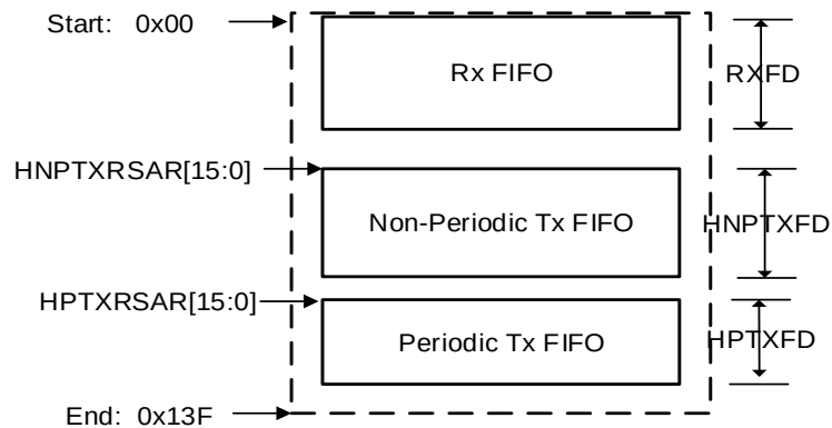
图 25-5. 主机模式 FIFO 空间
