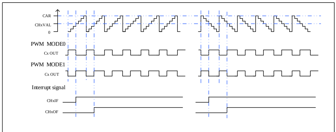
图 16-51. EAPWM 时序图
