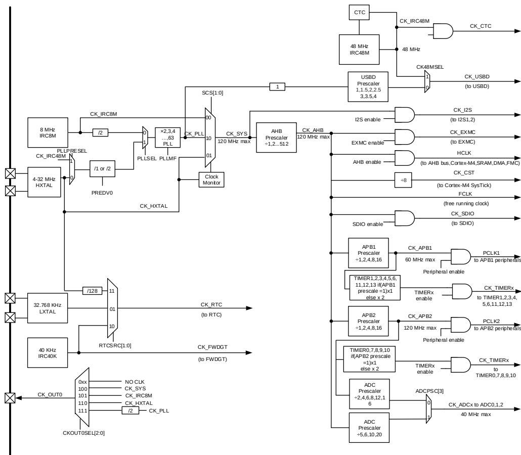
图5-2. 时钟树
