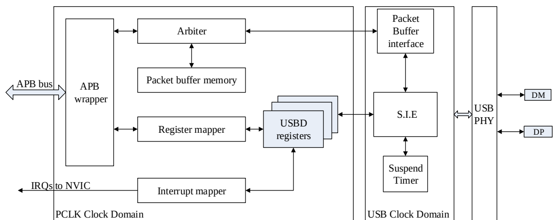
图 24-1. USBD 模块图
