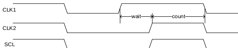
图 18-4. 时钟同步
