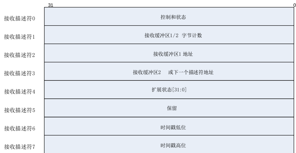
图 23-10. 增强接收描述符
