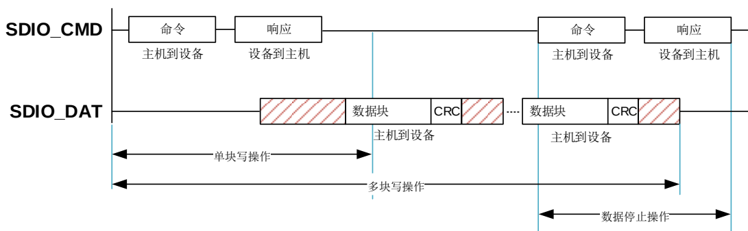
图 20-3. SDIO 多块写操作
