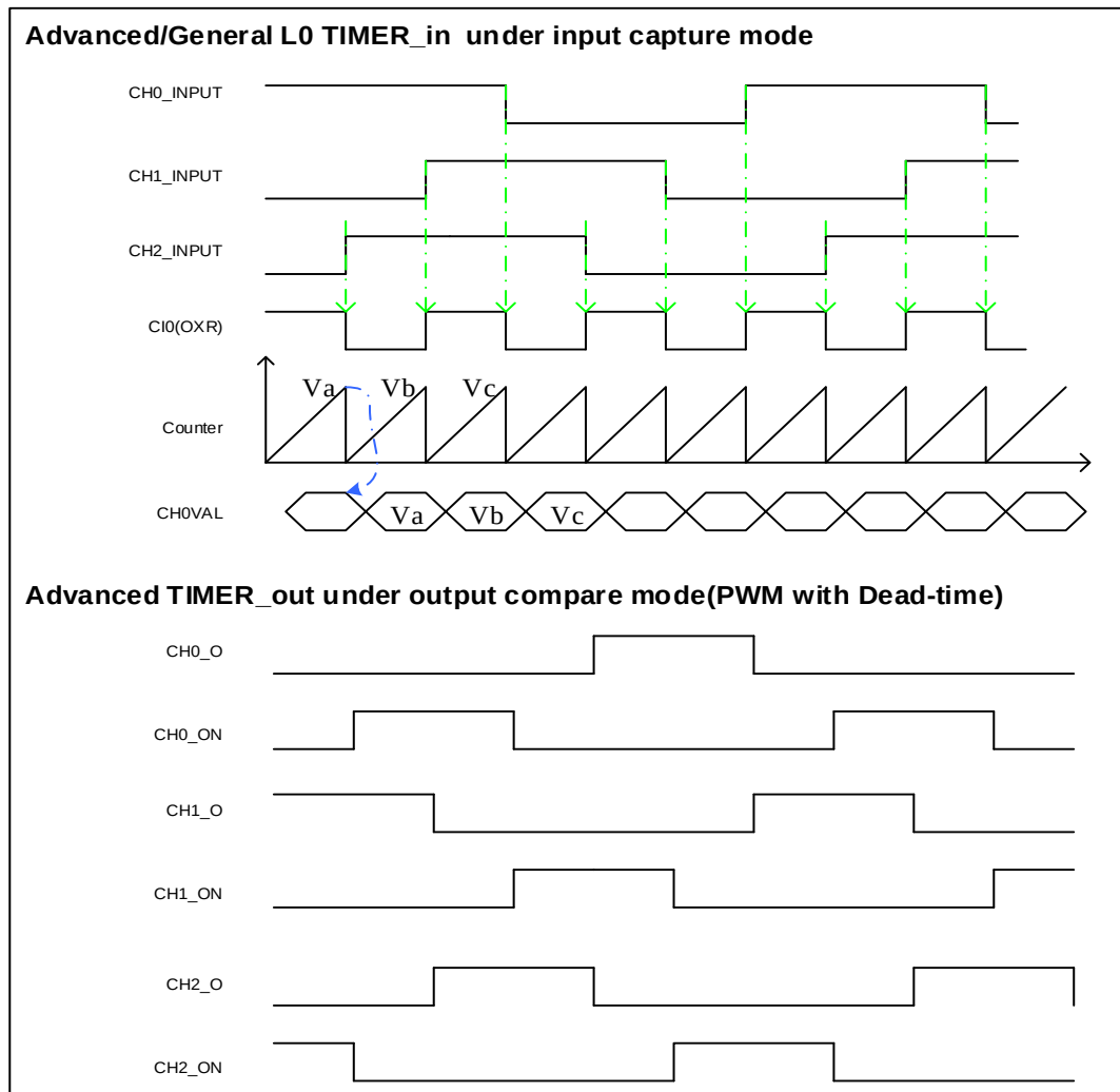
图 16-21. 两个定时器之间的霍尔传感器时序图
