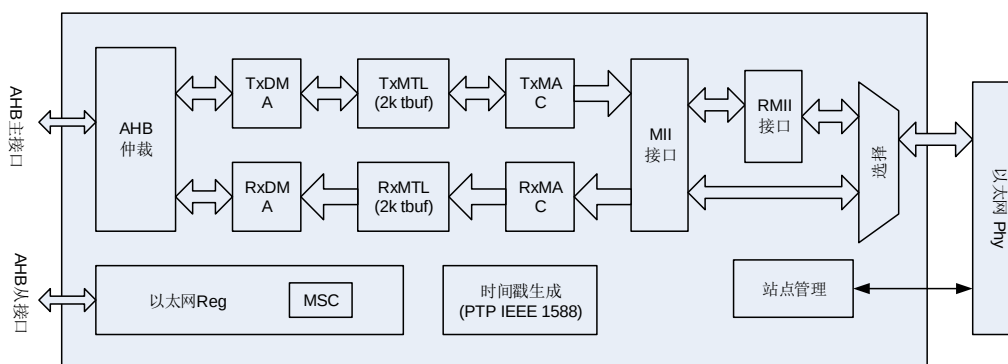
图 23-1. 以太网模块框图
