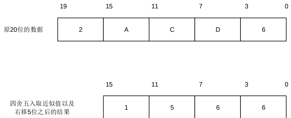
图 12-10. 右移 5 位和取整的数例
