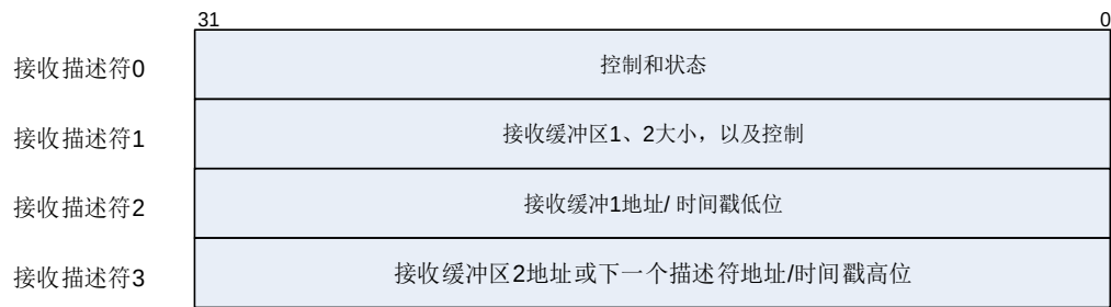
图 23-9. 接收描述符
