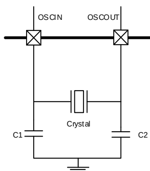
图5-7. HXTAL时钟源
