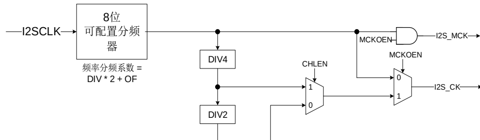
图 19-51. I2S 时钟生成结构框图
