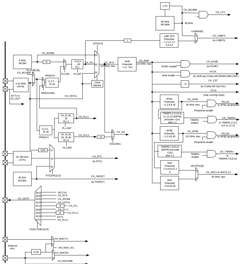
图5-6. 时钟树
