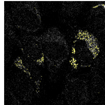
Green puncta: auto 32.4
