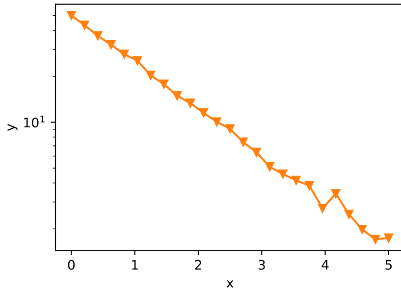
cosine
