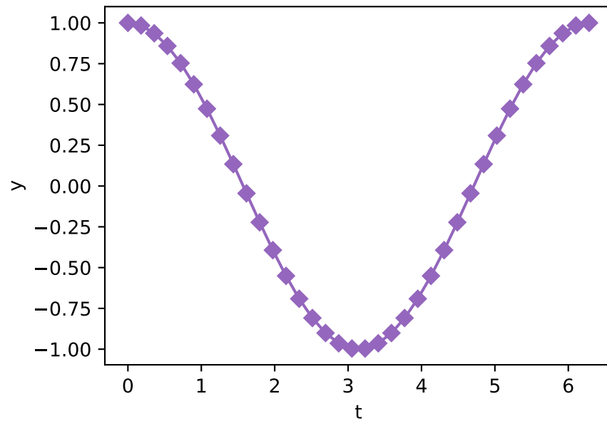
cosine
