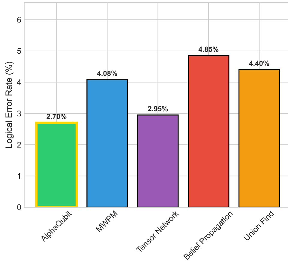
SI1000, p=1.0\% , d=5
