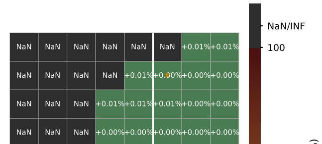
FP8 E4M3
