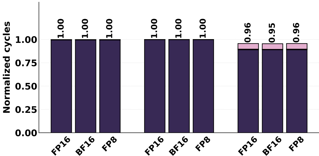
Llama 3.2-1B
