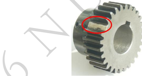
图 1 破损齿轮
