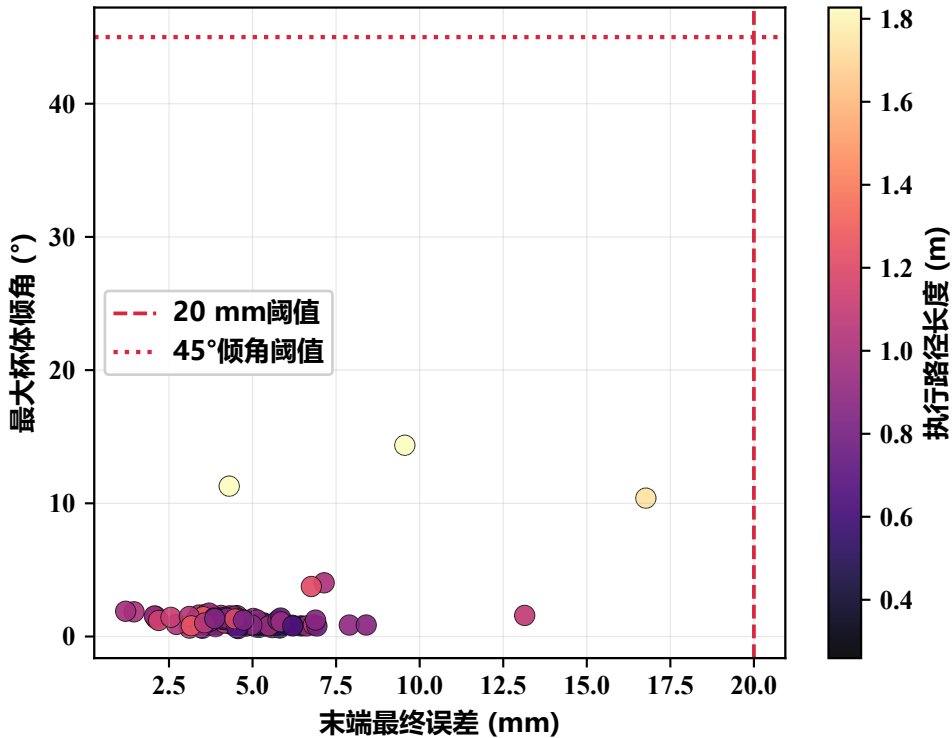
跟踪误差与杯体倾角安全裕度
