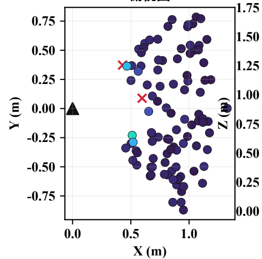
俯视图
