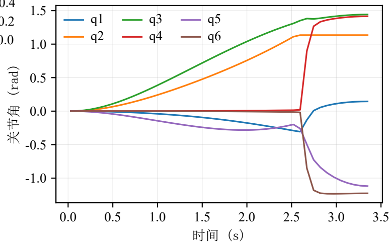
规划关节轨迹
