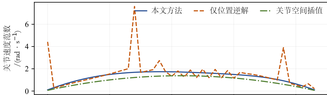
目标点 22 的关节空间顺滑性
