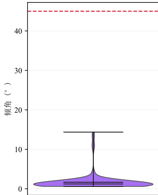
最大倾角分布
