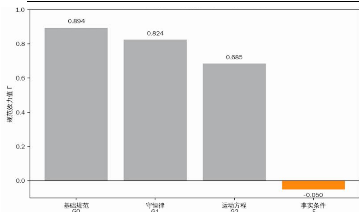
图 1-1 各规范层级规范效力值对比
