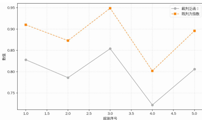
图 3-1 裁判泛函与既判力指数
