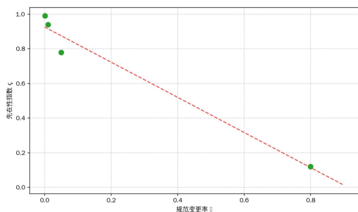
图 1-2 先在性指数与规范变更率关系
