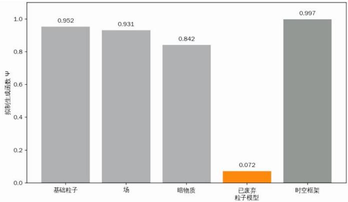
图 2-1 物理实体拟制生成函数对比
