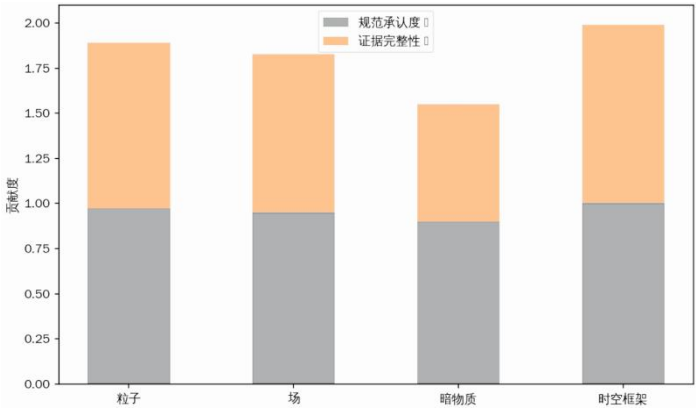
图 2-2 规范承认度与证据完整性堆叠
