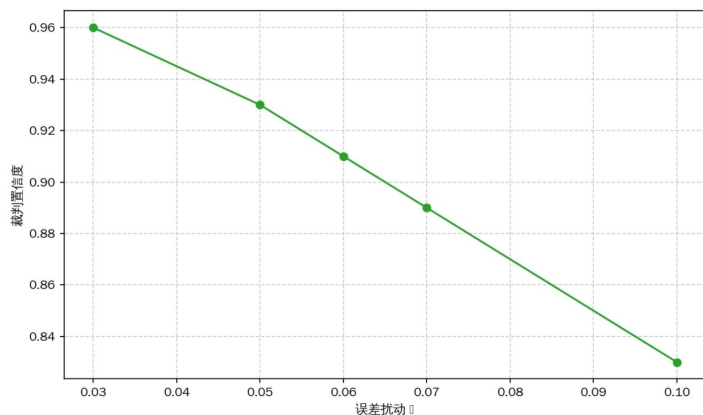
图 3-2 误差扰动对裁判置信度影响
