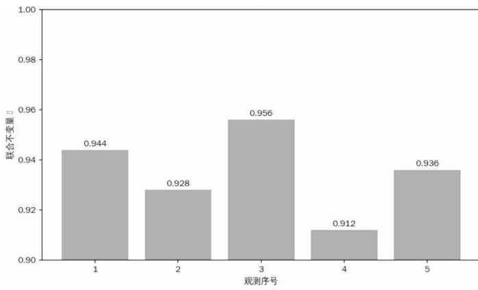
图 4-1 守恒—信赖联合不变量
