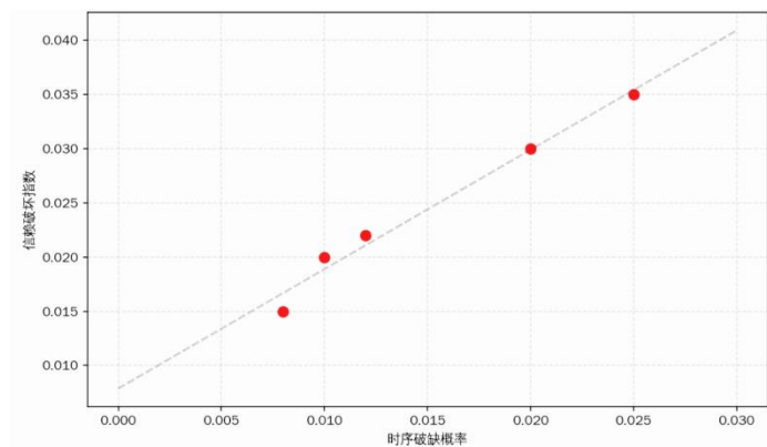
图 4-2 时序破缺概率与信赖破坏指数拟合
