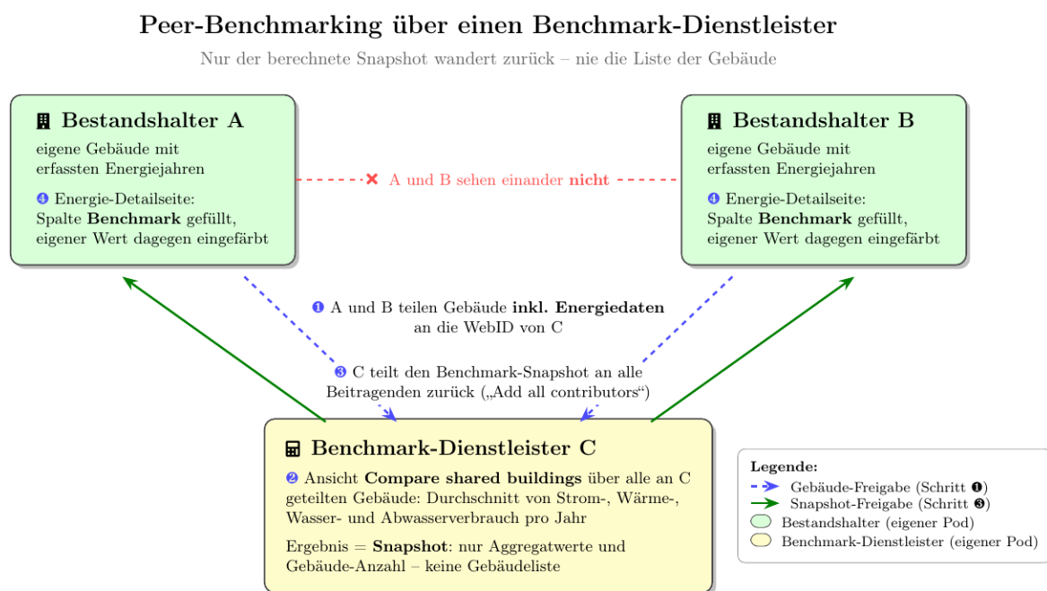
Abbildung 6.5: Der Benchmark-Roundtrip: A und B teilen Gebäude an den Dienstleister C, C berechnet den Durchschnitt und teilt nur den Snapshot zurück
